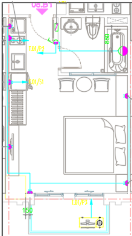
Mặt bằng cấp nguồn ổ cắm cho căn hộ 8-11B1 và 8C1
