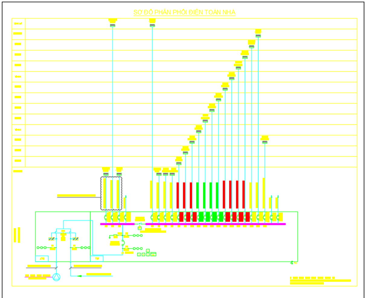
Hình 3.2 Sơ đồ nguyên lý cấp điện cho Tòa nhà 93 Trần Phú
