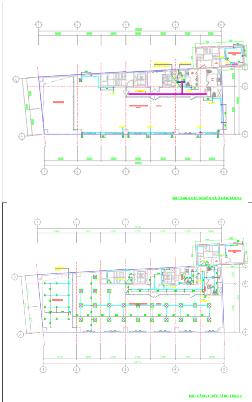
Hình 2.4 Sơ đồ mặt bằng tầng 2
