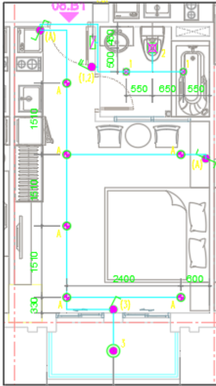
Mặt bằng chiếu sáng cho căn hộ 8-11B1 và 8C1
