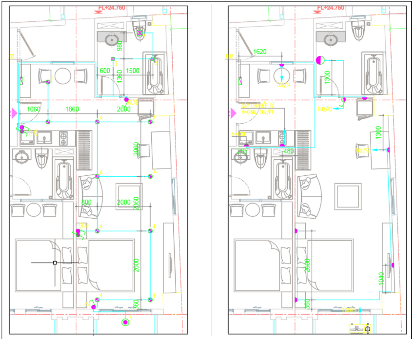
Mặt bằng chiếu sáng và cấp nguồn ổ cắm cho căn hộ 8-11B2
