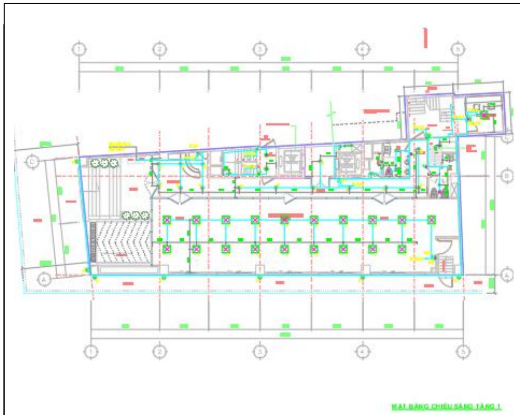
Hình 2.2 Sơ đồ mặt bằng tầng 1
