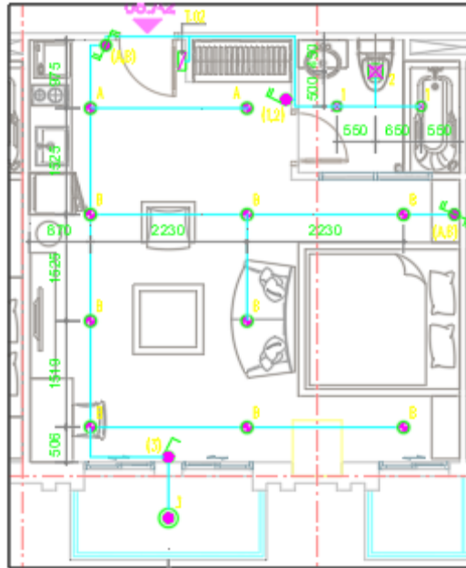
Mặt bằng chiếu sáng căn hộ 8-11A2, 8-11A3
