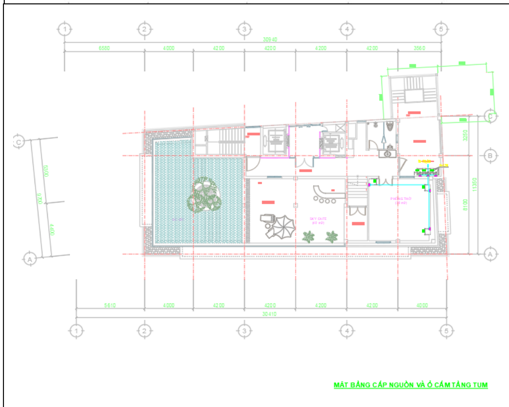
Hình 2.10 Sơ đồ mặt bằng tầng tum
