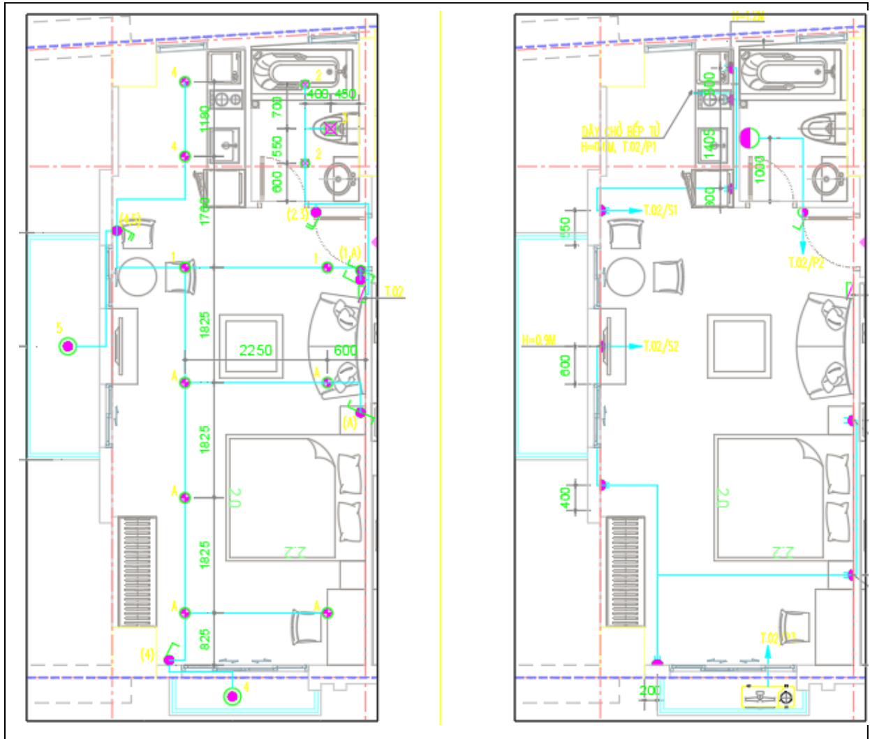
Mặt bằng chiếu sáng và cấp nguồn ổ cắm căn hộ 9-11A1
