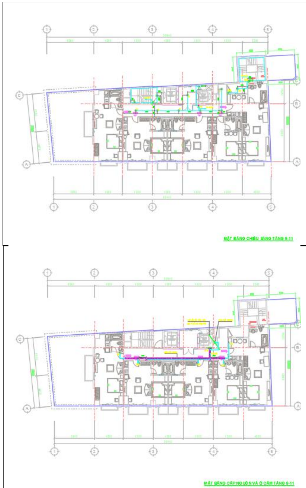
Hình 2.8 So đồ mặt bằng tầng 9-11
