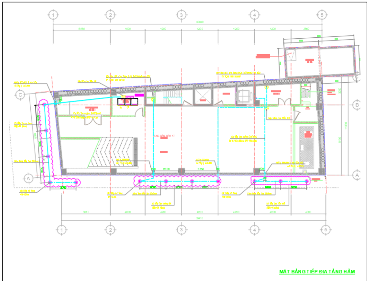
Hình 5.2 Mặt bằng bố trí cọc tiếp địa
