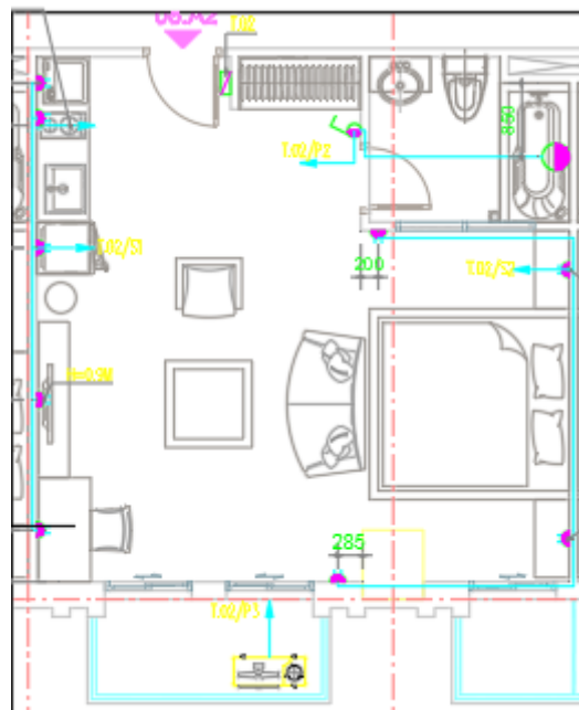
Mặt bằng cấp nguồn ổ cắm căn hộ 8-11A2, 8-11A3
