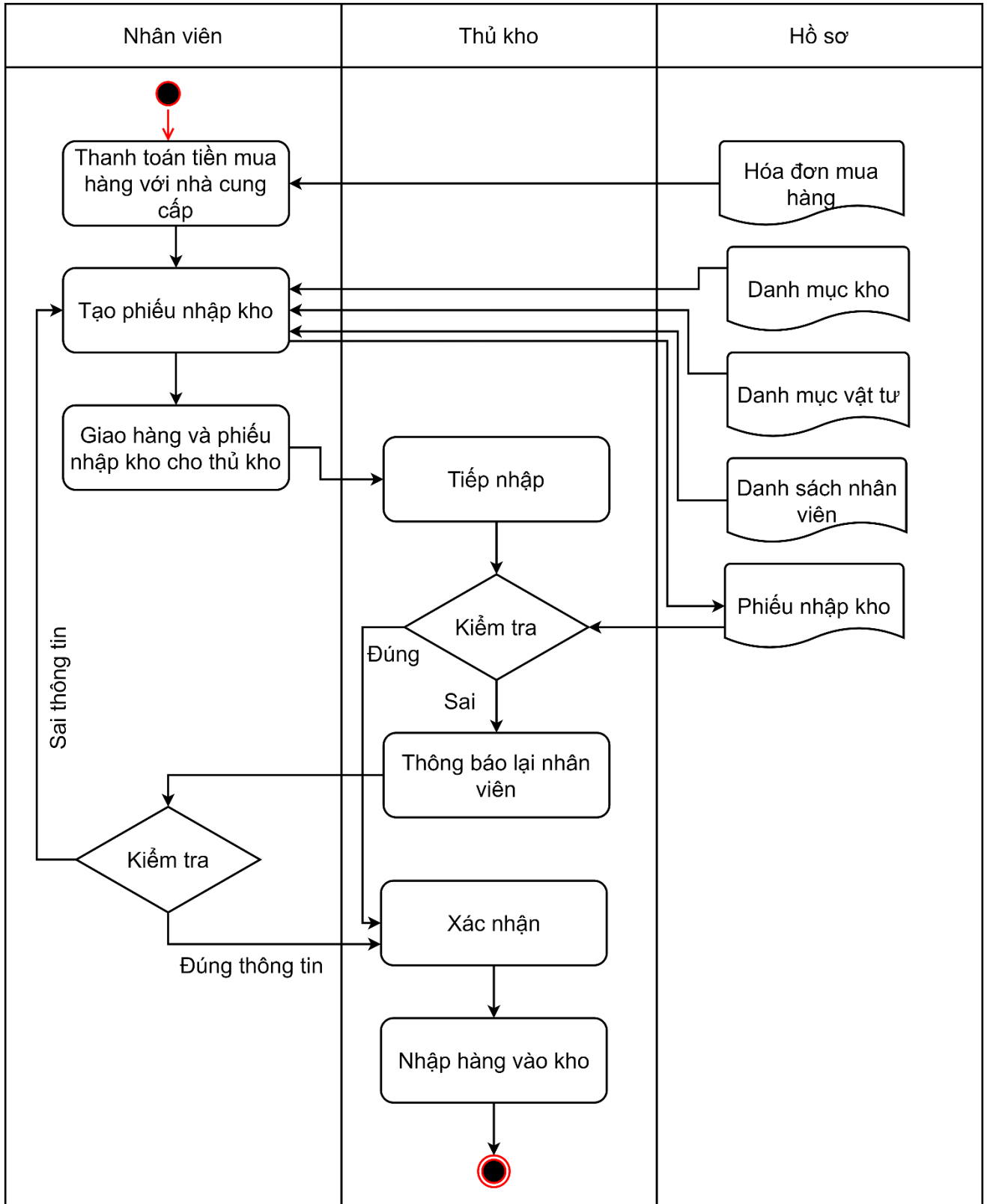
Hình 1. 2: Sơ đồ tiến trình nghiệp vụ “nhập hàng”
