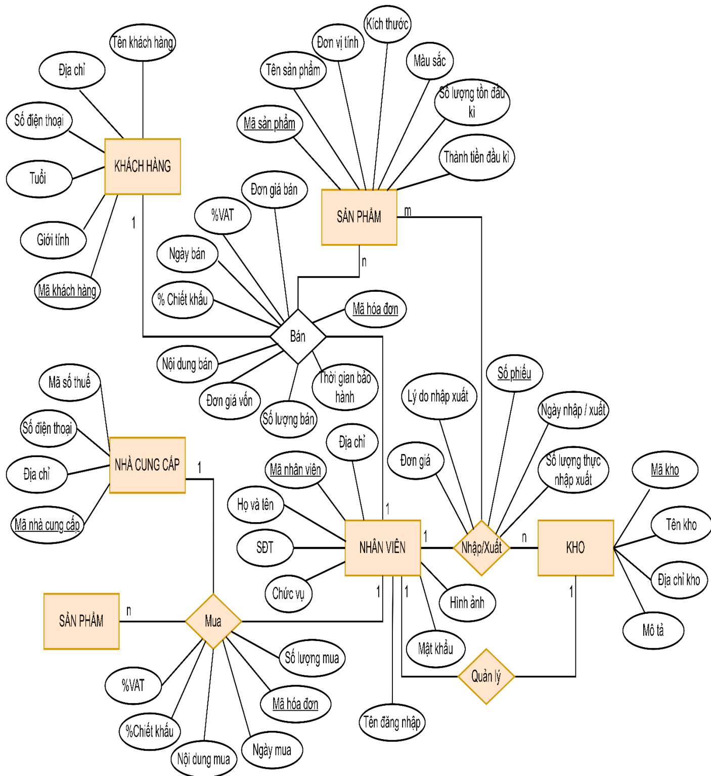
Hình 2. 14: Mô liên kết thực thể hình ER.
