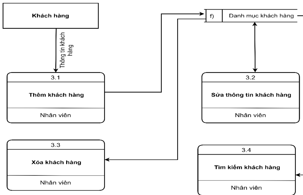
Hình 2. 6: Biểu đồ dữ liệu mức 1 chức năng xem khách hàng.
