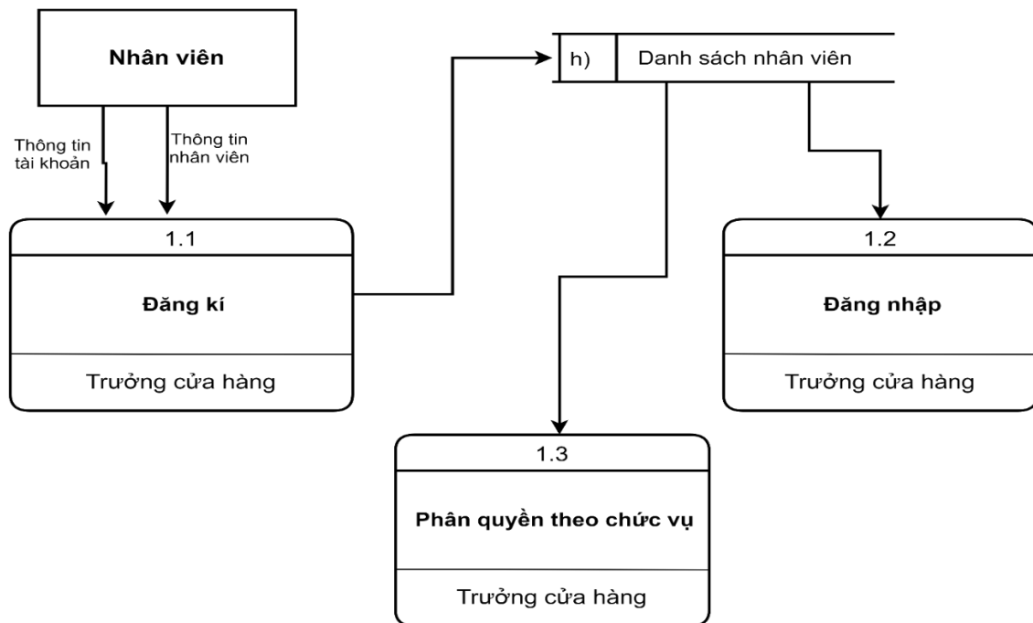
Hình 2. 4: Biểu đồ dữ liệu mức 1 chức năng phân quyền.
