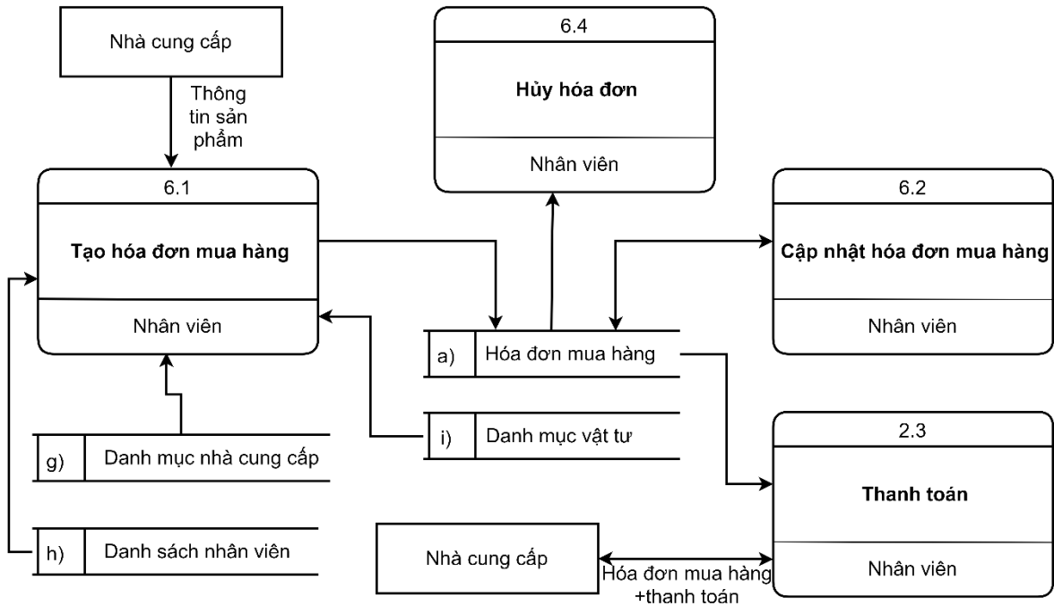
Hình 2. 9: Biểu đồ dữ liệu mức 1 chức năng mua hàng.
