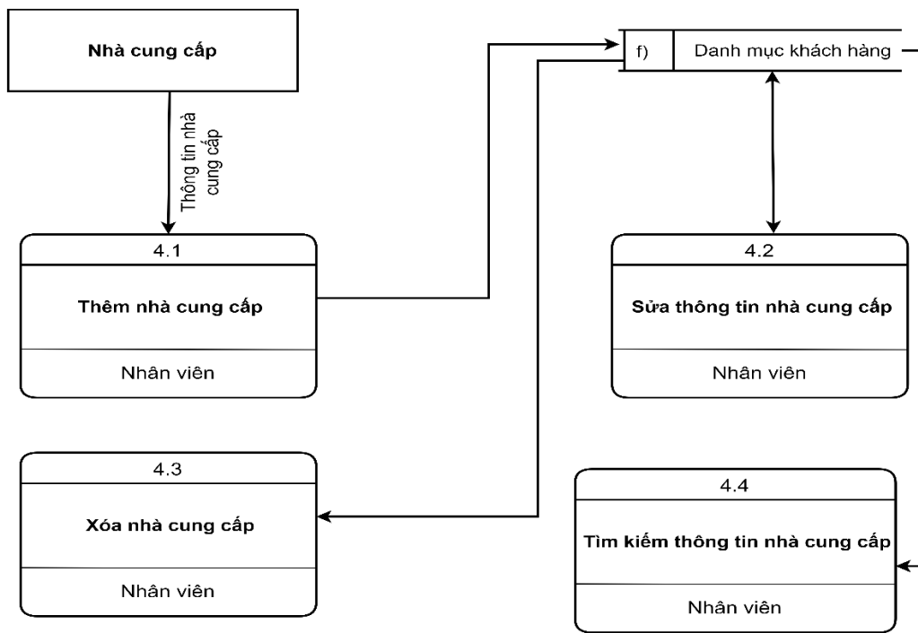
Hình 2. 7: Biểu đồ dữ liệu mức 1 chức năng xem nhà cung cấp.
