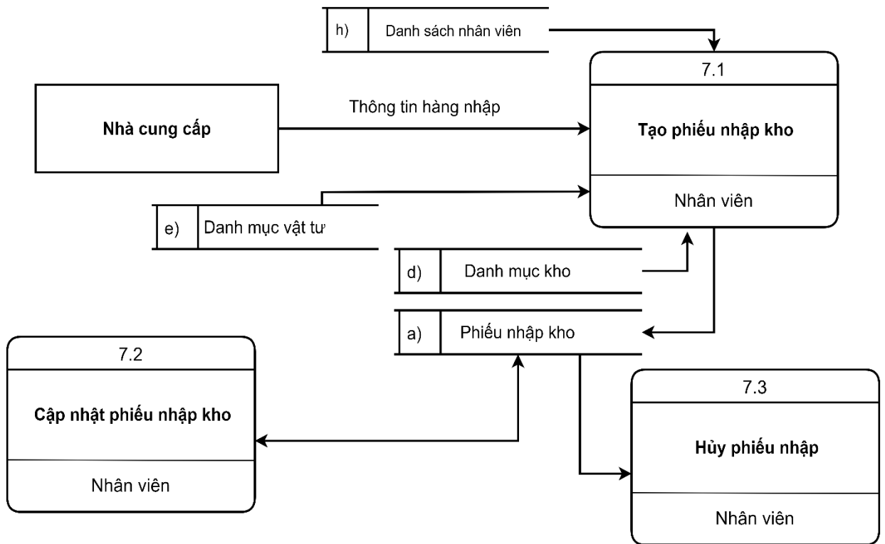
Hình 2. 10: Biểu đồ dữ liệu mức 1 chức năng nhập hàng.
