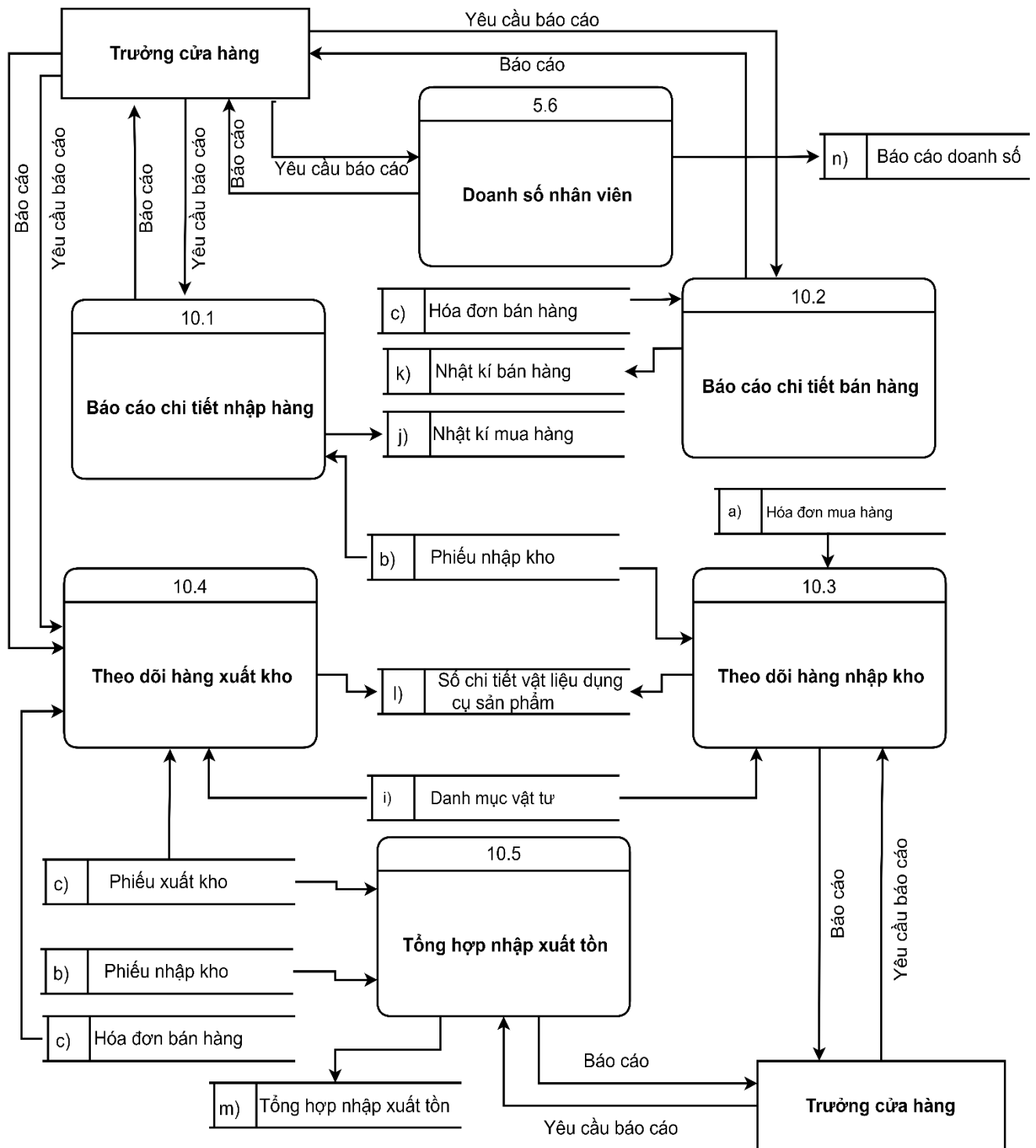
Hình 2. 13: Biểu đồ dữ liệu mức 1 chức năng báo cáo.
