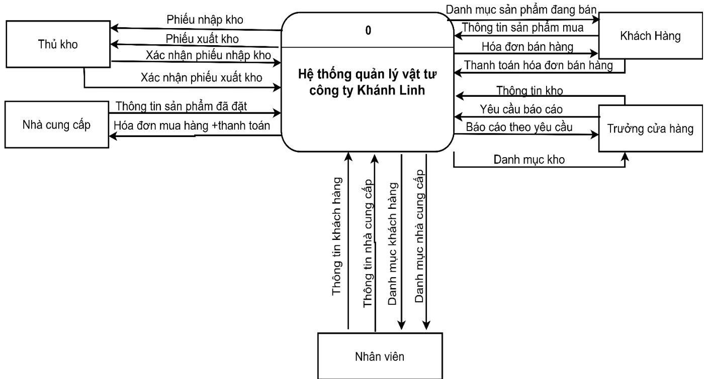
Hình 2. 1: Biểu đồ ngữ cảnh
