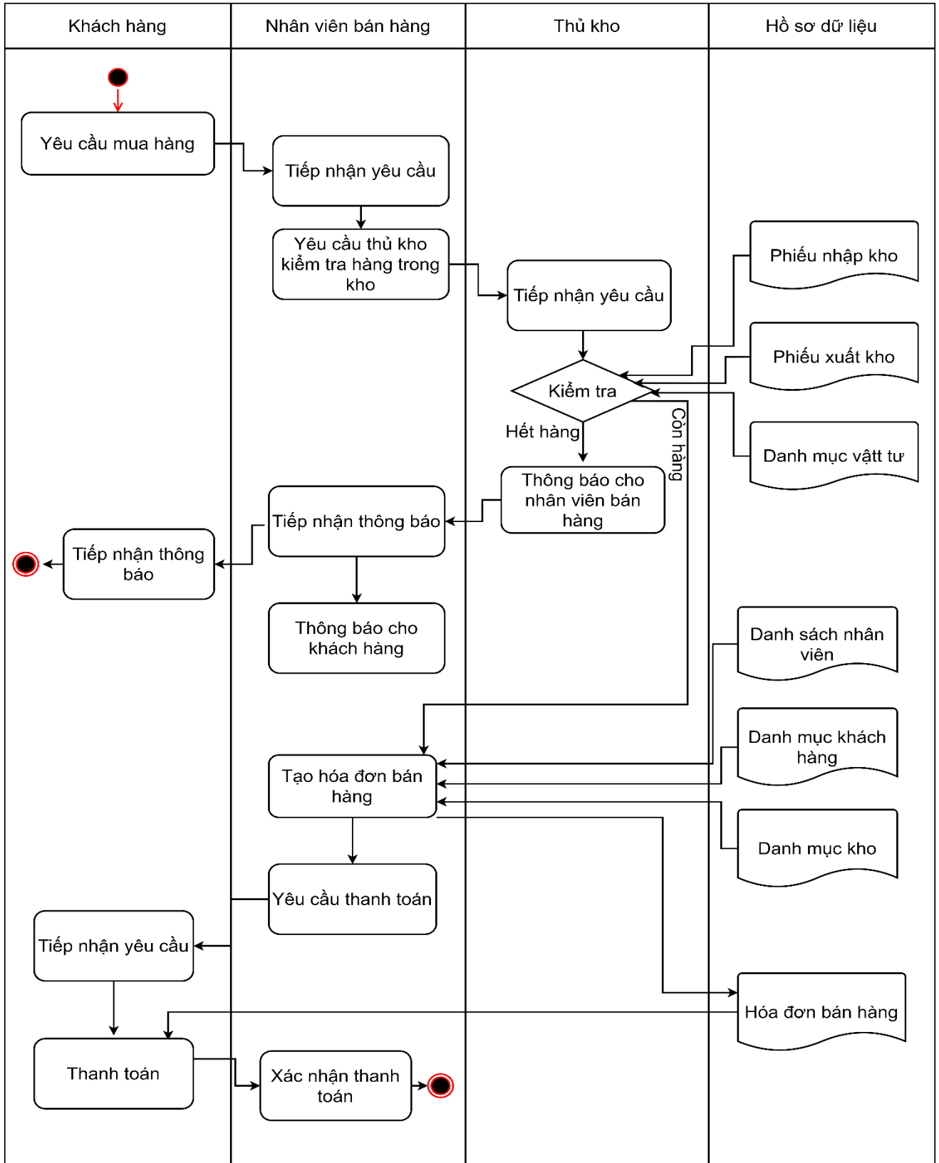
Hình 1. 3: Sơ đồ tiến trình nghiệp vụ “ bán hàng ”
