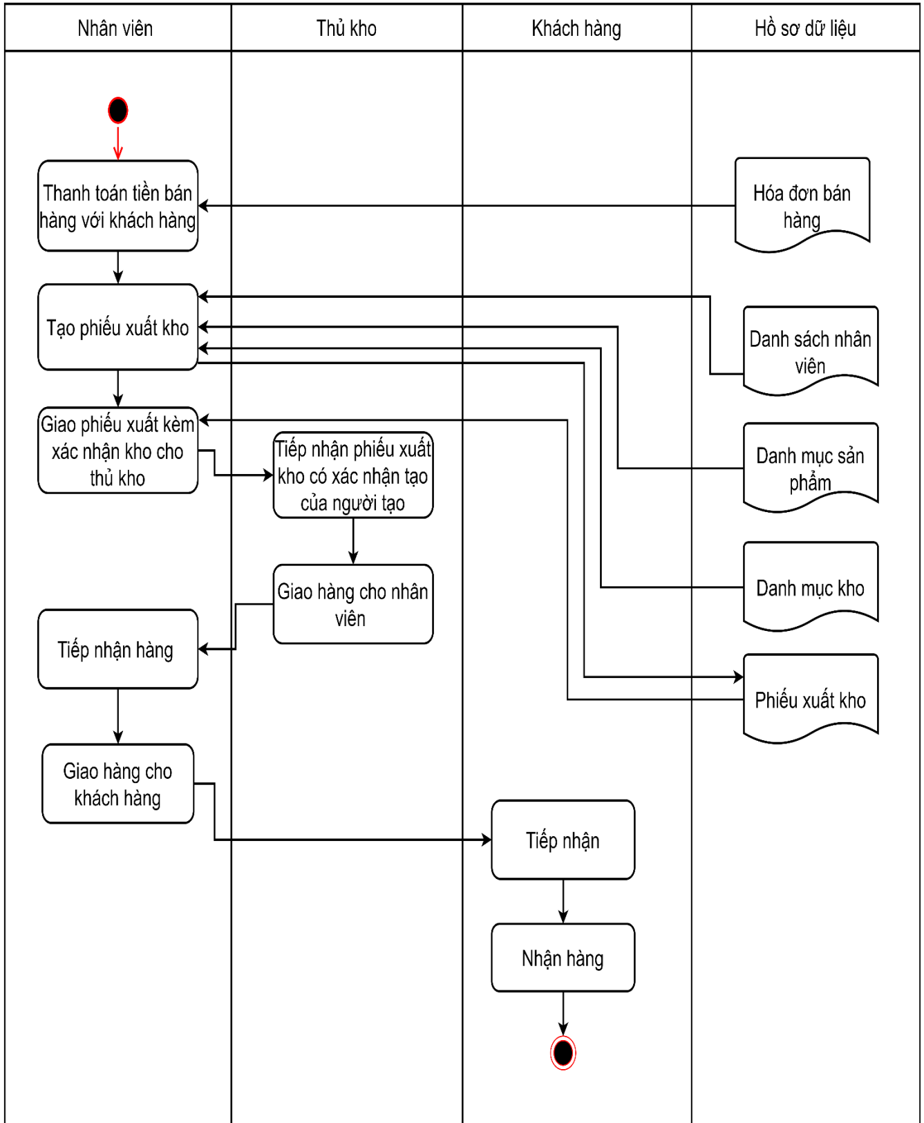
Hình 1. 4: Sơ đồ tiến trình nghiệp vụ “xuất hàng”
