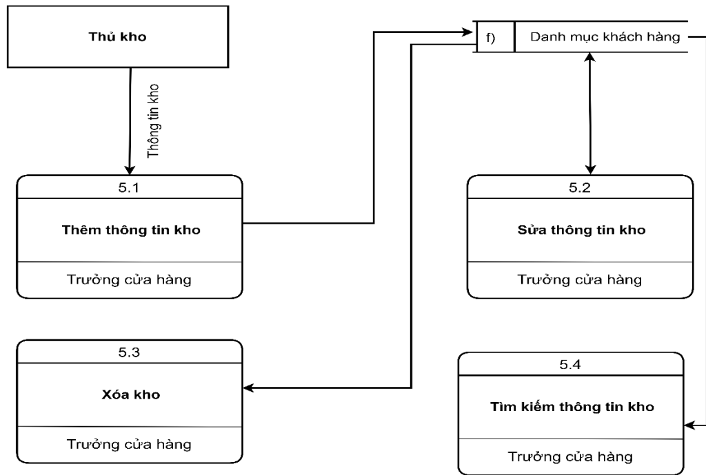
Hình 2. 8: Biểu đồ dữ liệu mức 1 chức năng xem kho.
