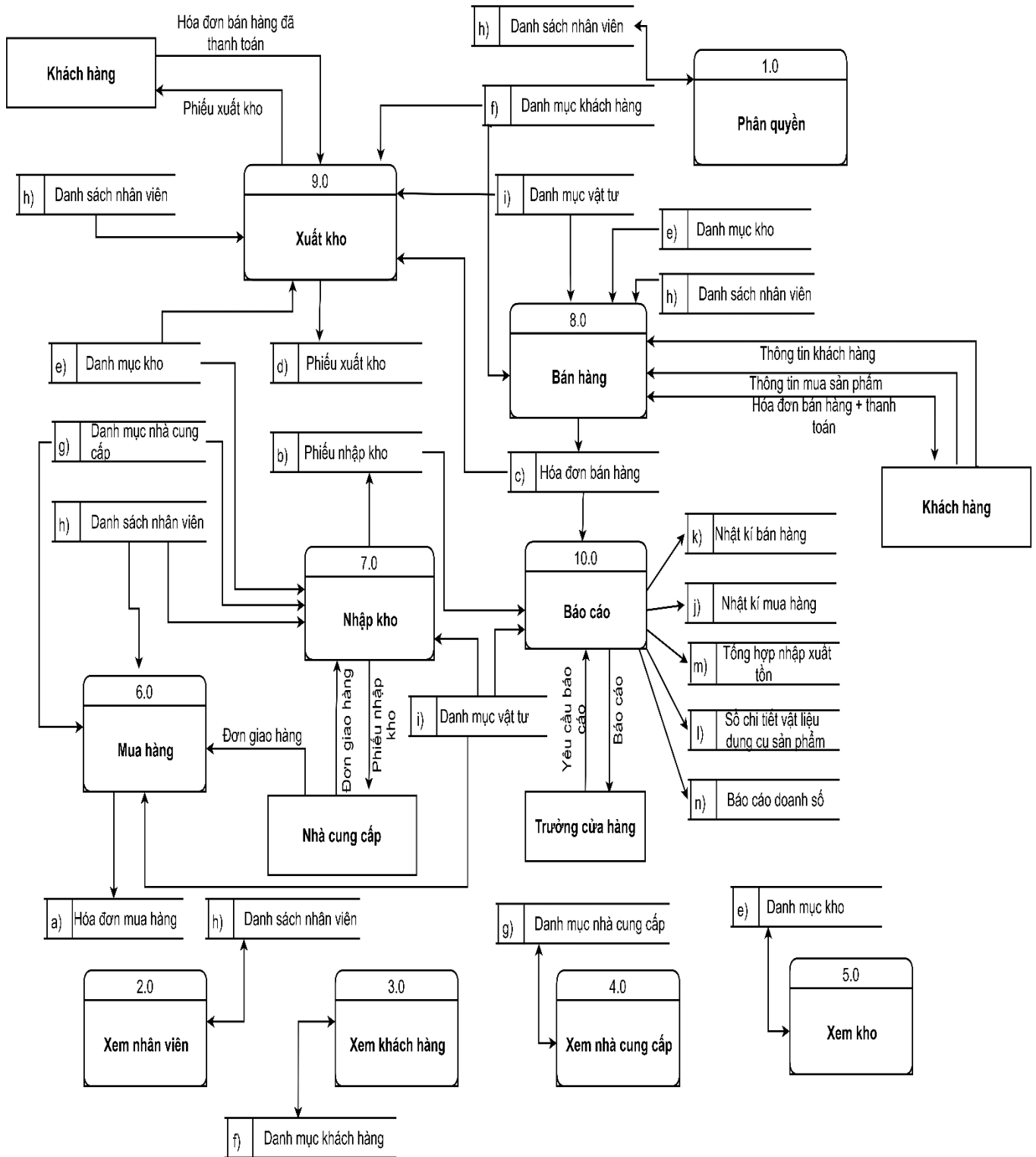
Hình 2. 3: Biểu đồ dữ liệu mức hệ thống.
