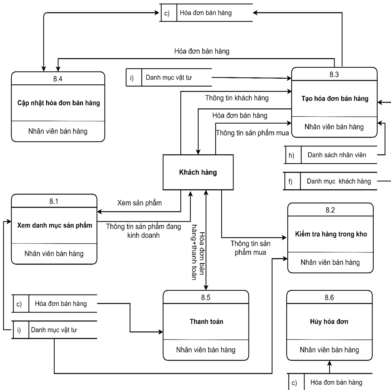
Hình 2. 11: Biểu đồ dữ liệu mức 1 chức năng bán hàng.
