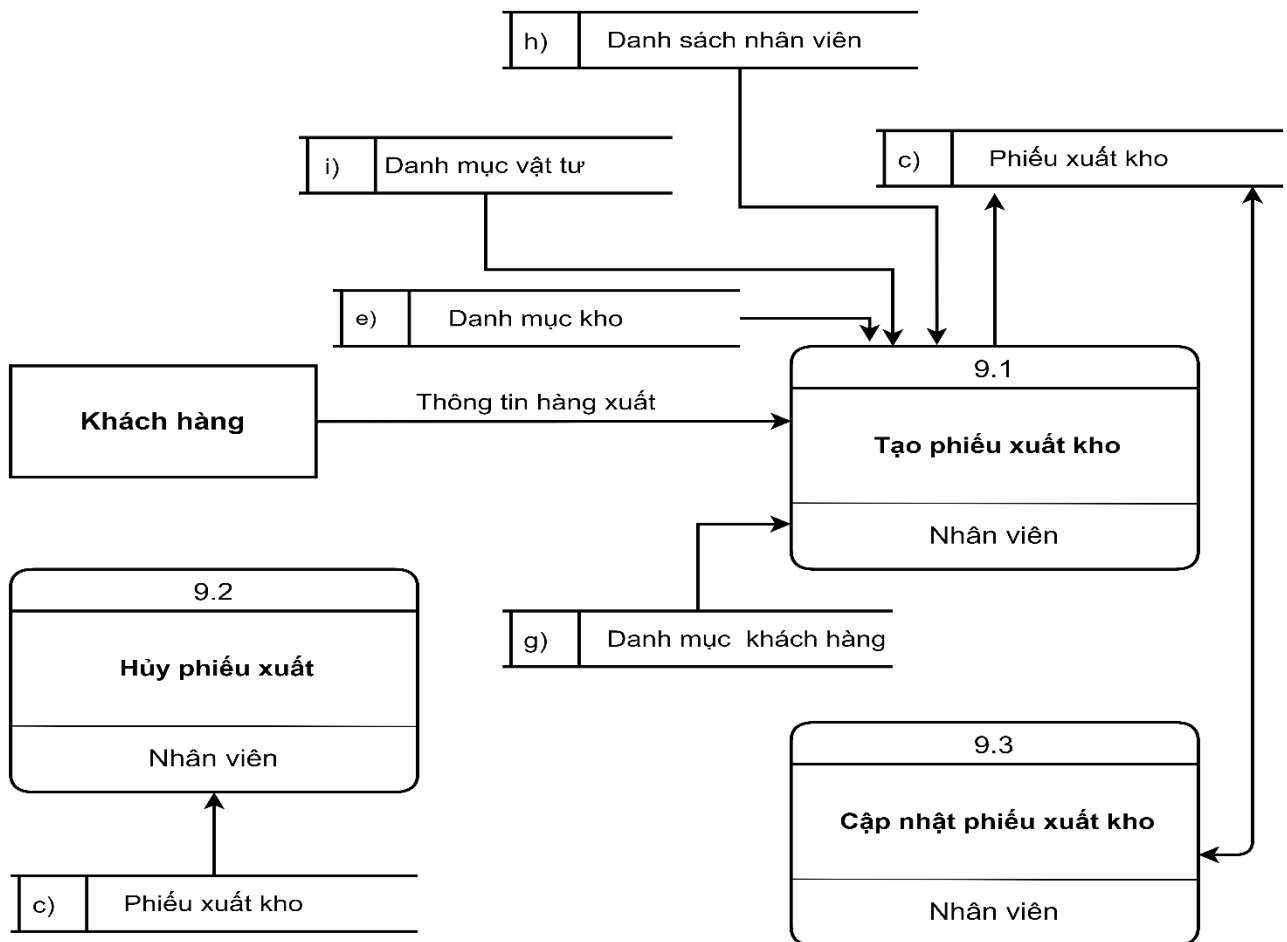
Hình 2. 12: Biểu đồ dữ liệu mức 1 chức năng xuất hàng.
