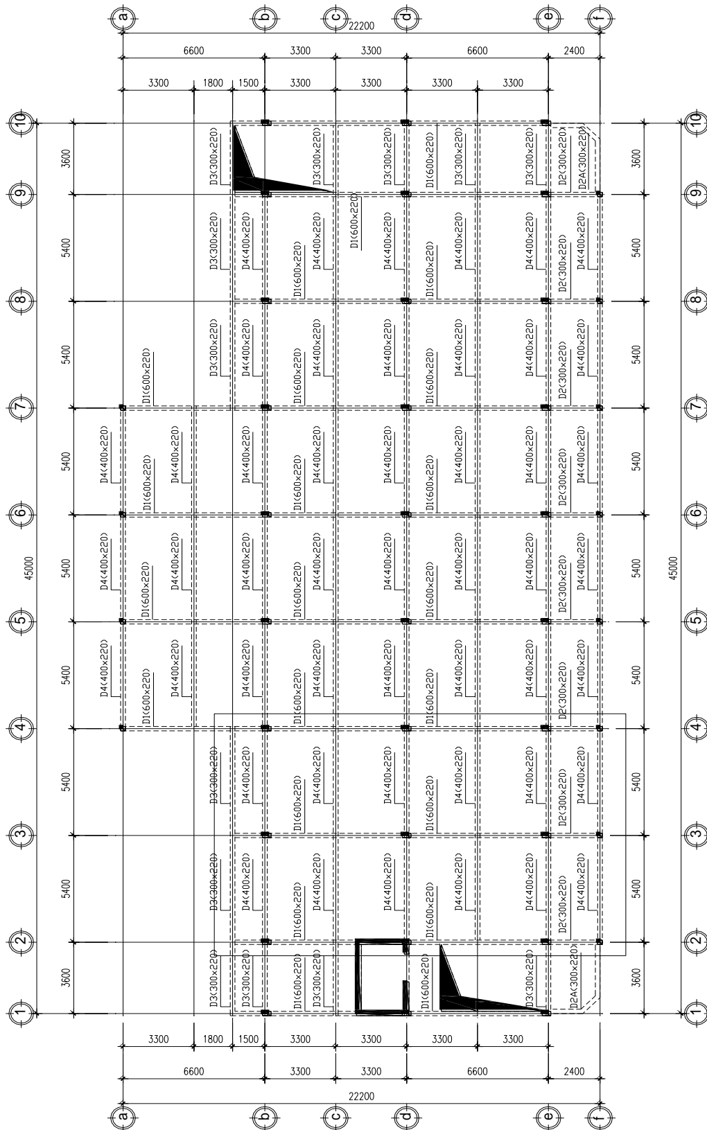
MẶT BÊN KẾT CẤU TỔNG SỐ HÌNH
