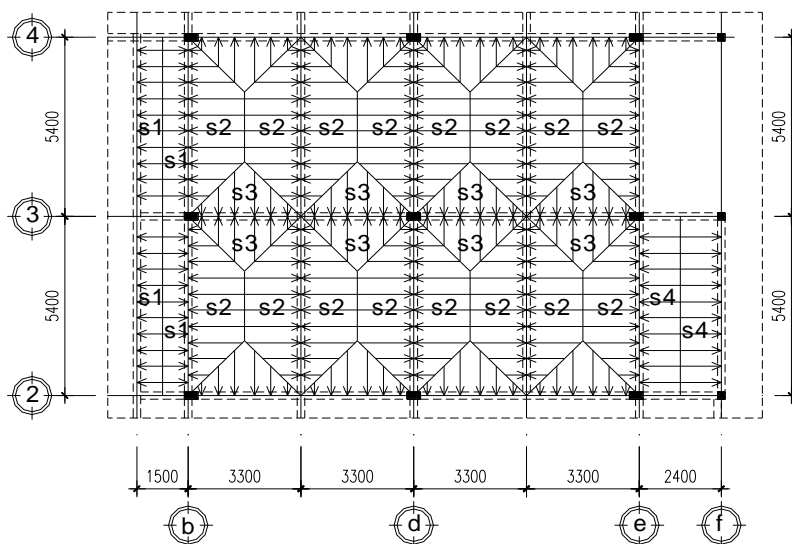
s - Tải phân bố tải trọng 1 vào khung k3
