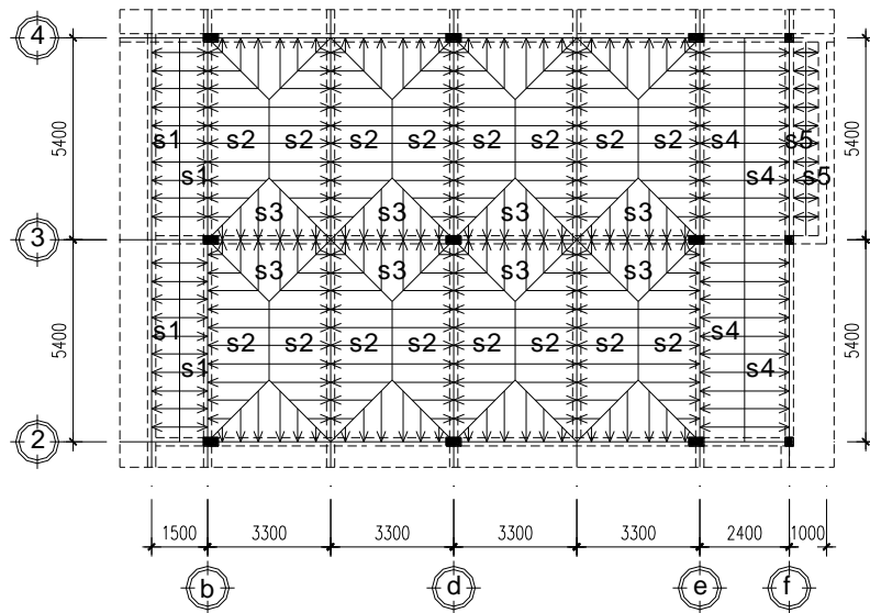
s - Bảng phân bố tải trọng tập trung 5 vòm khung k3
