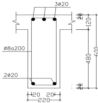
mặt cắt gèi tr i d C m 17
