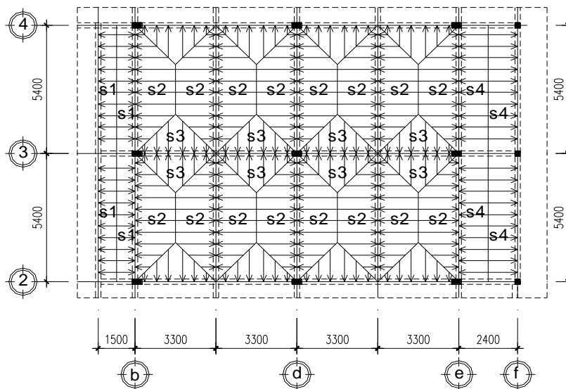
s - Bảng phân bố tải trọng 2,3,4 vào khung k3
