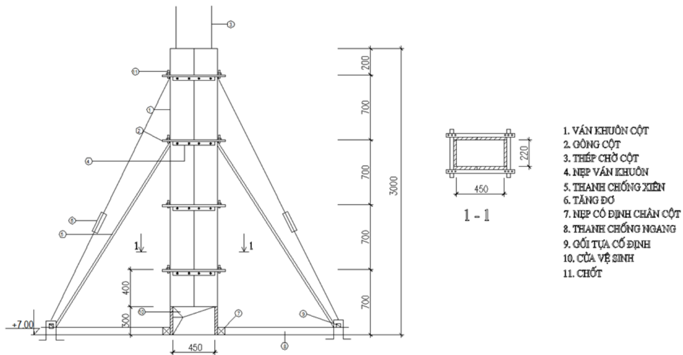
CHI TIẾT VÁN KHUÔN CỘT
