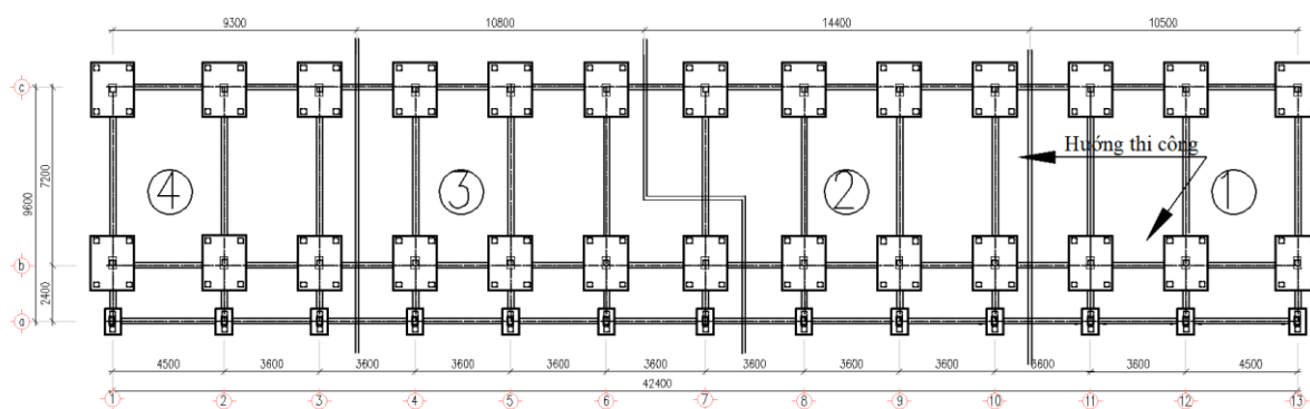
Sơ đồ thi công trên mặt bằng công trình
