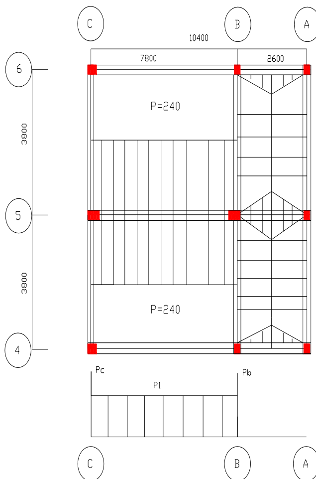
SƠ ĐỒ HOẠT TẢI 1 – TẦNG 2 HOẶC TẦNG 4 HOẠT TẢI 1 – TẦNG 2, 4 (daN/m; daN)
