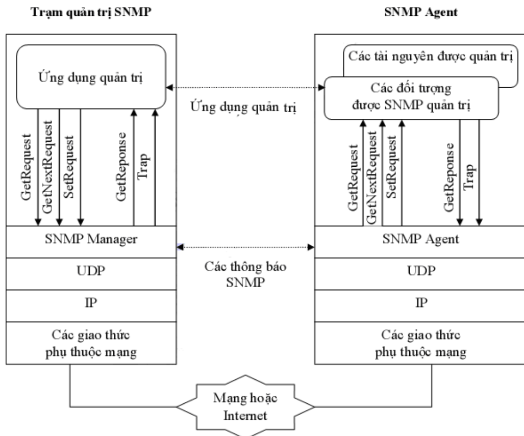
Hình 1-1: Mô hình giao thức hoạt động SNMP
