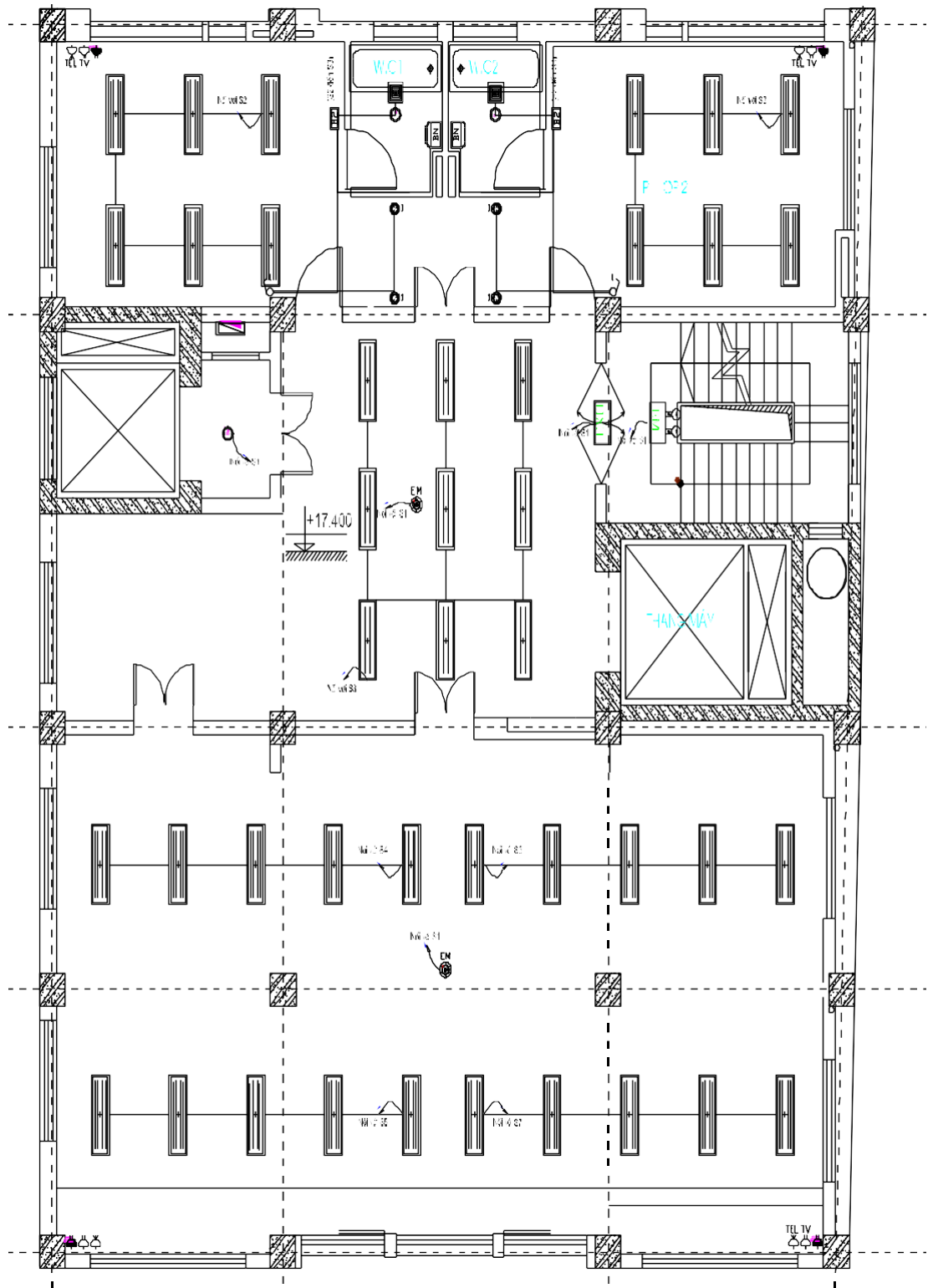
Sơ đồ bố trí chiếu sáng tầng 8
