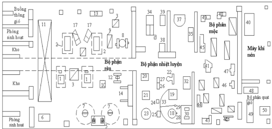
Hình 1.1. Sơ đồ mặt bằng xưởng cơ khí
