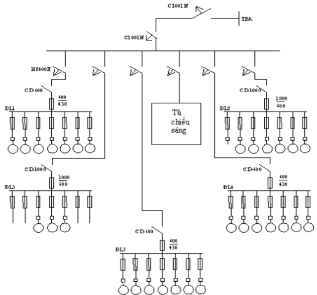
Hình 2.3. Sơ đồ nguyên lý hệ thống cấp điện cho xưởng cơ khí
