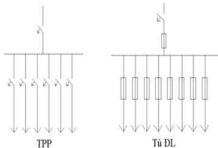
Hình 2.1. Sơ đồ tủ PP và tủ DL
