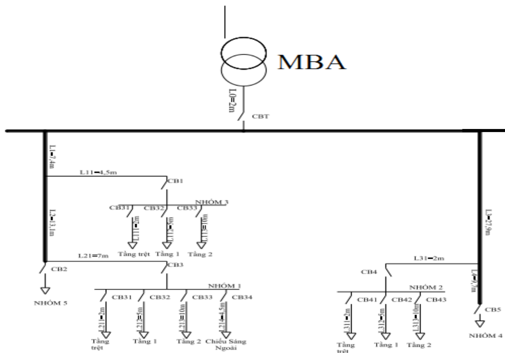
Hình 3.4. Sơ đồ tổng quát khu nhà ở
