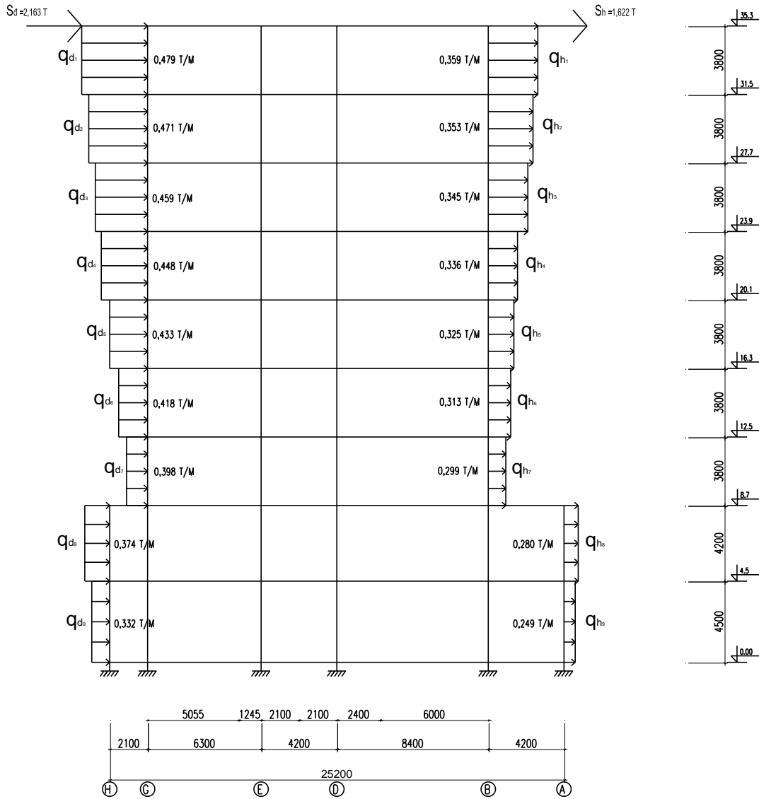
SƠ ĐỒ TẢI TRỌNG GIÓ TỪ TRÁI QUA PHẢI
