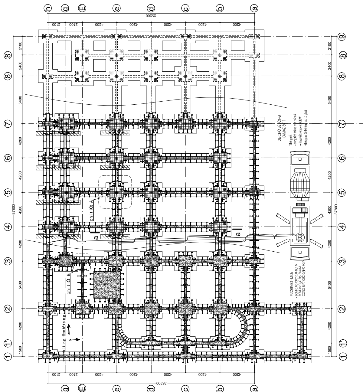
Mặt bằng đồ bê tông móng
