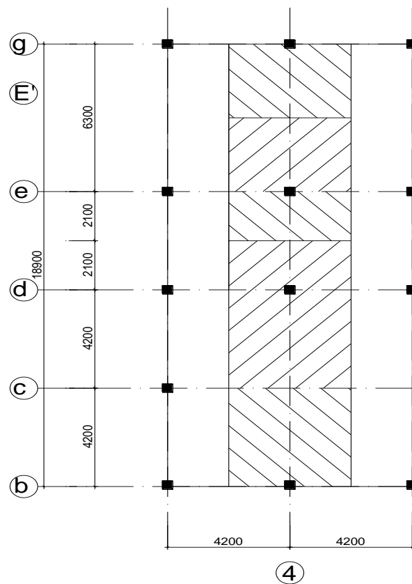
DIỆN CHỊU TẢI CỦA CỘT TRỤC 4
