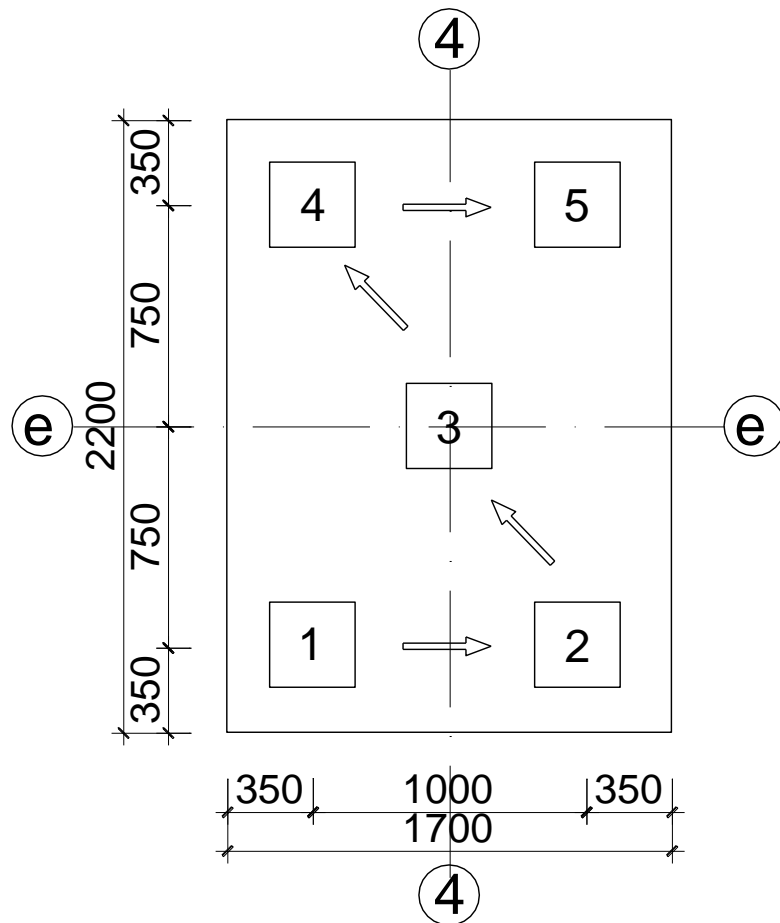
TRÌNH TỰ ÉP CỌC MÓNG M1(E4)
