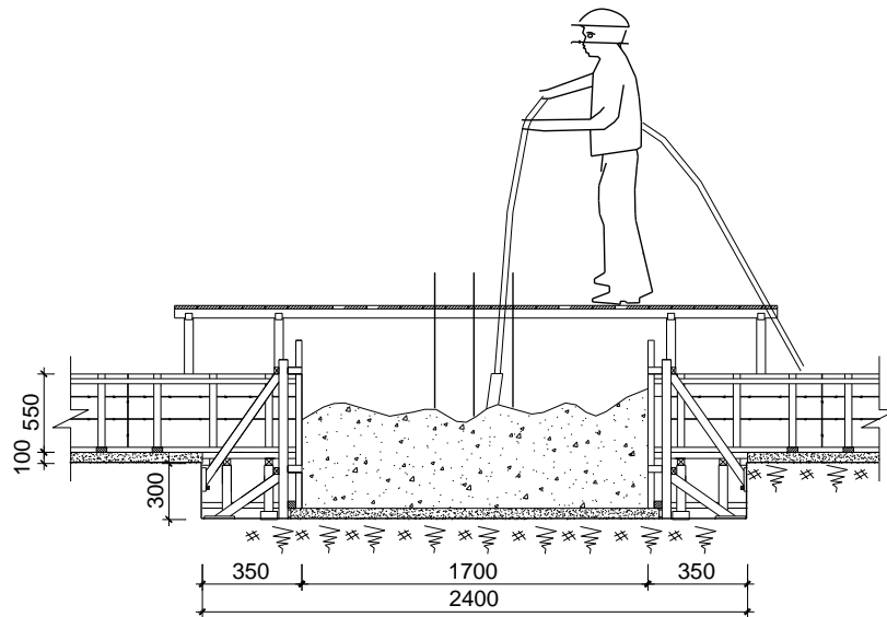
MẶT CẮT 1-1 VÁN KHUÔN GIẢNG
