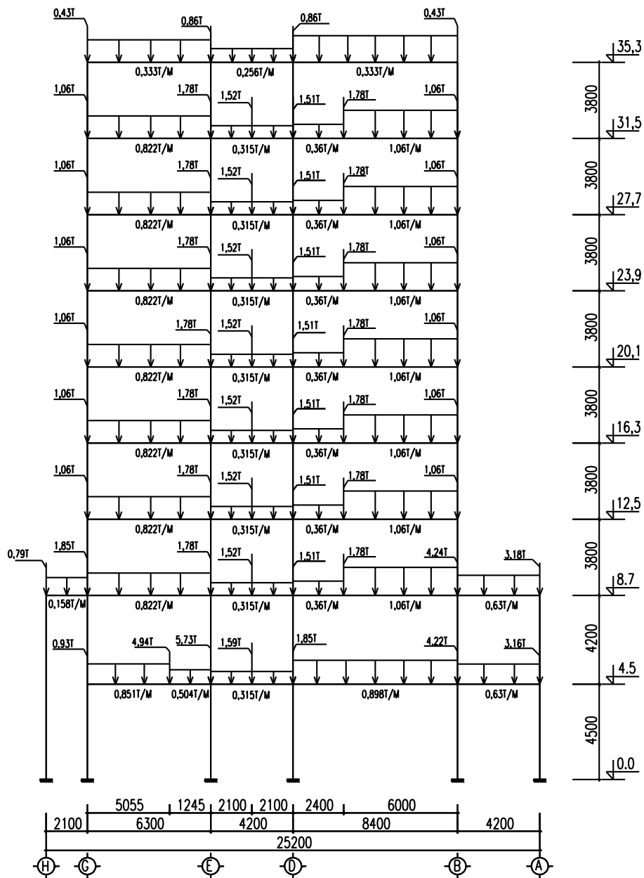
SƠ ĐỒ HOẠT TẢI III TÁC DỤNG LÊN KHUNG
