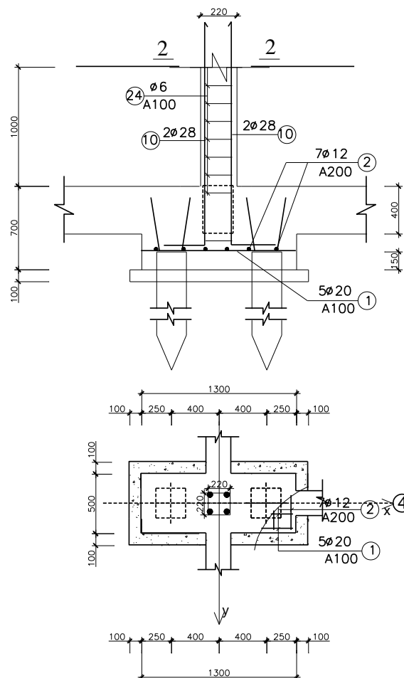
BỐ TRÍ CỐT THÉP MÓNG H4( MÓNG M2)
