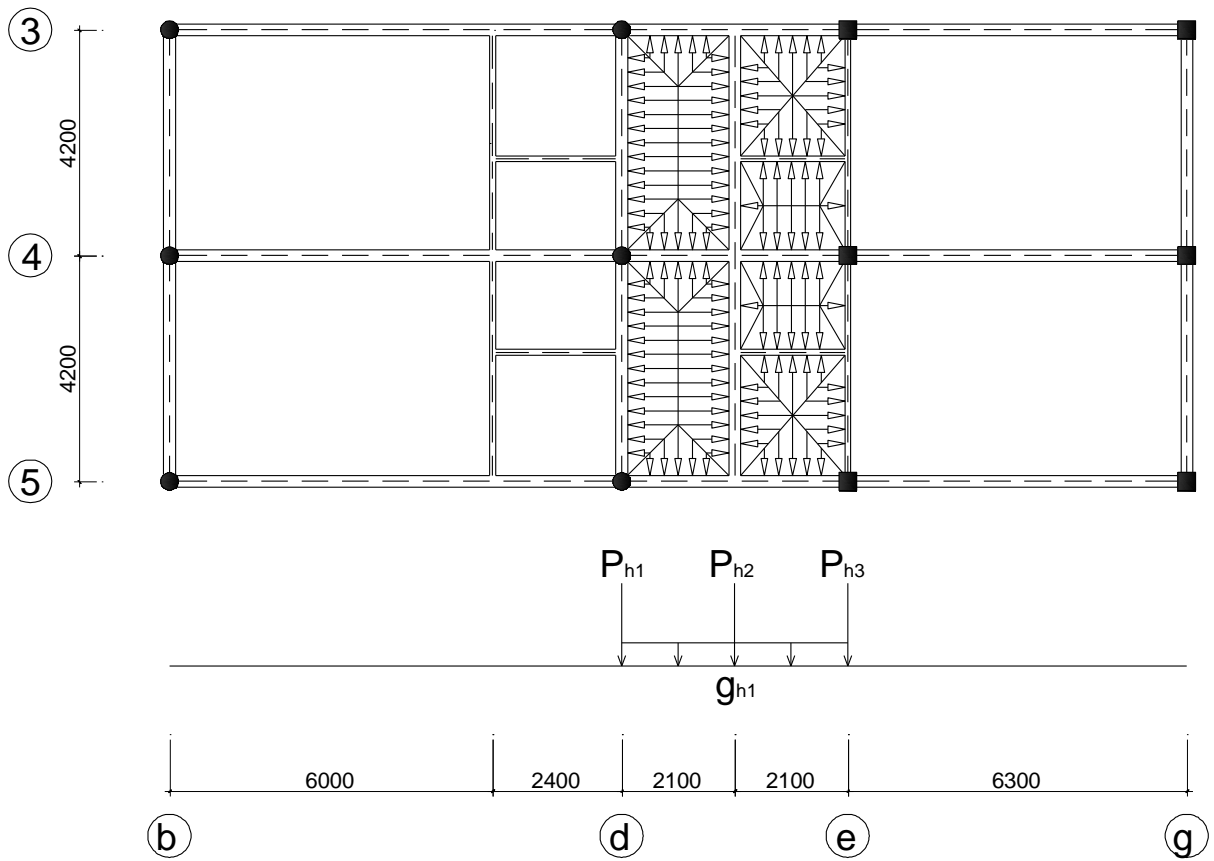
HOẠT TẢI II TẦNG ĐIỂN HÌNH
