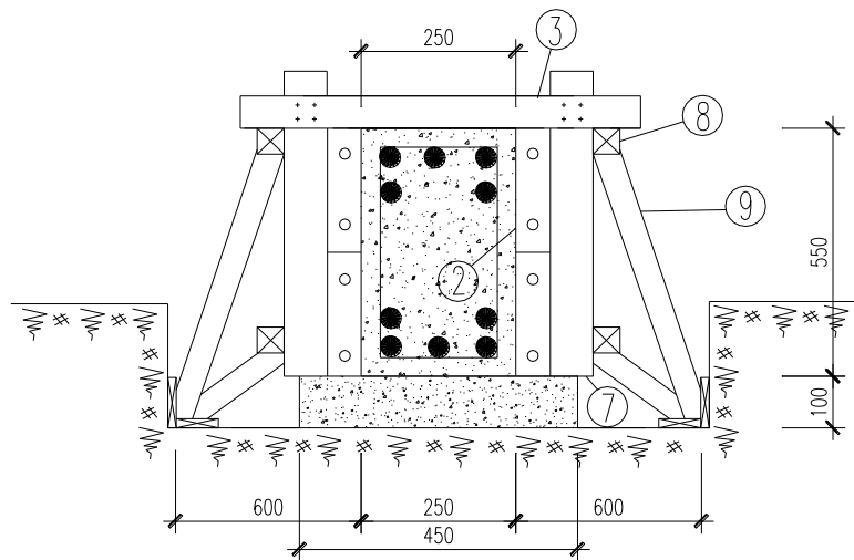
MẶT CẮT NGANG VÁN KHUÔN GIẢNG
