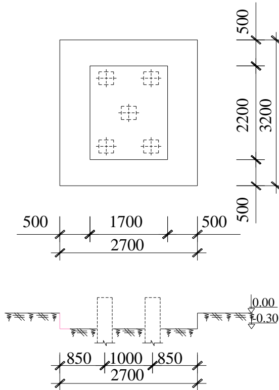
MẶT BẰNG, MẶT CẮT NGANG HỐ ĐÀO MÓNG M1(E4)
