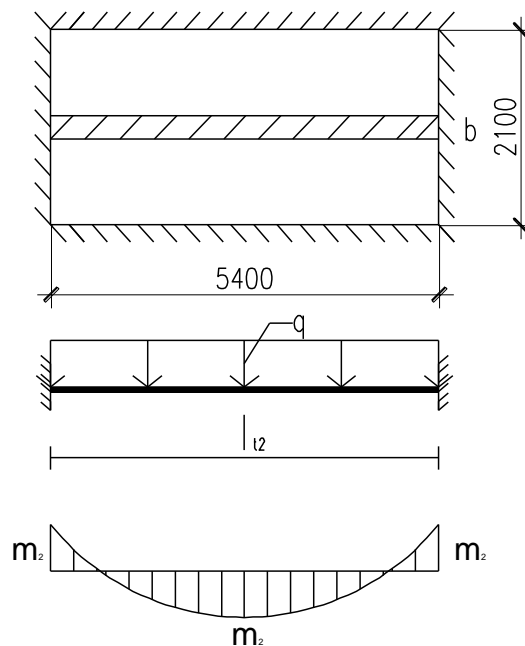
Sơ đồ kết cấu và sơ đồ momen
