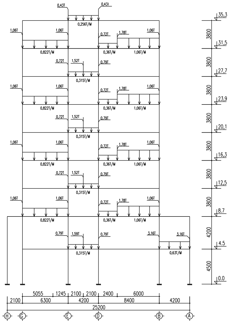
SƠ ĐỒ HOẠT TẢI II TÁC DỤNG LÊN KHUNG
