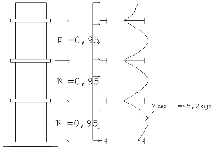
s- ảnh tính toán ván cốt
