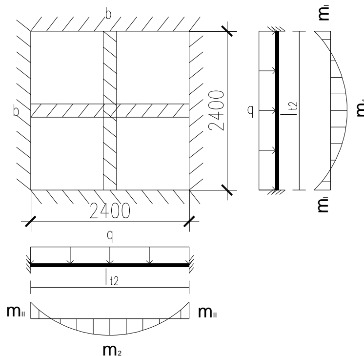
Sơ đồ kết cấu và sơ đồ momen
