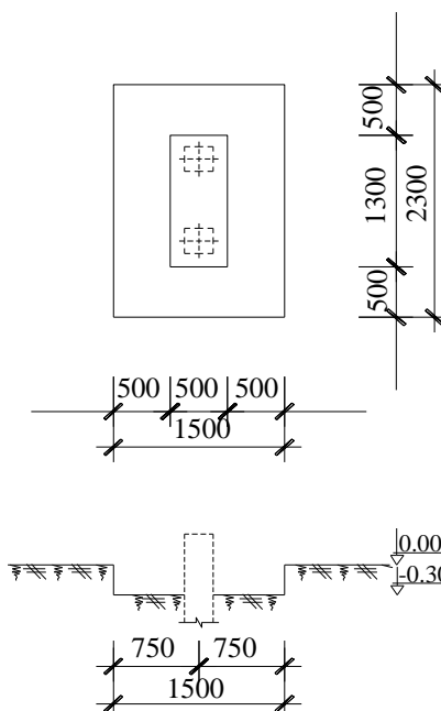
MẶT BẰNG, MẶT CẮT NGANG HỐ ĐÀO MÓNG M2(H4)
