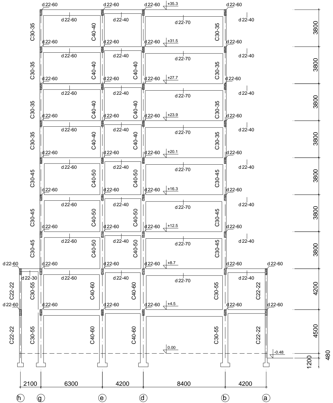
SƠ ĐỒ HÌNH HỌC KHUNG NGANG TRỤC 4
