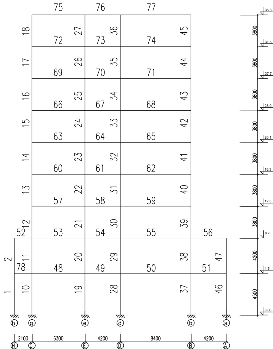
SƠ ĐỒ DẦM VÀ CỘT KHUNG TRỤC 4
