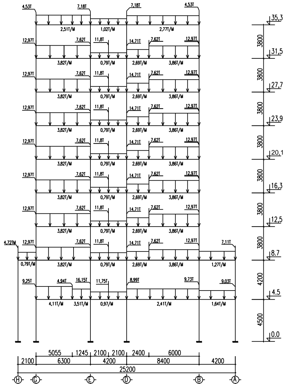
SƠ ĐỒ TĨNH TẢI TÁC ĐỘNG LÊN KHUNG
