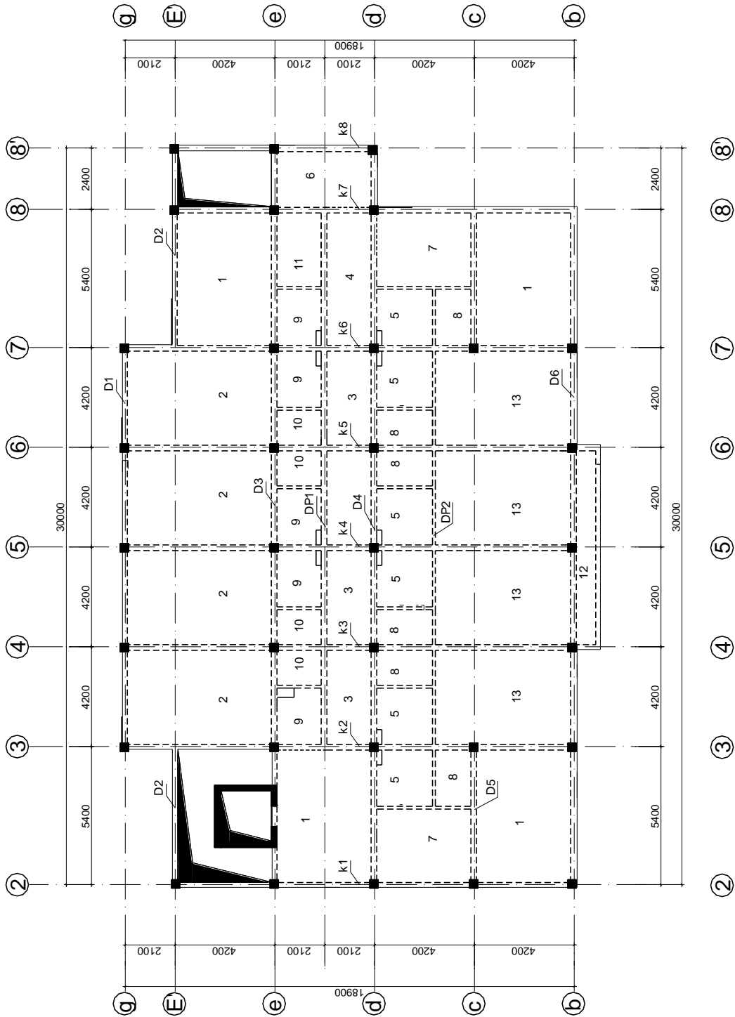
MẶT BẰNG KC TẦNG 4
