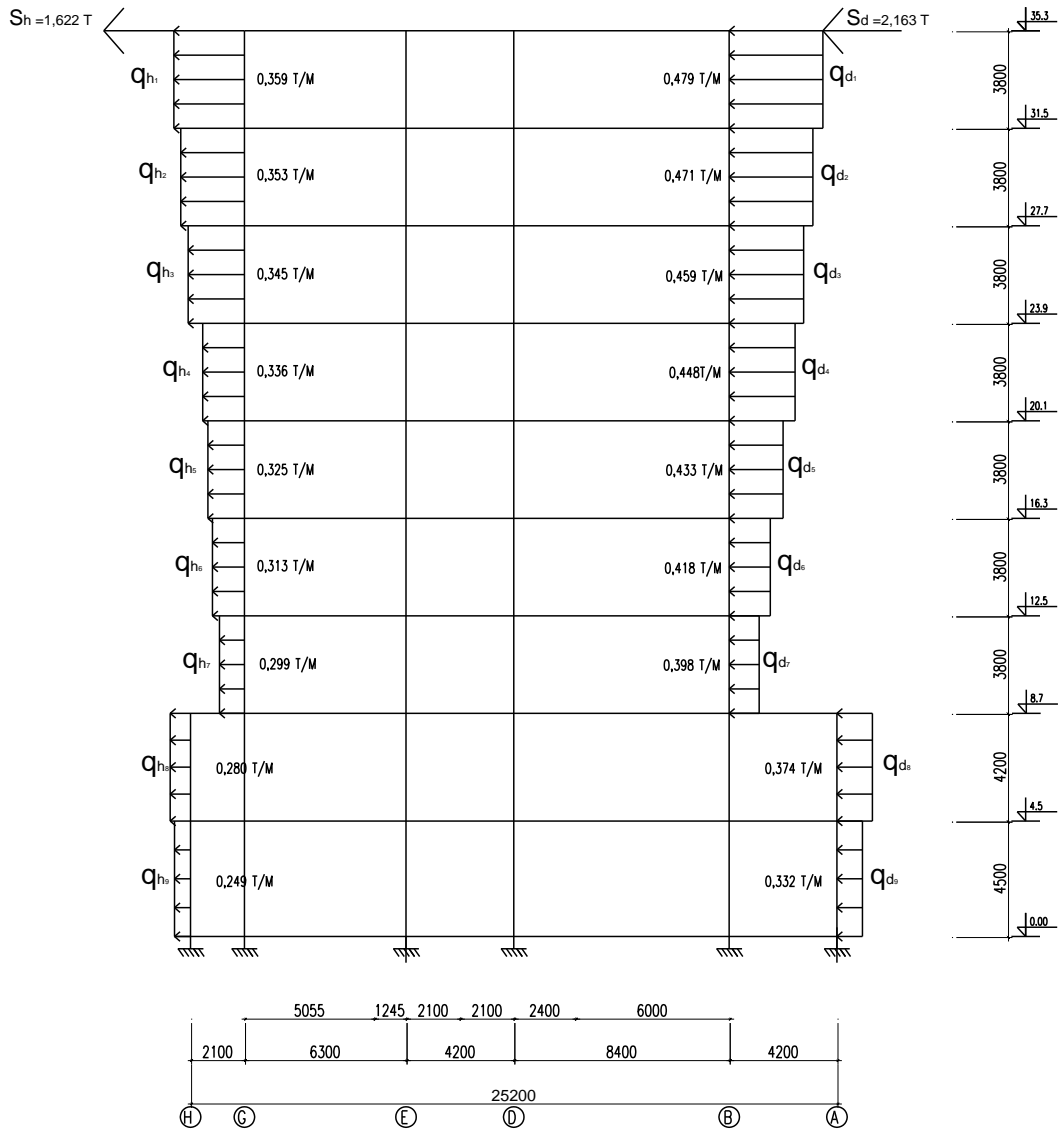
SƠ ĐỒ TẢI TRỌNG GIÓ TỪ PHẢI QUA TRÁI
