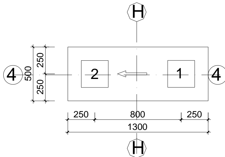
TRÌNH TỰ ÉP CỌC MÓNG M2(H4)
