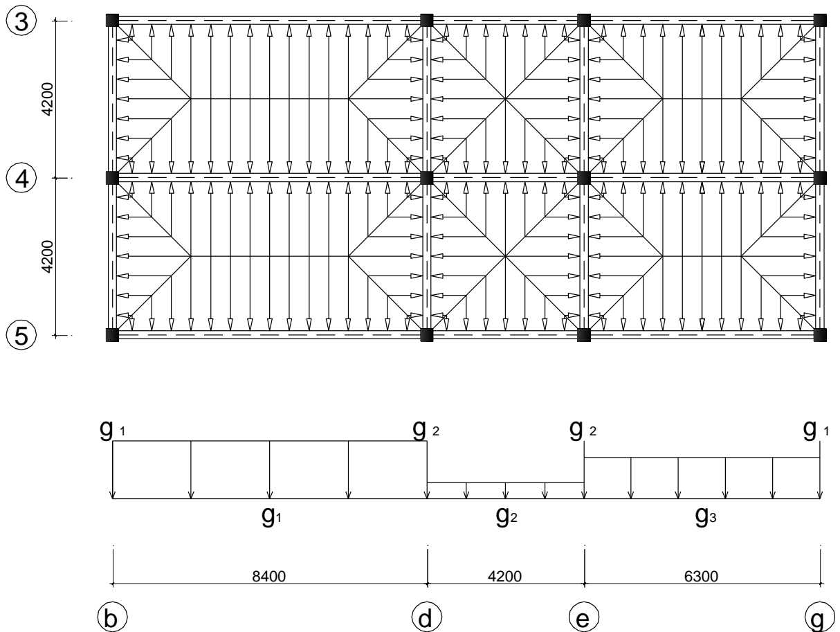
MẶT BẰNG TRUYỀN TẢI VÀ SƠ ĐỒ TRUYỀN TẢI TẦNG MÁI
