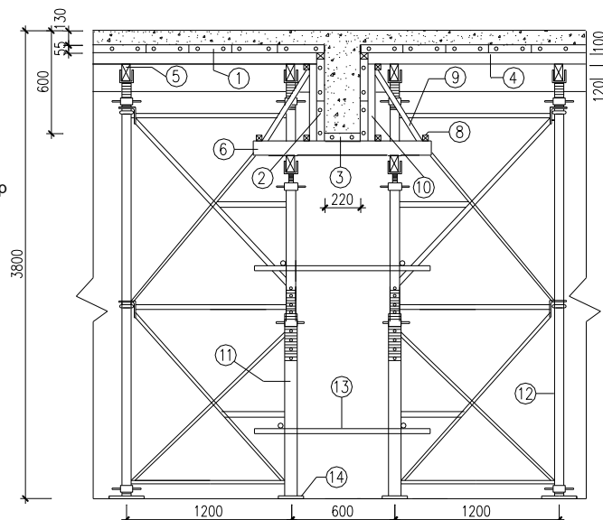
CÊU T O V, N KHU«N DÇM CHÝNH t l 1:25
