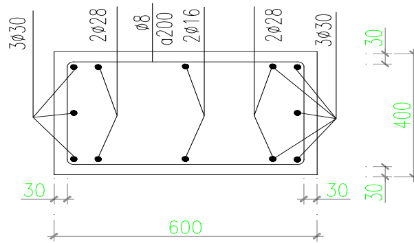
MẶT CẮT CỘT TRỤC B-G TẦNG 1-7
