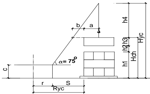
Hỡnh 4: Sơ đồ cầu đối trọng
