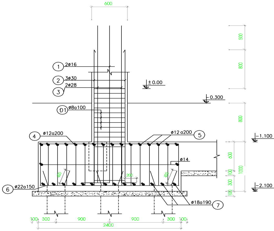
MẶT CẮT 1-1
