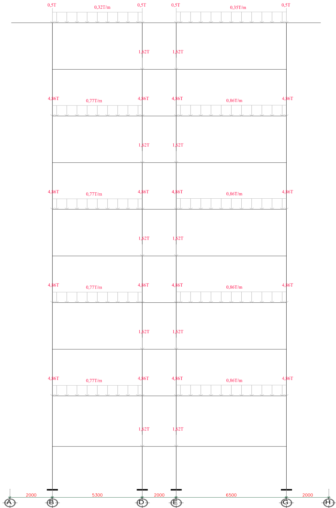
HOẠT TẢI- SƠ ĐỒ 2
