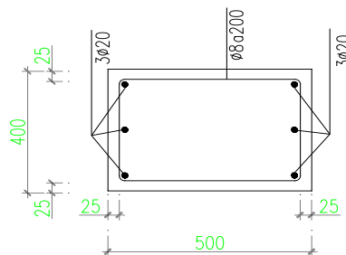
MẶT CẮT CỘT TRỤC D-E TẦNG 8-10
