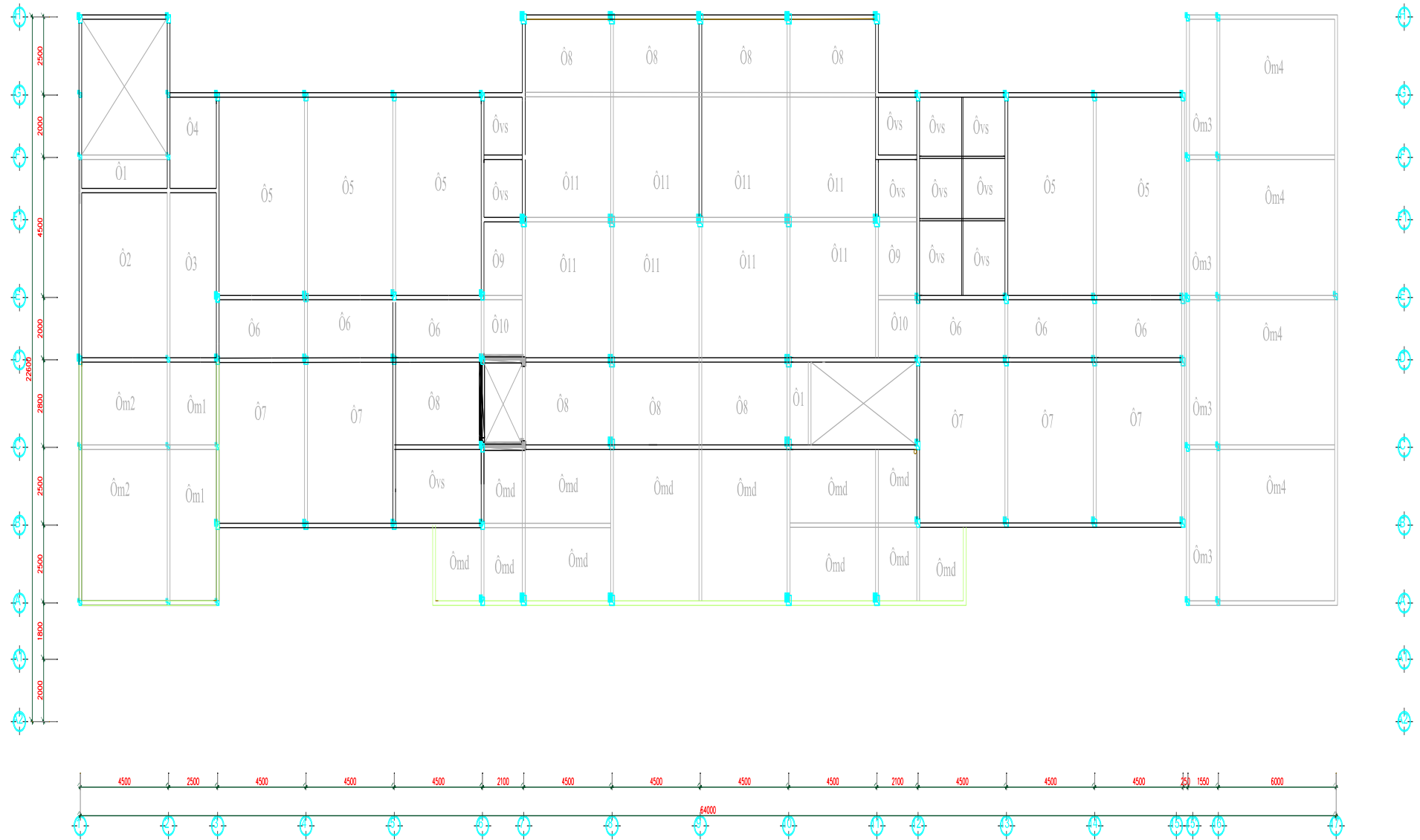
MẶT BẰNG KẾT CẤU Ô SÀN TẦNG 3
