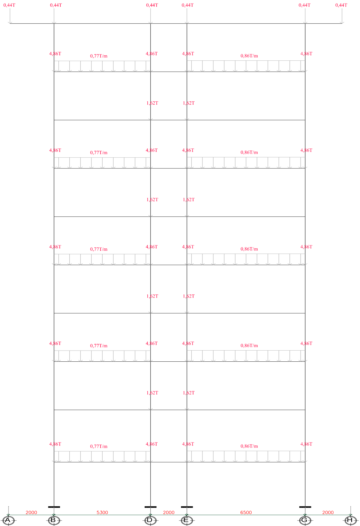
HOẠT TẢI - SƠ ĐỒ 1
