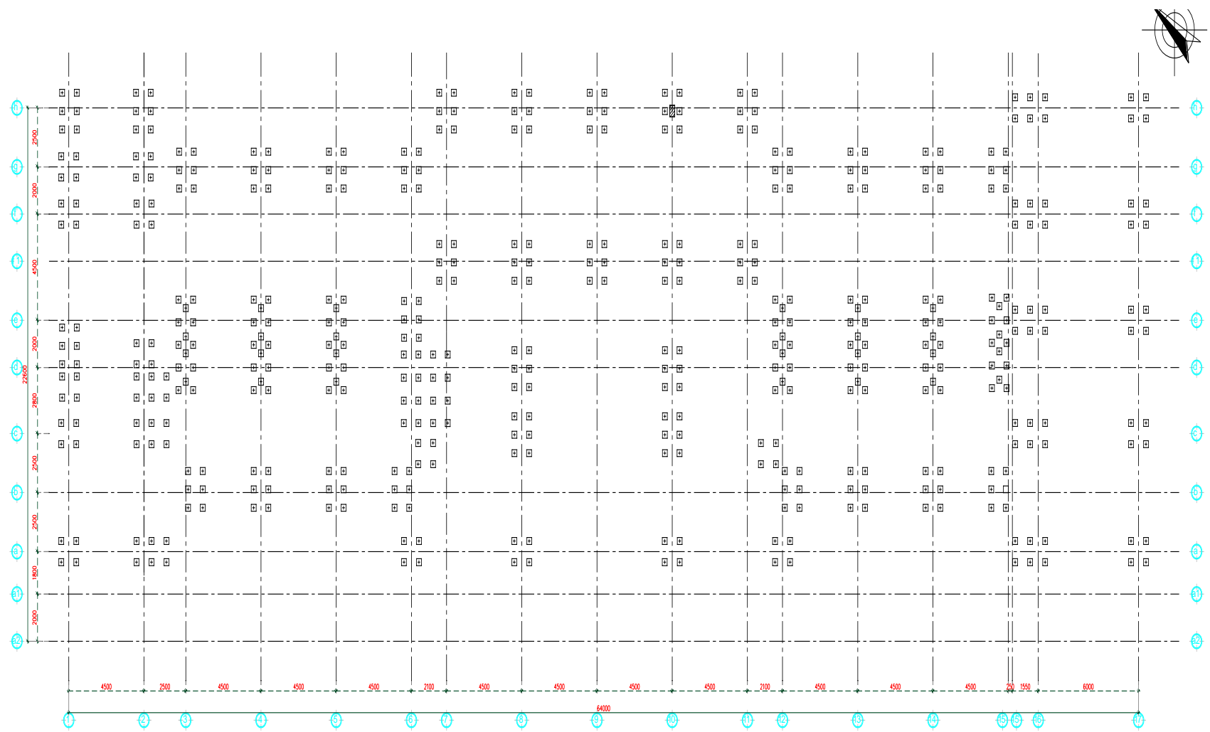
Hình 1: Mặt bằng định vị cọc
