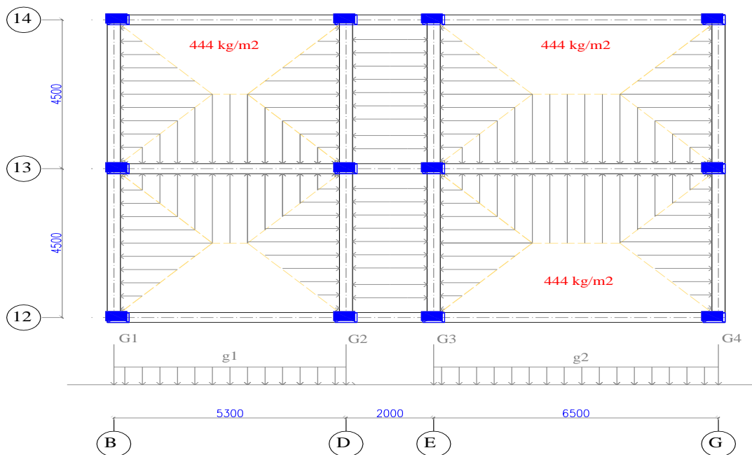
MẶT BẰNG DỒN TẢI TẦNG 2
