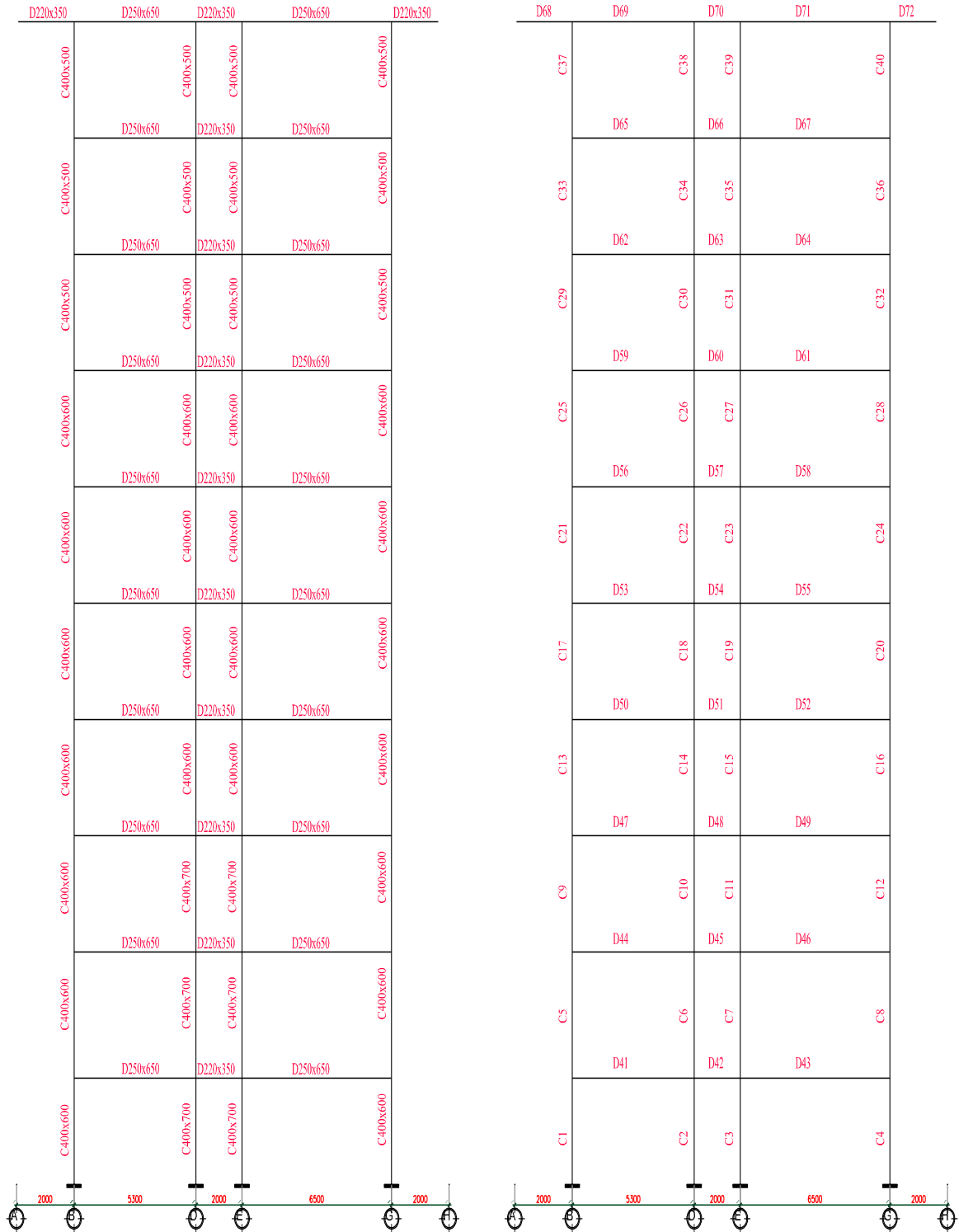
SƠ ĐỒ KẾT CẤU KHUNG
