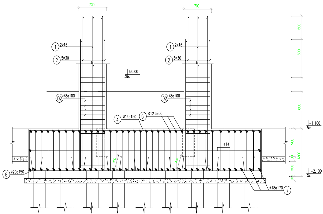
MẶT CẮT 2-2
