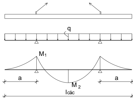
Biểu đồ Momen các khi vận chuyển
