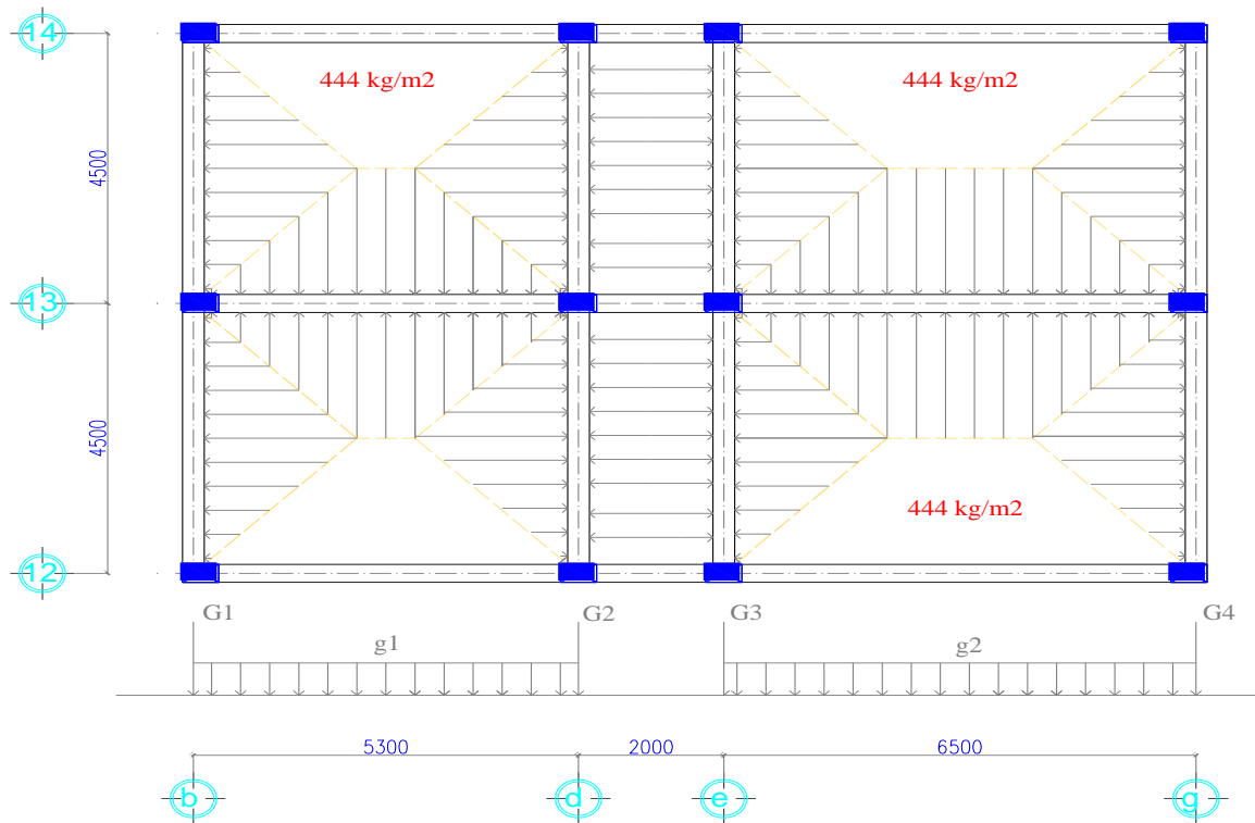
MẶT BẰNG DÒN TẢI TẦNG 3-10
