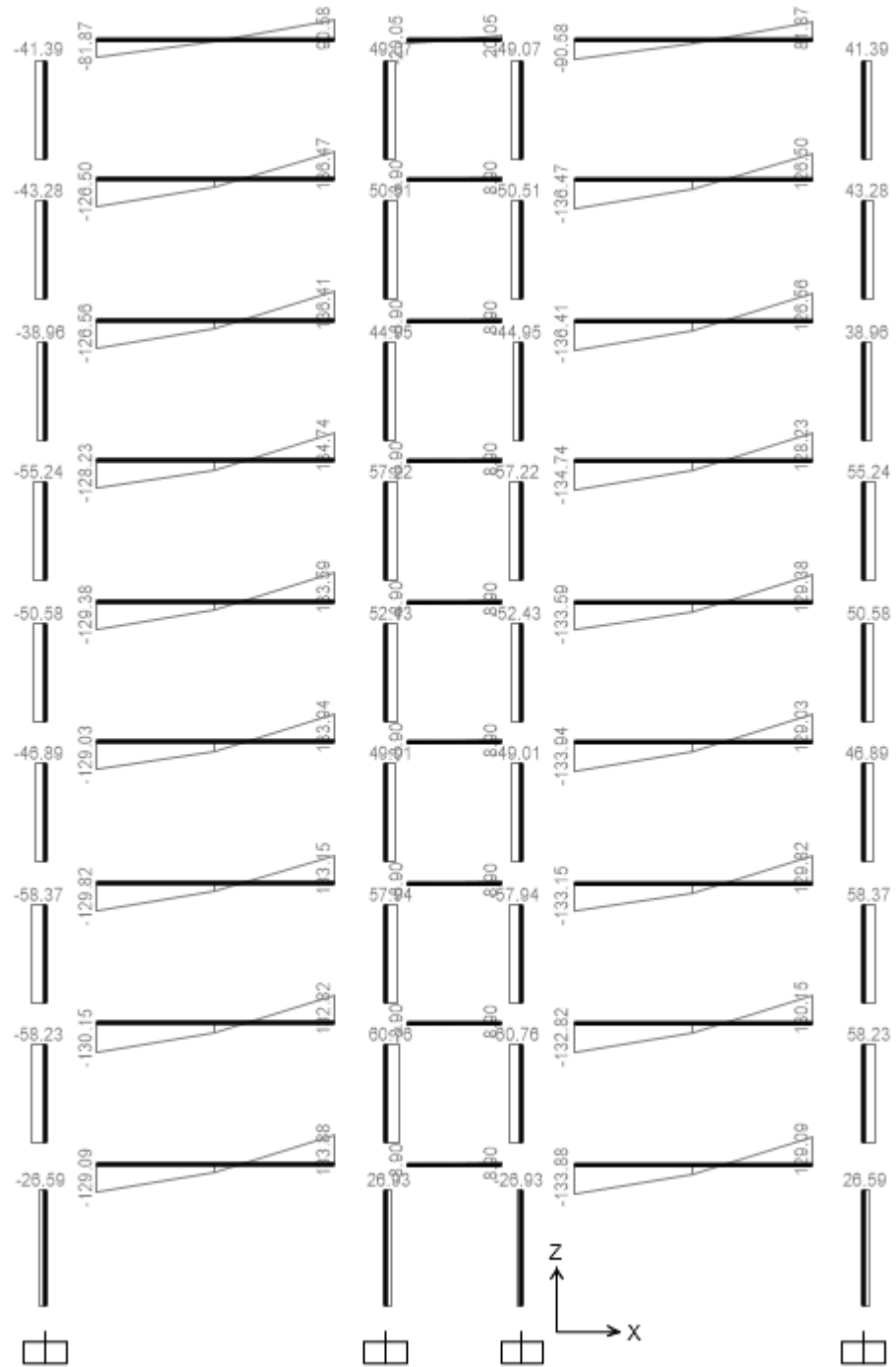
Lực cắt do tĩnh tải gây ra.
