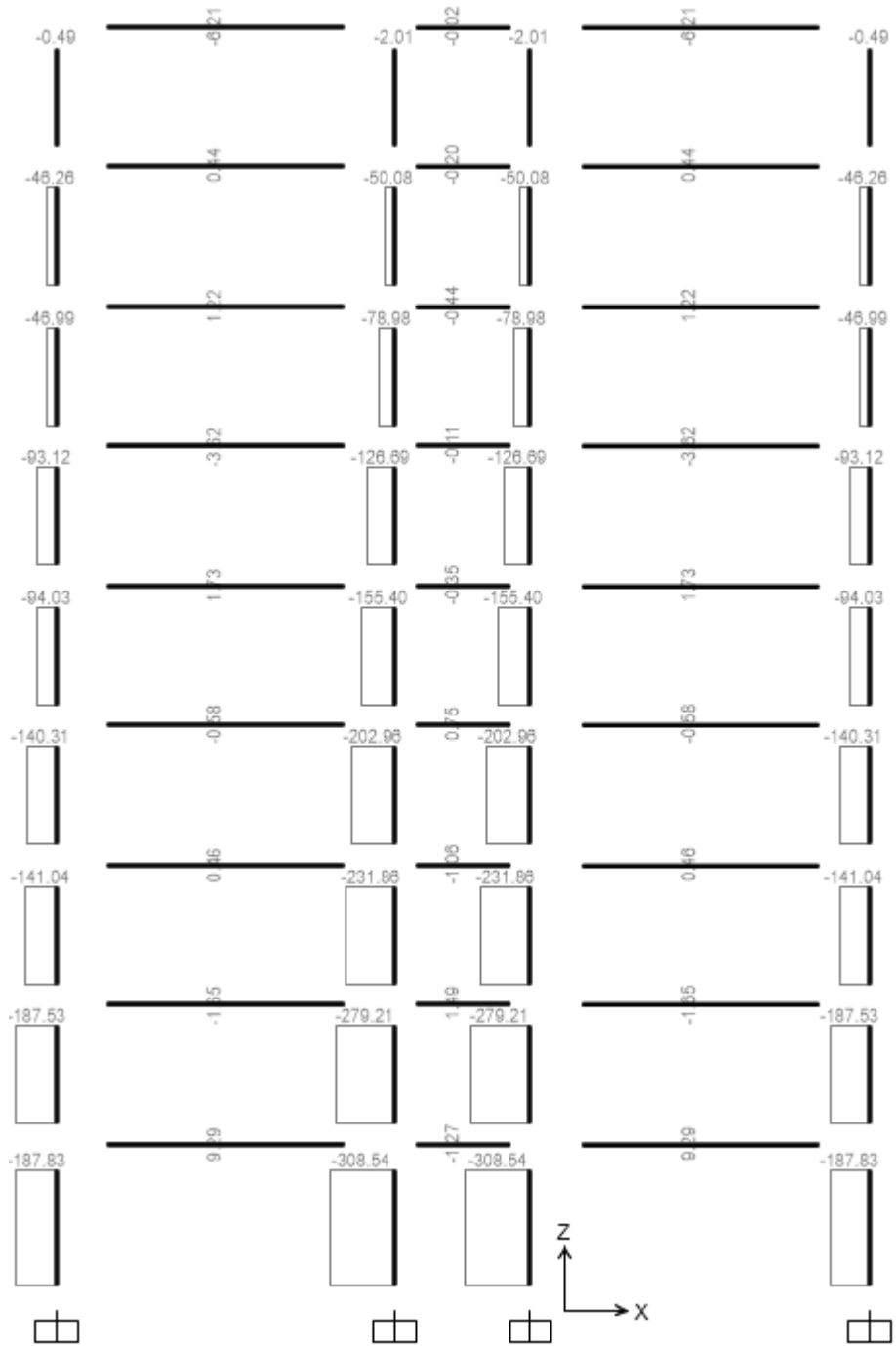
Lực dọc do hoạt tải 2 gây ra.
