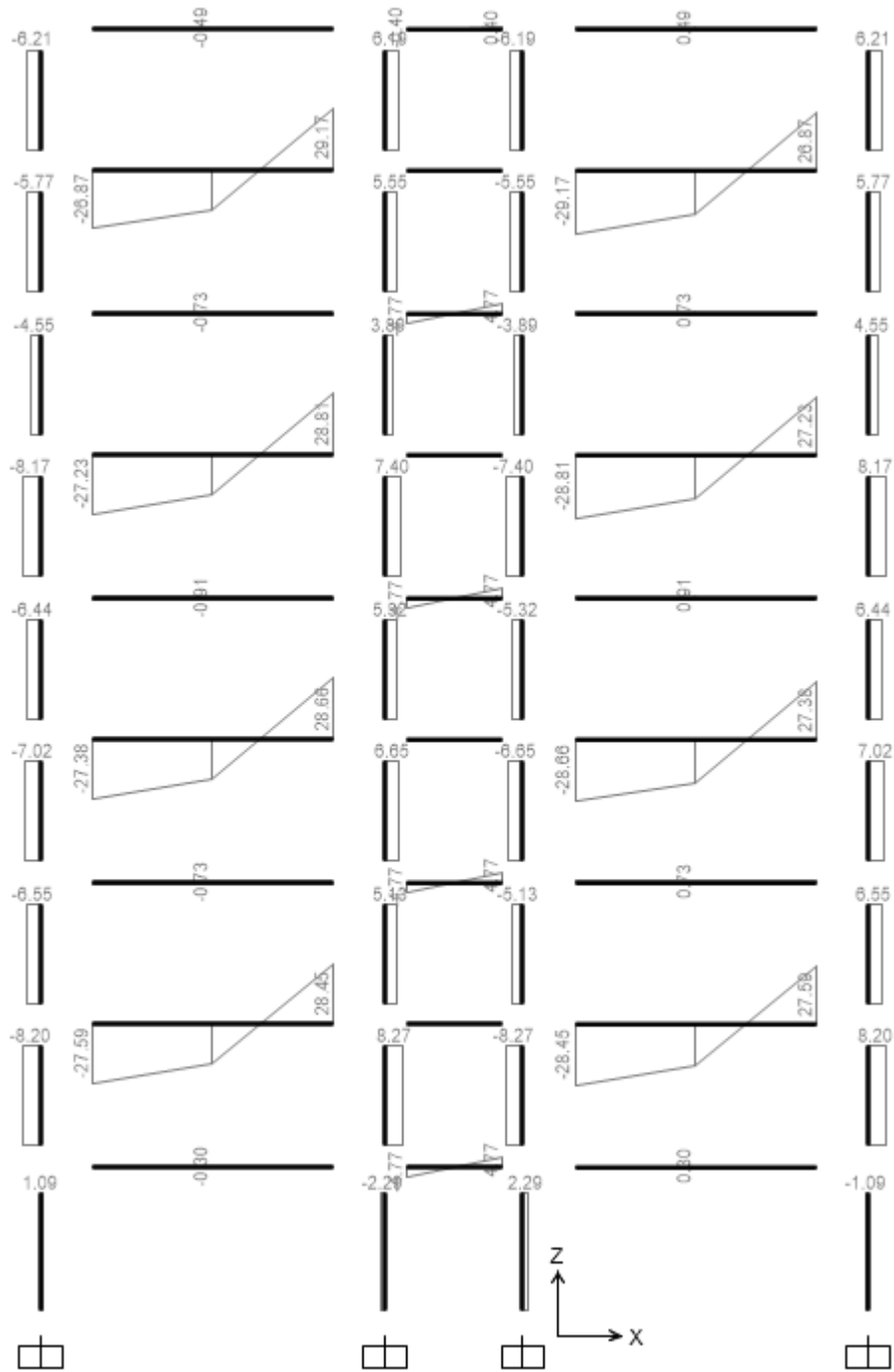
Lực cắt do hoạt tải 2 gây ra.
