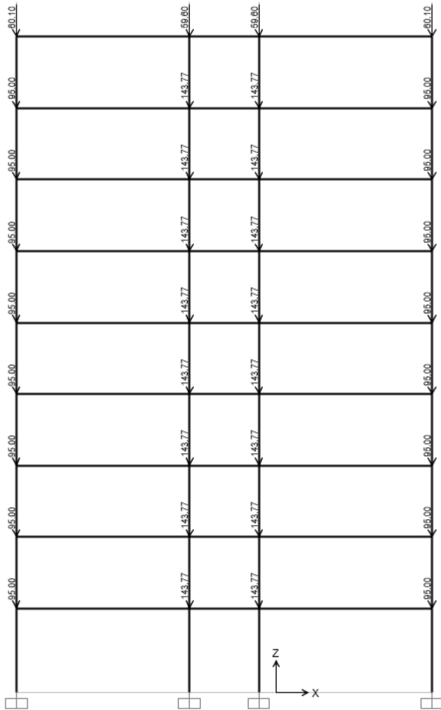
Sơ đồ tính tải tác dụng lên nút khung trục 4
