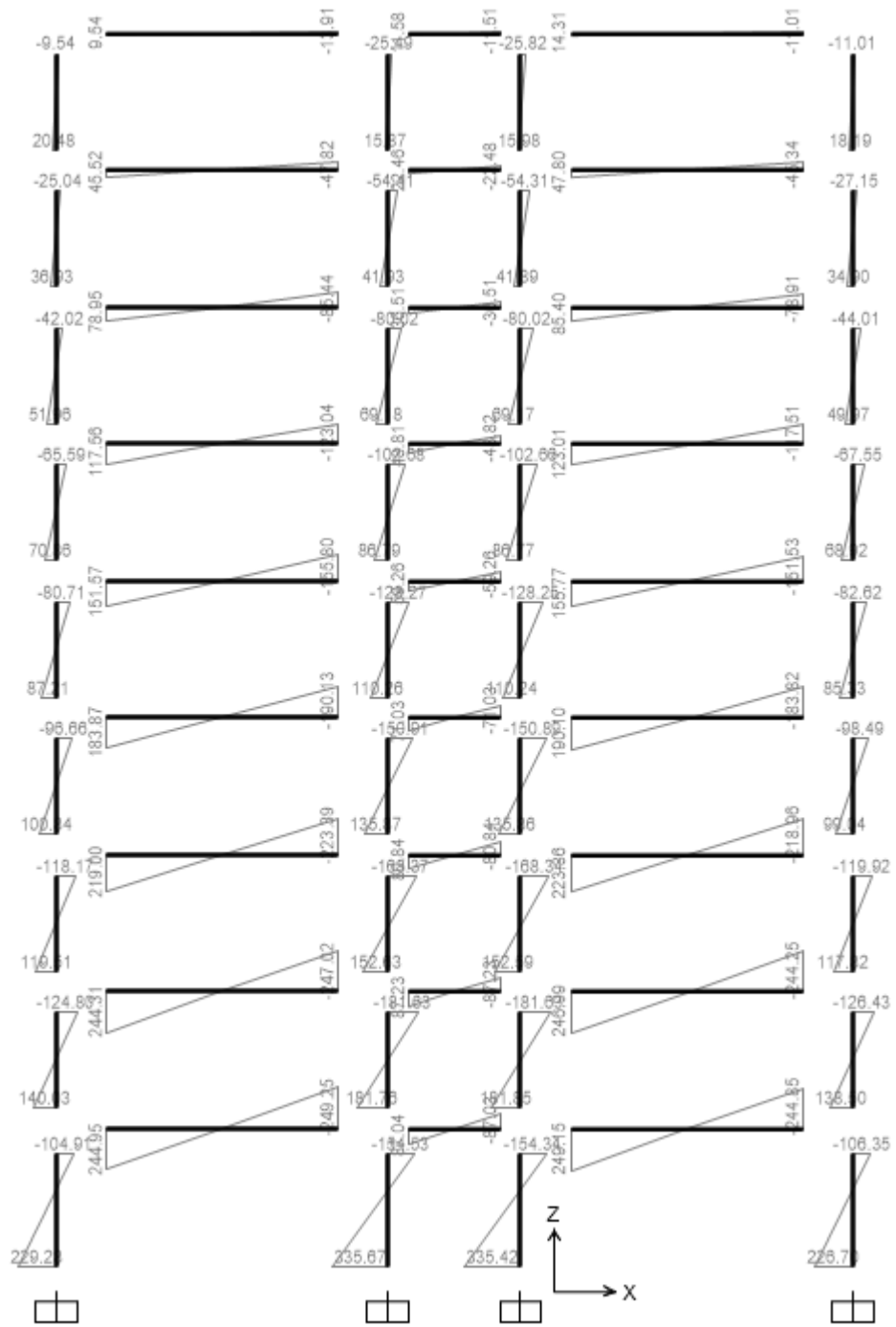
Momen do gió trái gây ra.
