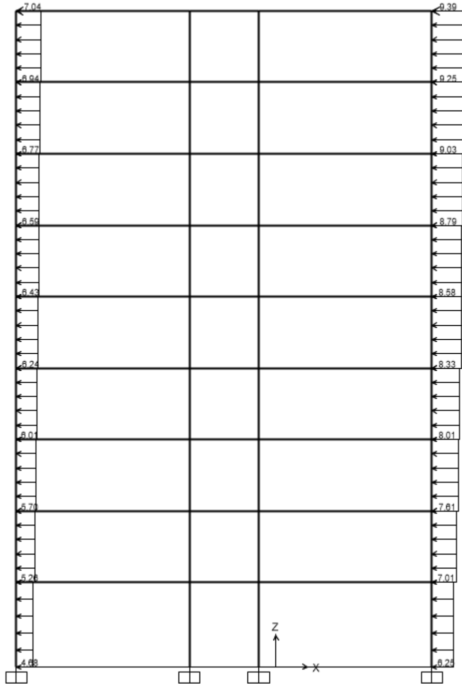
Sơ đồ gió phải tác dụng lên khung trục 4.
