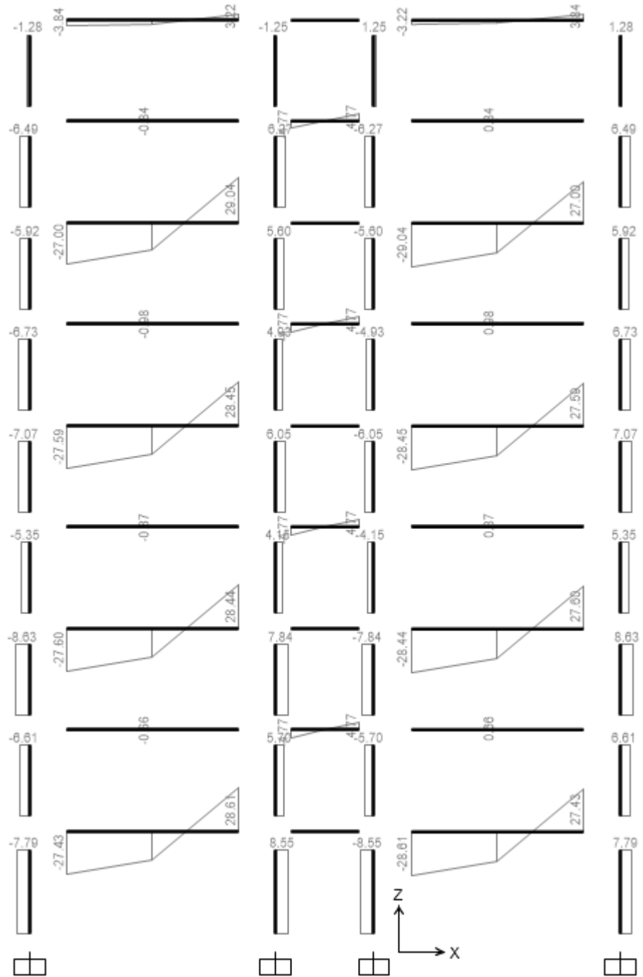
Lực cắt do hoạt tải 1 gây ra.
