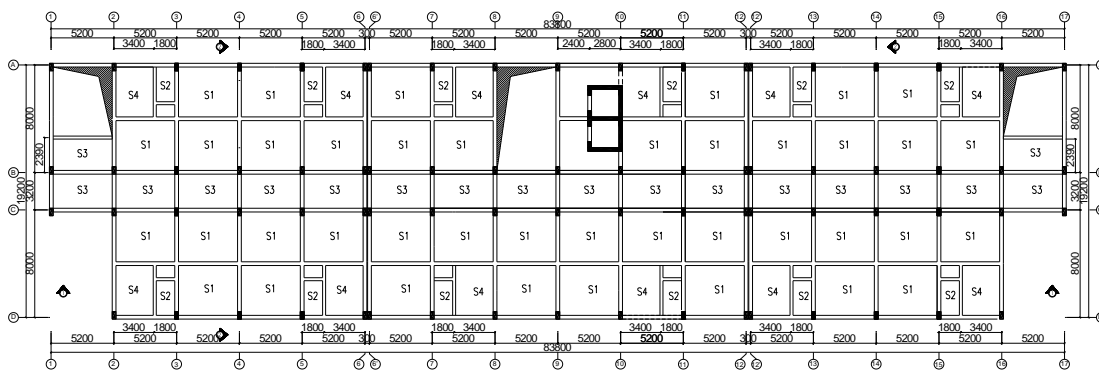
Mặt bằng kết cấu sàn tầng điển hình
