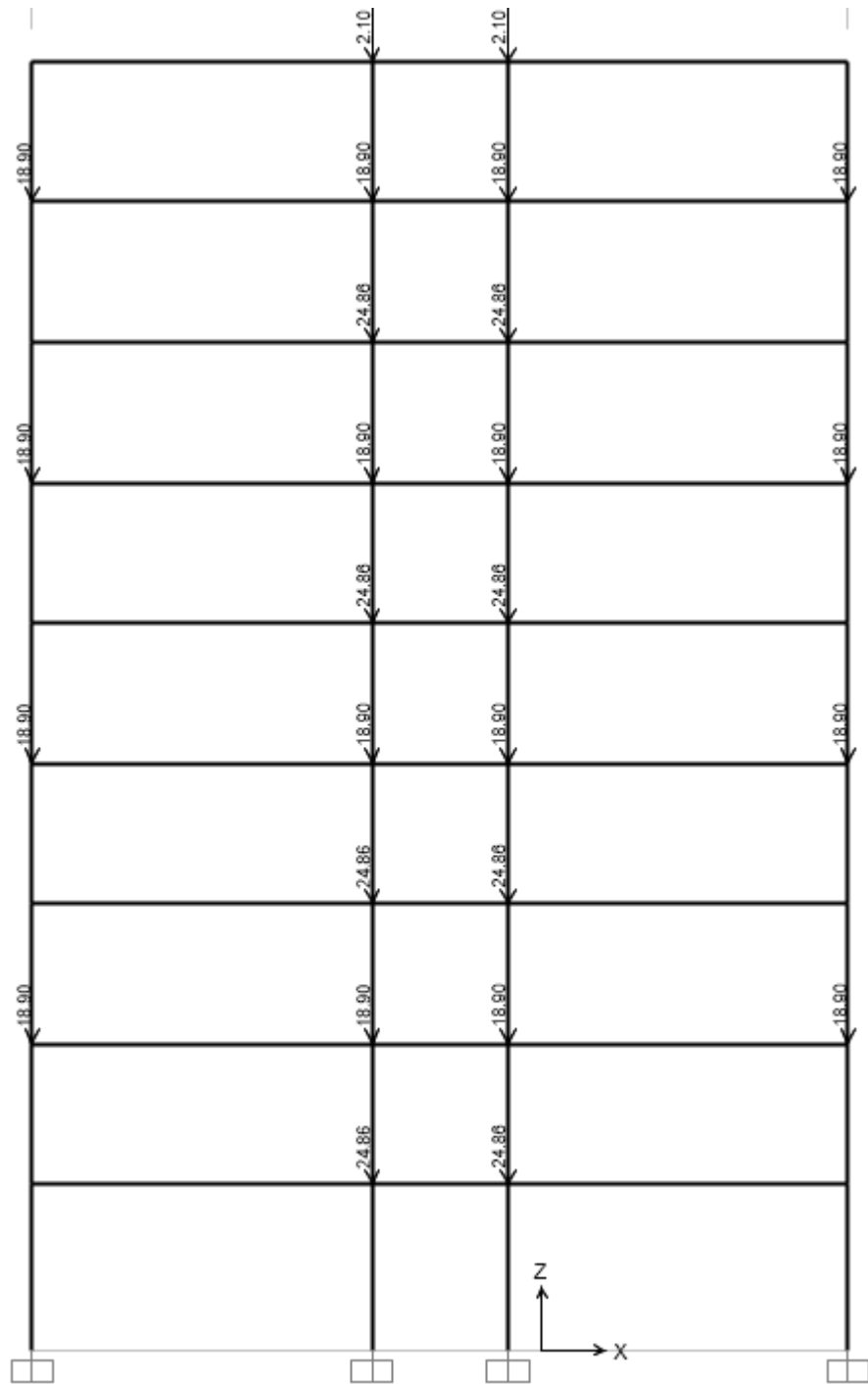
Sơ đồ hoạt tải 2 tác dụng lên nút khung trục 4.
