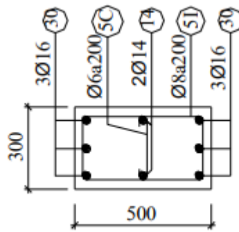
CẮT B8
