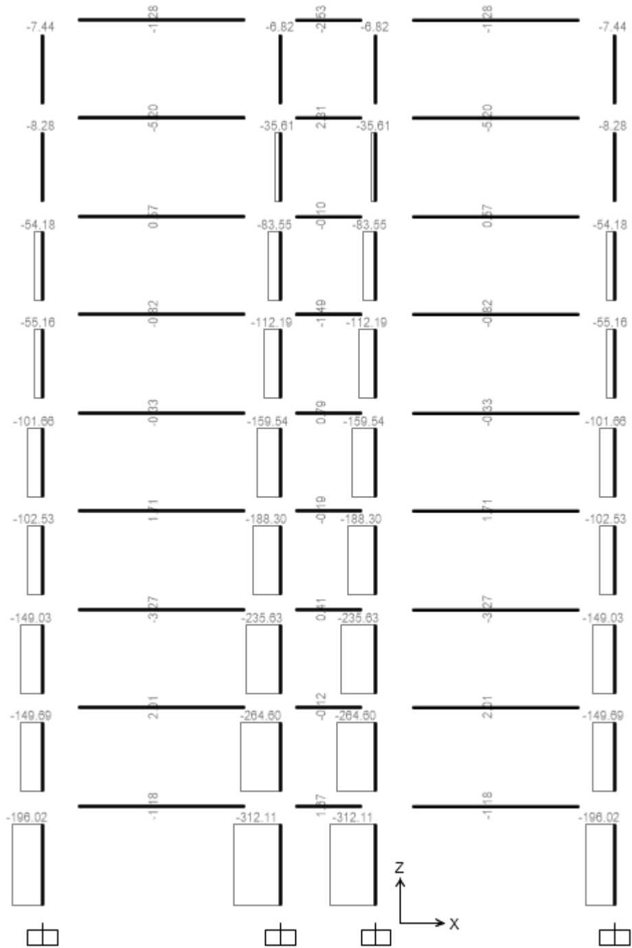
Lực dọc do hoạt tải 1 gây ra.
