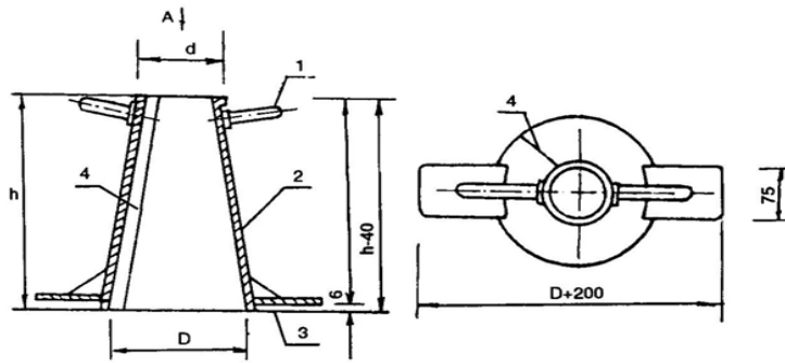
Hình 1 . 1. Tay cầm ; 2. Thành khuôn ; 3. Gói đặt chân ; 4. Đường hàn hoặc tán
