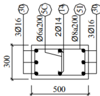
CẮT B8
