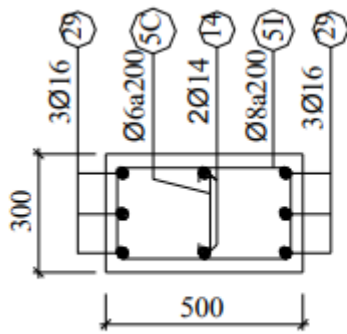
CẮT B7
