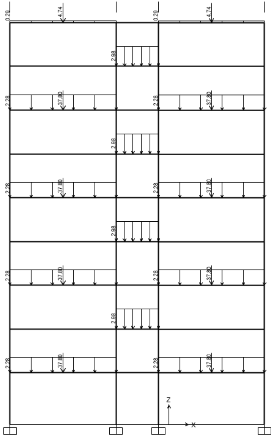
Sơ đồ hoạt tải 1 tác dụng lên thanh khung trục 4.
