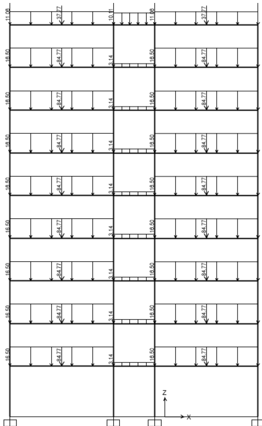
Sơ đồ tính tải tác dụng lên thanh khung trục 4
