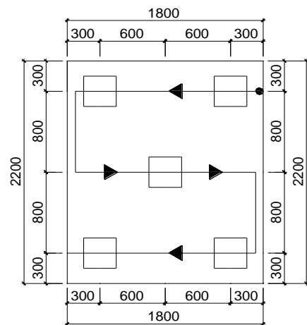
MÓNG M1 TL 1/50
