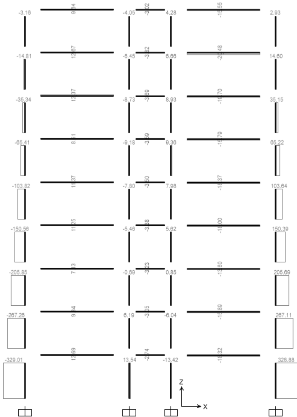
Lực dọc do gió phải gây ra.
