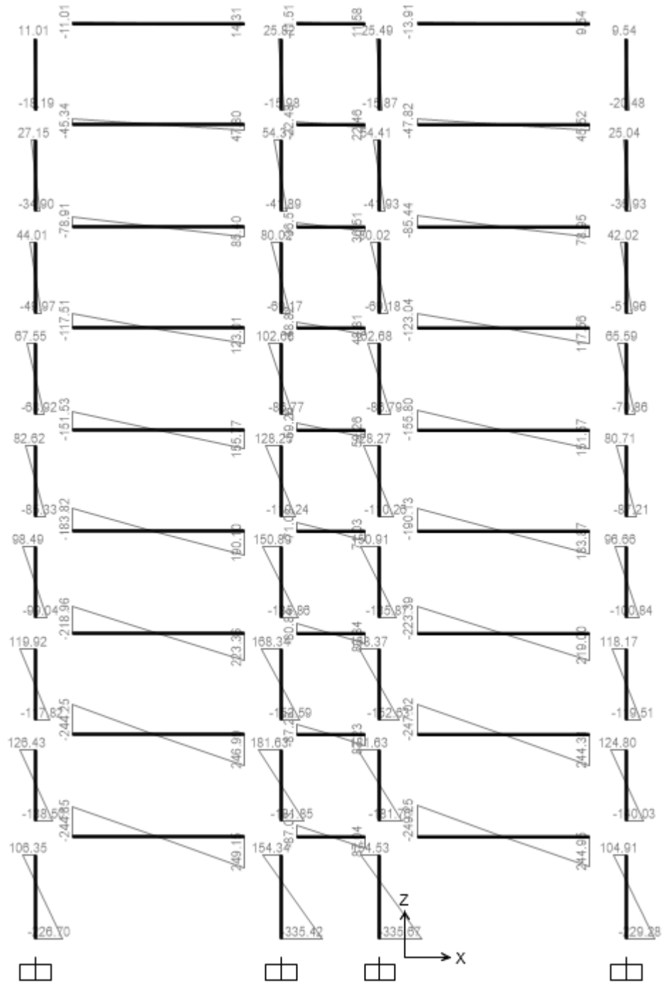
Momen do gió phải gây ra.
