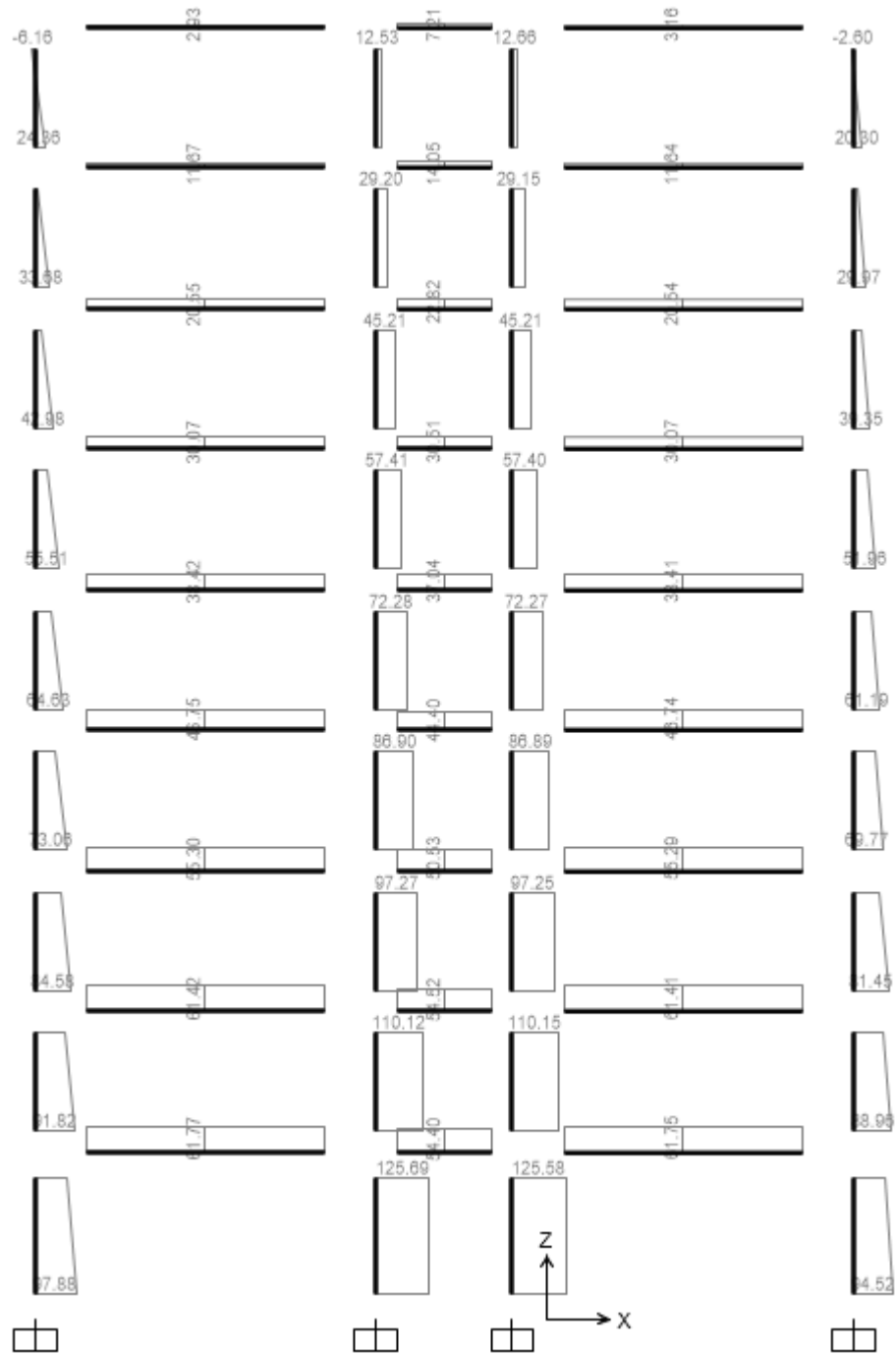
Lực cắt do gió trái gây ra.
