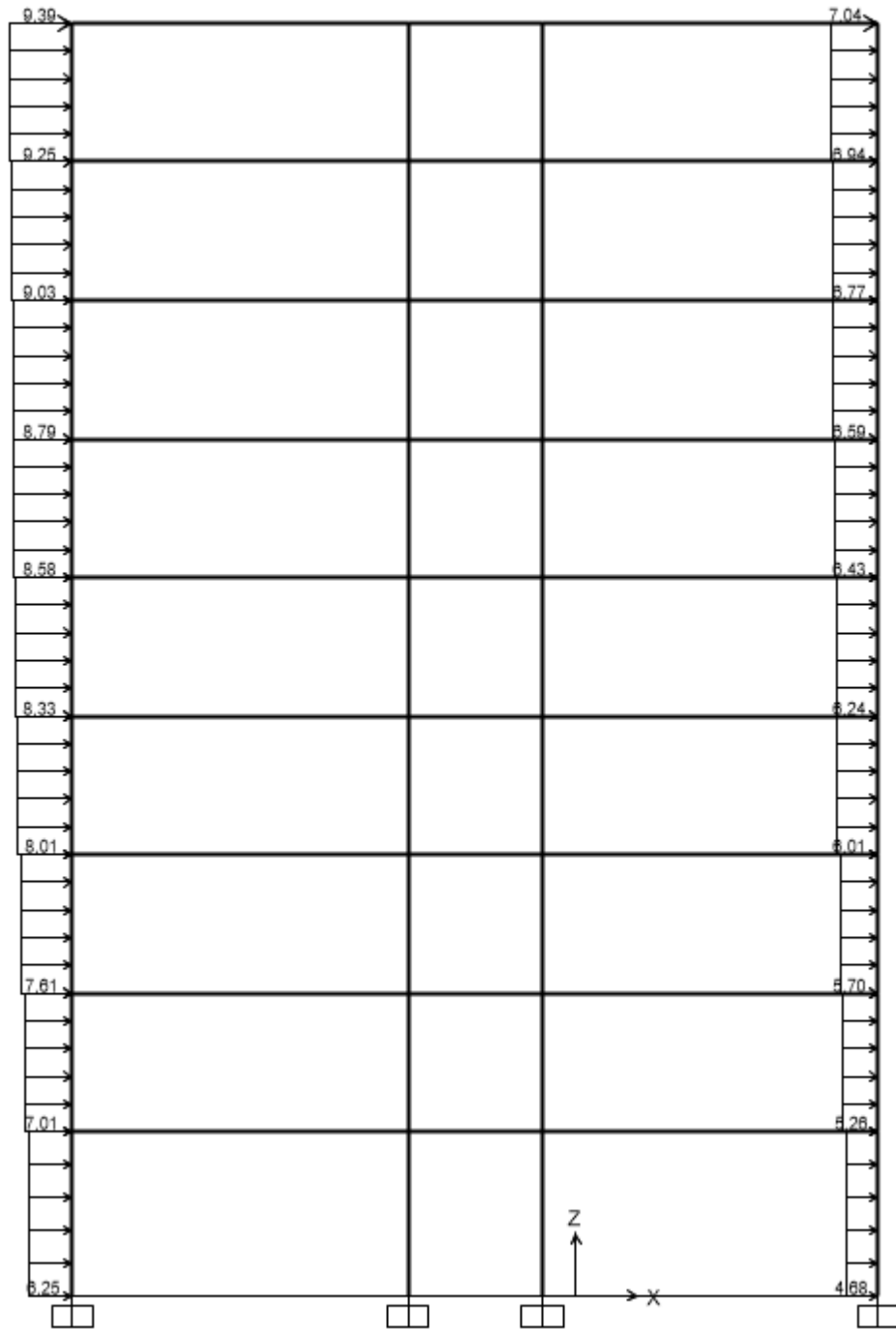
Sơ đồ gió trái tác dụng lên khung trục 4.
