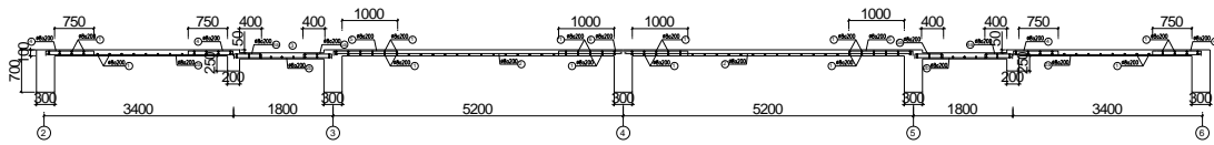
Mặt cắt 1-1
