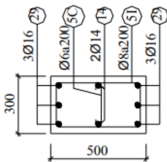
CẮT B7
