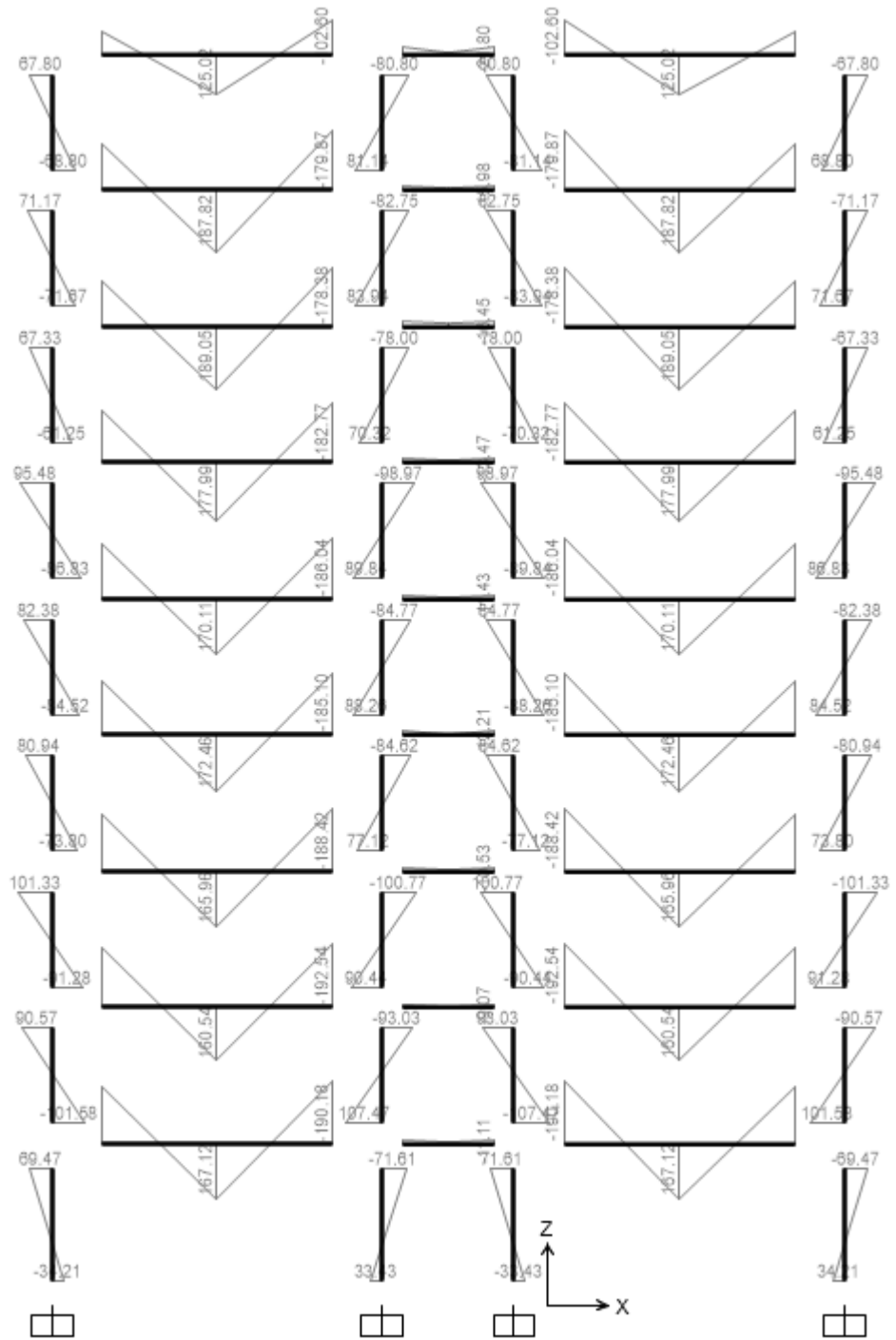
Momen do tĩnh tải gây ra.
