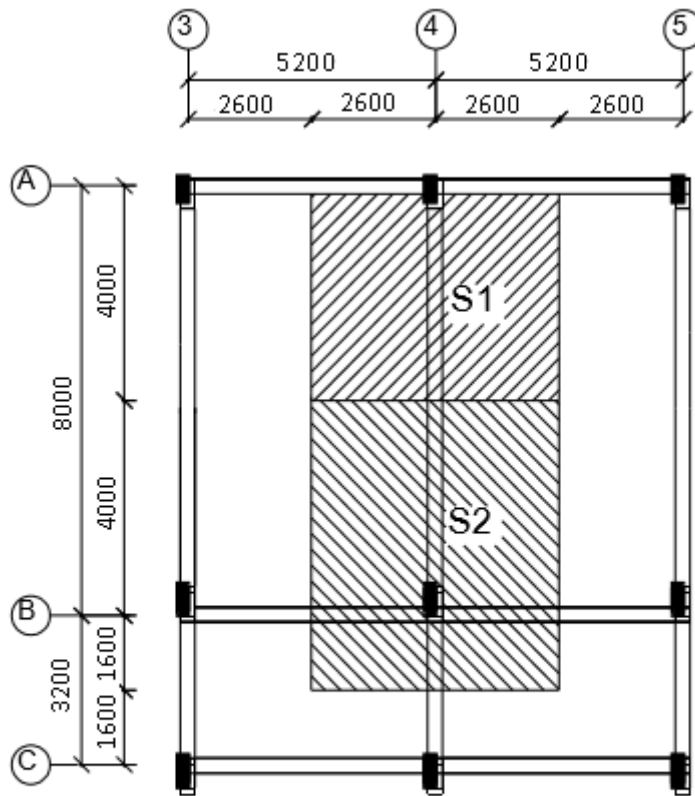
Diện Truyền Tải Của Cột
