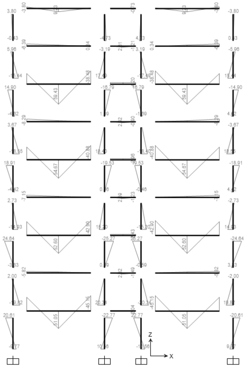
Momen do hoạt tải 1 gây ra.
