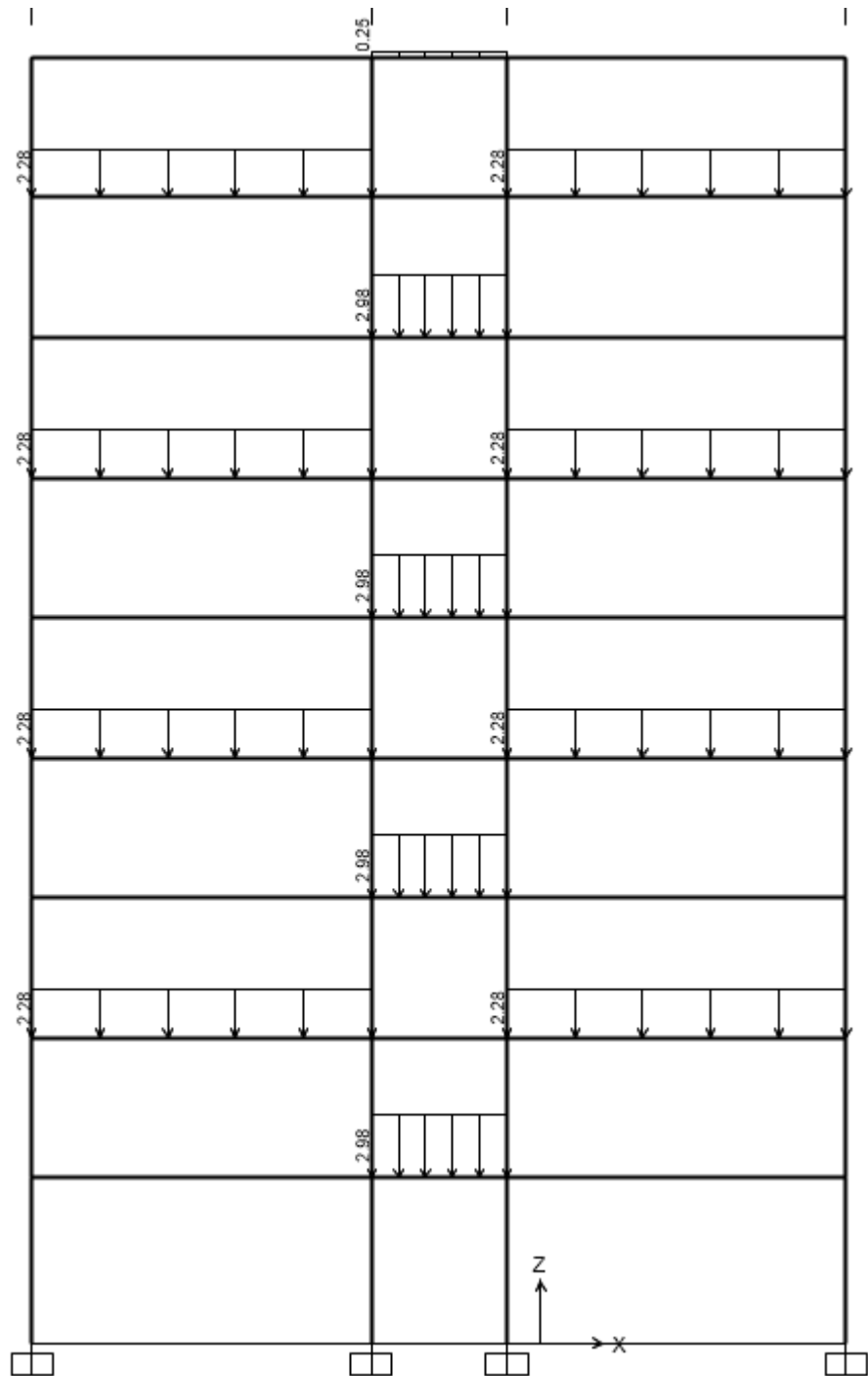
Sơ đồ hoạt tải 2 tác dụng lên thanh khung trục 4.
