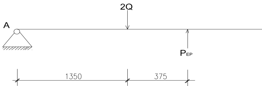
Hình : Kiểm tra chống lật tại điểm A
