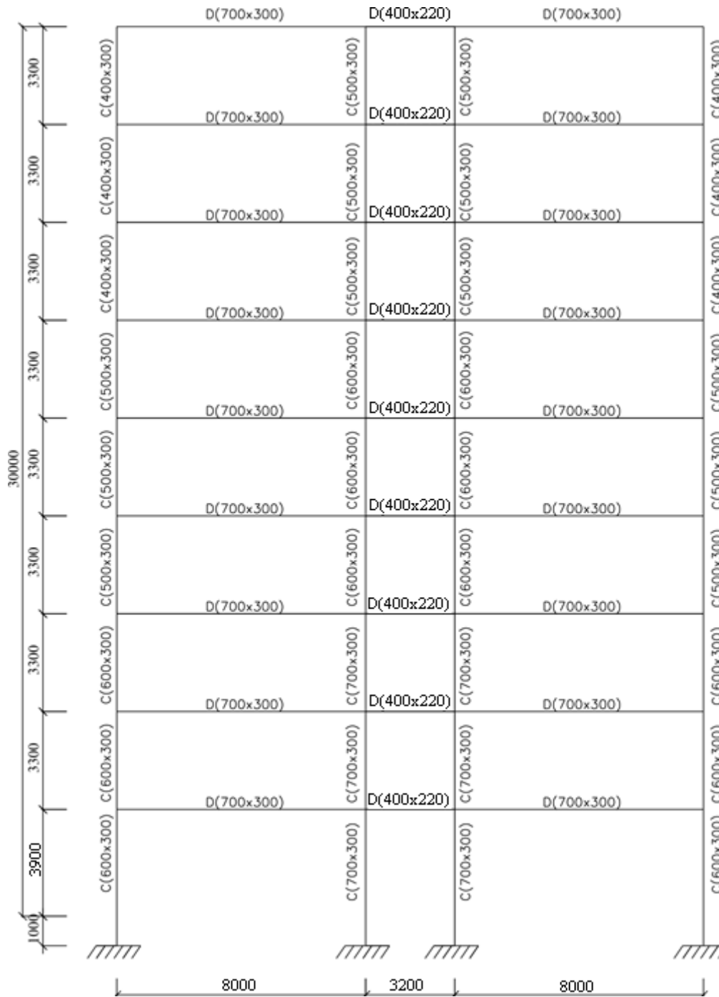
Sơ đồ hình học khung trục 4
