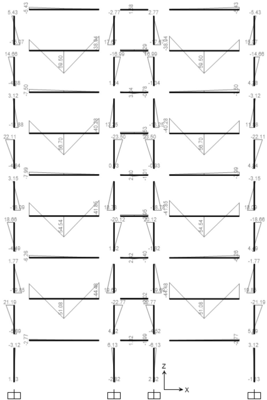
Momen do hoạt tải 2 gây ra.
