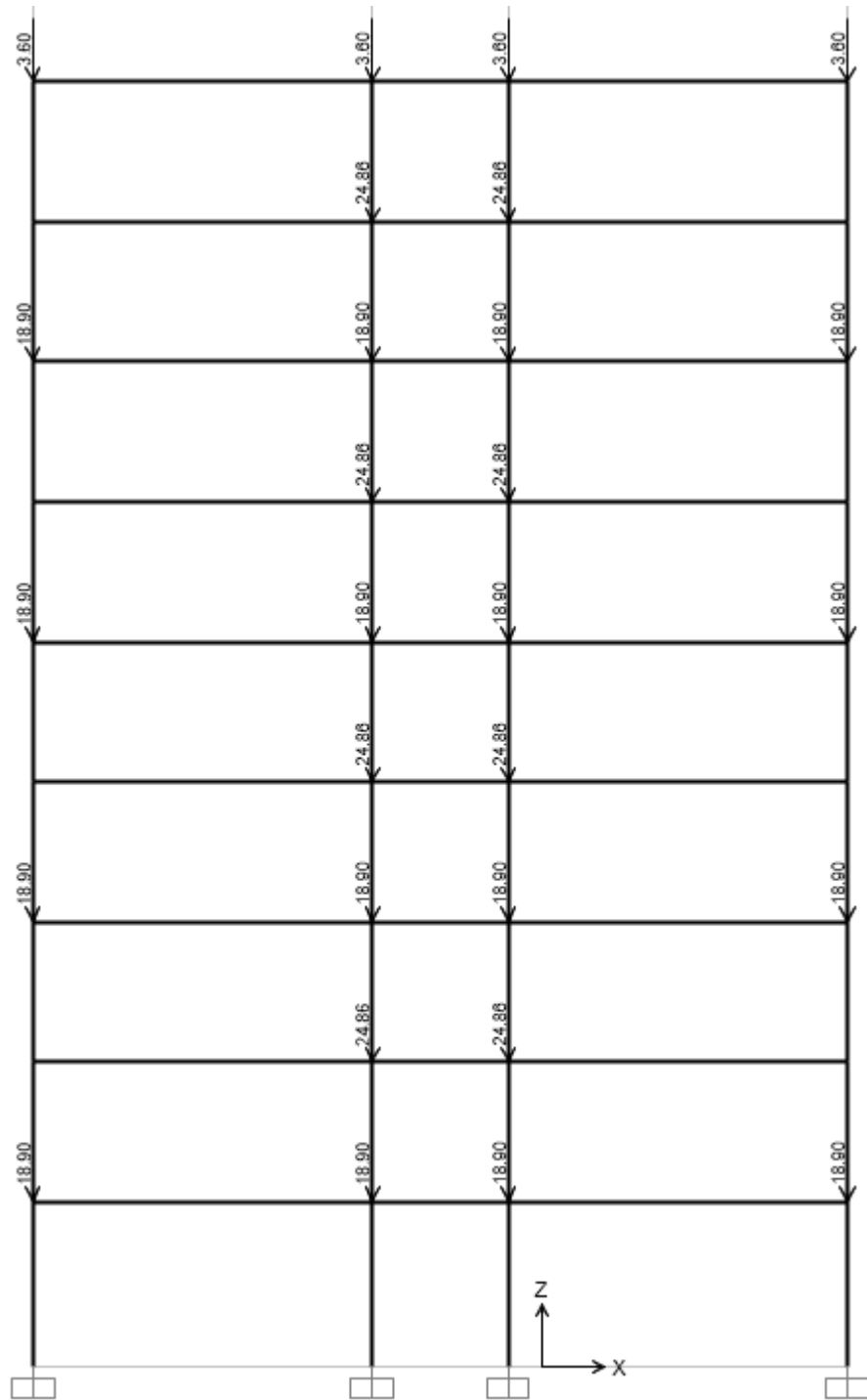
Sơ đồ hoạt tải 1 tác dụng lên nút khung trục 4
