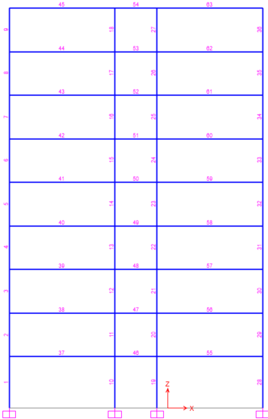
Sơ đồ các phần tử dầm và cột của khung.
