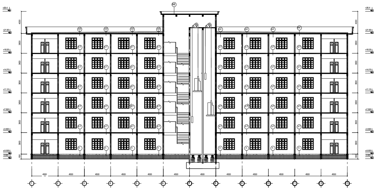
mặt c 3/4 a-a - tl 1/100
