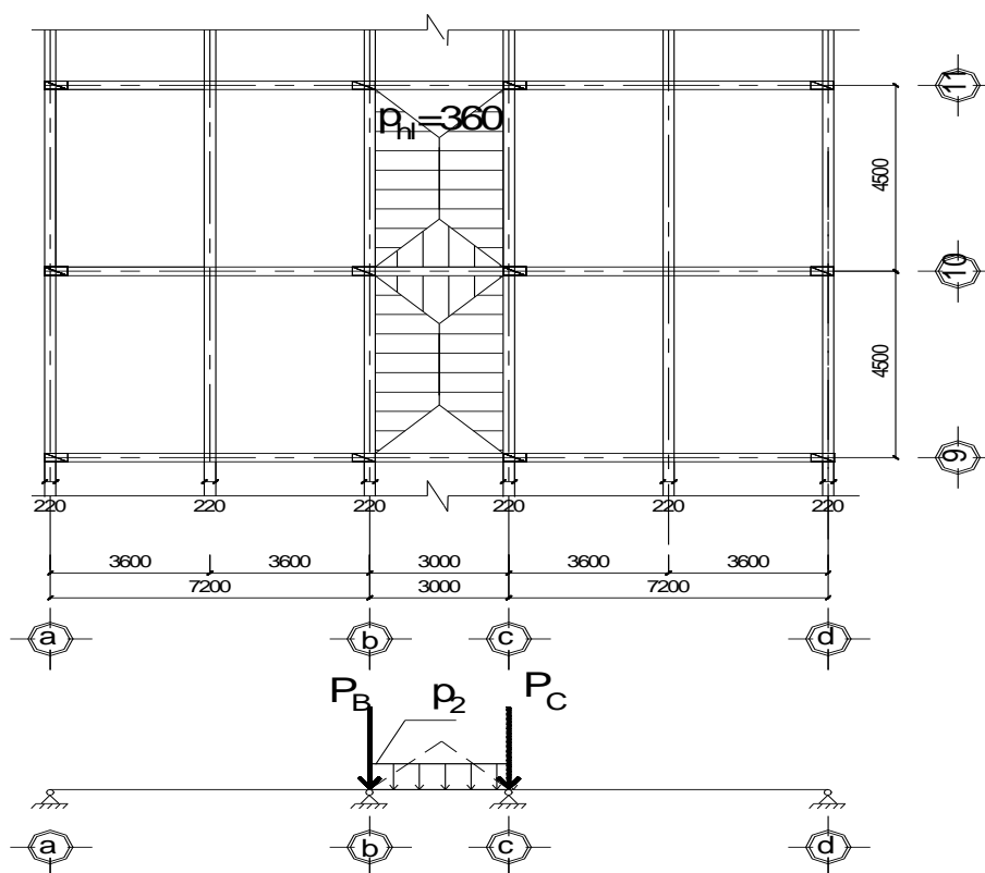
Trường hợp 2: ( tải truyền vào nhịp BC )
