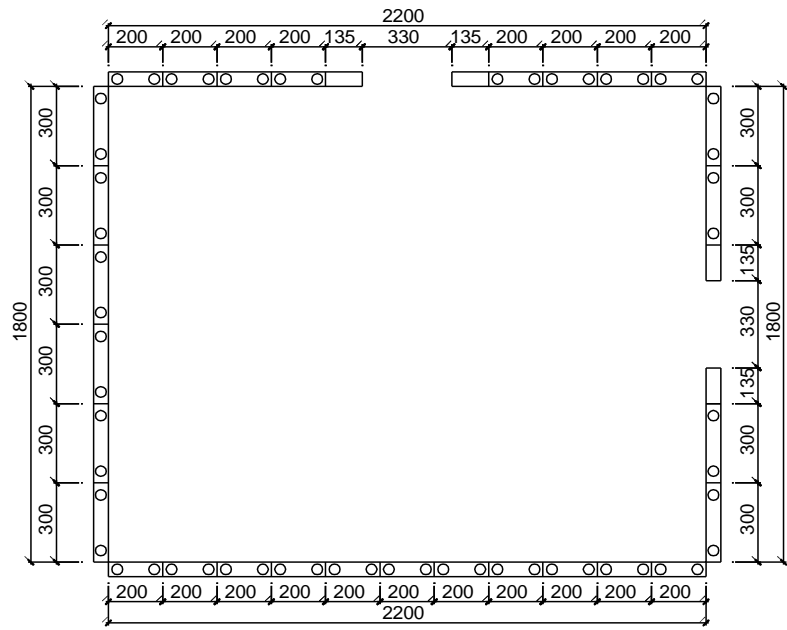
mặt b»ng mǎng A - 1
