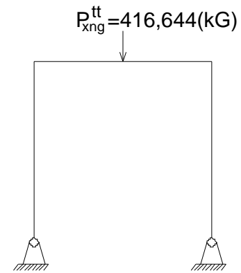
Sơ đồ truyền tải lên cột chống
