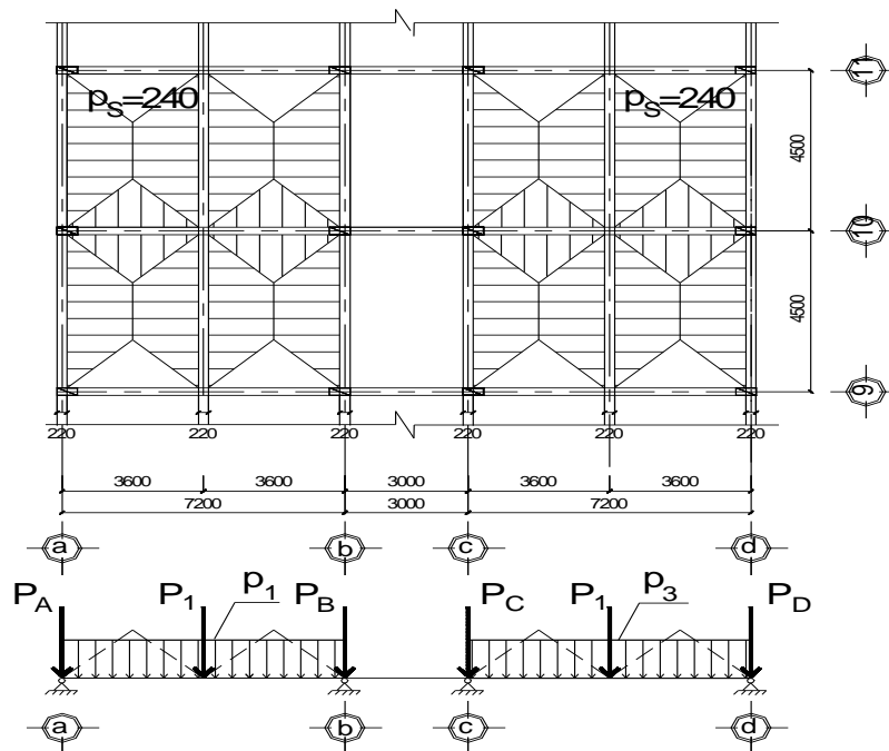
SƠ ĐỒ HOẠT TẢI TÁC DỤNG TRƯỜNG HỢP 1
