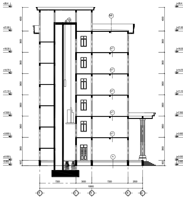
mặt c 3/4 b-b - tl 1/100
