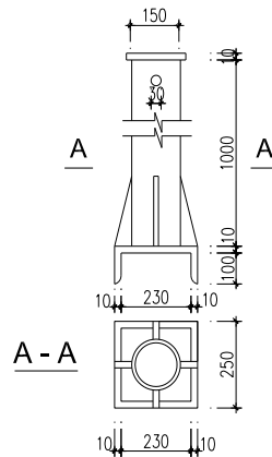
CHI TIẾT CỌC DẪN ÉP ÂM
