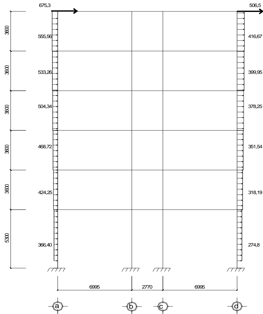
Sơ đồ phân bố tải trọng gió tác dụng lên khung k10
