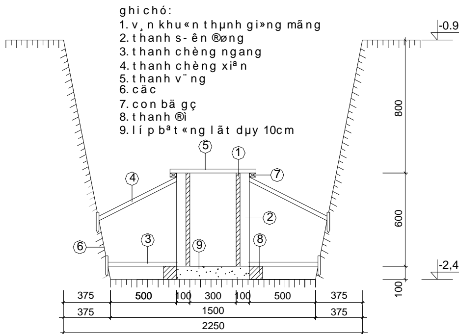
Biểu đồ 1.0 v, n khu«n gi»ng mǎng gm2
