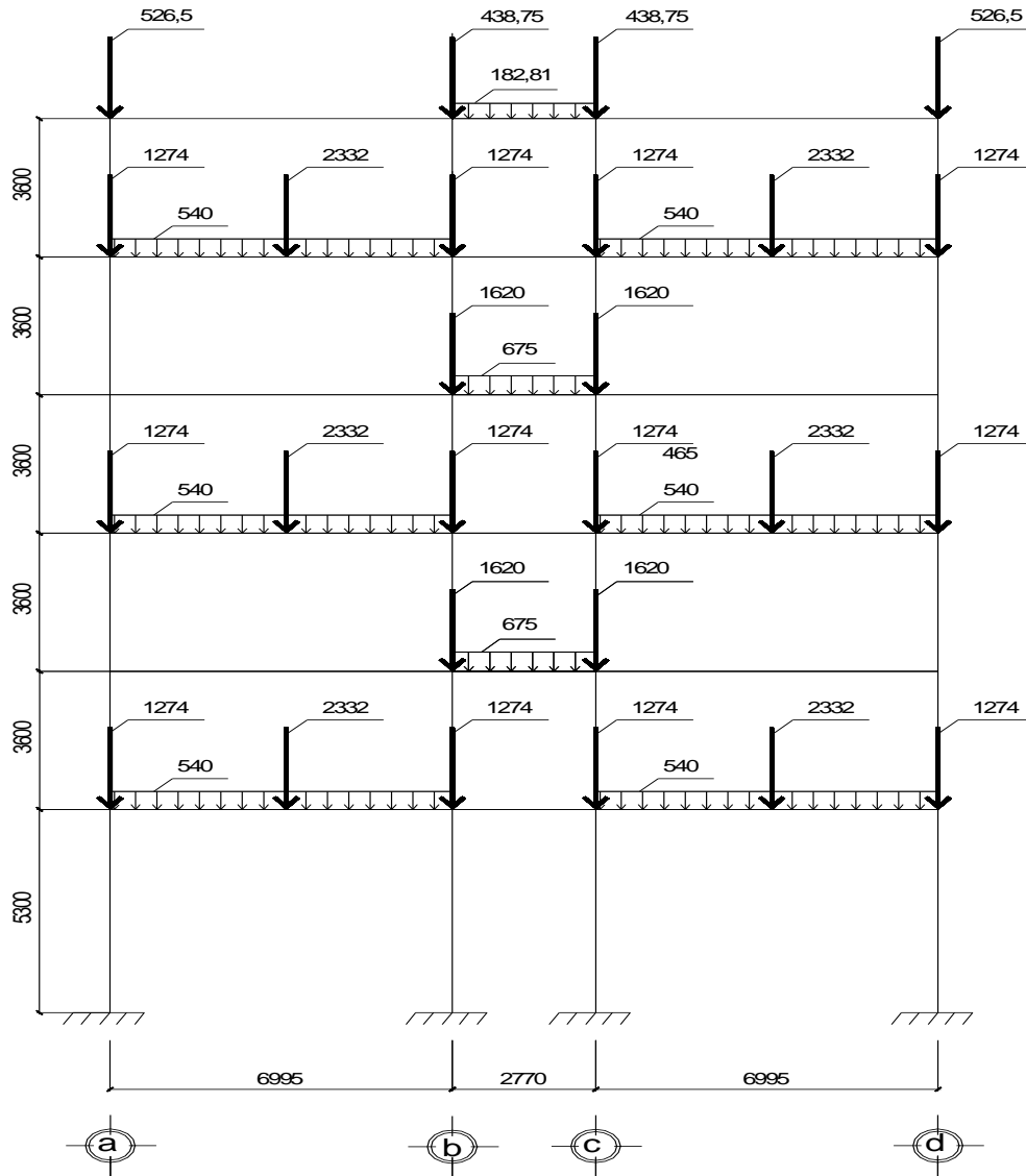
Sơ đồ tải trọng sàn hành lang và tải trọng sê nô truyền vào cột
