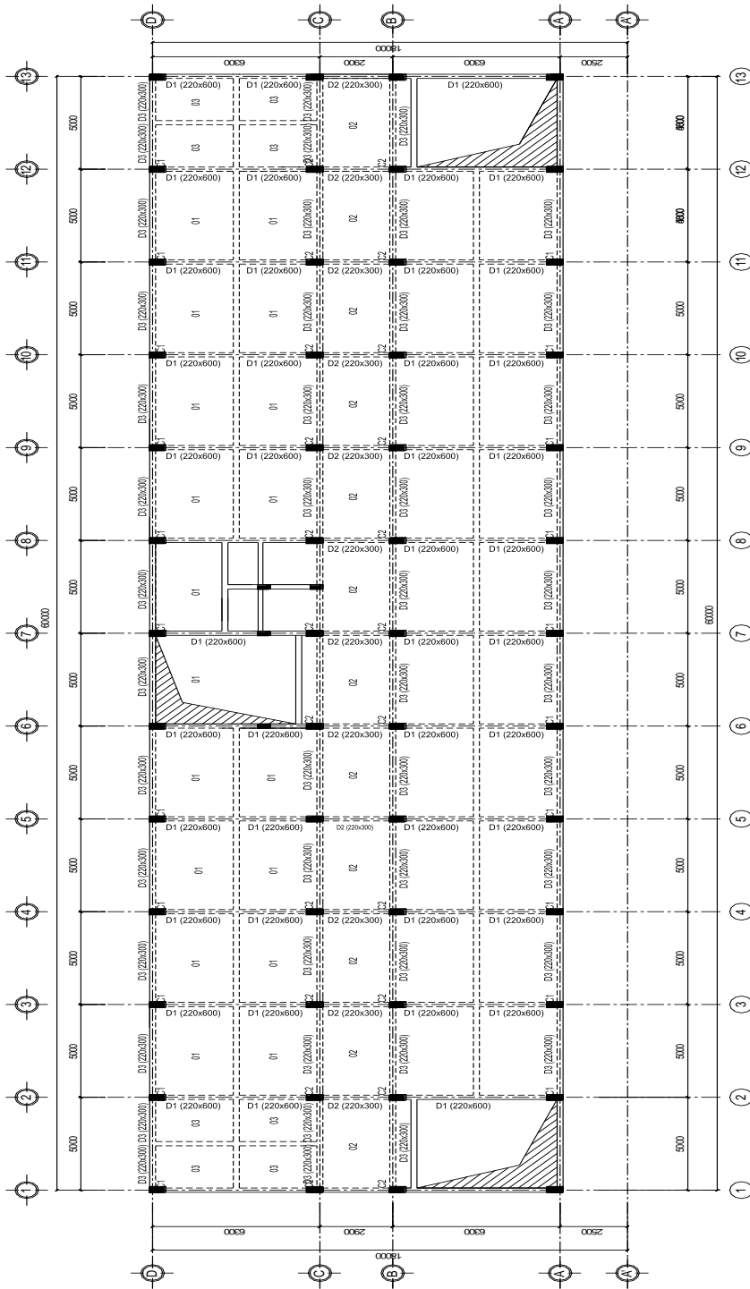
MẶT BẰNG KẾT CẤU SÀN TẦNG ĐIỀN HÌNH
