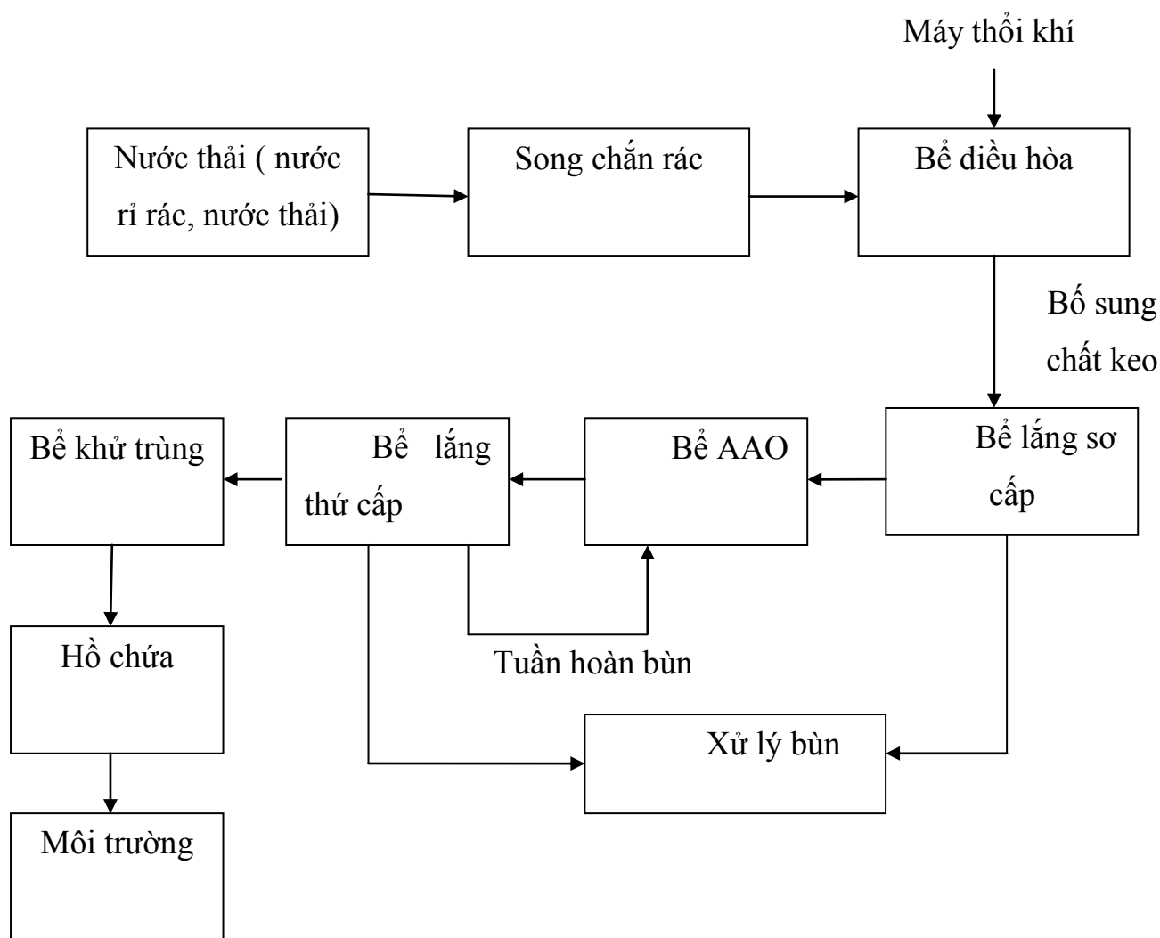
Hình 2.5. Quy trình xử lý nước thải tại nhà máy chế biến phân Compost.
