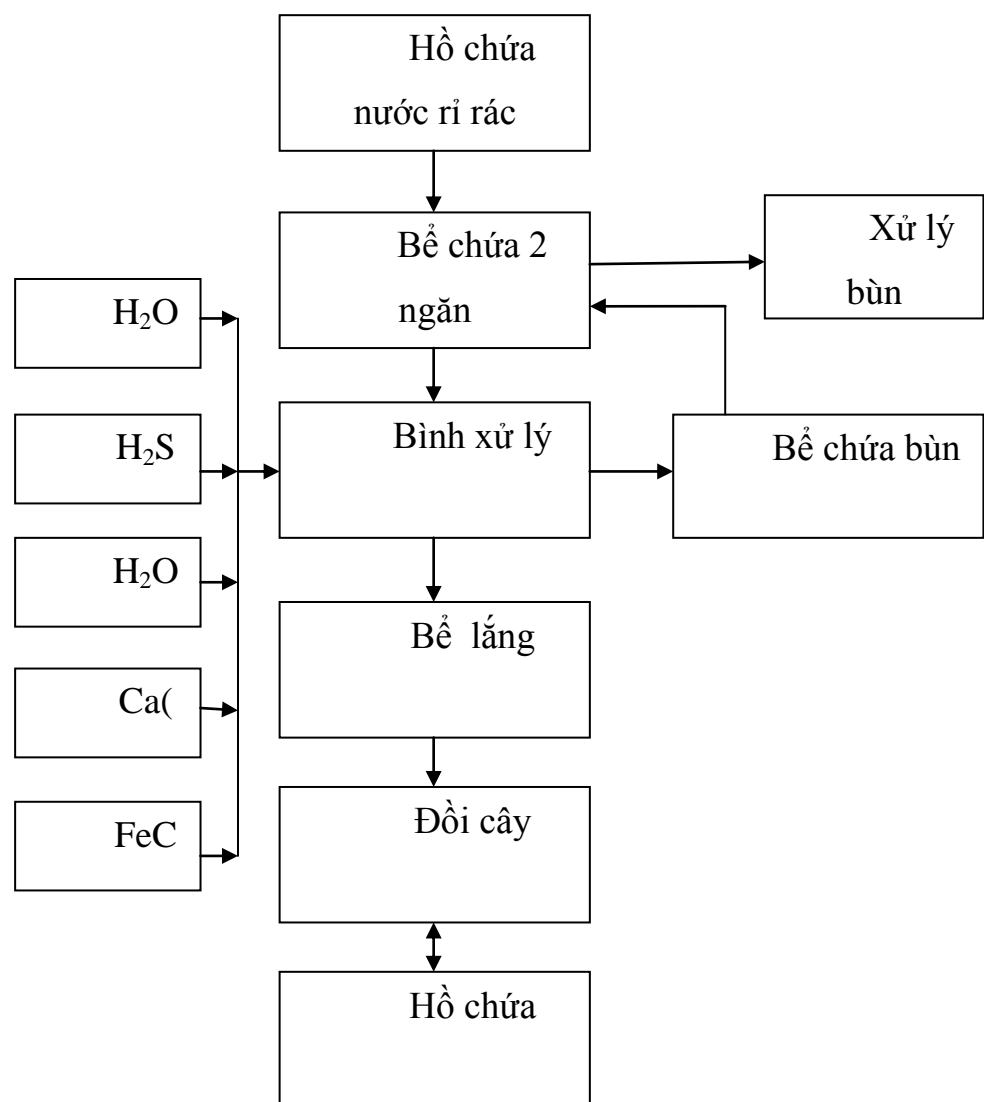
Hình 2.3. Quy trình xử lý nước thải tại ô rác số 2
