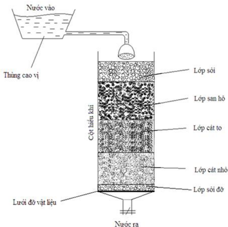
Hình 2.3: Sơ đồ cột hiếu khí
