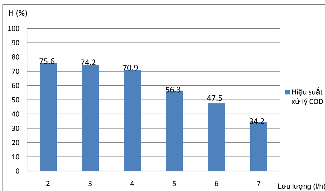
Hình 3.1: Ảnh hưởng của lưu lượng dòng tới hiệu quả xử lý COD
