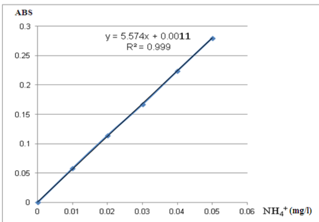
Hình 2.2: Biểu đồ đường chuẩn \text{NH}_4^+
