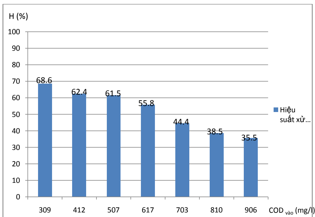
Hình 3.2: Ảnh hưởng của tải trọng COD tới hiệu quả xử lý COD
