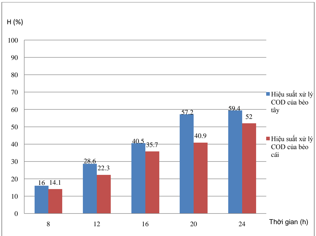
Hình 3.4: Ảnh hưởng của thời gian nuôi bèo tới hiệu quả xử lý COD
