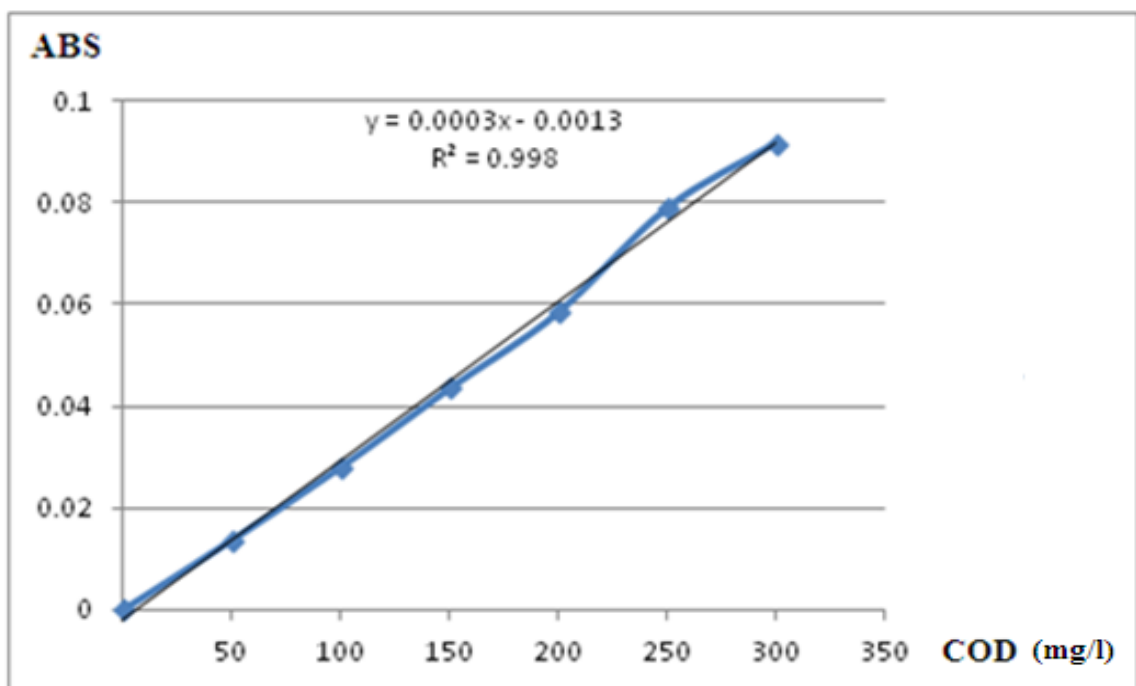
Hình 2.1: Biểu đồ đường chuẩn COD
