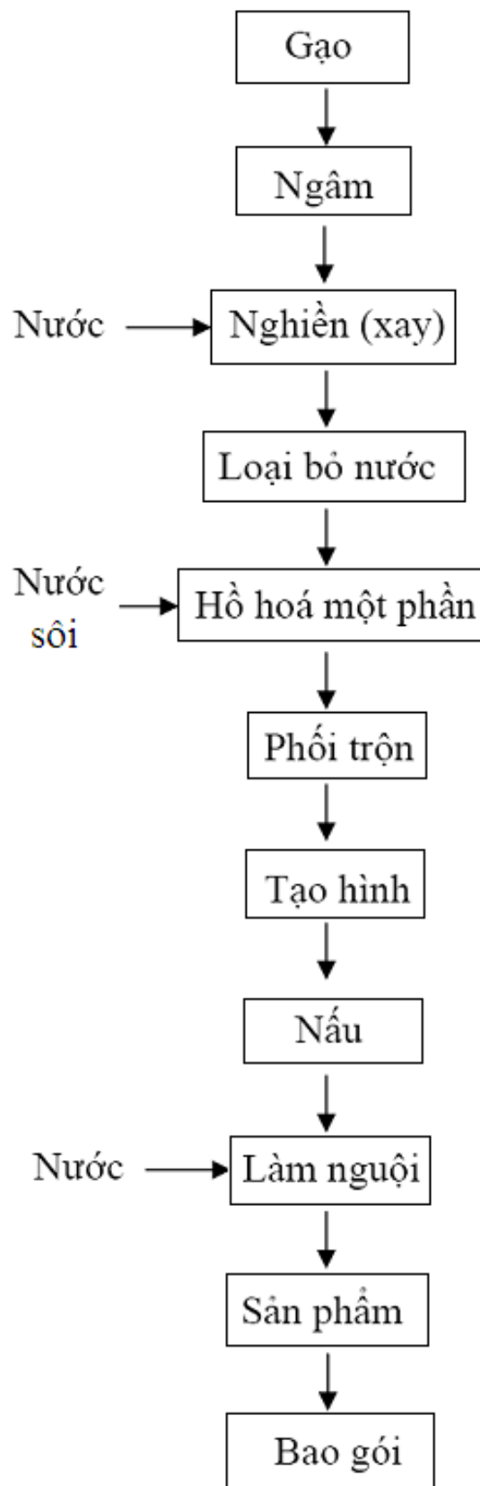
Hình 1.2: Quy trình sản xuất bún
