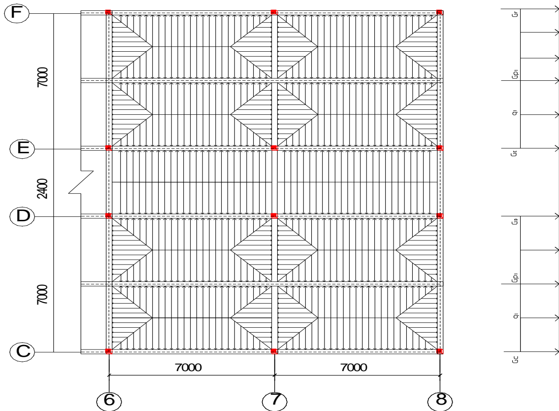
MẶT BẰNG PHÂN TĨNH TẢI TẦNG 5, 6, 7
