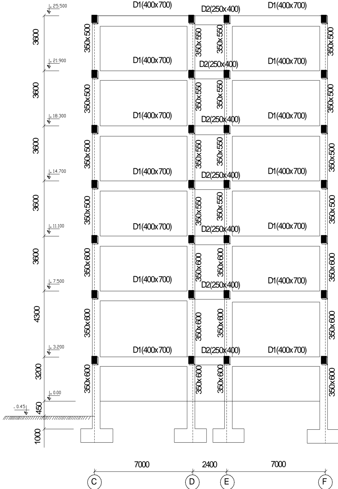
SƠ ĐỒ HÌNH HỌC KHUNG NGANG TRỤC 7
