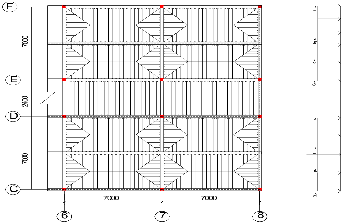
MẶT BẰNG PHÂN TẢI TẦNG MÁI
