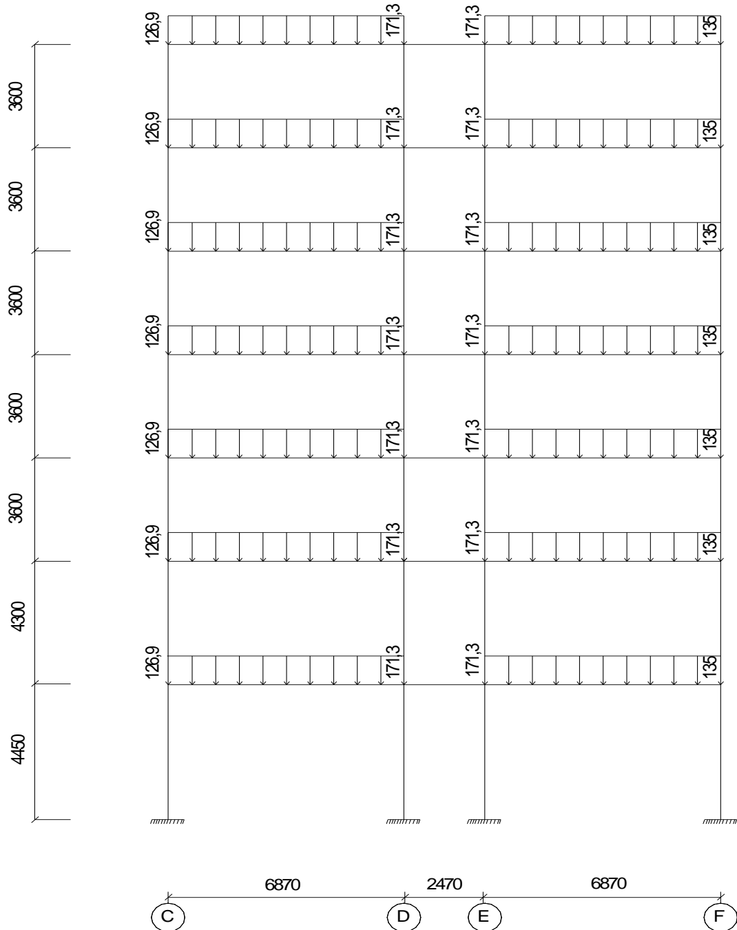
SƠ ĐỒ TÍNH TẢI TÁC DỤNG LÊN KHUNG TRỤC 7
