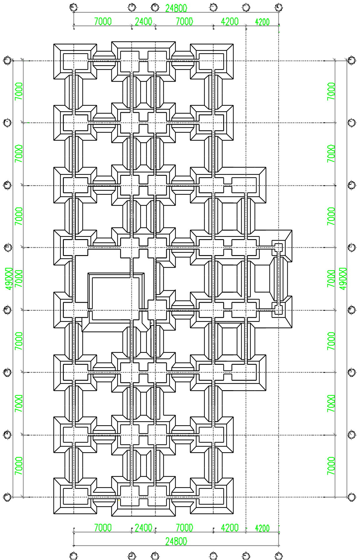
MẶT BẰNG THIẾT KẾ HỒ ĐÀO
