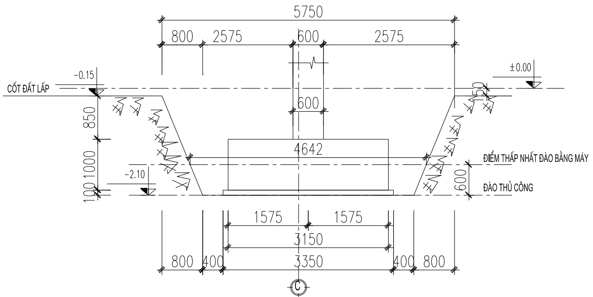
MẶT CẮT DỌC HỒ MÓNG M1( TRỤC C, F)
