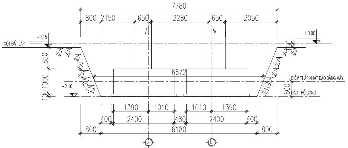
MẶT CẮT DỌC HỒ MÓNG M2( TRỤC D, E)
