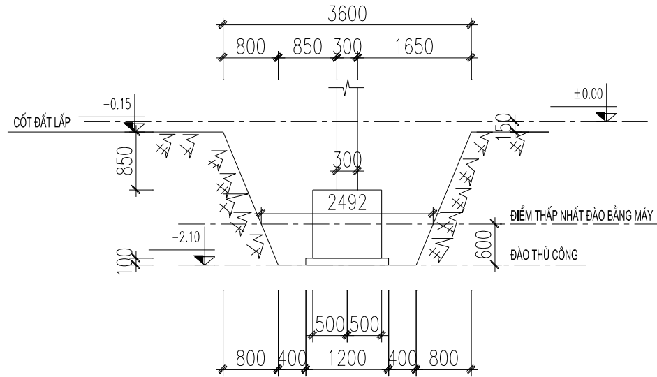
MẶT CẮT HỒ MÓNG M3( TRỤC A)
