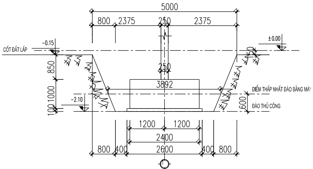
MẶT CẮT NGANG HỒ MÓNG M2( TRỤC D, E)
