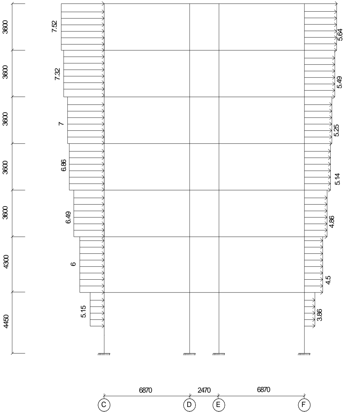
SƠ ĐỒ GIÓ TRÁI TÁC DỤNG LÊN KHUNG TRỤC 7
