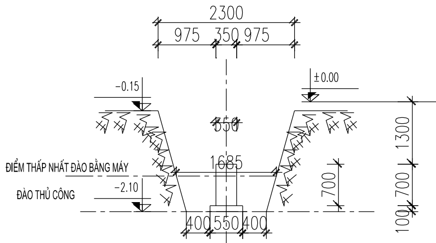
MẶT CẮT NGANG GIƯỜNG MÓNG
