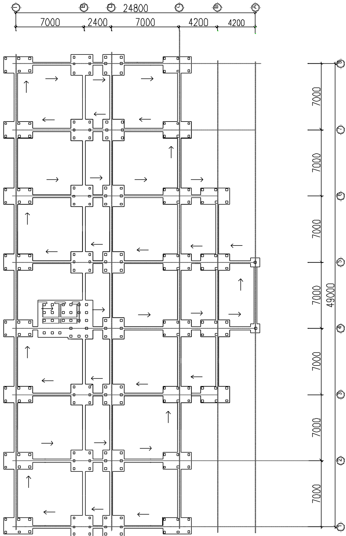
SƠ ĐỒ ÉP CỌC MÓNG
