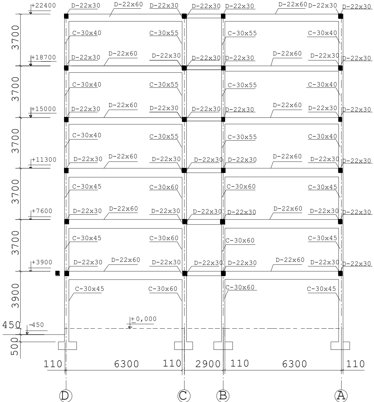
SƠ ĐỒ HÌNH HỌC KHUNG TRỤC 10
