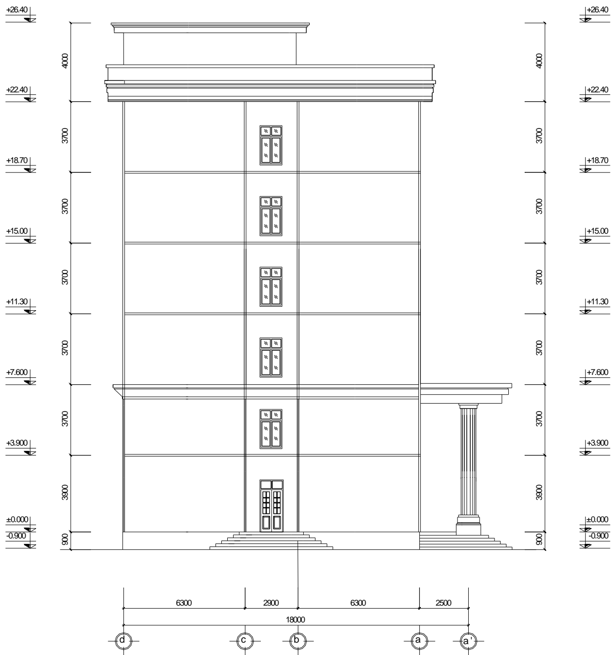
mặt ®ong tróc D - a' - tl 1/100
