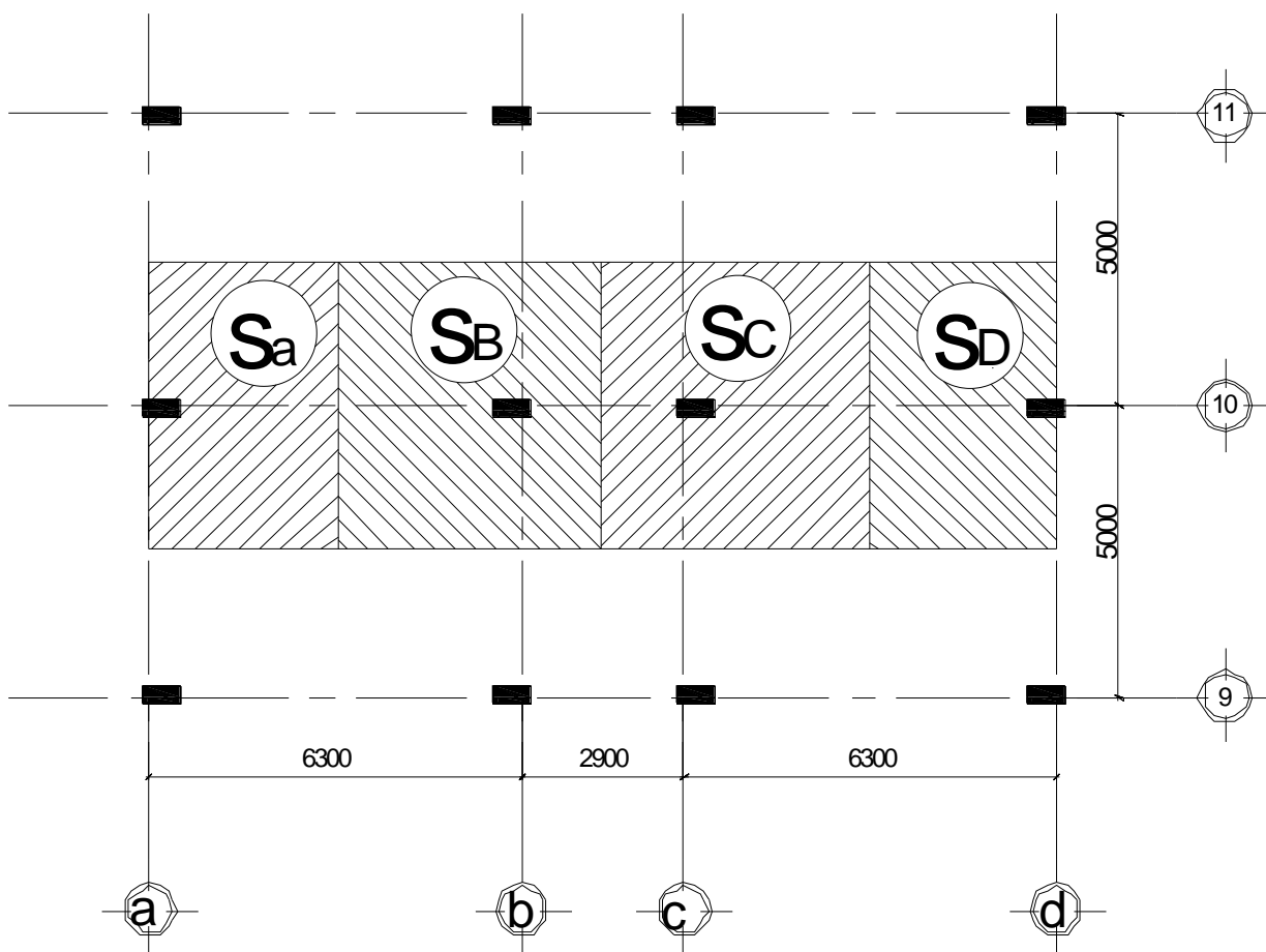
DIỆN CHỊU TẢI CỦA CỘT.
