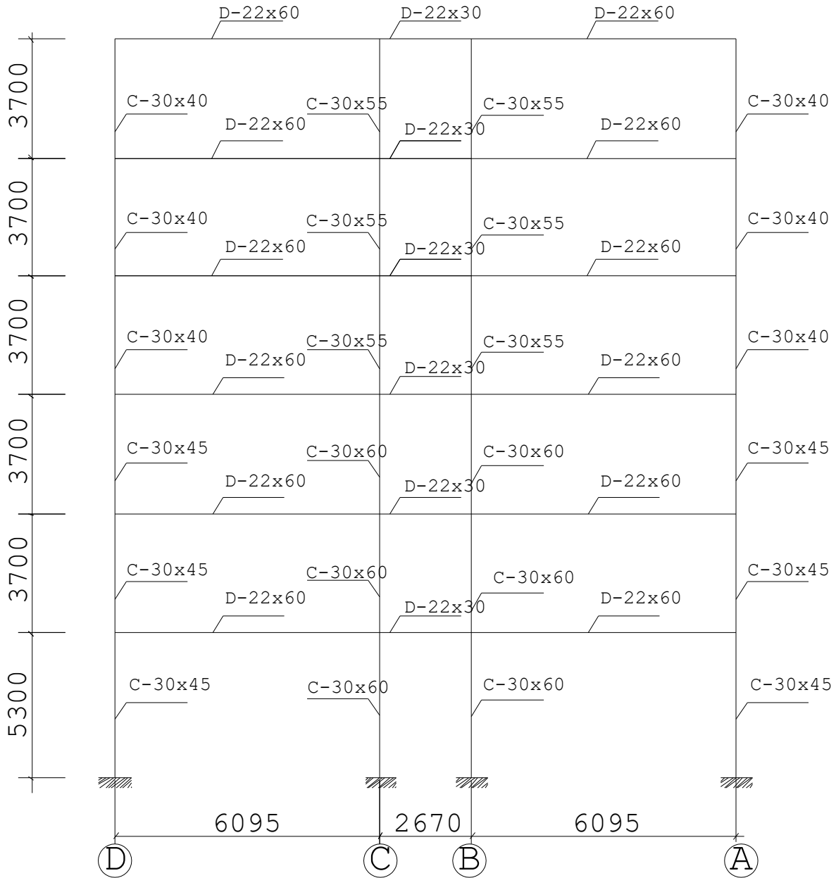
SƠ ĐỒ KẾT CẤU KHUNG TRỤC 10
