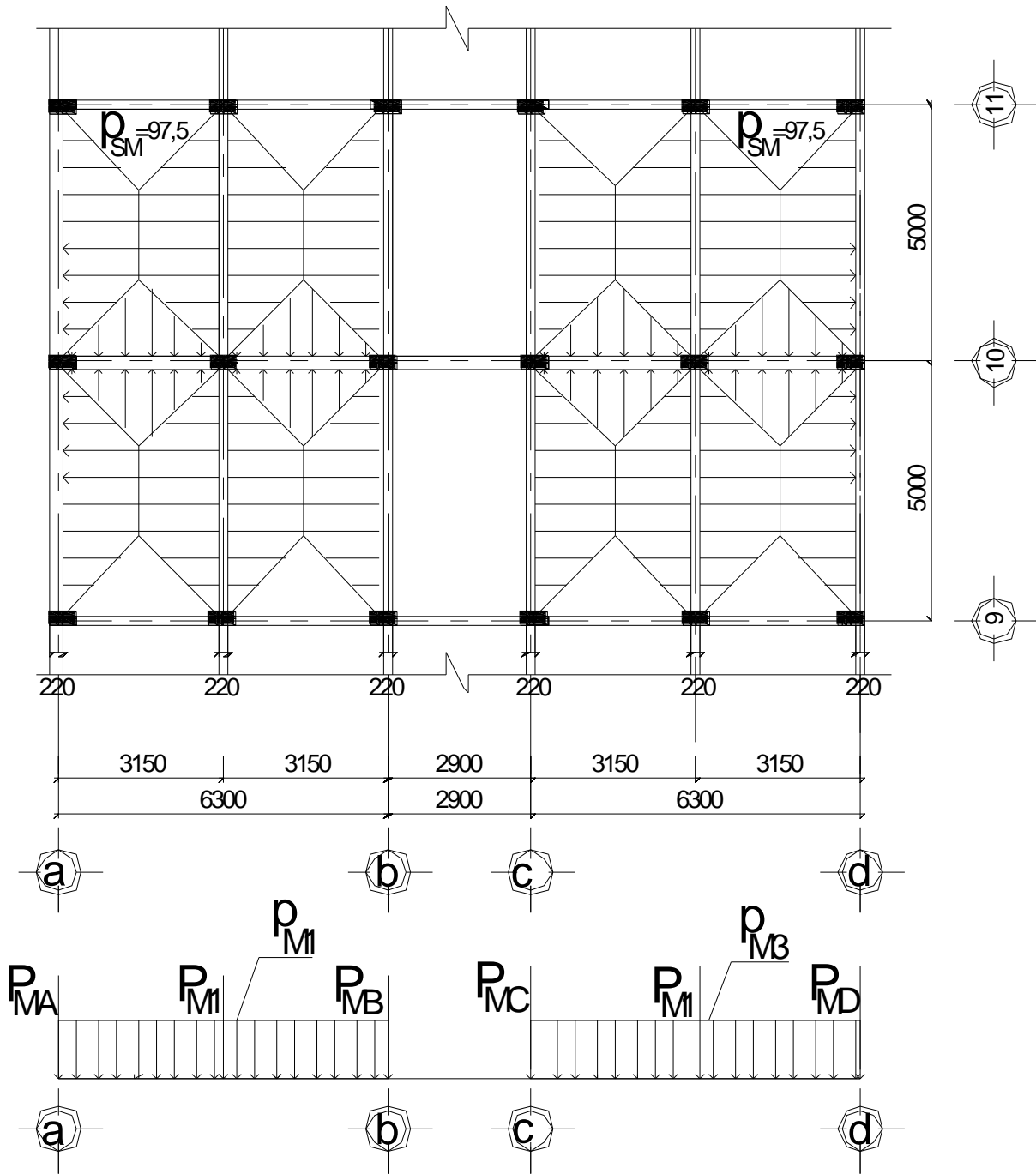
SƠ ĐỒ HOẠT TẢI MÁI TÁC DỤNG TRƯỜNG HỢP 1
