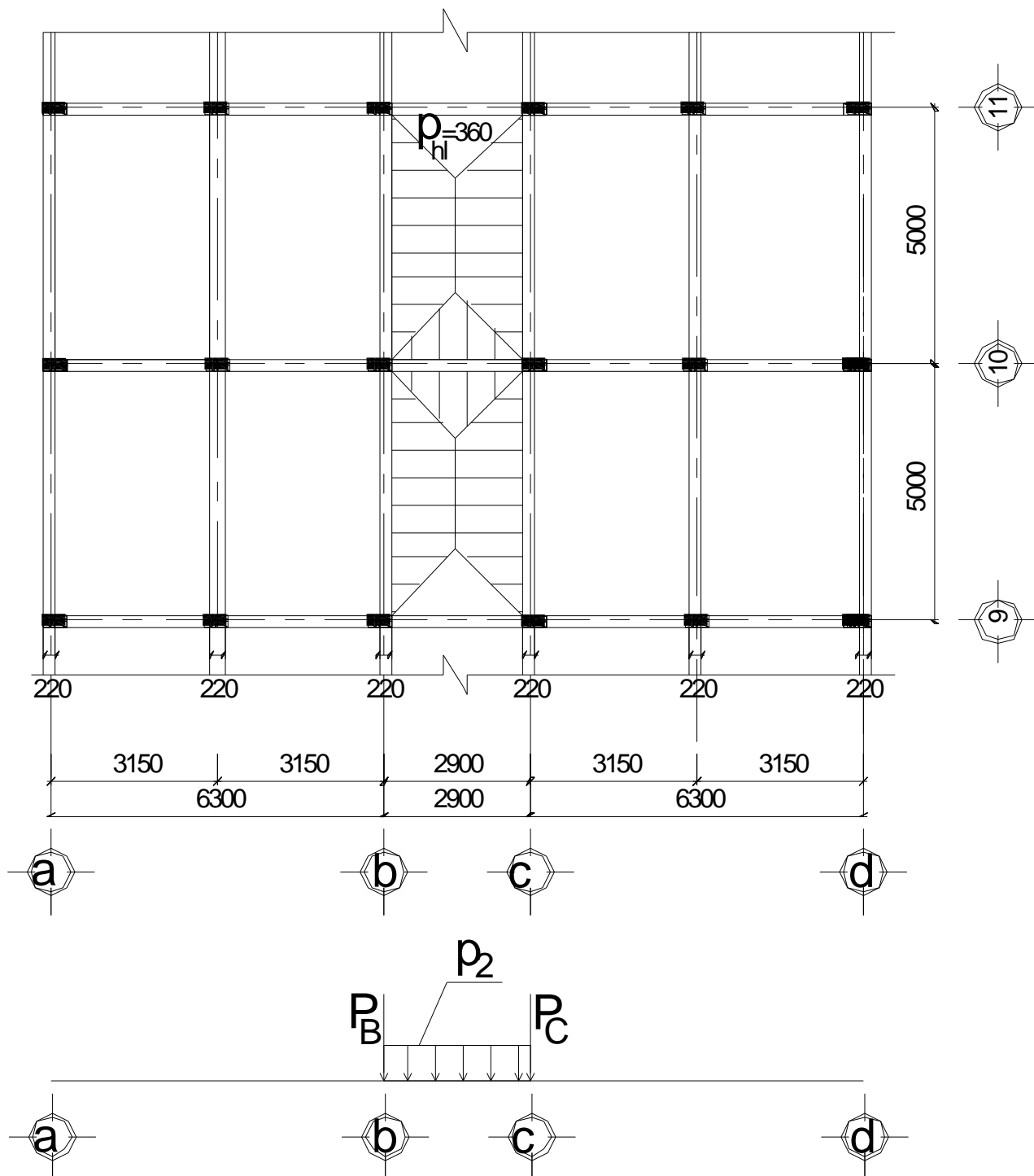
SƠ ĐỒ HOẠT TẢI TÁC DỤNG TRƯỜNG HỢP 2
