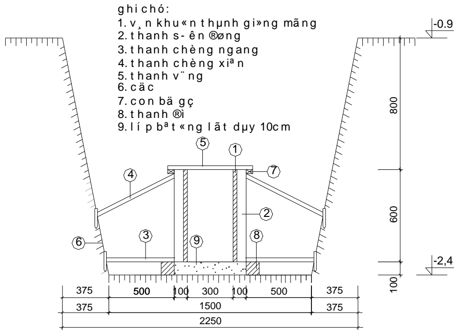
c Ếu t 1 o v, n khu «n gi»ng mǎng gm2
