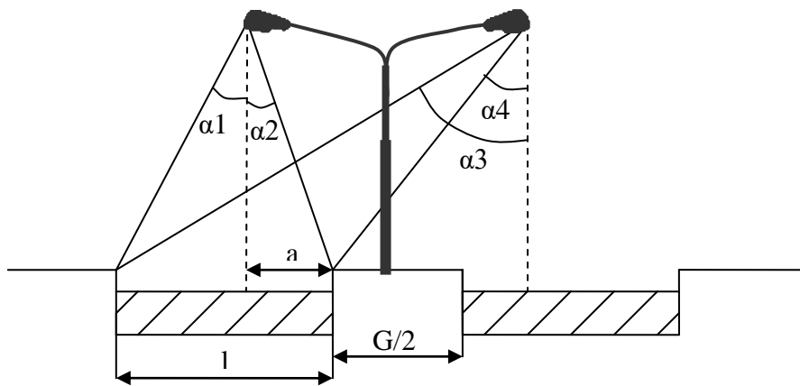
Hình 2.9 : Bố trí đèn trên giải phân
