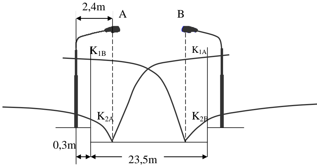
Hình 3.2: Bố trí đèn hai bên đối diện
