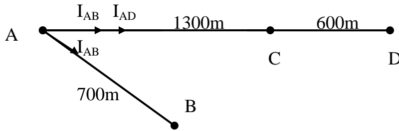
Hình 3.3: Sơ đồ mạng chiếu sáng
