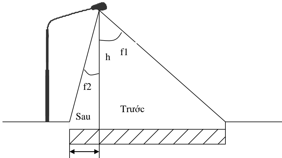
Hình 2.6: Độ rọi bề mặt chiếu sáng
