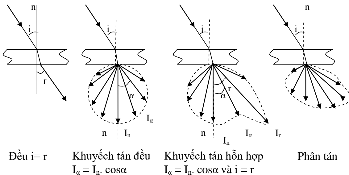
Hình 1.6: Hiện tượng truyền xạ
