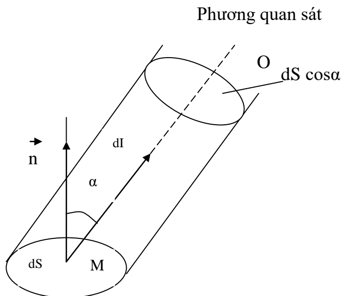
Hình 1.2: Định nghĩa độ chói
