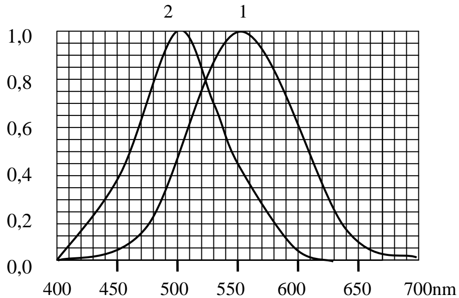
Hình 1.1: Đường cong hiệu quả ánh sáng của mắt người
