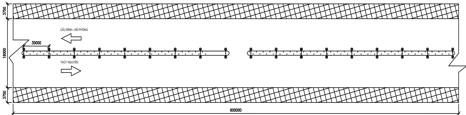
MẶT BẰNG BỐ TRÍ ĐIỆN CHIẾU SÁNG (03)
