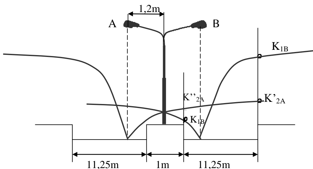
Hình 3.1: Bố trí đèn trên giải phân cách
