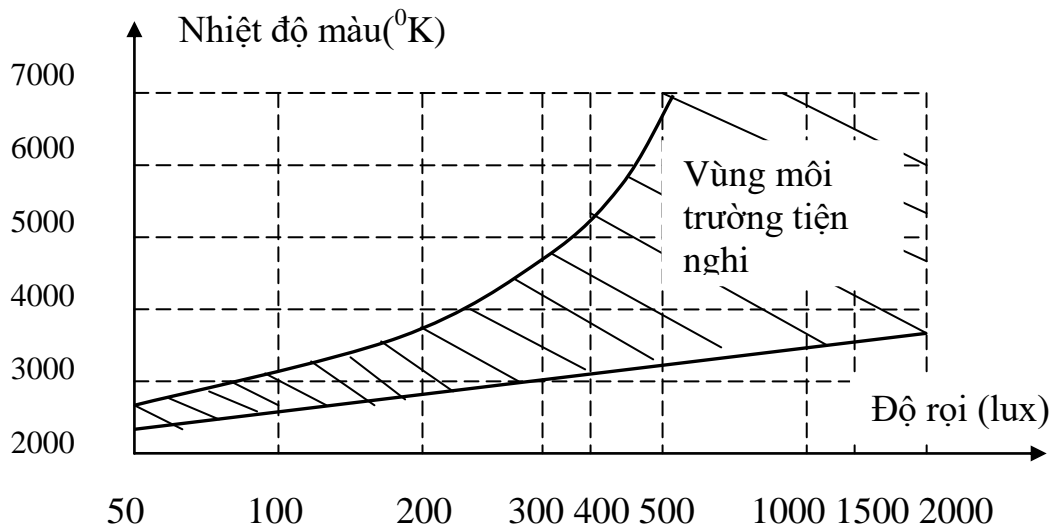
Hình 1.3: Biểu đồ kruithof
