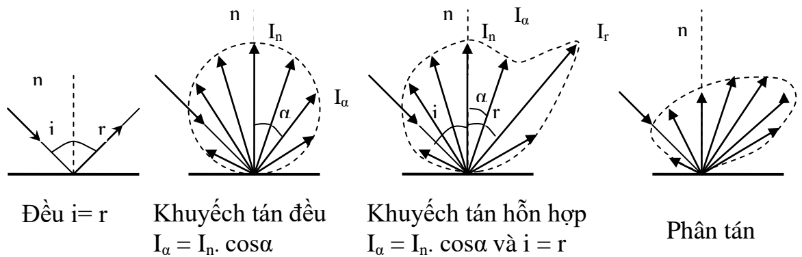
Hình 1.4: Các hiện tượng phản xạ
