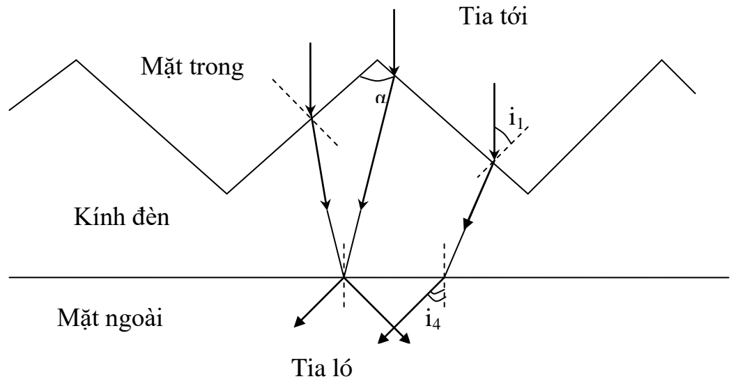
Hình 1.5: Hiện tượng khúc xạ
