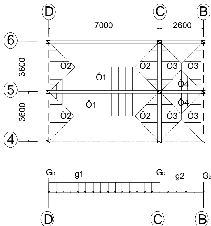
Bảng 2- 3 :Phân tải khung K5(Tĩnh tải từ tầng 2 đến tầng 6)
