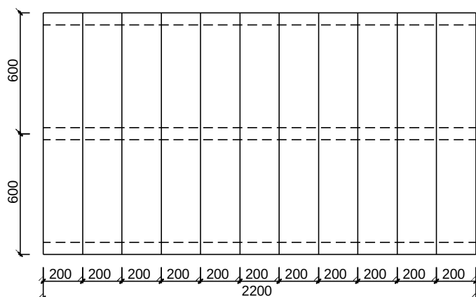
MẶT ĐÚNG KHÔNG GIẰNG
