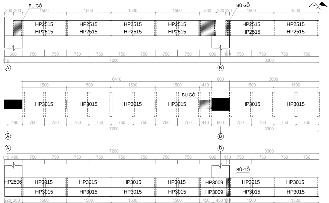
TỔ HỢP VÁN KHUÔN DẦM D1 TẦNG 1,2,3,4
