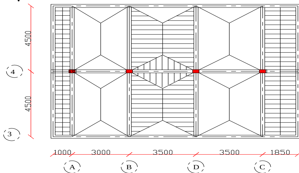
Sơ đồ phân hoạt tải tầng 1,3,mái
