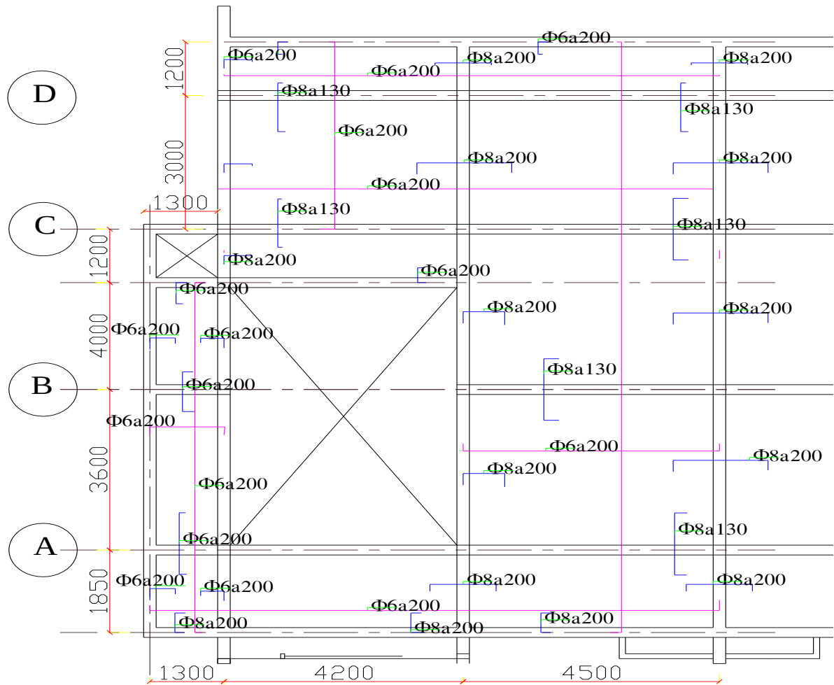
Bố Trí Thép Sàn
