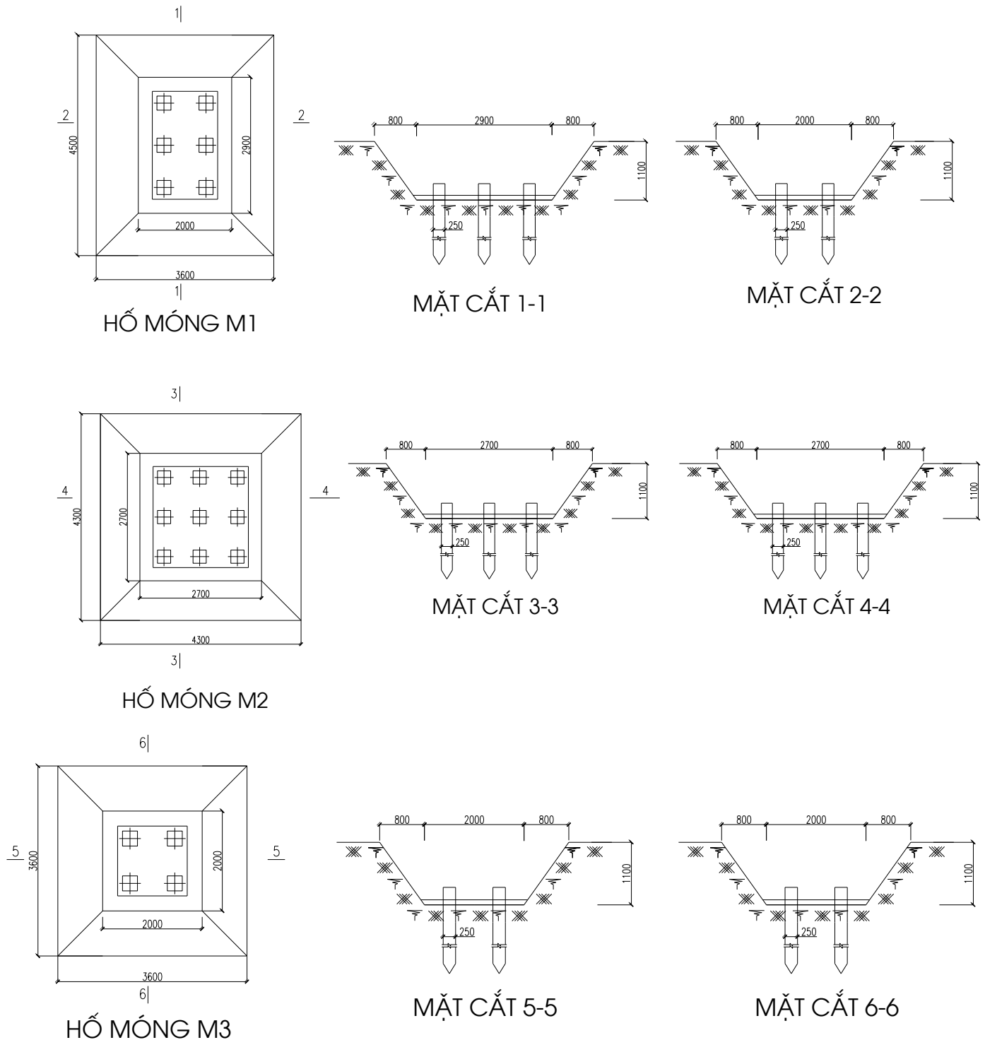
Hình 5-2. Kích thước hình học hố móng
