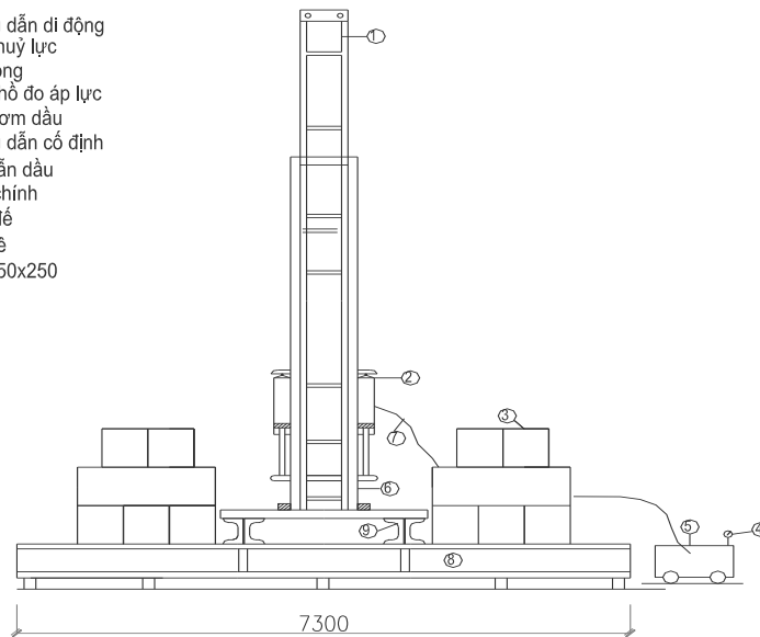
MẶT ĐỨNG MÁY ÉP CỌC
