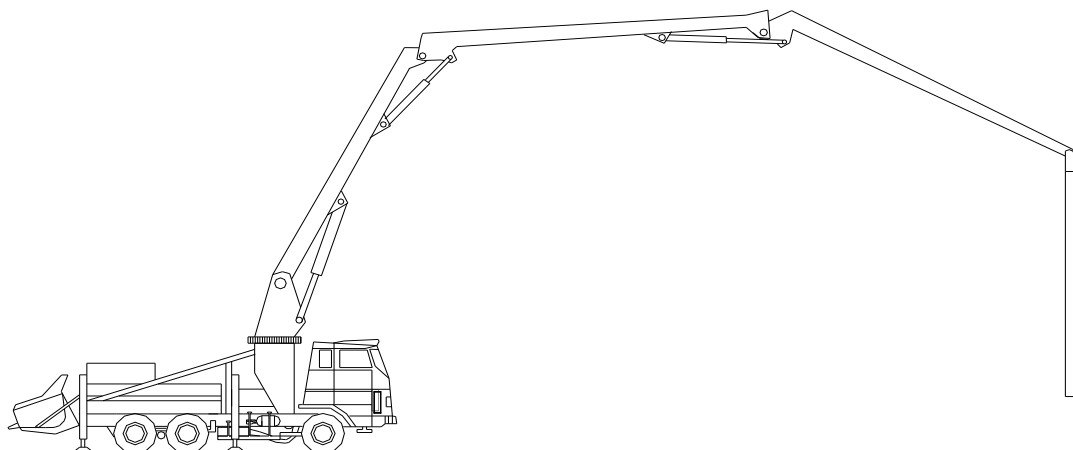
Hình 8-8 . Xe bơm bê tông Putzmeister
