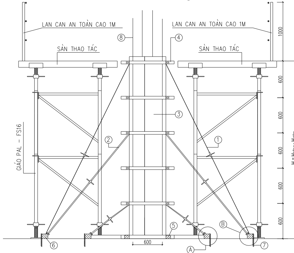
Hình 6-2. Ván khuôn cột giữa.
