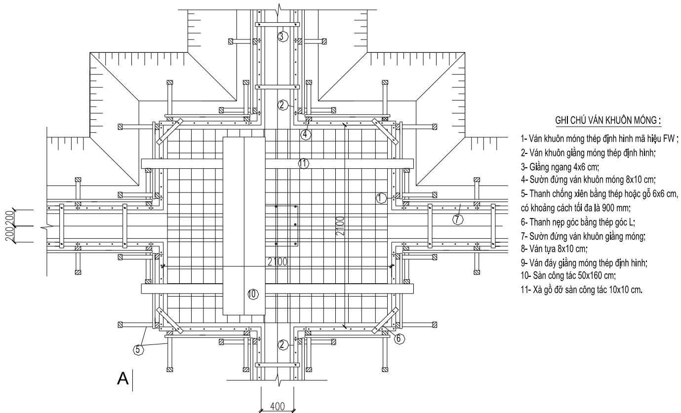
Hình 8-8 . Cấu tạo đài móng
