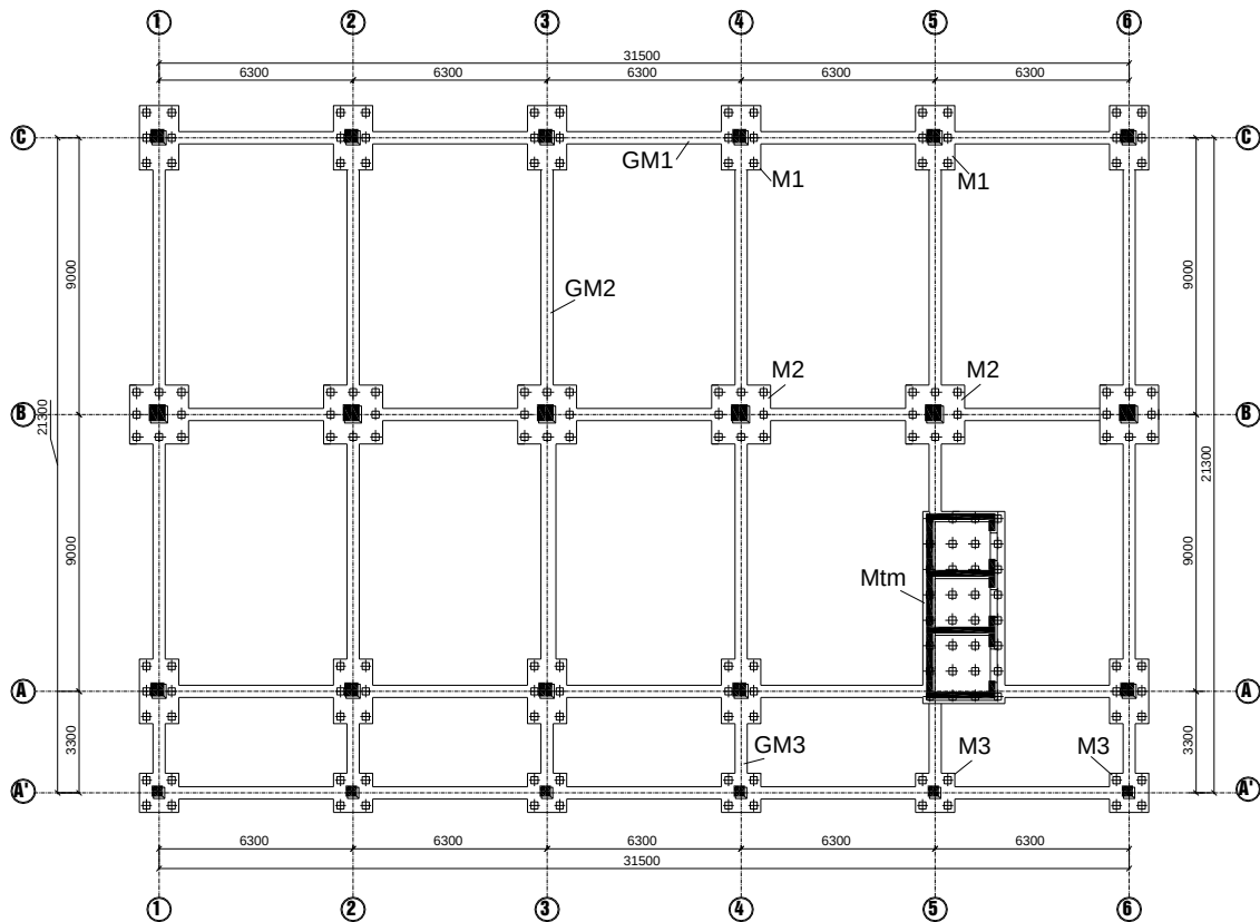
Mặt bằng móng
