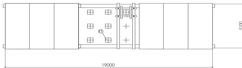
MẶT BẰNG MÁY ÉP CỌC
