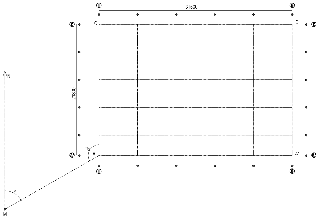
Hình 5-1. Sơ đồ định vị công trình
