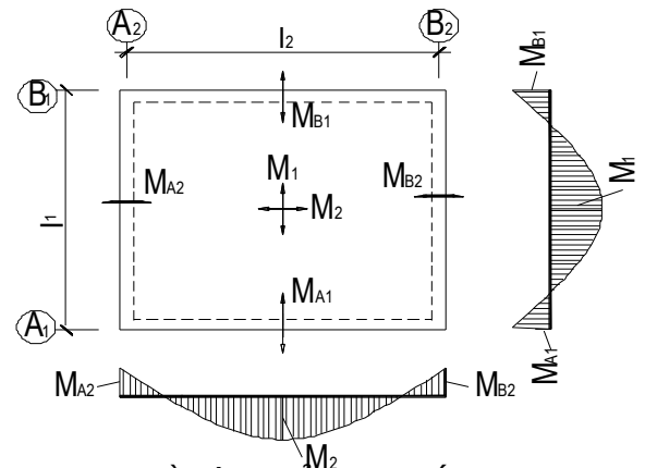
SƠ ĐỒ TÍNH BẢN KÊ BỐN CẠNH
