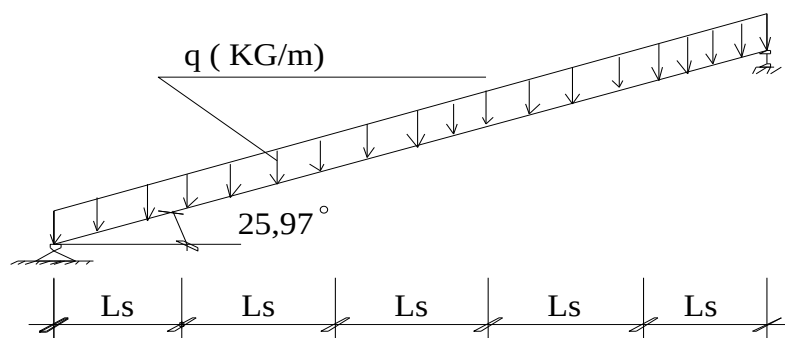
Hình 9.14: Sơ đồ tính toán cột chống cầu thang
