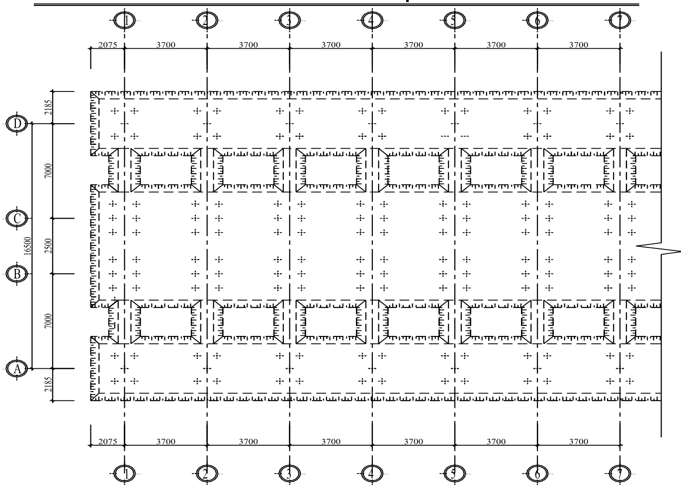
MẶT BẰNG ĐÀO MÓNG
