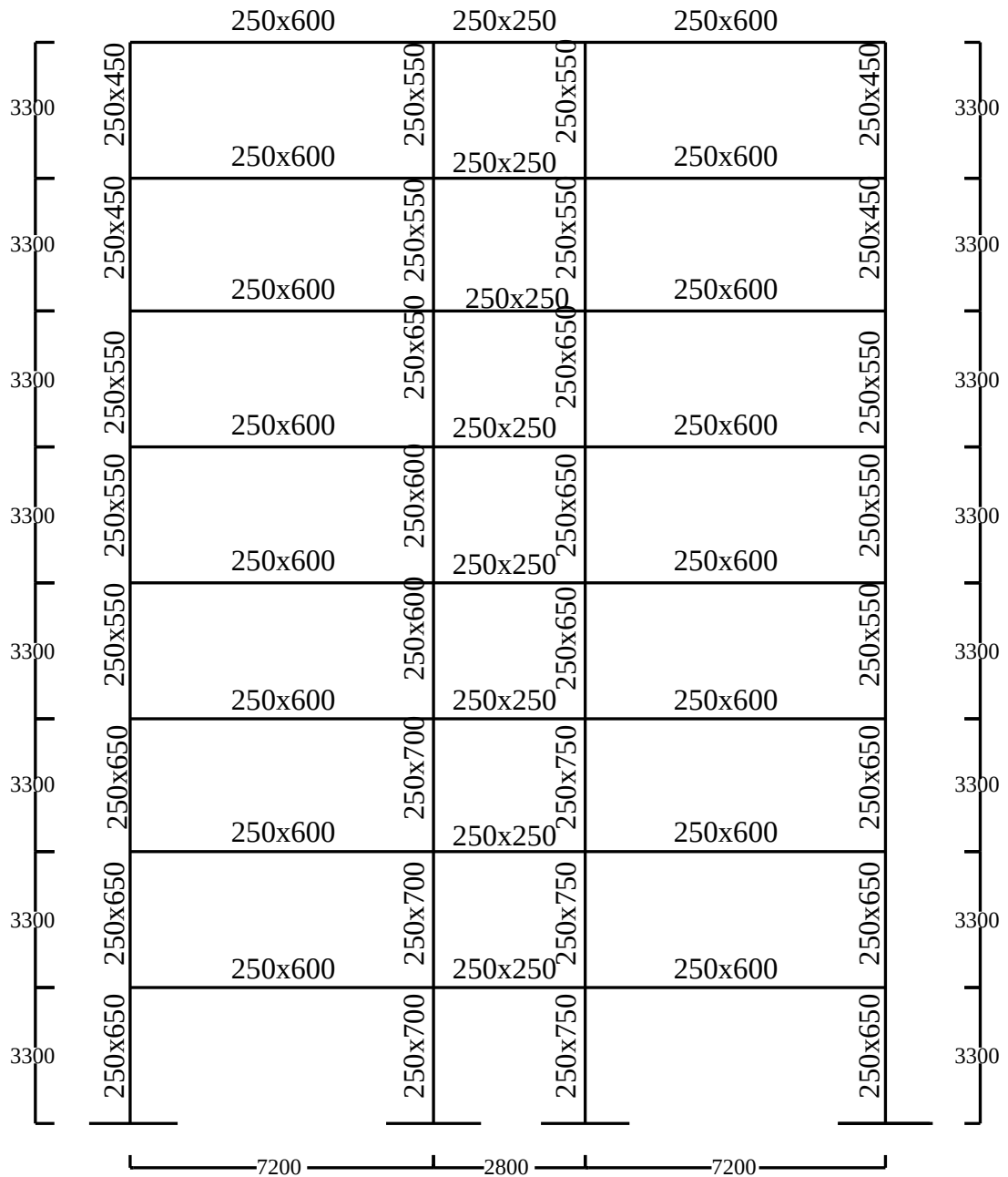
Hõnh 2: sơ đồ hõnh học khung K2
