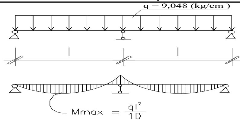
Hình 6: Sơ đồ tính toán kiểm tra thanh sườn đứng
