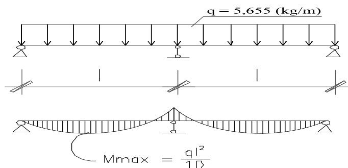
Hình 5: Sơ đồ tính toán kiểm tra thanh sườn
