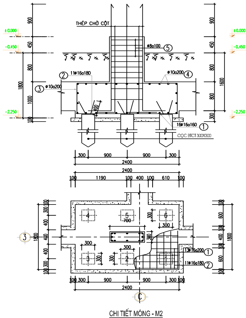
Hình 7.10: Bố trí cốt thép móng M2
