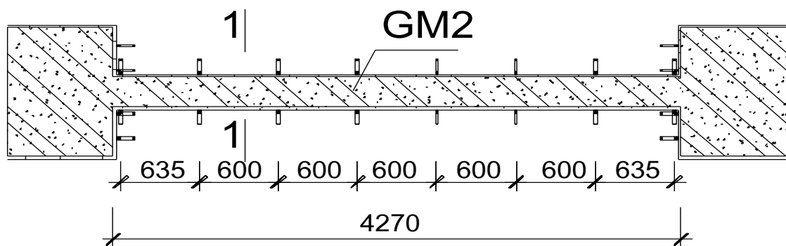
MẶT BẰNG VÁN KHUÔN GM2
