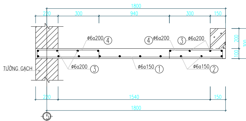
Hình 6.4. Mặt cắt bản thang
