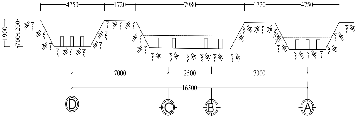
MẶT ĐỪNG HỐ ĐÀO
