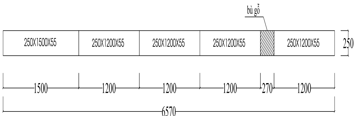
Hình 9.3: Tổ hợp ván khuôn đáy dầm
