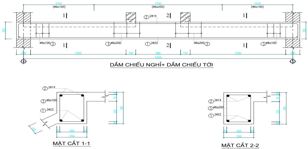
Hình 6.9. Bố trí thép dầm chiếu nghỉ và dầm chiếu tới
