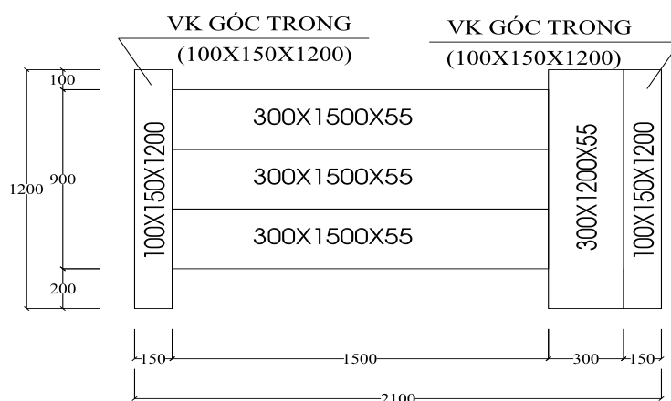
Hình 9: Tổ hợp ván khuôn giằng móng trục 1-2
