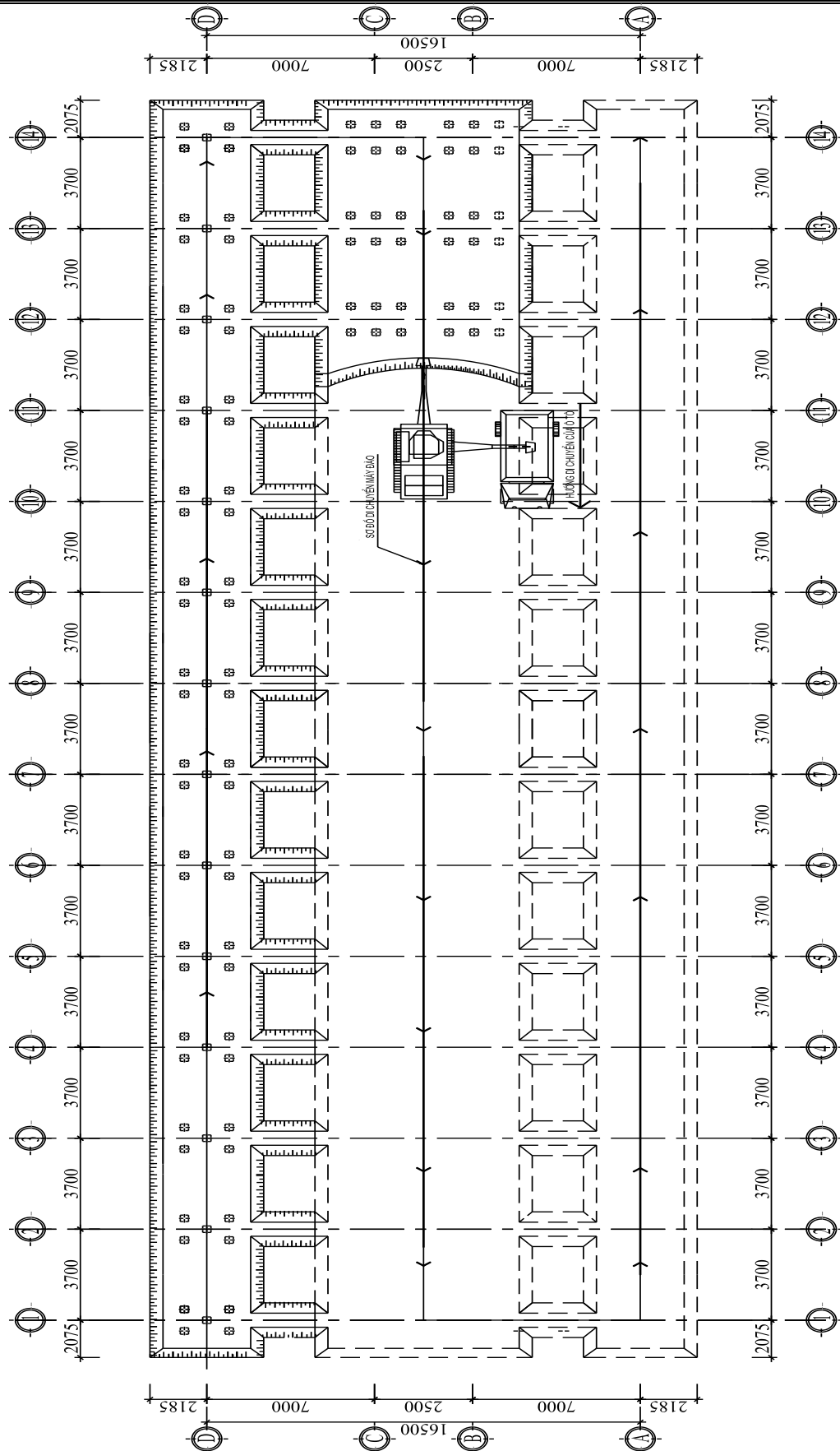
MẶT BẰNG THI CÔNG ĐÀO HỒ MÓNG
