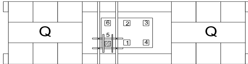
SƠ ĐỒ ẦP ĐÀI CỌC M2
