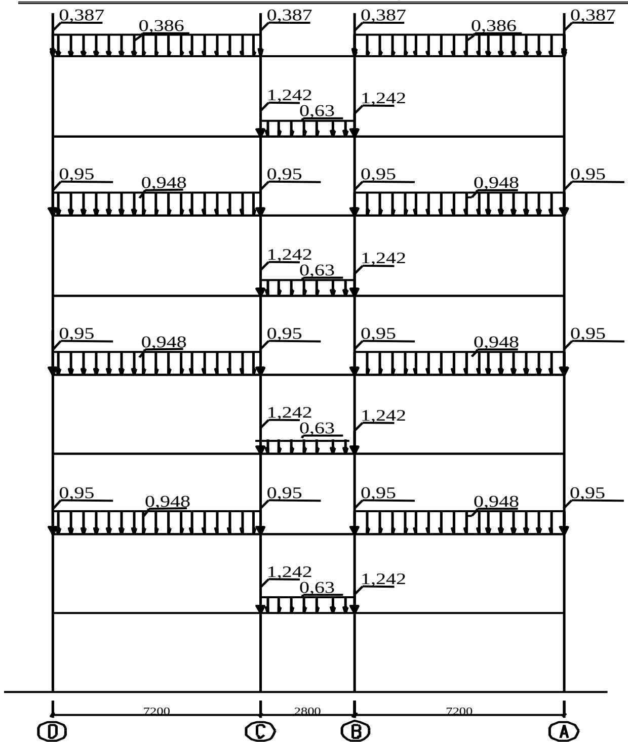
Hình 2.14: Hoạt tải 1 Hình 2.15: Hoạt tải 2
