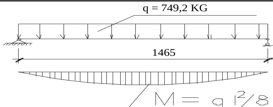
Hình 6.7.2. Sơ đồ tính bản chiều nghỉ
