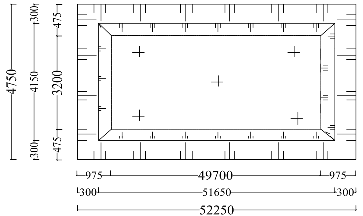
MẶT BẰNG HỐ ĐÀO
