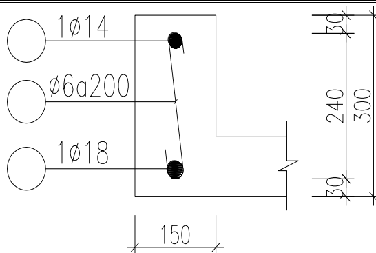
Hình 6.6. Mặt cắt cốt thang
