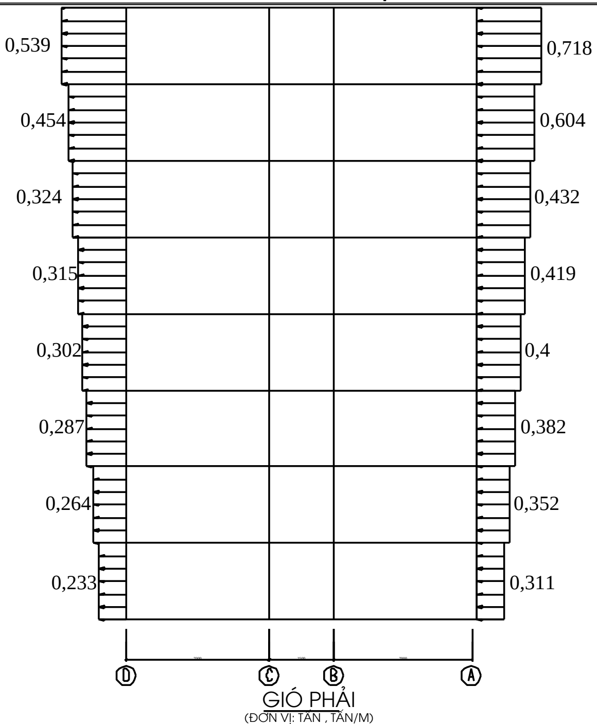
Hình 2.17: Gió phải
