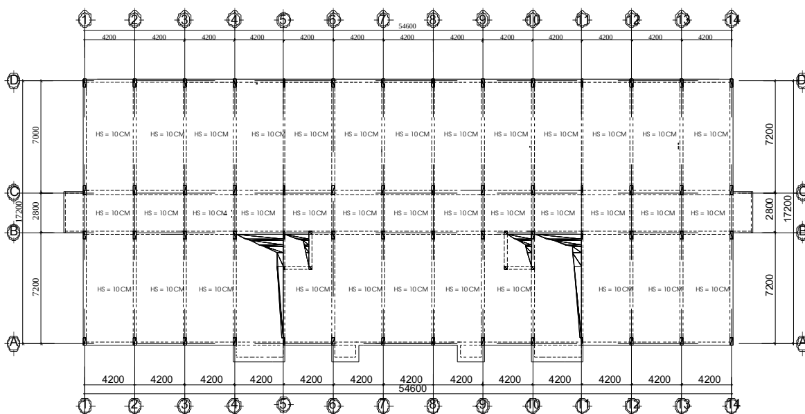
Hình 2.1: Mặt bằng kết cấu tầng điển hình
