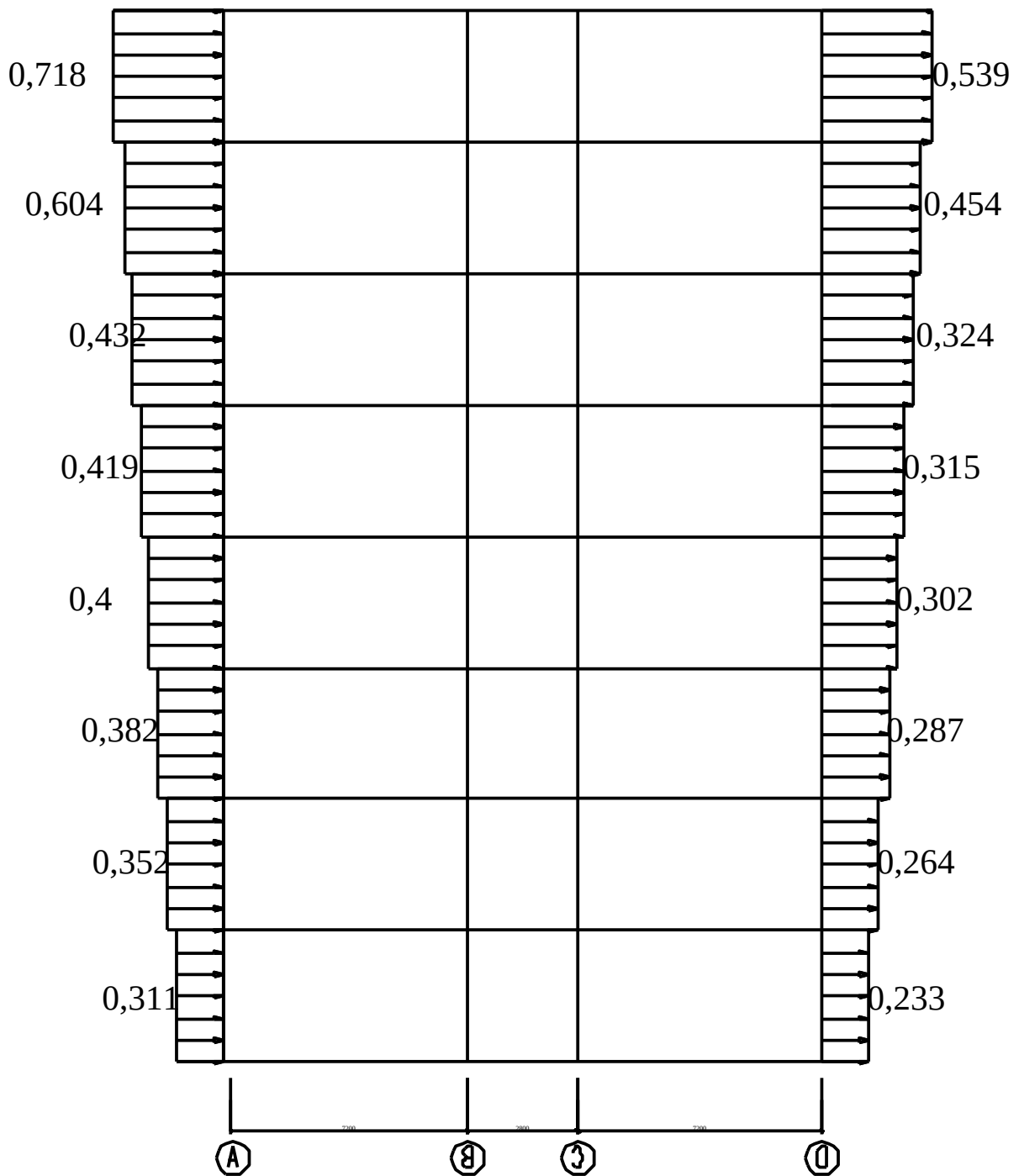
Hình 2.16: Gió trái
