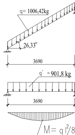
Hình 6.5. Sơ đồ tính cốt thang
