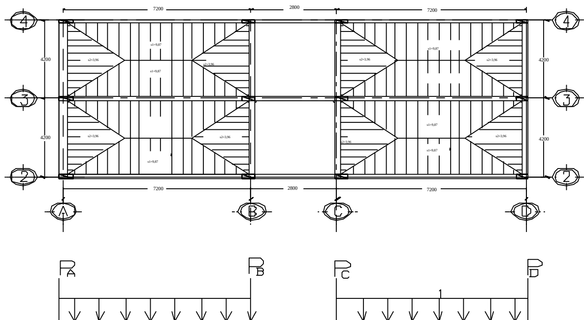
Hình 2.10: Trường hợp hoạt tải 2(tầng mái)
