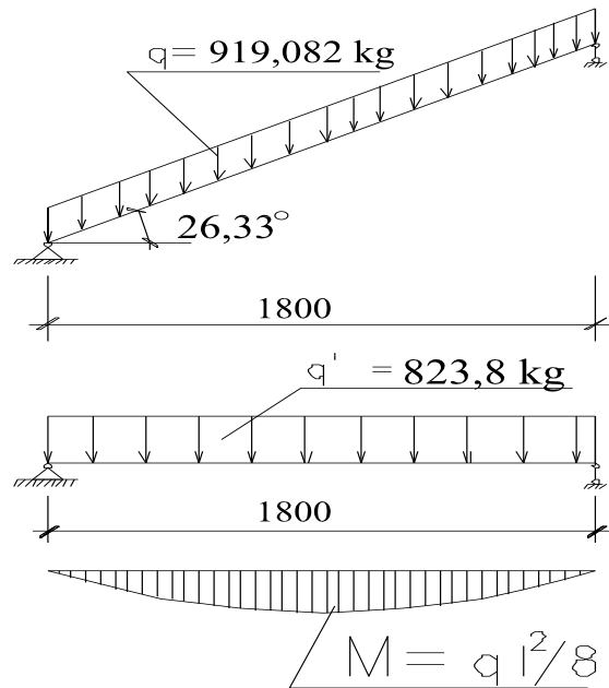
Hình 6.3. Sơ đồ tính bản thang
