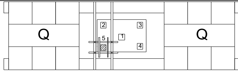
SƠ ĐỒ ẦP ĐÀI CỌC M1
