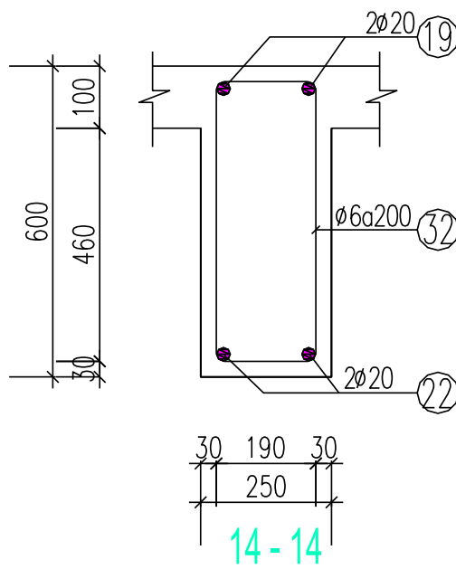
Hình 4.1. Mặt cắt dầm 36
