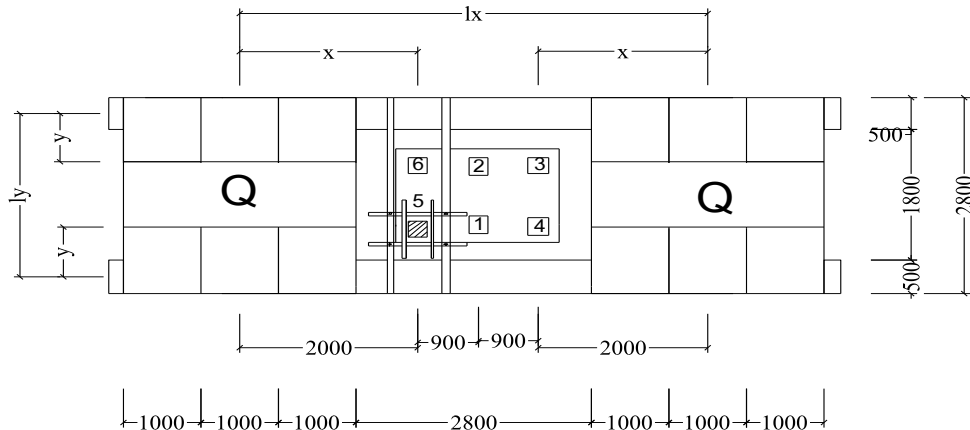
Hình 8.3: Mặt bằng bố trí đối trọng ép cọc
