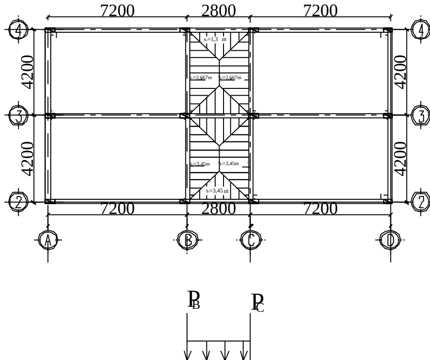
Hình 2.9: Trường hợp hoạt tải 2 (tầng 3,5,7)
