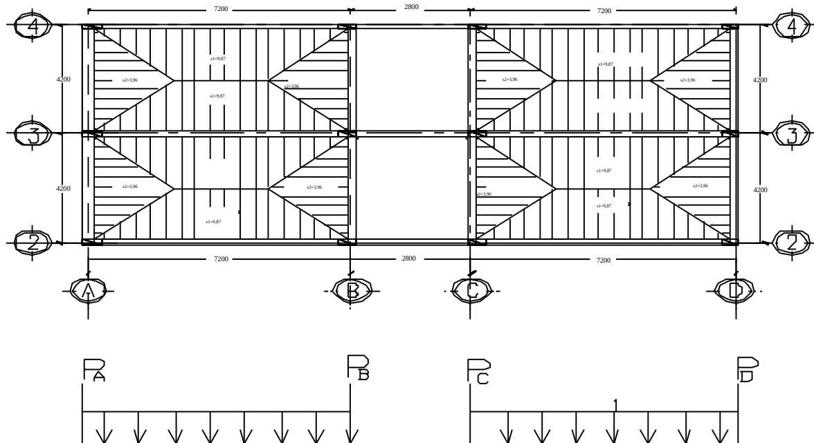
Hình 2.10: Trường hợp hoạt tải 1(tầng 3,5,7)
