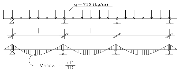
Hình 9.10: Sơ đồ tính toán kiểm tra ván khuôn
