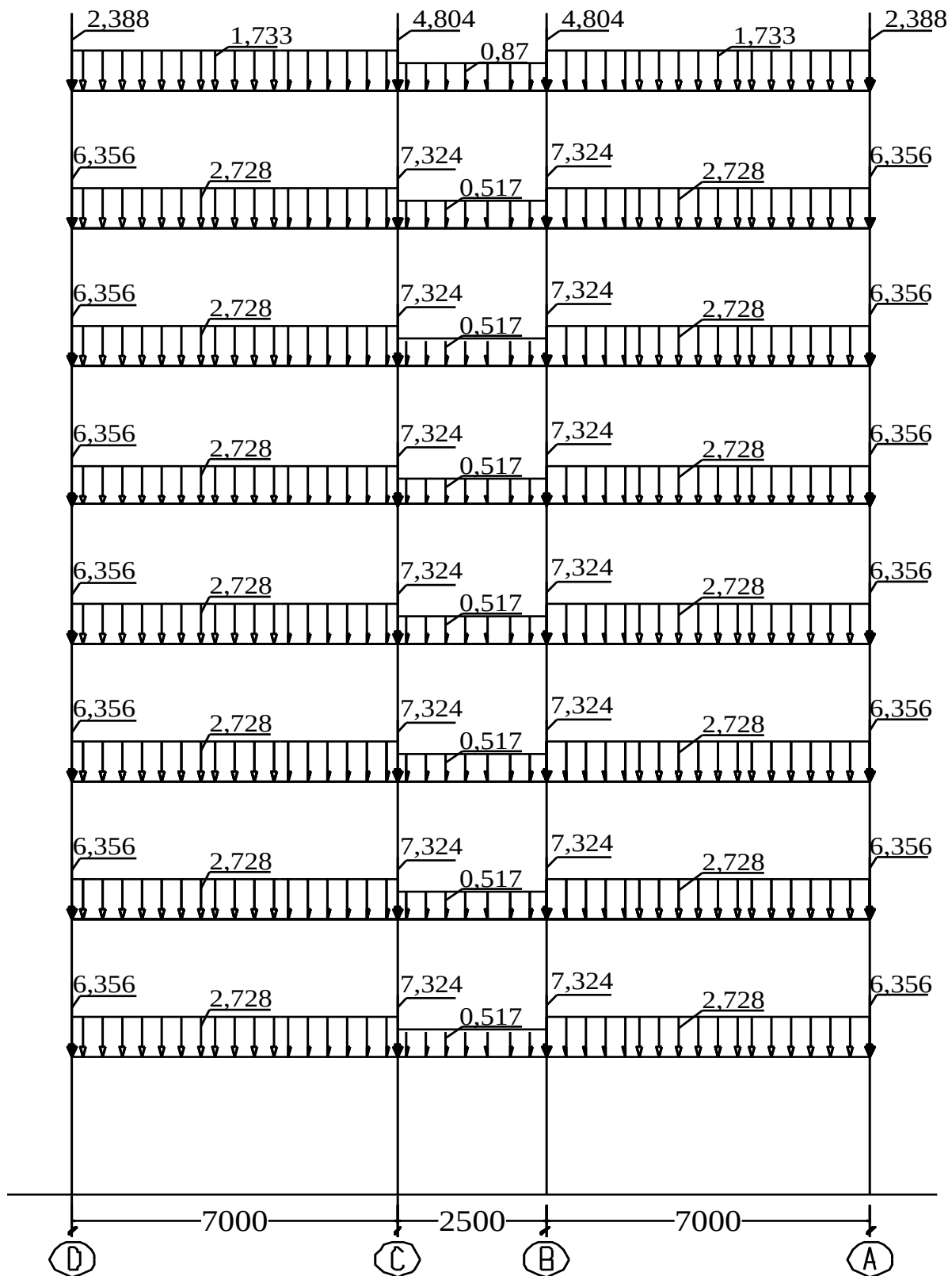
Hình 2.13: Tĩnh tải
