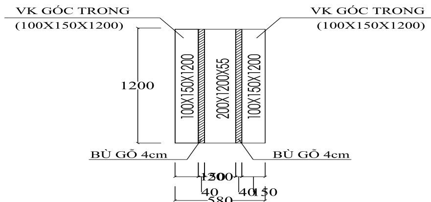
Hình 8: Tổ hợp ván khuôn giằng móng trục B-C
