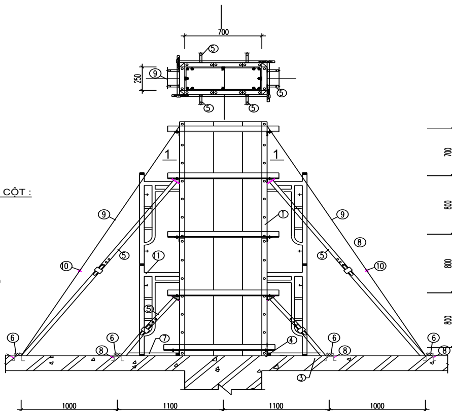
CHI TIẾT VÁN KHUÔN CỘT GIỮA
