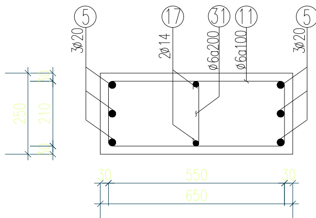
Hình 5.6. Mặt cắt cột trục C (tầng 4,5,6)
