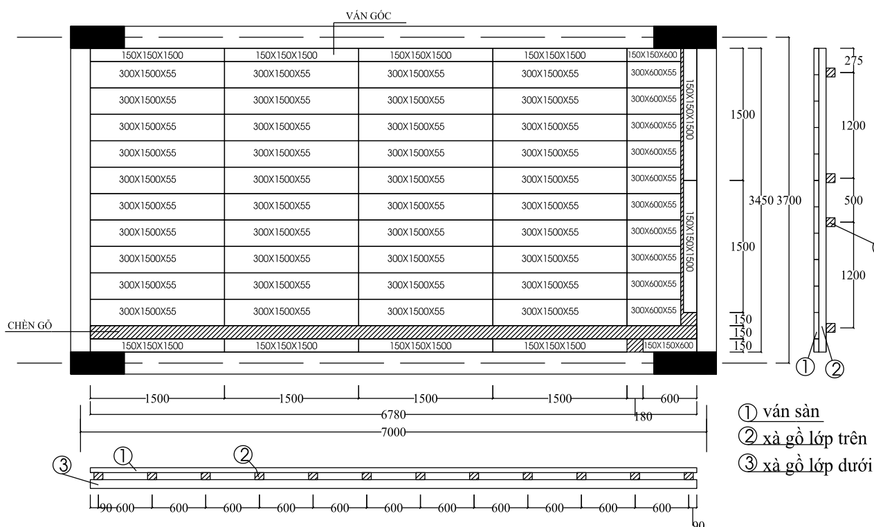
Hình 9.2: Tổ hợp ván khuôn cho ô sàn điển hình
