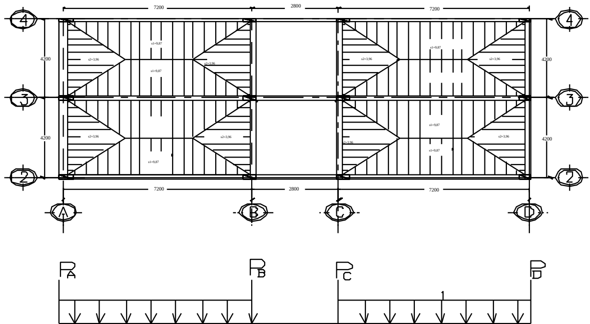
Hình 2.7: Trường hợp hoạt tải 1(tầng 2,4,6,8)
