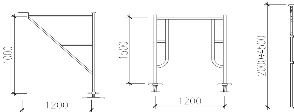
Hình 9.1: Khung giáo và cây chống
