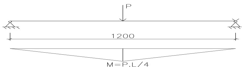
Hình 9.5: Sơ đồ tính xà ngang đỡ đáy dầm
