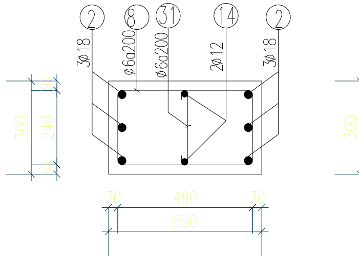
Hình 5.8. Mặt cắt cột trục C (tầng 7,8)
