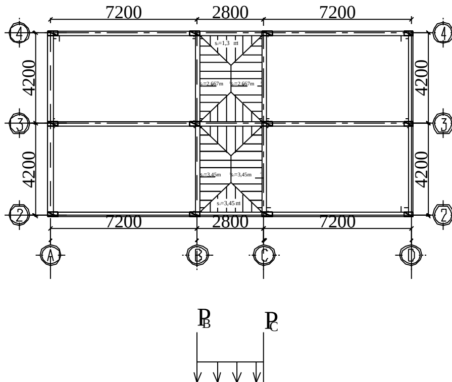
Hình 2.8: Trường hợp hoạt tải 2(tầng 2,4,6,8)
