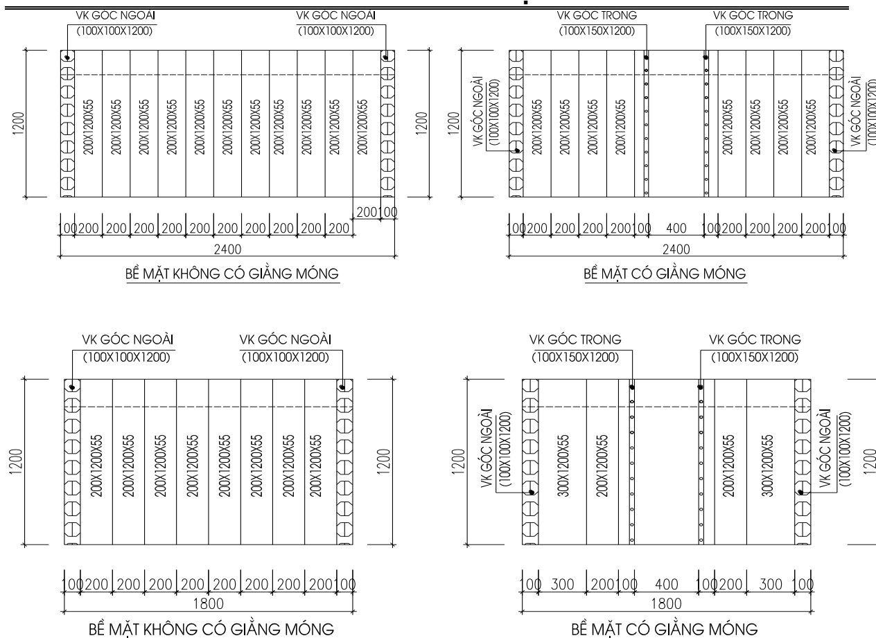
Hình 3: Tổ hợp ván khuôn các cạnh của móng M2
