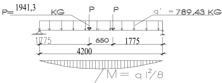
Hình 6.8. Sơ đồ tính dầm chiếu nghỉ
