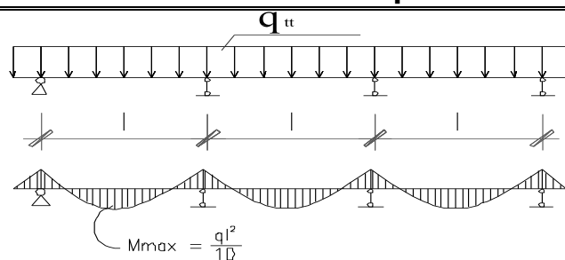
Hình 9.13: Sơ đồ tính xà gồ đỡ thang bộ
