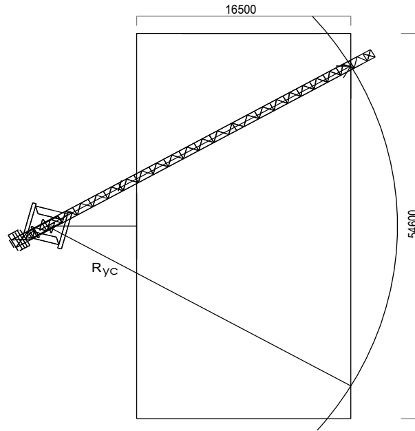
Hình 9.17,2: Xác định tầm với của cần trục tháp
