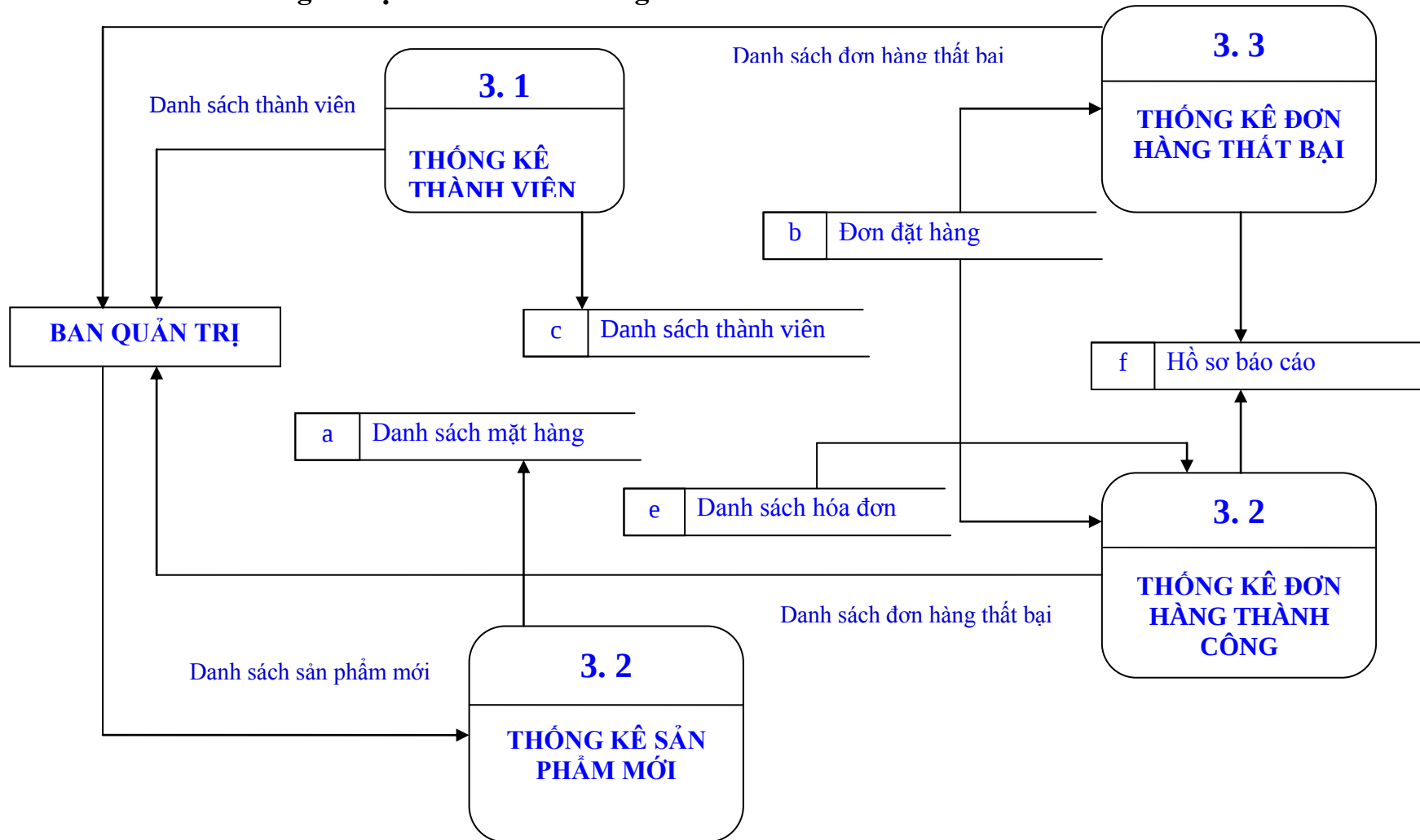
Hình 3.0. 7 Biểu đồ luồng dữ liệu
