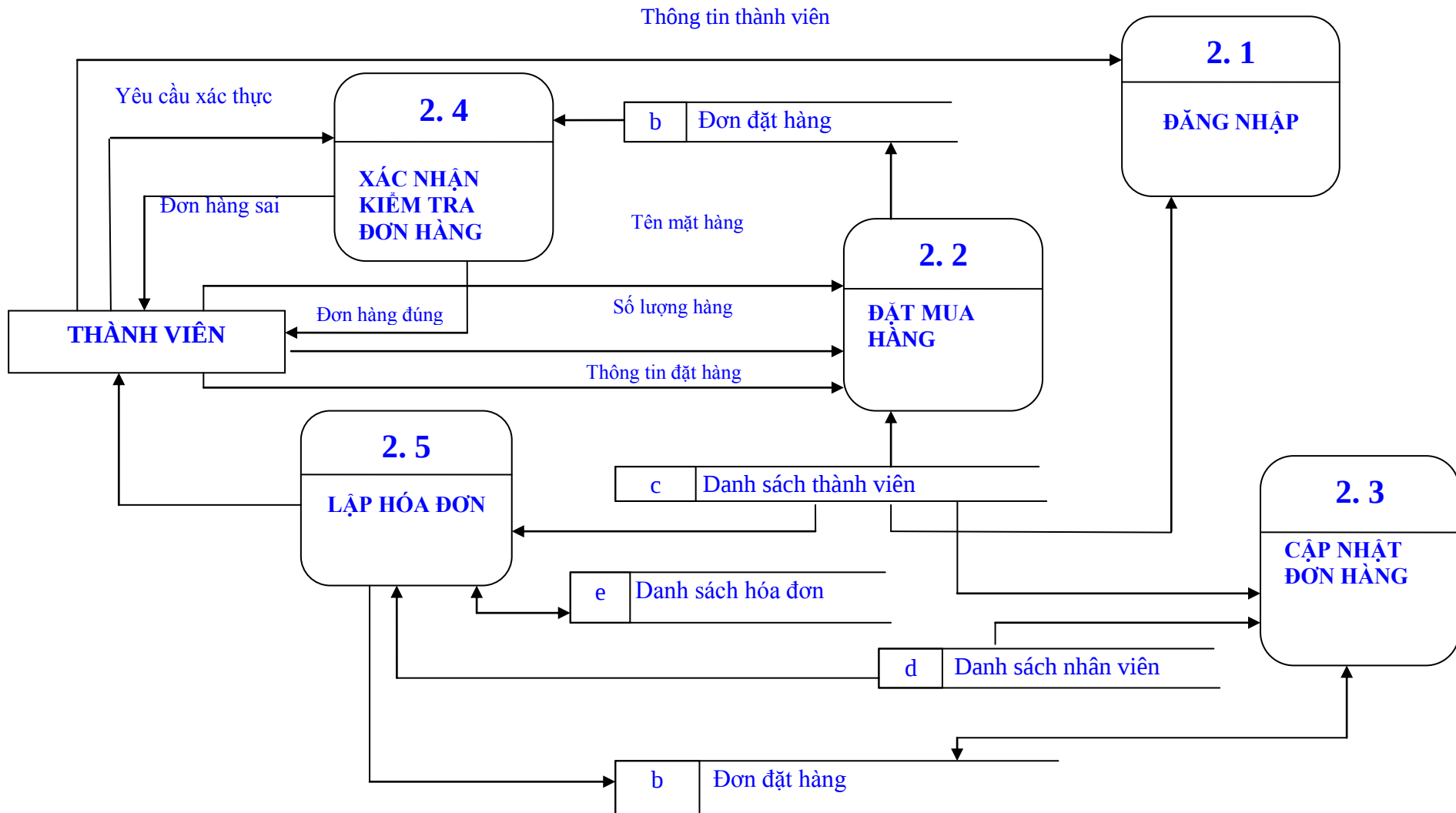
Hình 3. 0.6 Biểu đồ luồng dữ liệu
