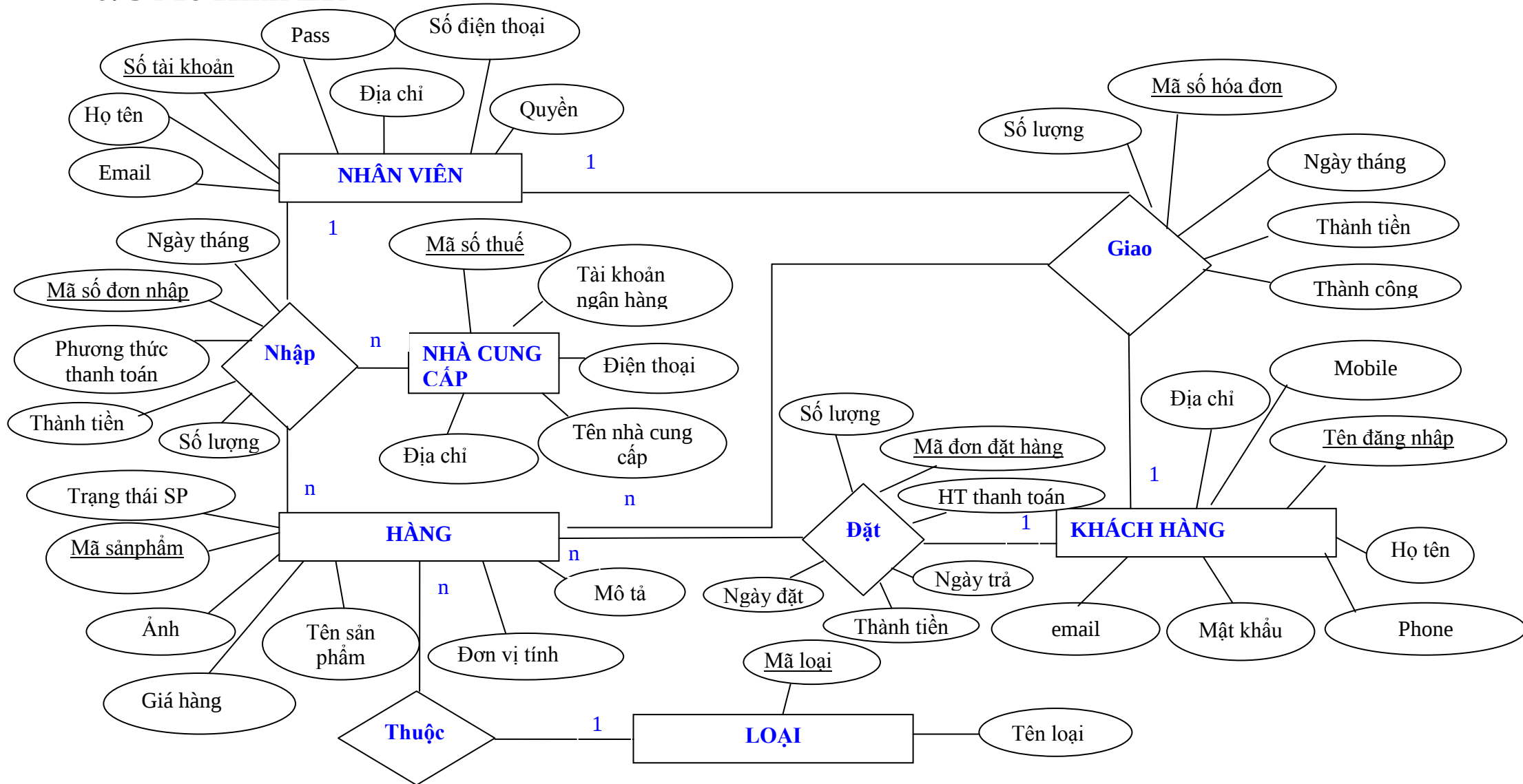
Hình 3. 0.8 Mô hình ER
