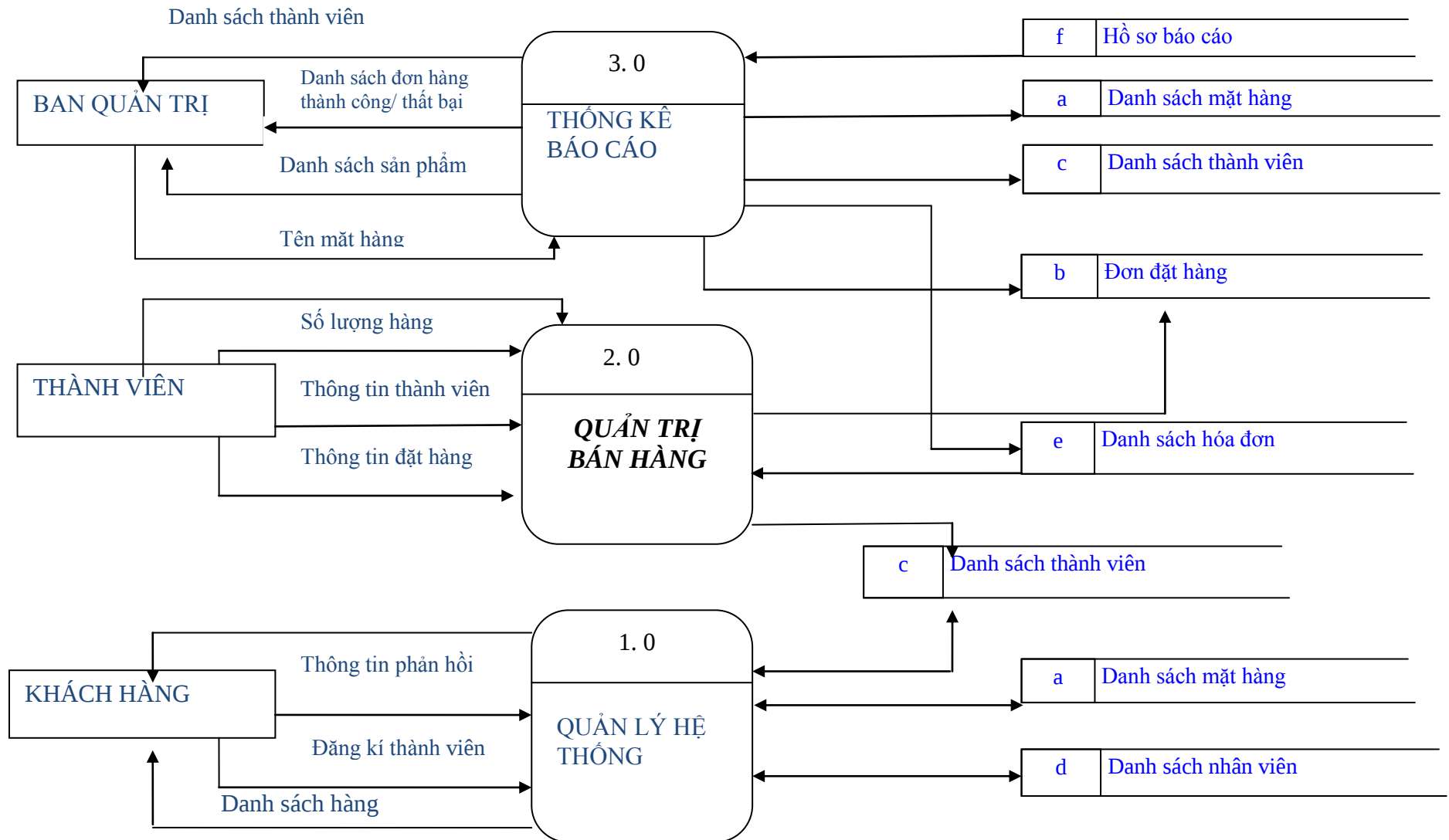
Hình 3. 0.4 biểu đồ luồng dữ liệu mức 0
