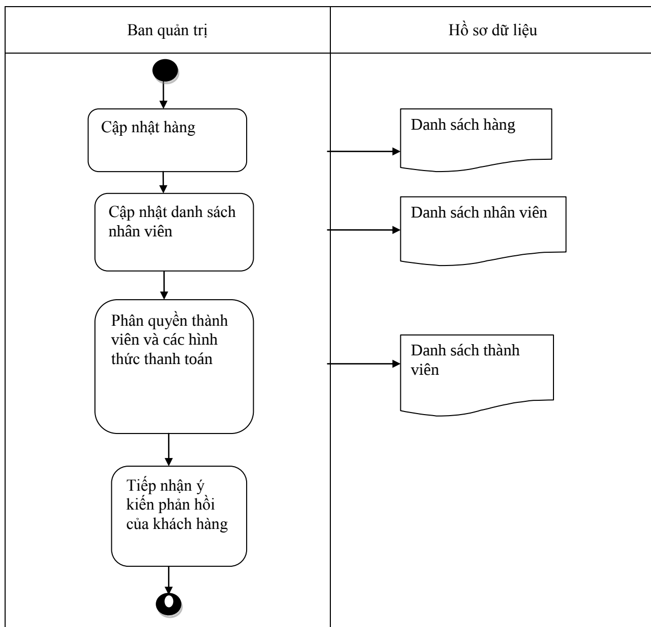
Bảng3. 0. 1 Sơ đồ tiến trình nghiệp vụ quản lý hệ thống
