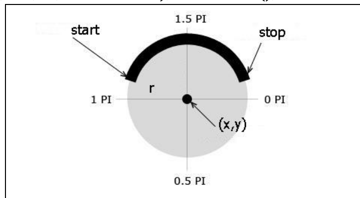
Hình 1. 0. 2 Mô tả phương thức arc()
