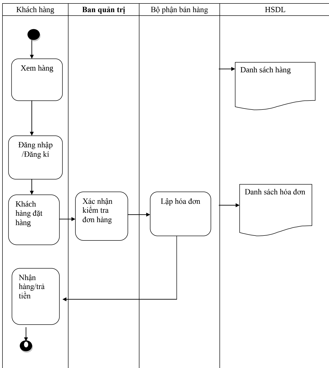
Bảng 3. 0. 2 Sơ đồ tiến trình nghiệp vụ quản trị bán hàng
