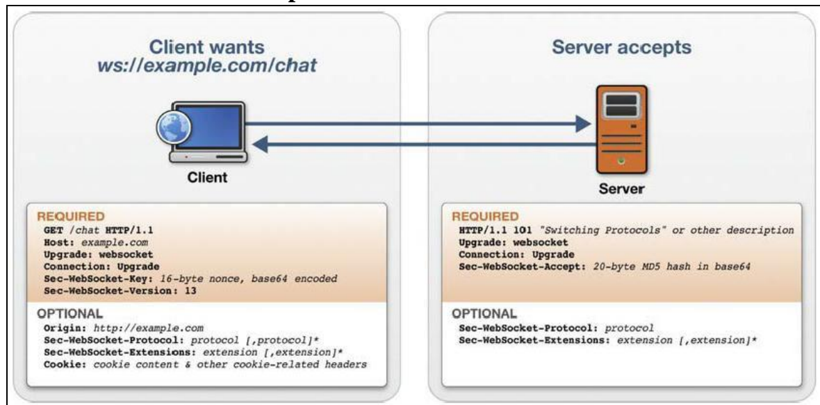
Hình 1. 0. 8Quá trình bắt tay Websocket
