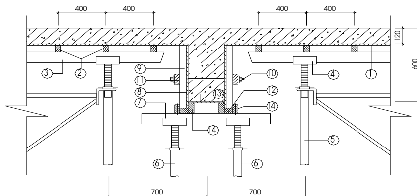
VÁN KHUÔN ĐẦM TL1/20.
