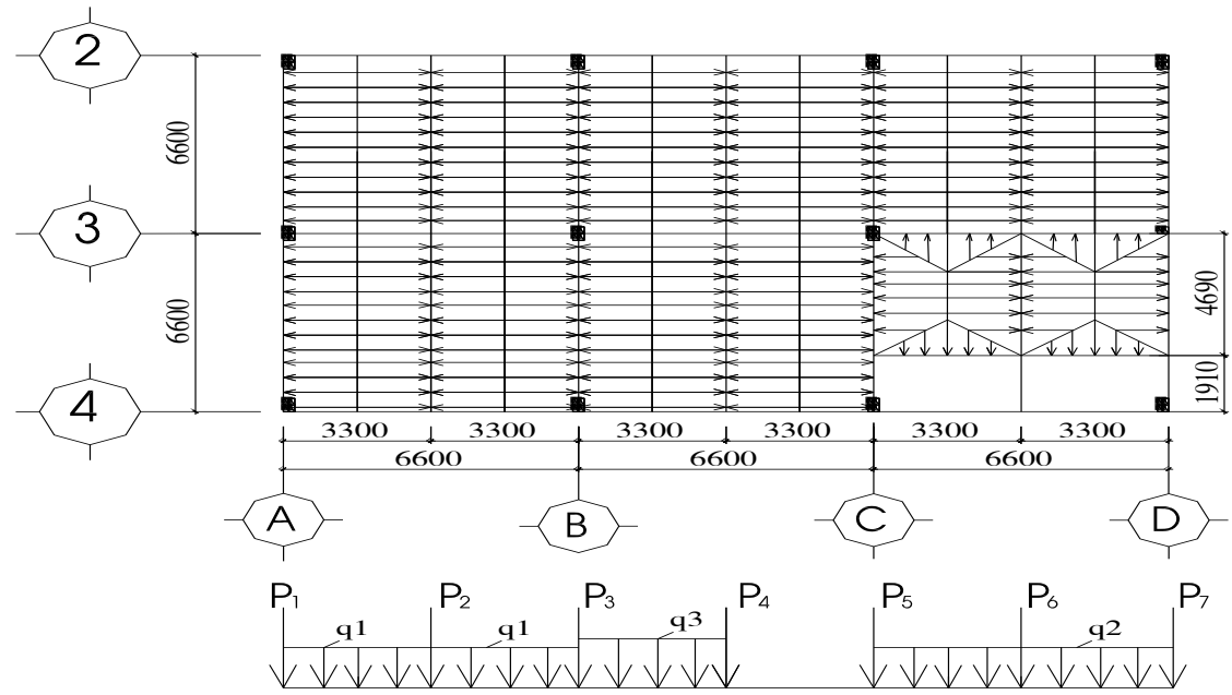
MẶT BẰNG PHÂN TẢI TẦNG 1
