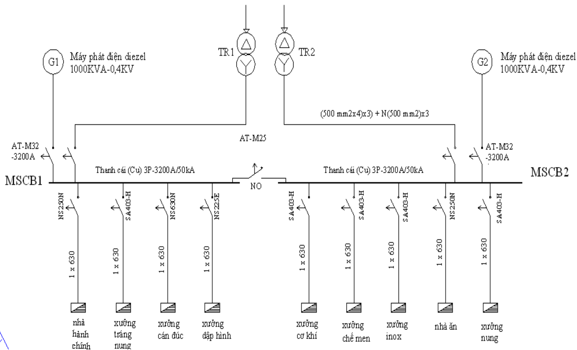
Hình 3.3. Sơ đồ hạ áp của công ty
