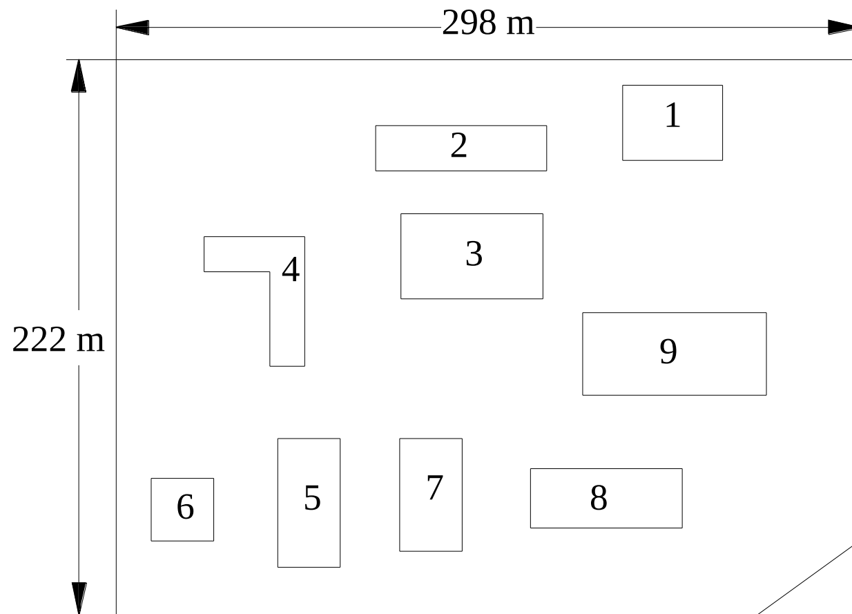
Hình 1.3. Sơ đồ mặt bằng toàn nhà máy.
