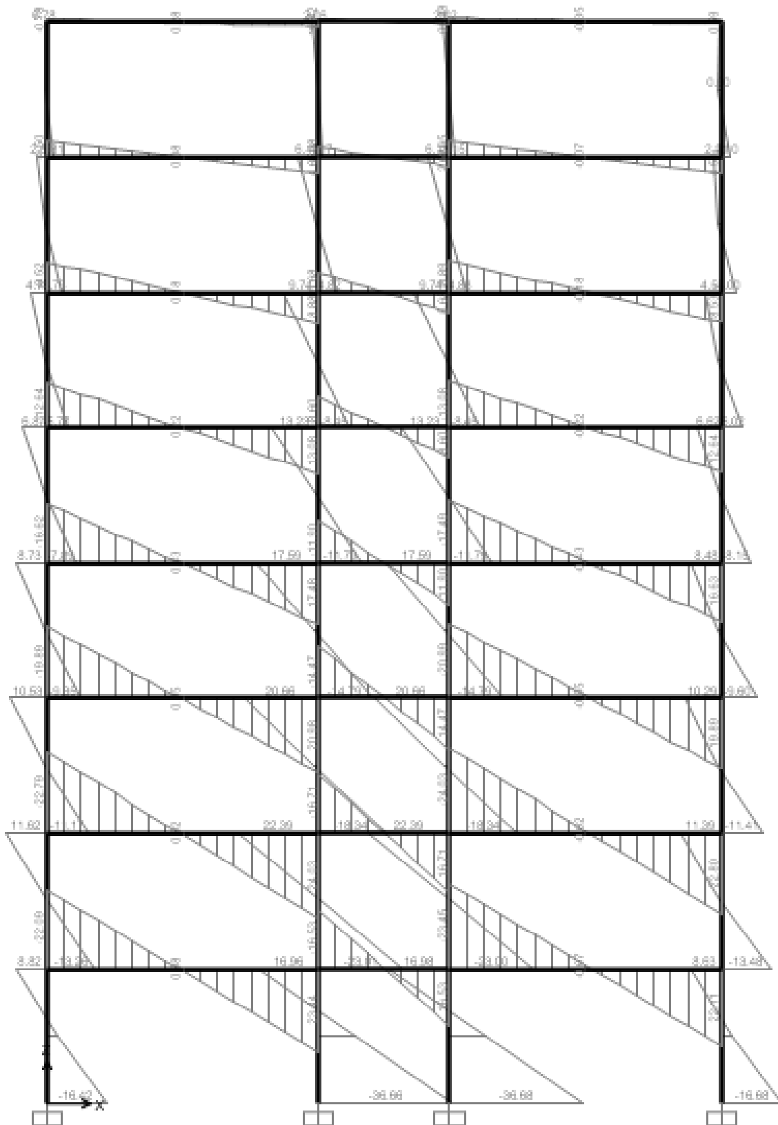
MOMEN DO GIÓ PHẢI GÂY RA
