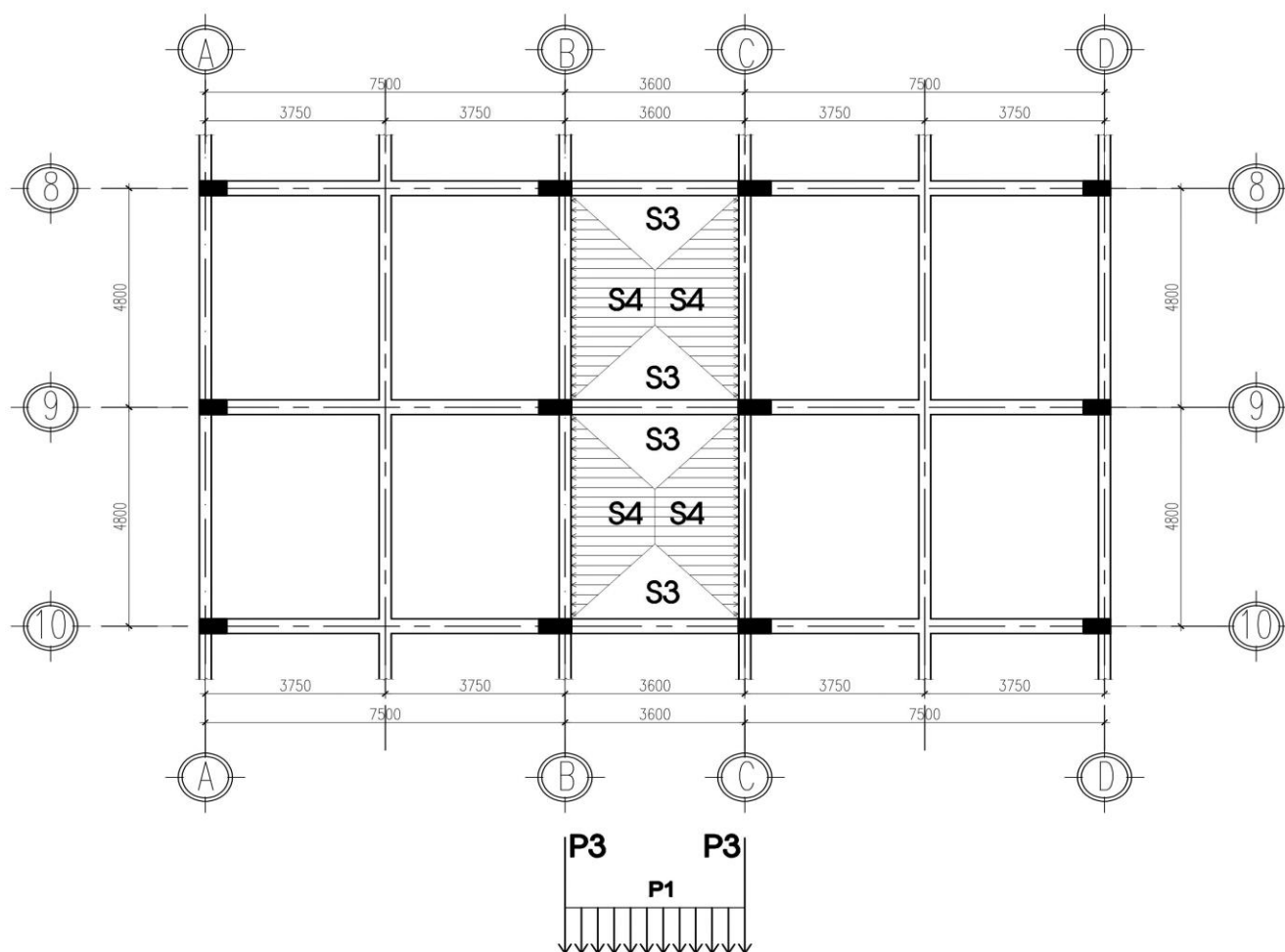
SƠ ĐỒ HOẠT TẢI TÁC DỤNG TH2
