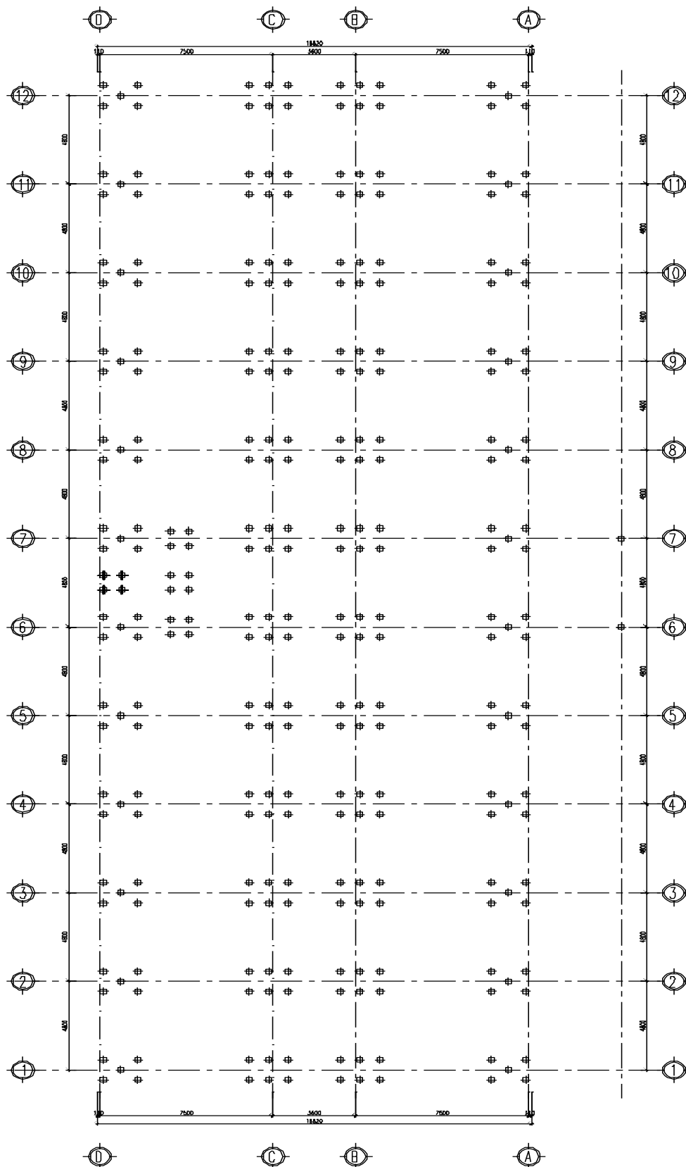
a. Mặt bằng lưới cọc
