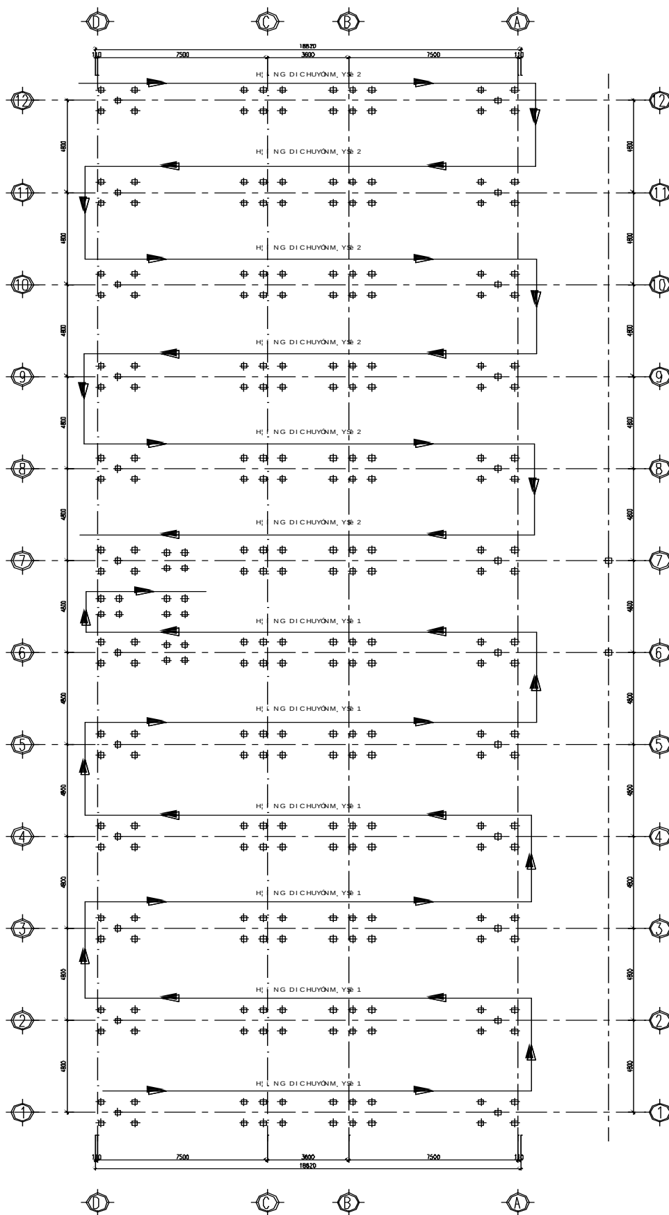
Hướng di chuyển máy ép cọc
