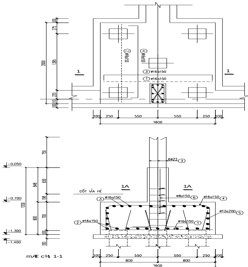
BỐ TRÍ CỐT THÉP MÓNG – TRỤC A (M2)
