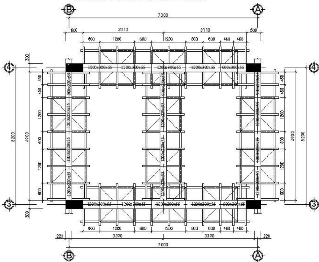
MẶT BẰNG BỐ TRÍ VÁN KHUÔN Ở SÀN ĐIỂN HÌNH
