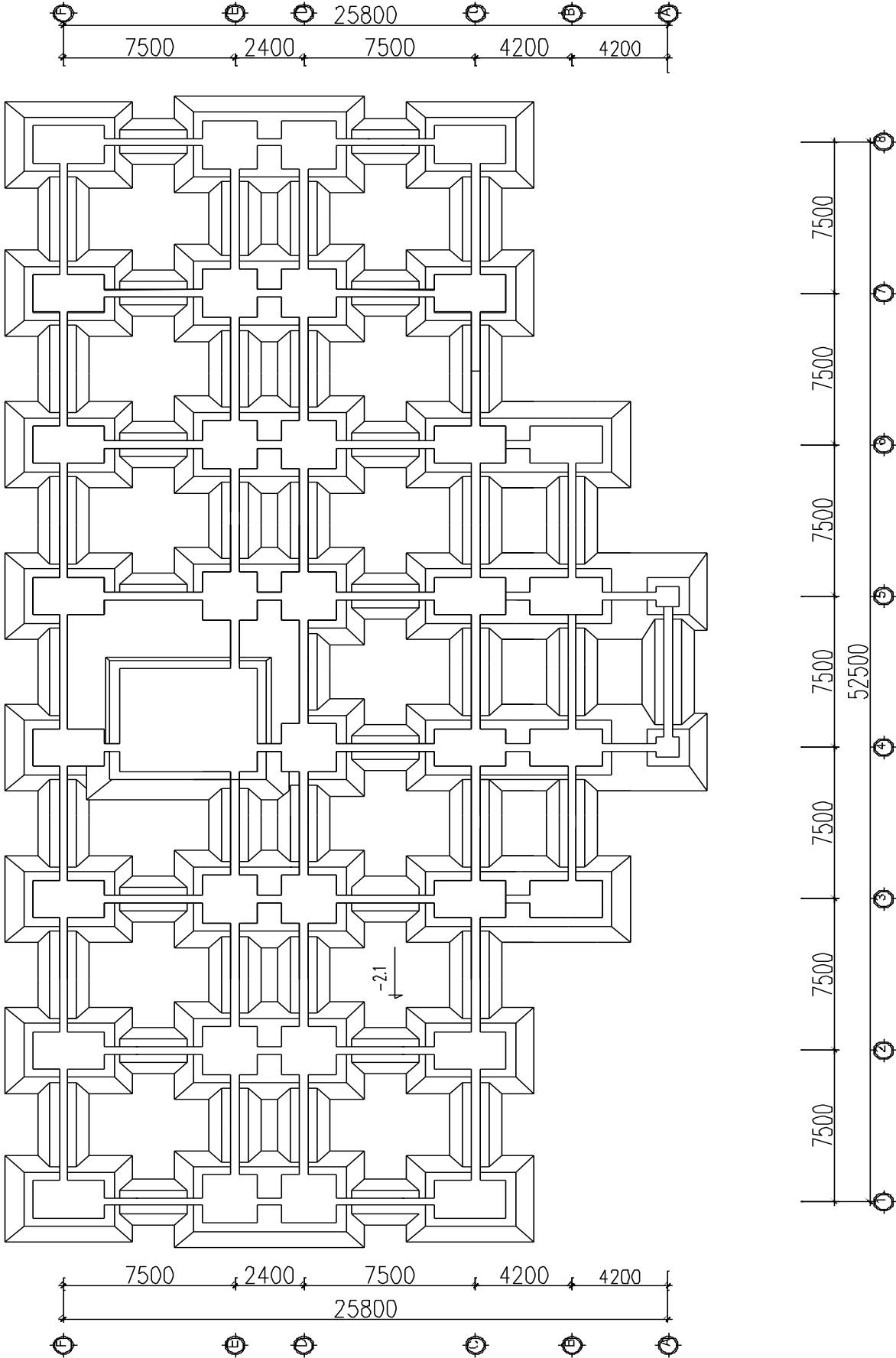
MẶT BẢNG THIẾT KẾ HỒ ĐÀO
