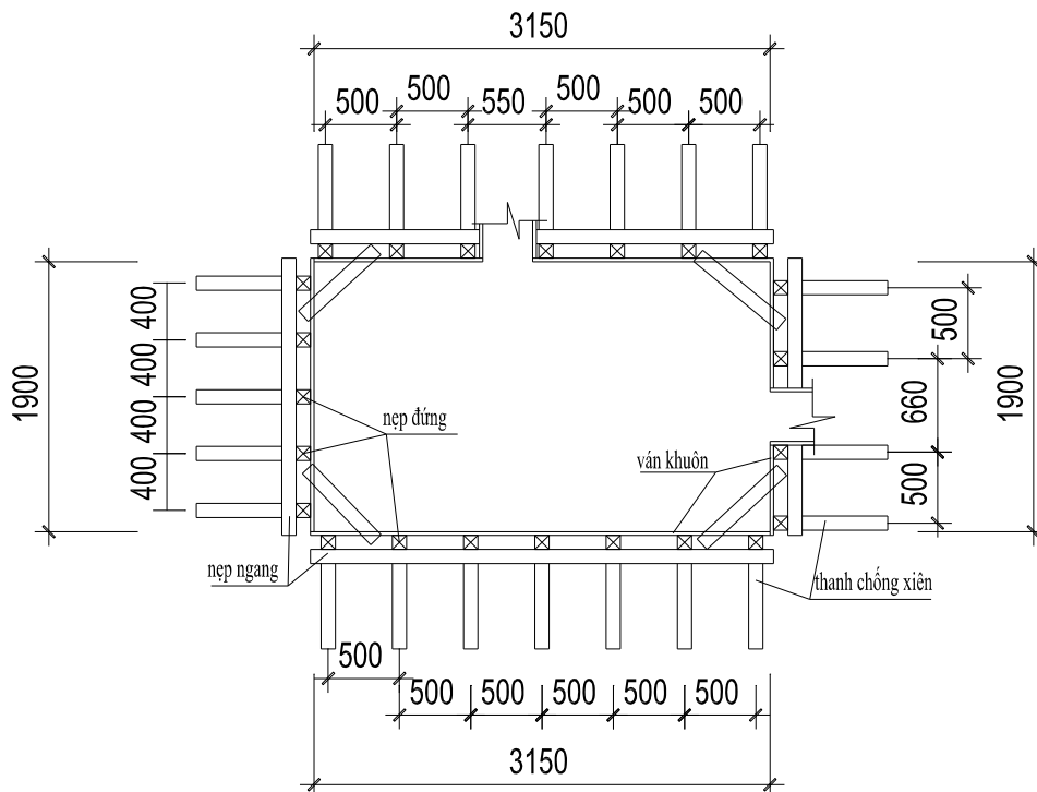
MẶT BẰNG MÓNG M1
