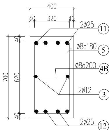
MẶT CẮT CỘT 2 TRỤC D
