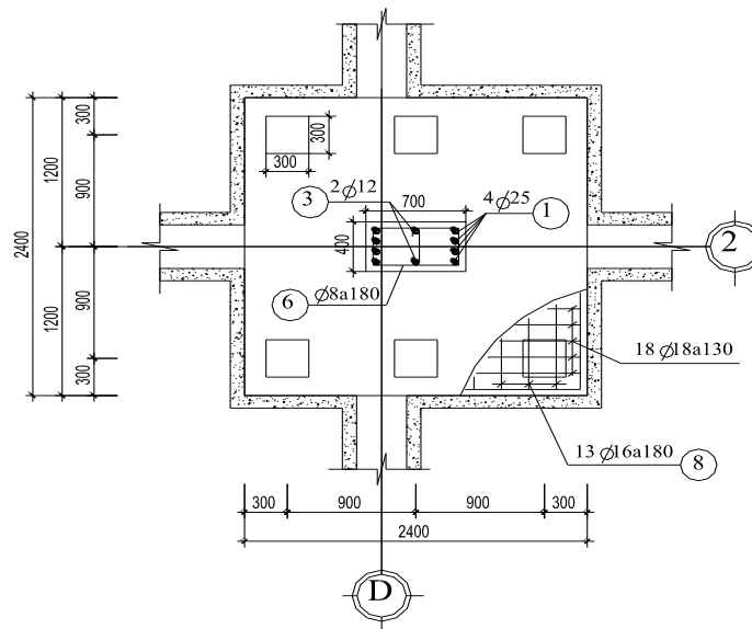
CỐT THÉP ĐÀI CỌC MÓNG M2
