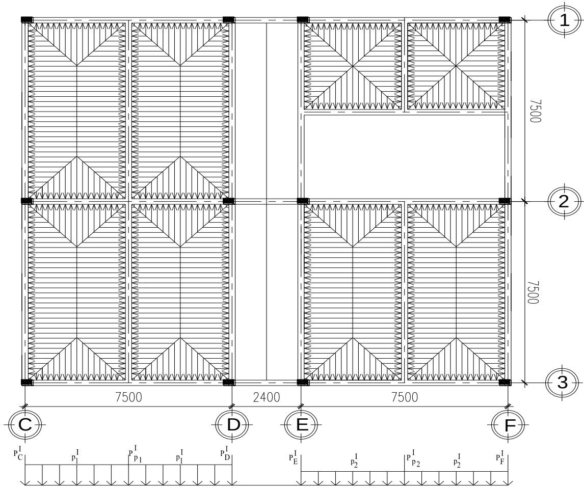
MẶT BẰNG PHÂN BỐ HOẠT TẢI 1 TẦNG 1,3,5
