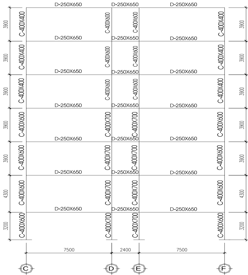
SƠ ĐỒ KHUNG TRỤC 2
