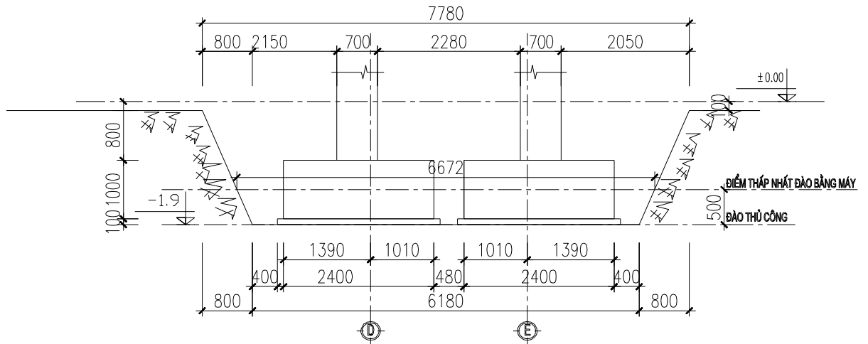
MẶT CẮT DỌC HỒ MÓNG M2( TRỤC D, E)
