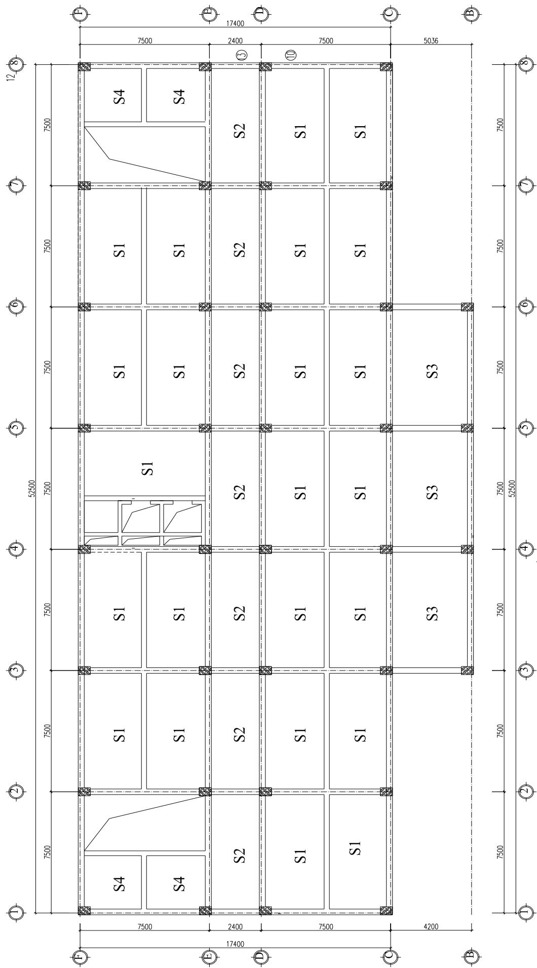
MẶT BẰNG PHÂN CHIA SÀN TẦNG 3
