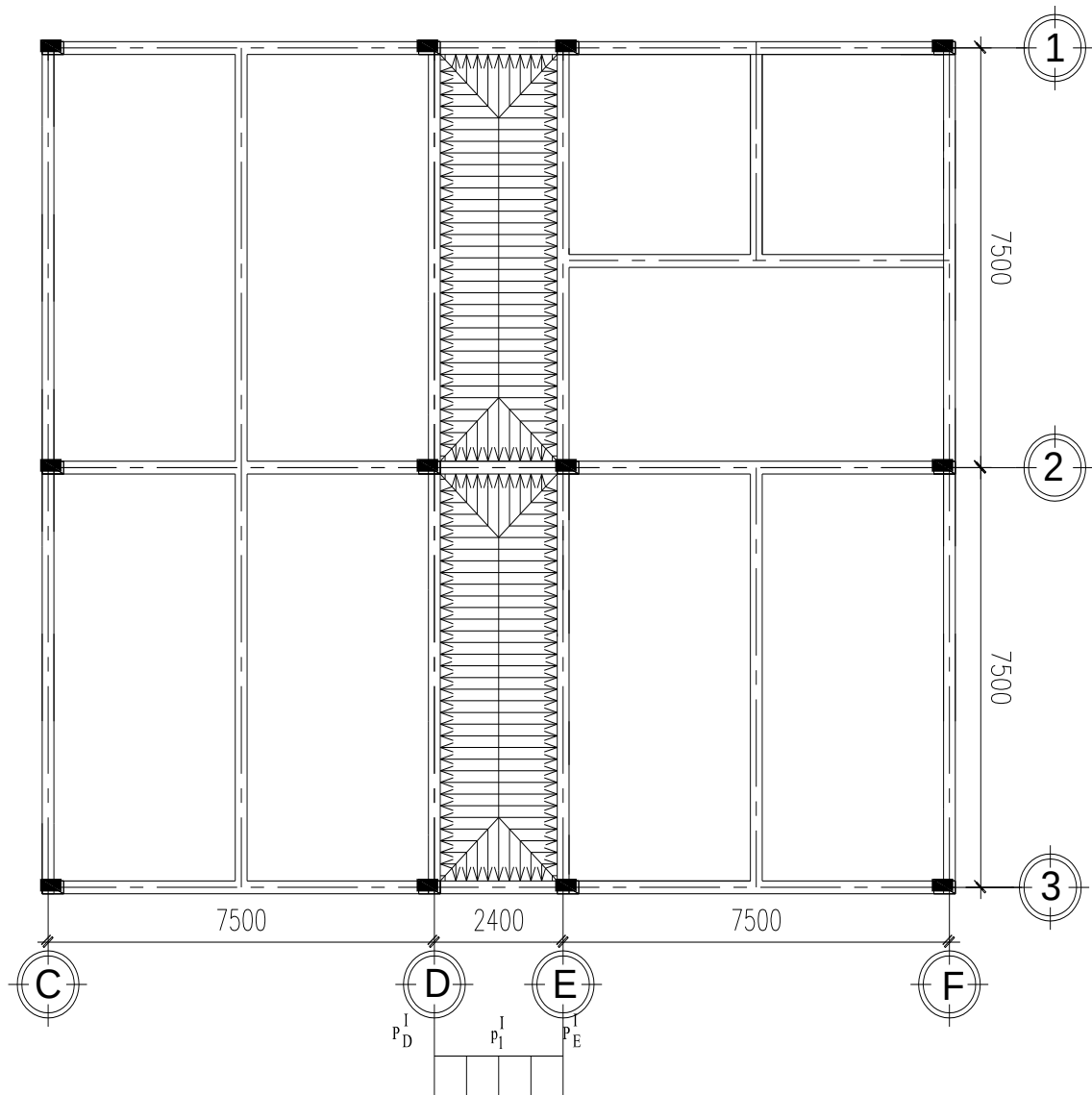
MẶT BẰNG PHÂN BỐ HOẠT TẢI 1 TẦNG 2,4,6
