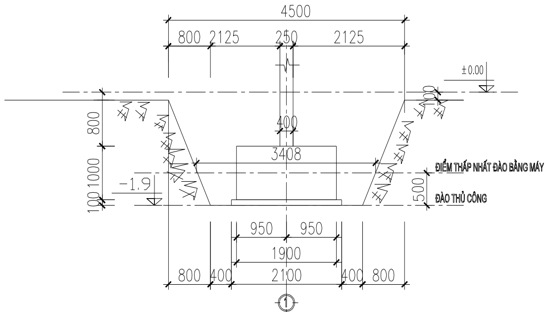
MẶT CẮT NGANG HỐ MÓNG M1( TRỤC C, F)
