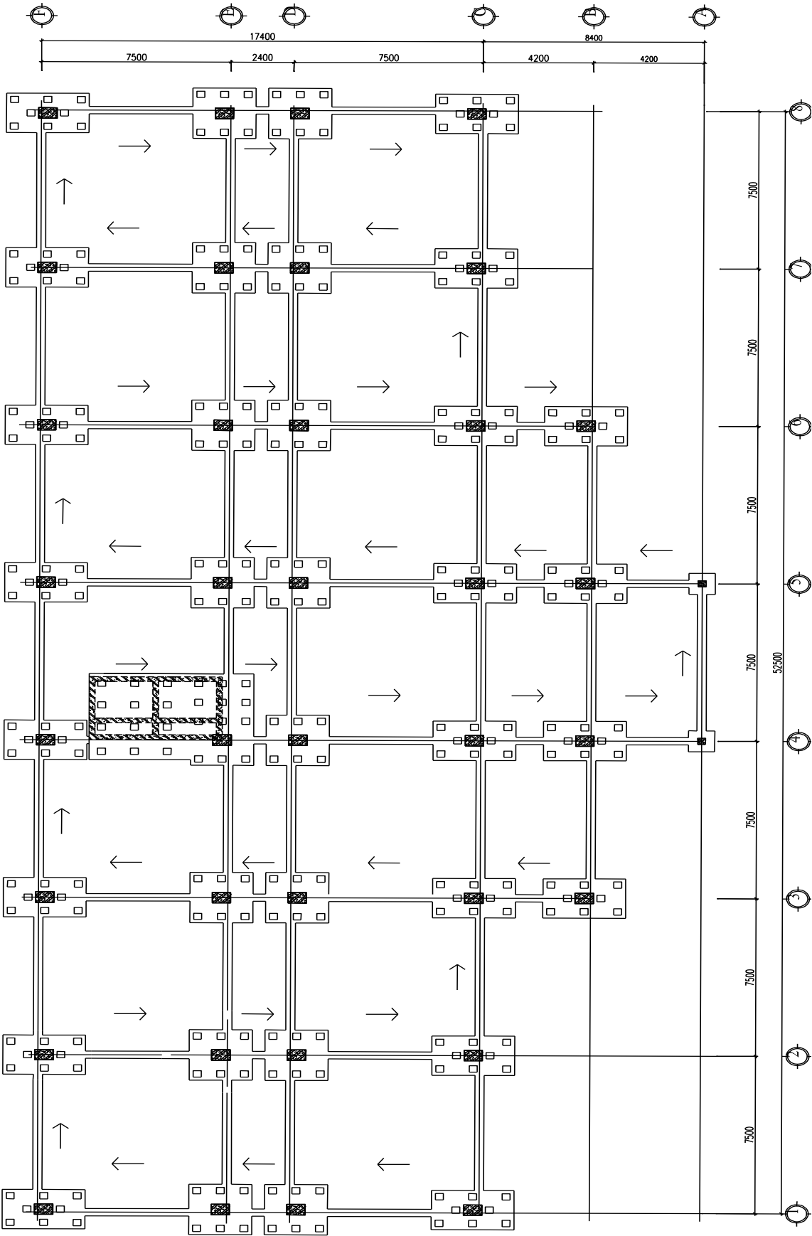
SƠ ĐỒ ÉP CỌC MÓNG
