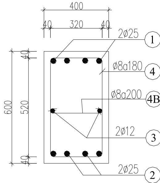
MẶT CẮT CỘT 1 TRỤC C
