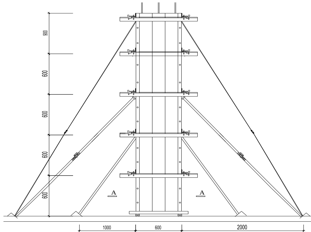
VÁN KHUÔN CỘT TẦNG 3
