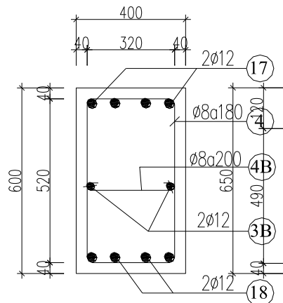
MẶT CẮT CỘT 18 TRỤC D
