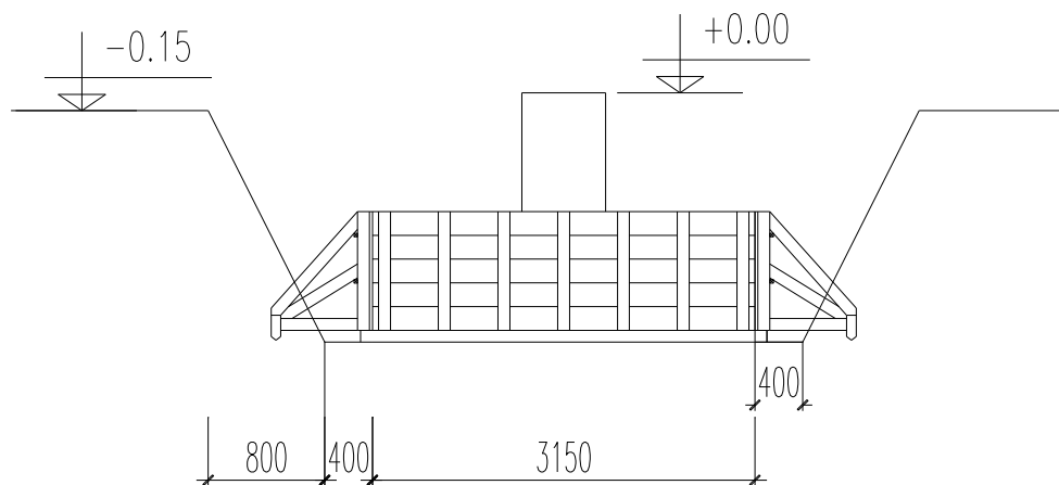
MẶT CẮT VÁN KHUÔN MÓNG
