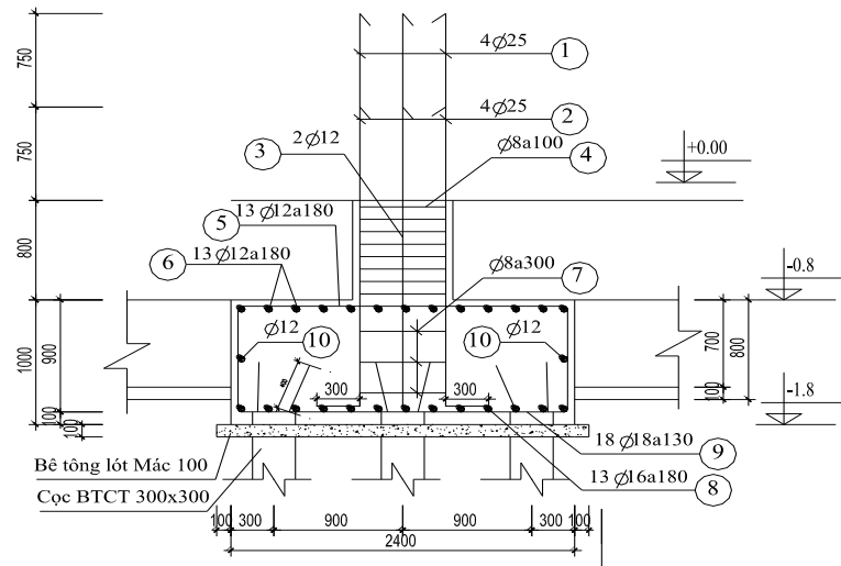
CỐT THÉP ĐÀI CỌC MÓNG M2
