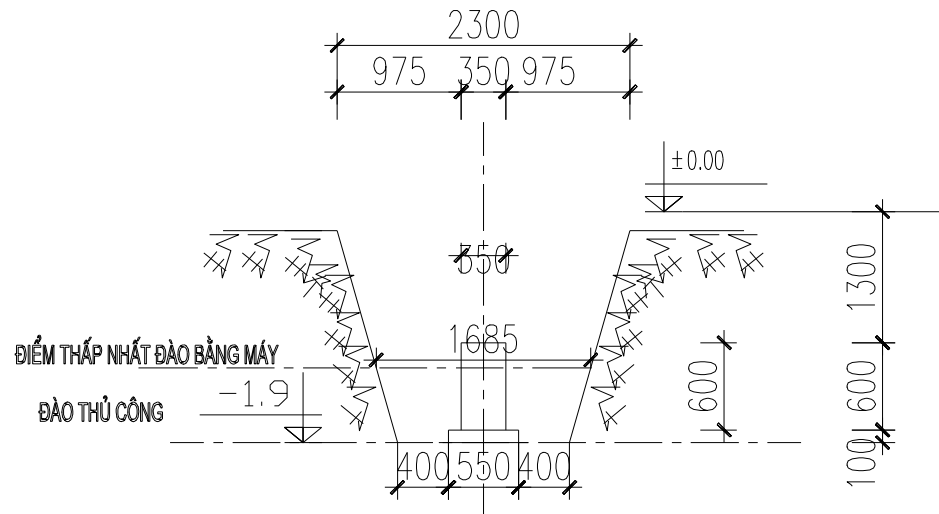
MẶT CẮT NGANG GIĂNG MÓNG
