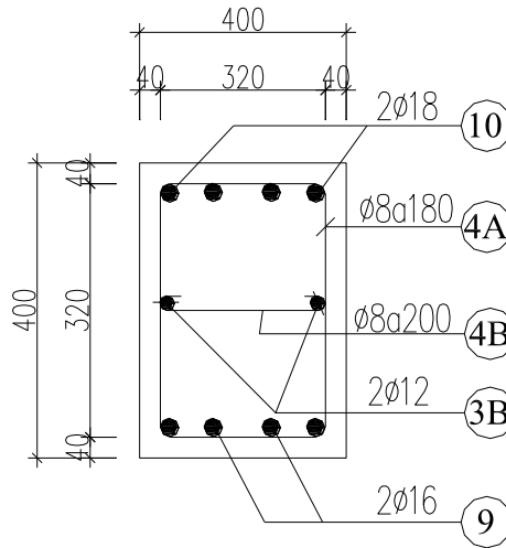
MẶT CẮT CỘT 17 TRỤC C
