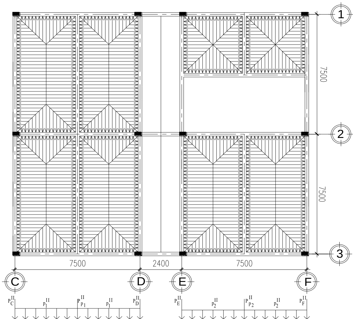
MẶT BẰNG PHÂN BỐ HOẠT TẢI 2 TẦNG 2,4,6
