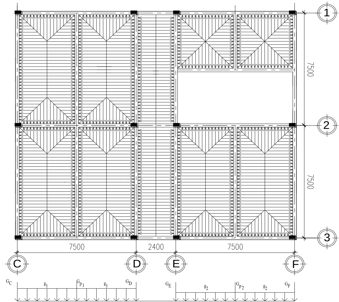
MẶT BẰNG PHÂN BỐ TÍNH TẢI TẦNG 1,2, 3, 4, 5, 6
