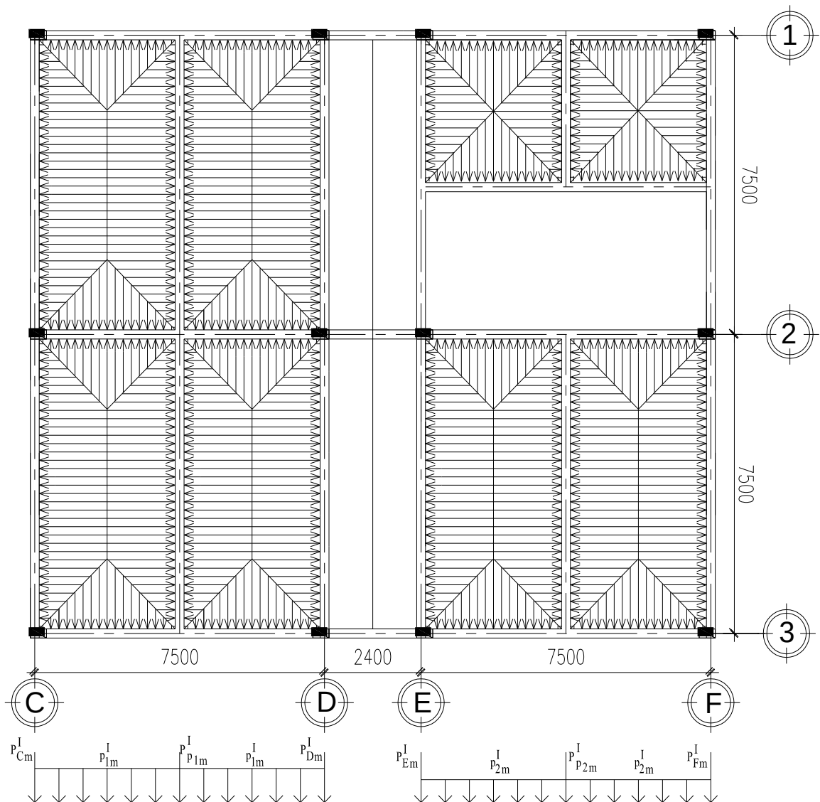
MẶT BẰNG PHÂN BỐ HOẠT NHỊP 1 TẦNG MÁI
