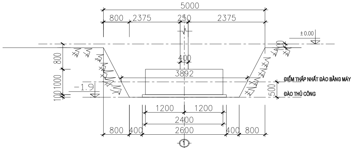
MẶT CẮT NGANG HỒ MÓNG M2( TRỤC D, E)
