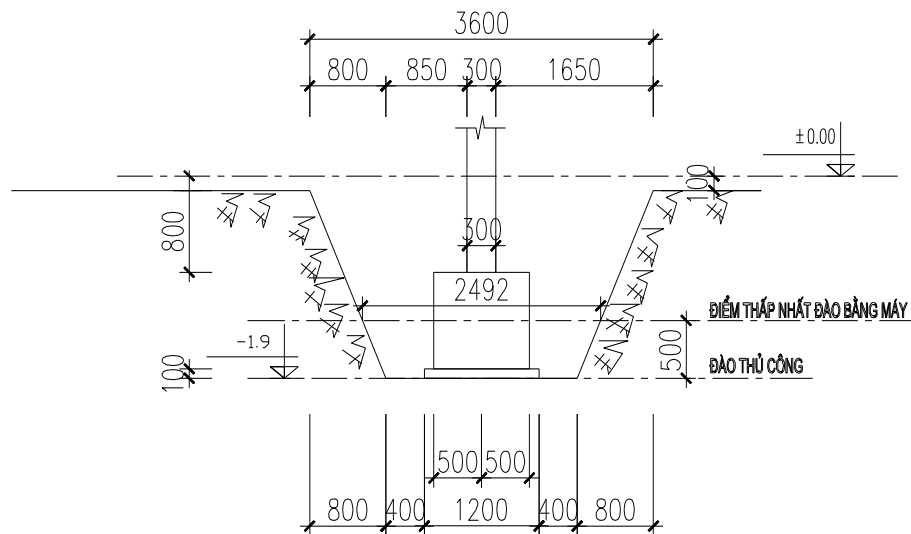
MẶT CẮT HỒ MÓNG M3 (TRỤC A)
