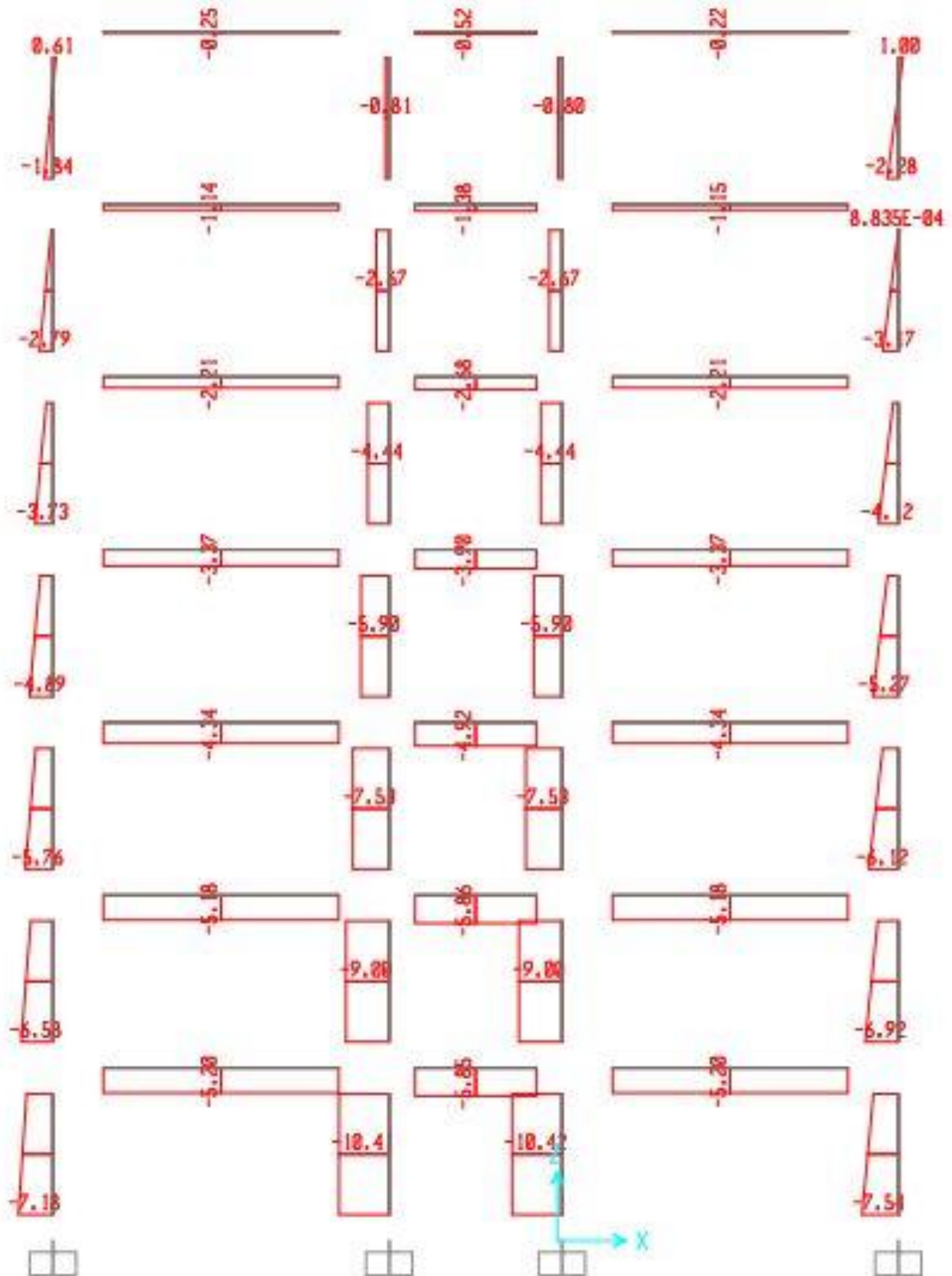
LỰC CẮT DO GIÓ PHẢI TÁC DỤNG LÊN KHUNG K10
