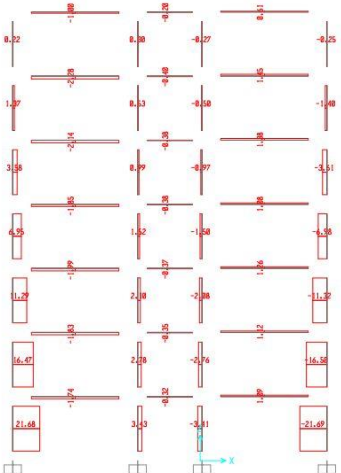
LỰC DỌC DO GIÓ TRÁI TÁC DỤNG LÊN KHUNG K10
