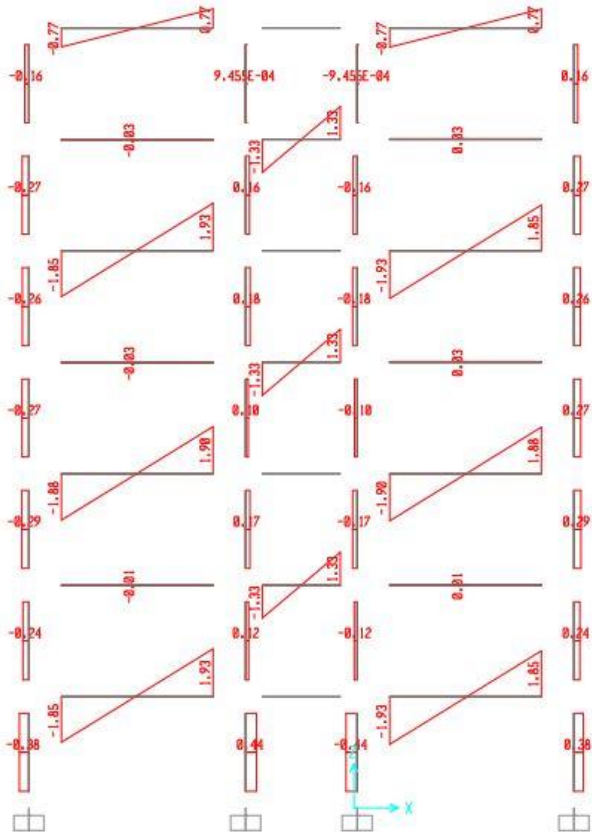
LỰC CẮT DO HOẠT TẢI 1 TÁC DỤNG LÊN KHUNG K10
