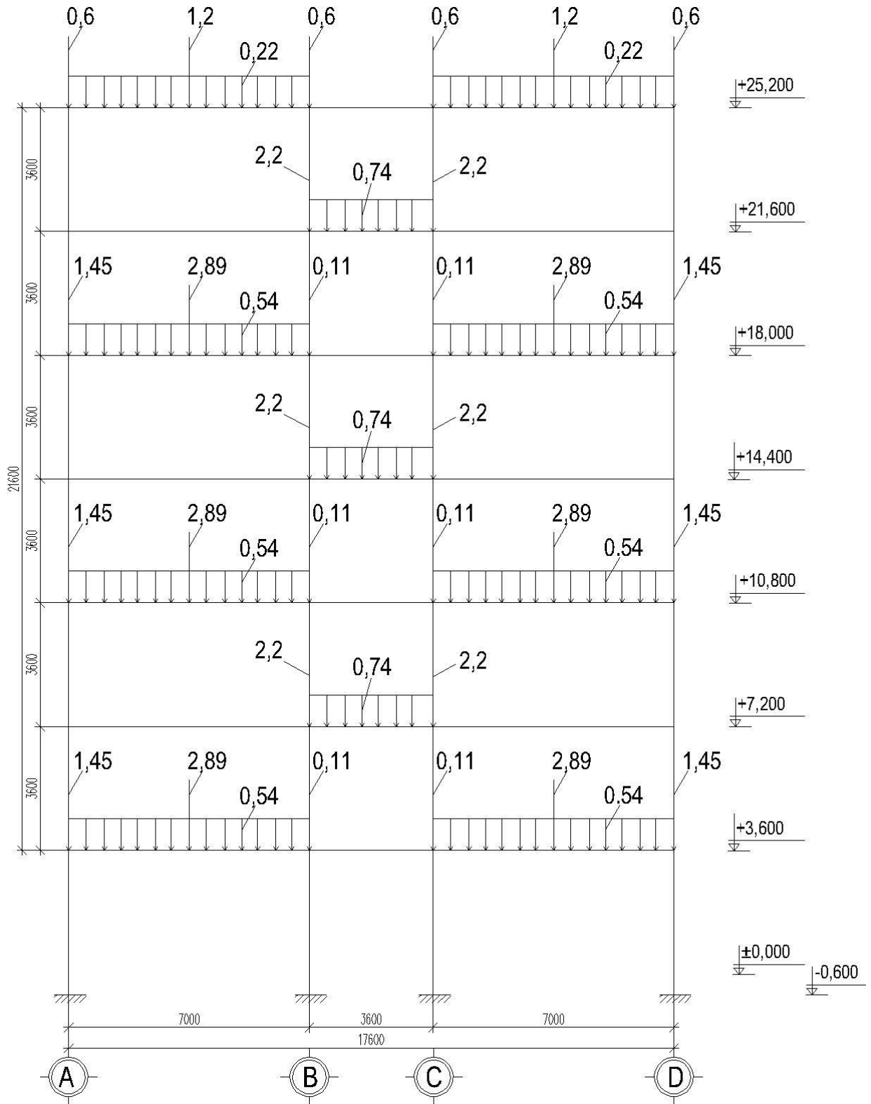
SƠ ĐỒ HOẠT TẢI 1 TÁC DỤNG LÊN KHUNG TRỤC 10 (ĐV: TẤN)
