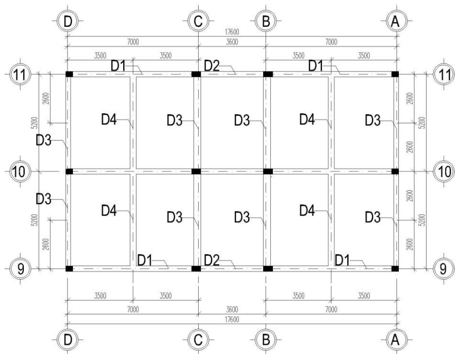
Mặt bằng khung K10
