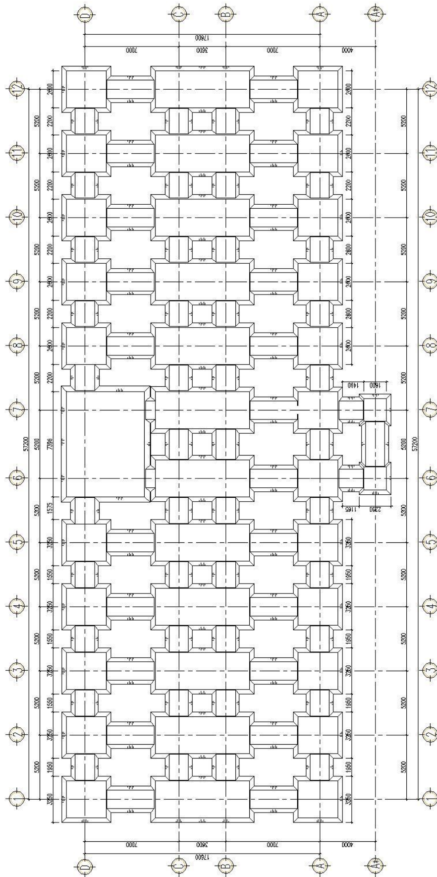
MẶT BẰNG HỒ ĐÀO
