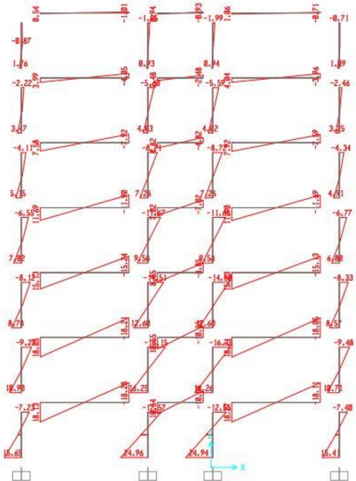
MOMEN DO GIÓ TRÁI TÁC DỤNG LÊN KHUNG K10
