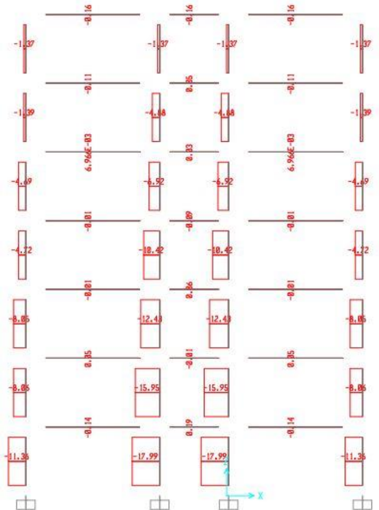
LỰC DỌC DO HOẠT TẢI 1 TÁC DỤNG LÊN KHUNG K10
