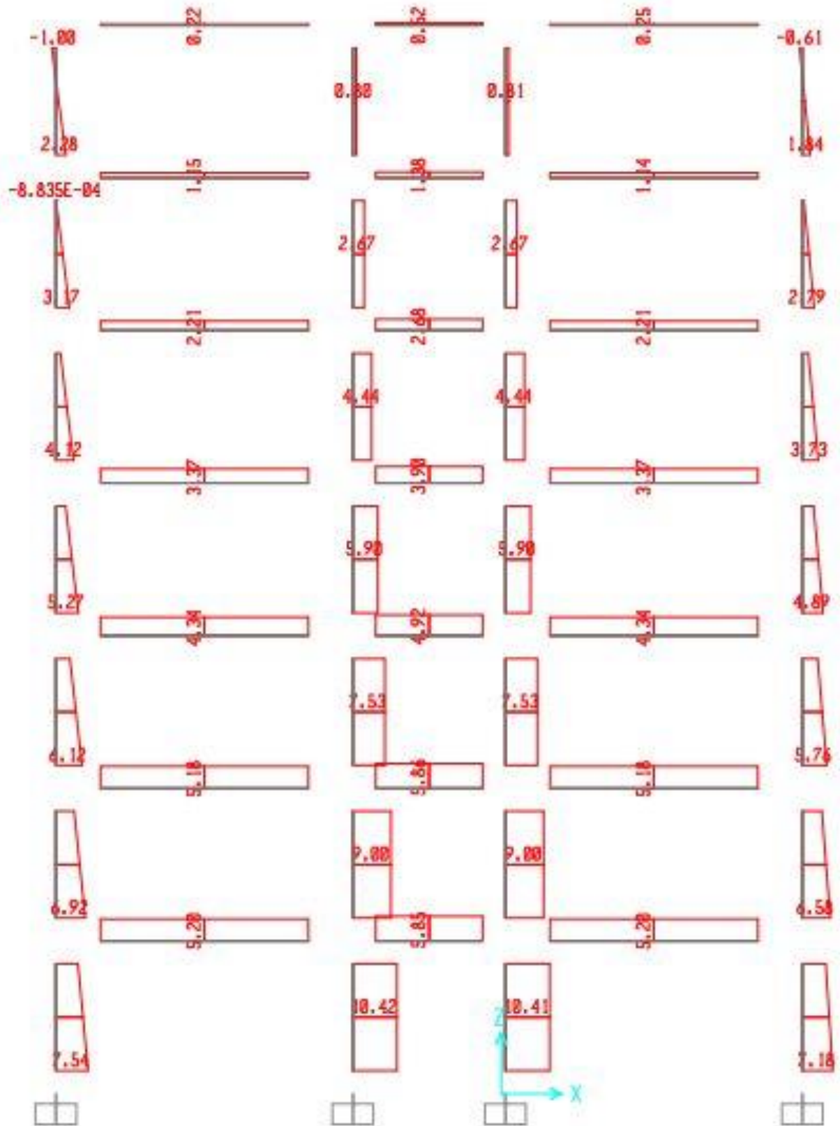
LỰC CẮT DO GIÓ TRÁI TÁC DỤNG LÊN KHUNG K10
