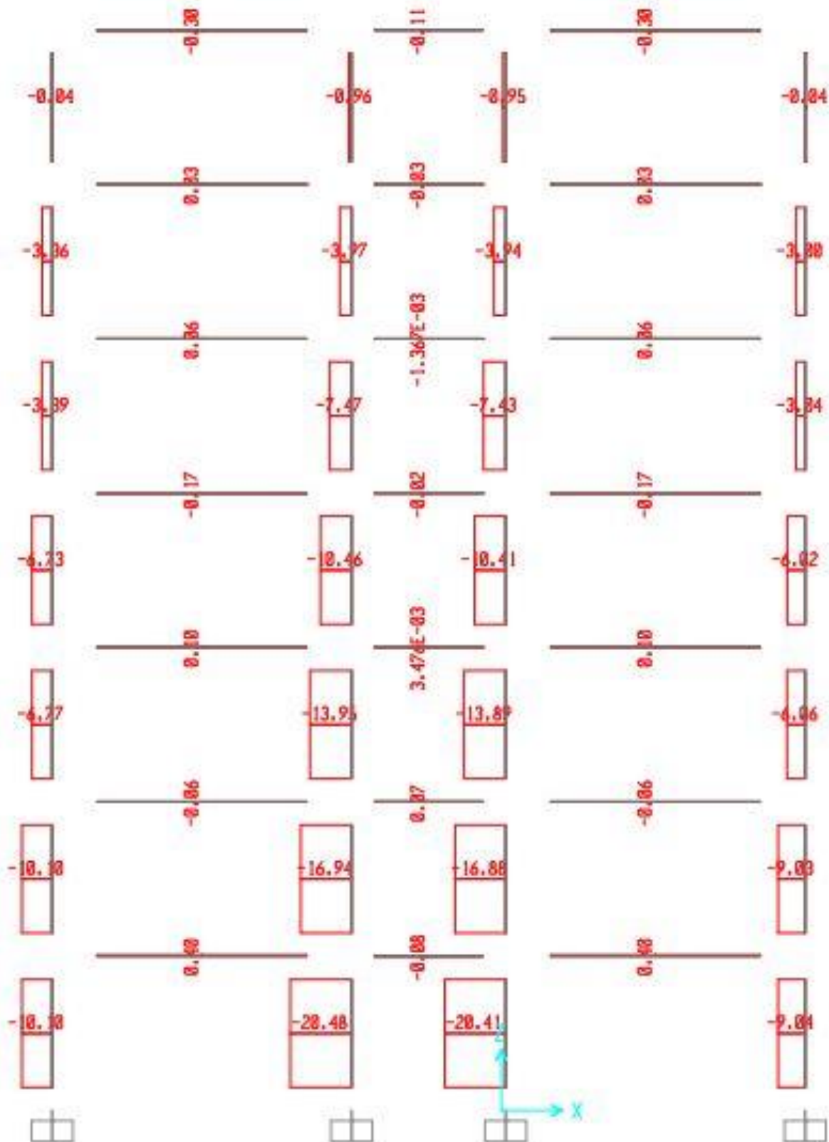
LỰC DỌC DO HOẠT TẢI 2 TẮC DỰNG LÊN KHUNG K10
