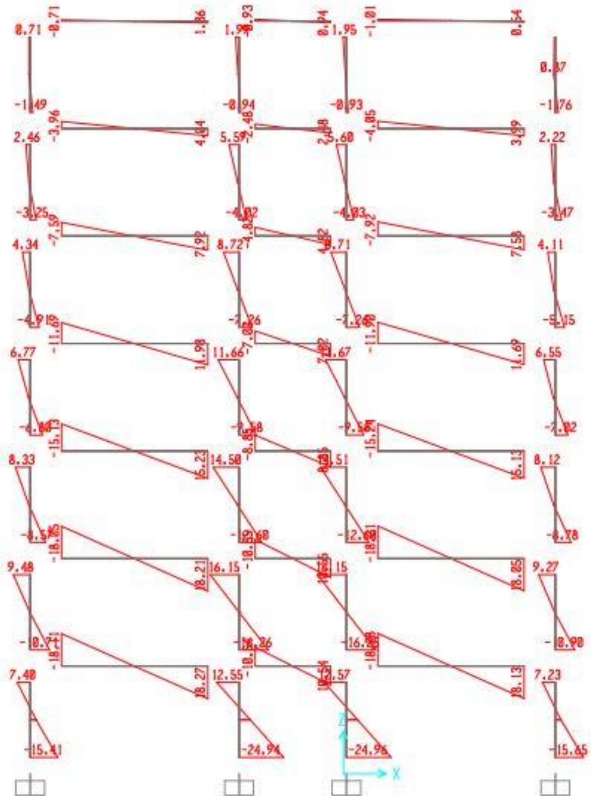
MOMEN DO GIÓ PHẢI TÁC DỤNG LÊN KHUNG K10
