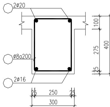
Mặt cắt dầm 42
