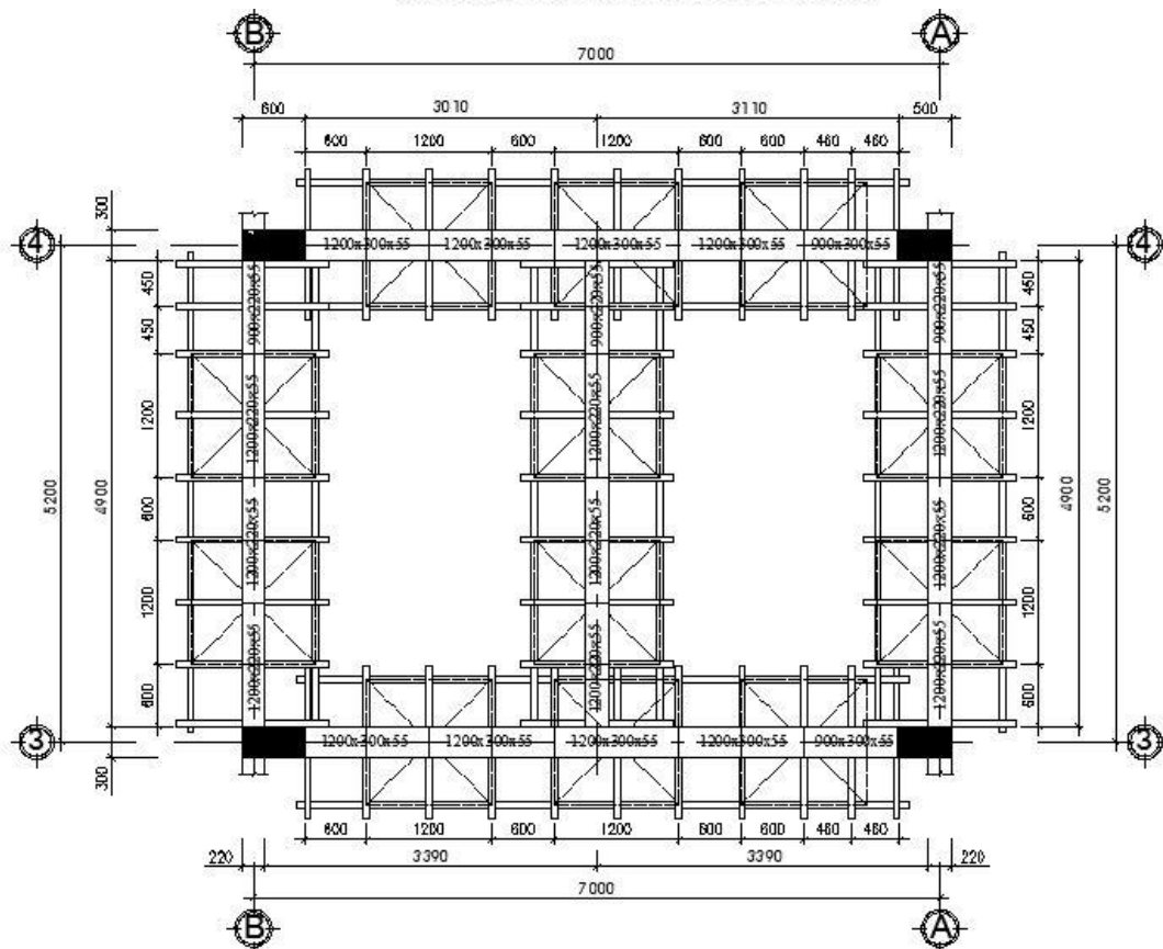
MẶT BẰNG BỐ TRÍ VÁN KHUÔN Ở SÀN ĐIỀN HÌNH
