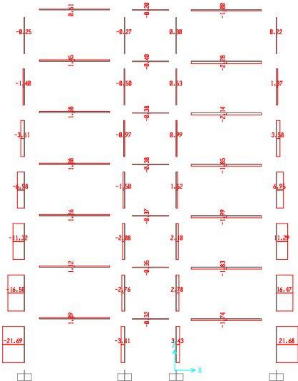
LỰC DỌC DO GIÓ PHẢI TÁC DỤNG LÊN KHUNG K10
