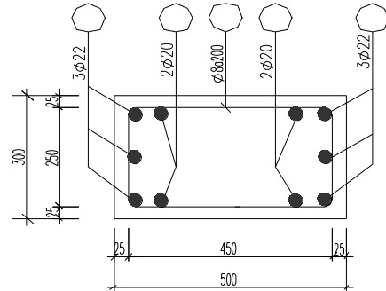
Mặt cắt cột
