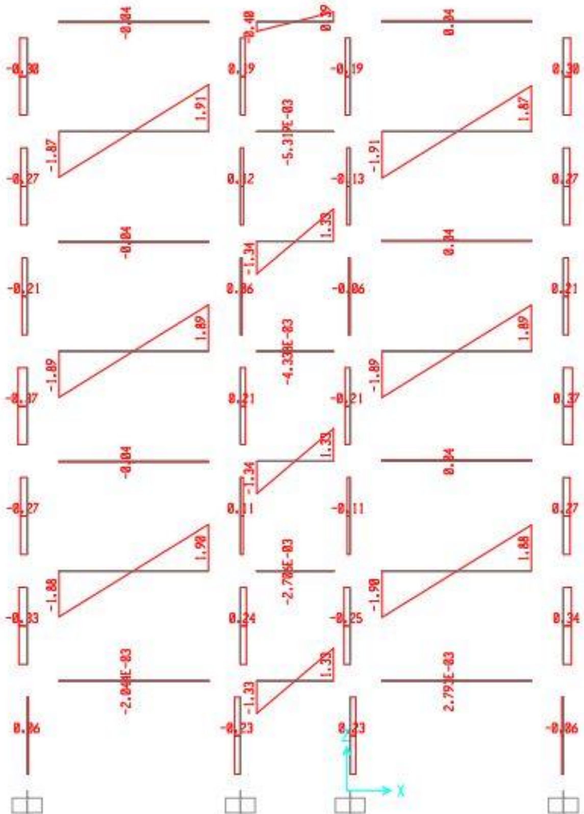
LỰC CẮT DO HOẠT TẢI 2 TÁC DỤNG LÊN KHUNG K10
