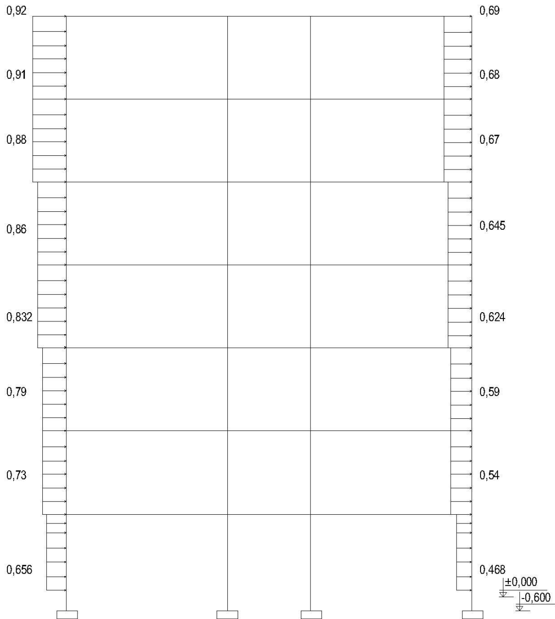
SƠ ĐỒ HOẠT TẢI GIÓ TRÁI TÁC DỤNG LÊN KHUNG TRỤC 10 (ĐV:TẤN/M)
