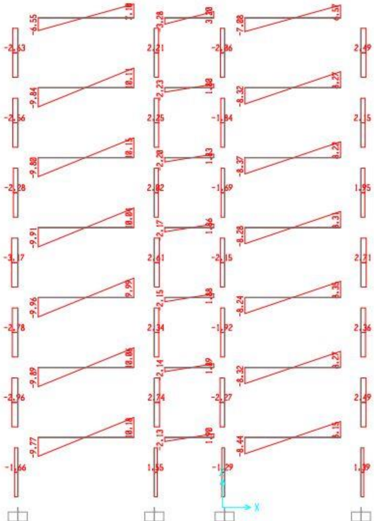
LỰC CẮT DO TÍNH TẢI TÁC DỤNG LÊN KHUNG K10
