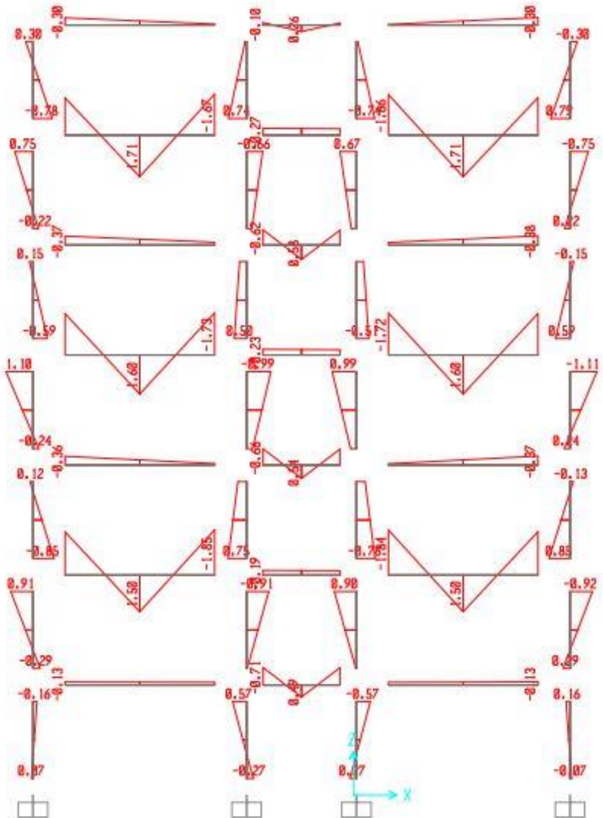
MOMEN DO HOẠT TẢI 2 TÁC DỤNG LÊN KHUNG K10
