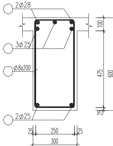
Mặt cắt dầm 29
