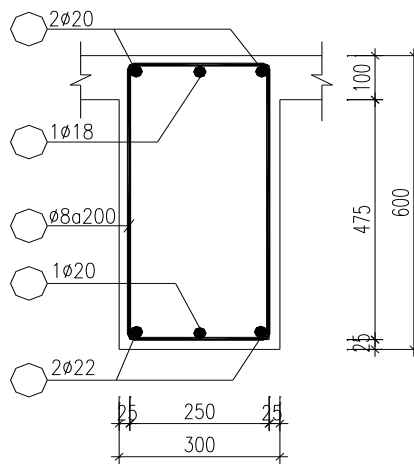
Mắt cắt dầm 35
