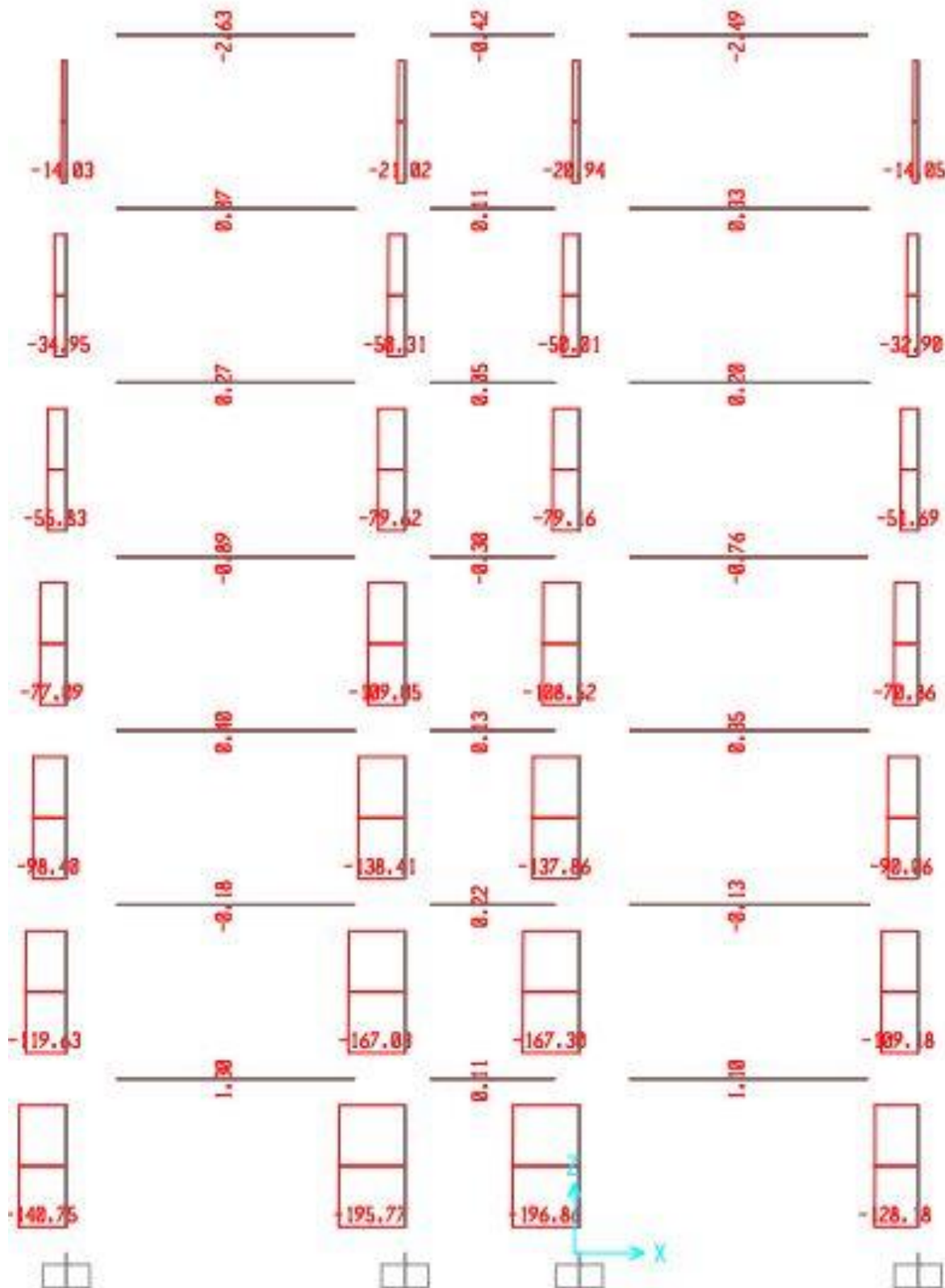
LỰC DỌC DO TÍNH TẢI TẢI DỤNG LÊN KHUNG K10
