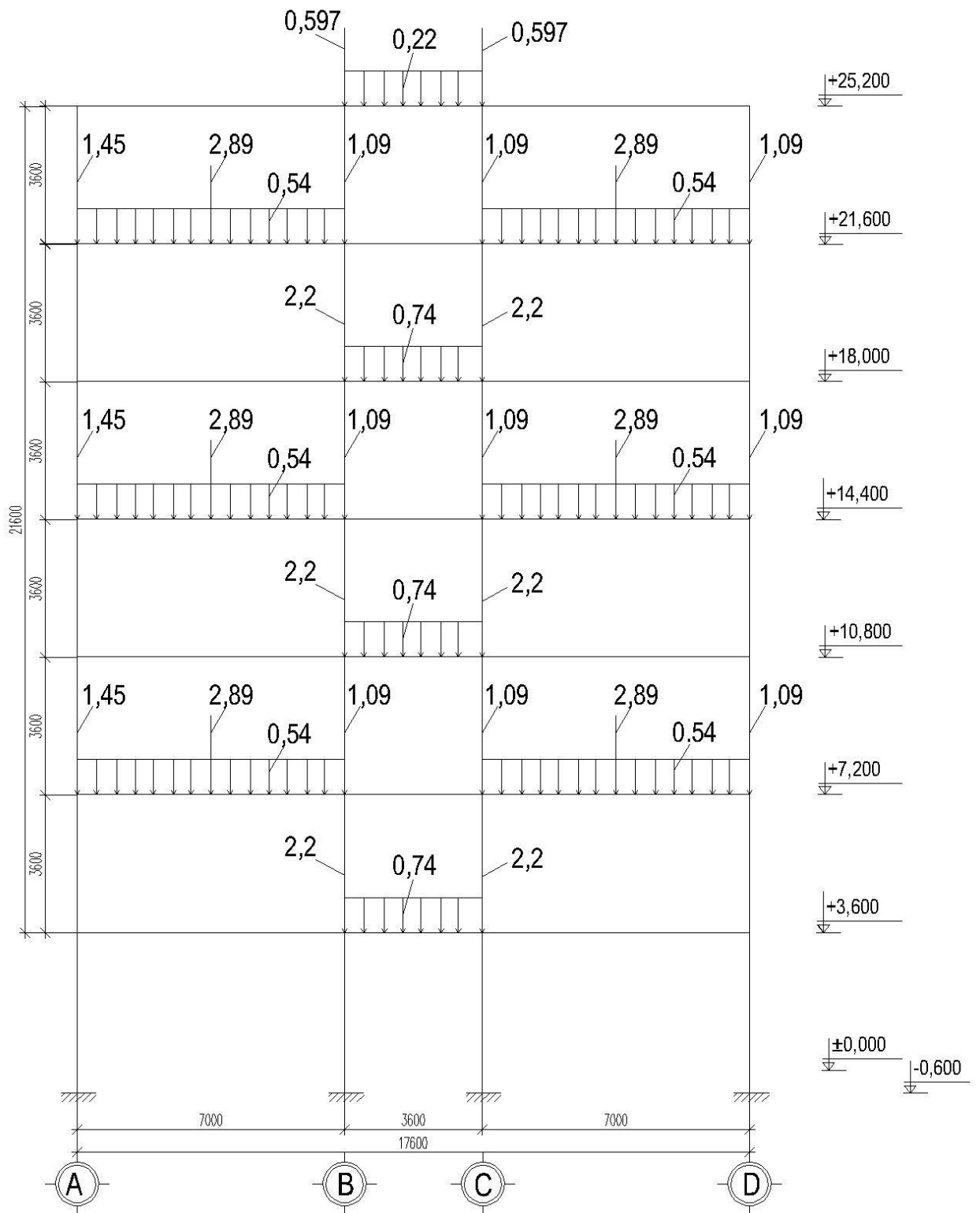
SƠ ĐỒ HOẠT TẢI 2 TÁC DỤNG LÊN KHUNG TRỤC 10 (ĐV: TẤN)
