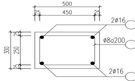
Mặt cắt cột trục B
