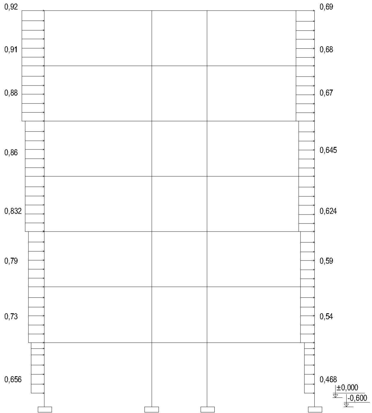
SƠ ĐỒ HOẠT TẢI GIÓ PHẢI TÁC DỤNG LÊN KHUNG TRỤC 3 (ĐV: TẤN/M)
