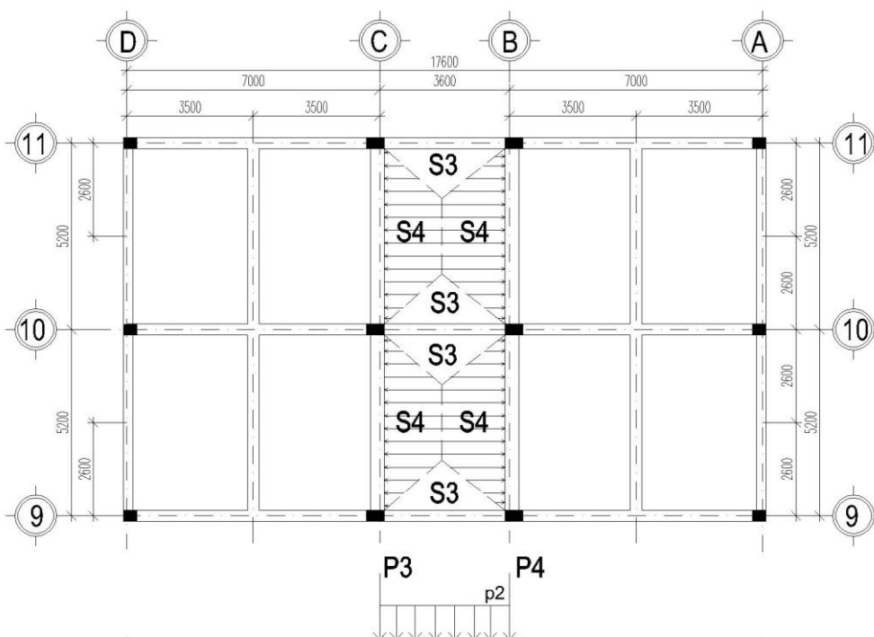
Sơ đồ hoạt tải mái tác dụng trường hợp 2
