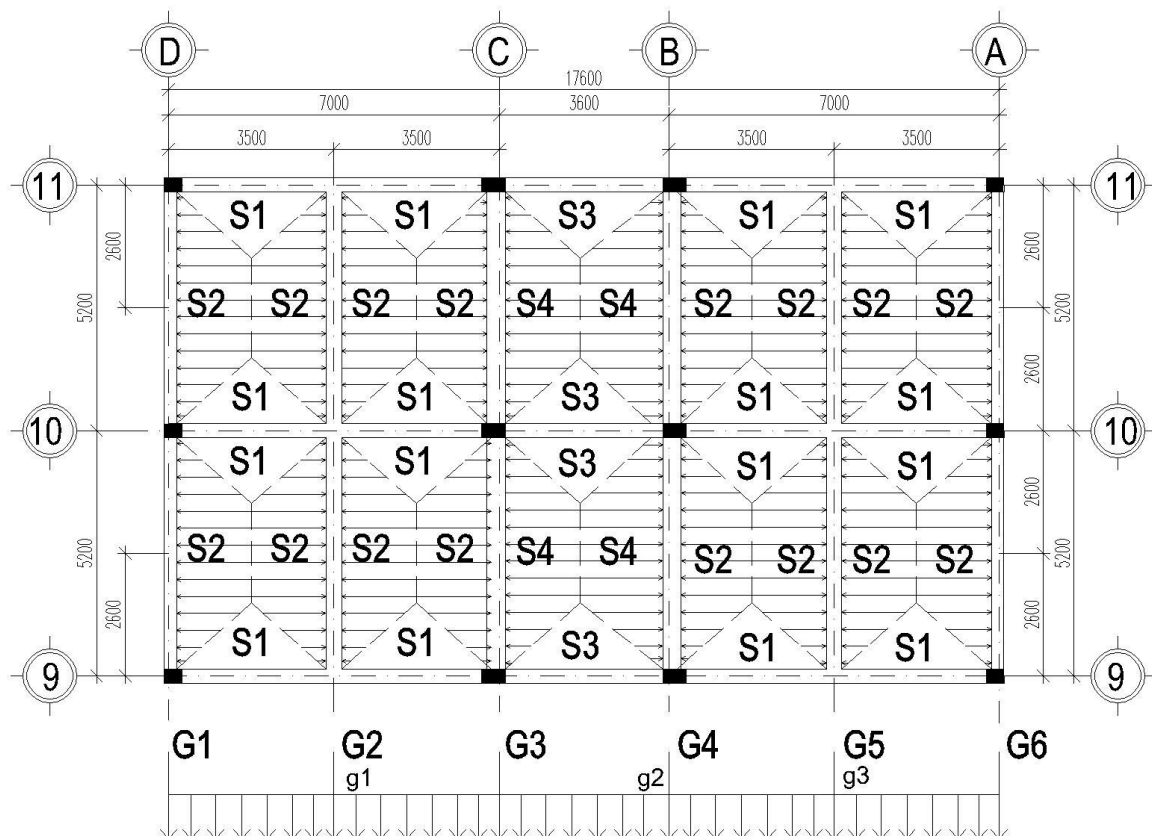
Sơ đồ truyền tải lên khung trục 10
