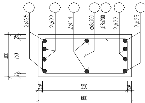
Mặt cắt cột trục
