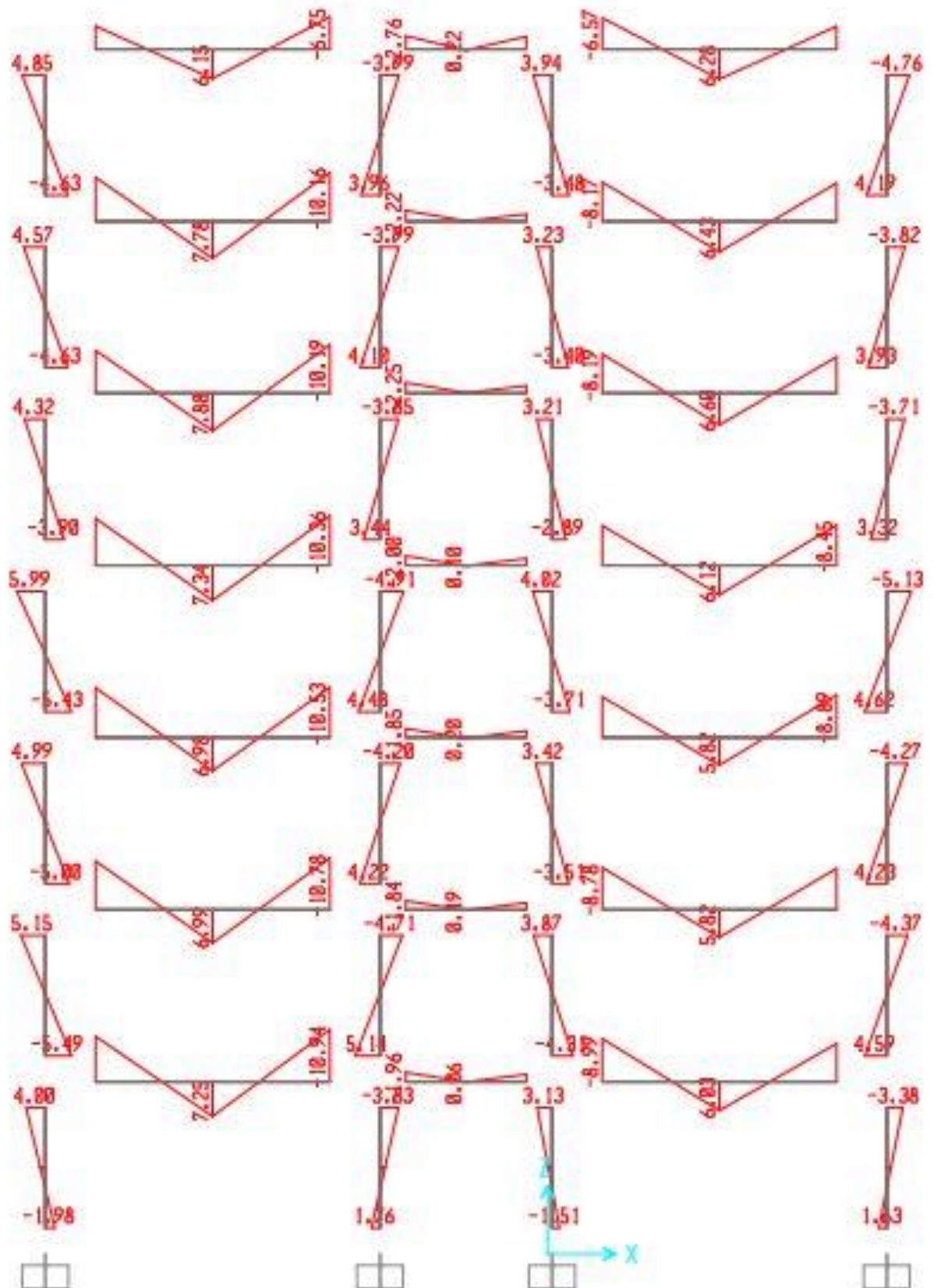
MOMEN DO TÍNH TẢI TÁC DỤNG LÊN KHUNG K10
