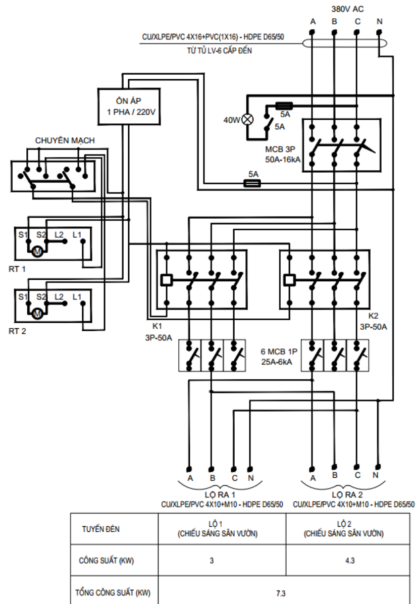
Sơ đồ đấu nối tủ điện chiếu sáng ngoài nhà
