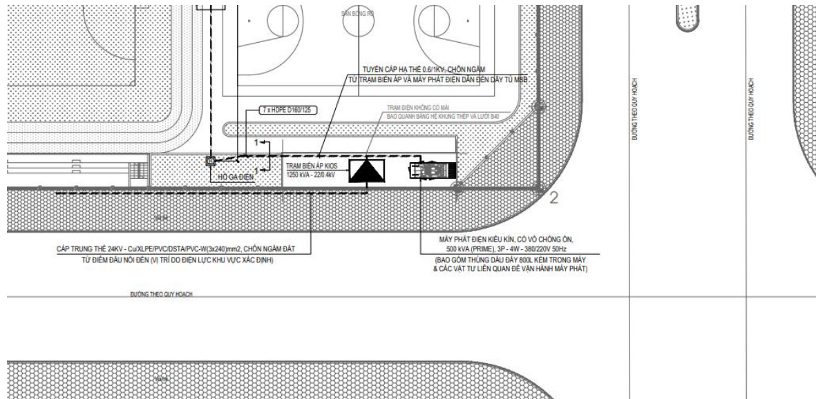
Hình 3.2 Vị trí đặt trạm biến áp
