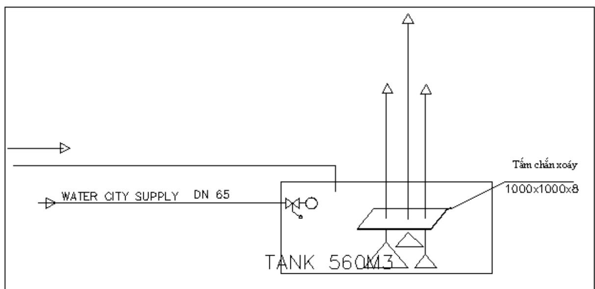
Hình 3.10 Sơ đồ tách riêng 2 rọ bơm số 1 và bơm số 2
