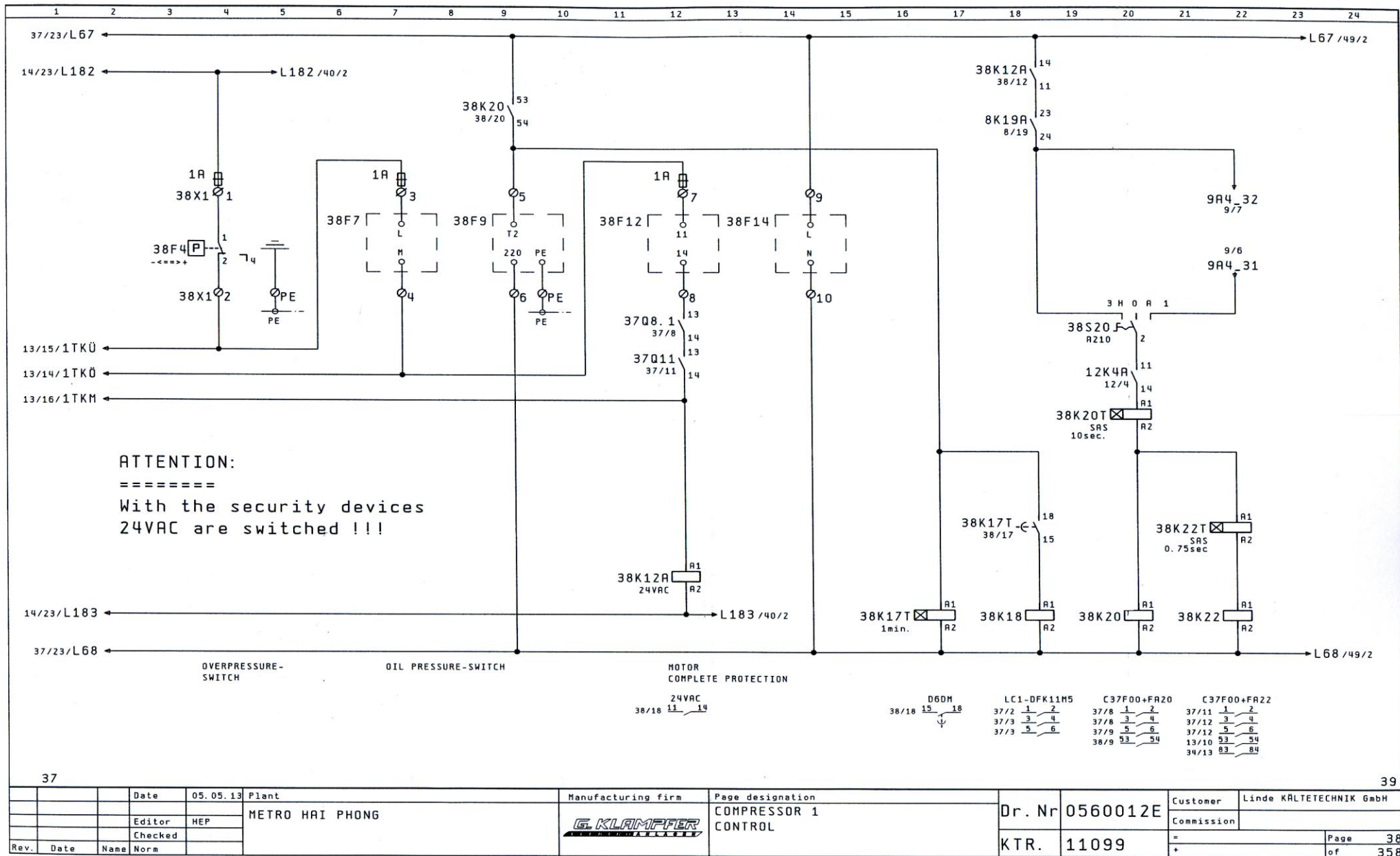
Hình 2.5. Mạch điều khiển máy nén lạnh của hệ thống lạnh sâu
