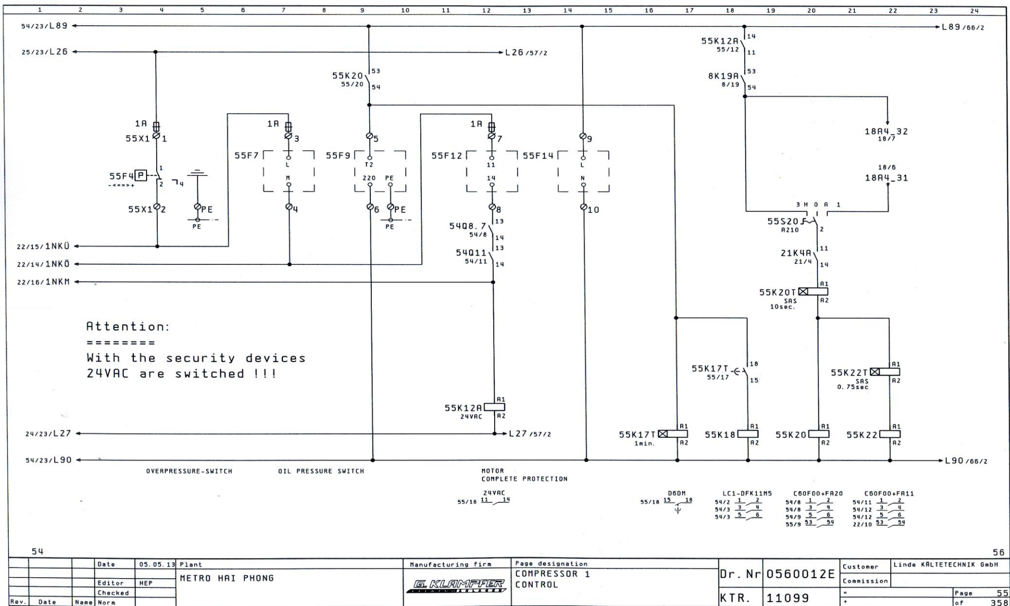
Hình 2.8. Mạch điều khiển máy nén lạnh của hệ thống lạnh duy trì thực phẩm
