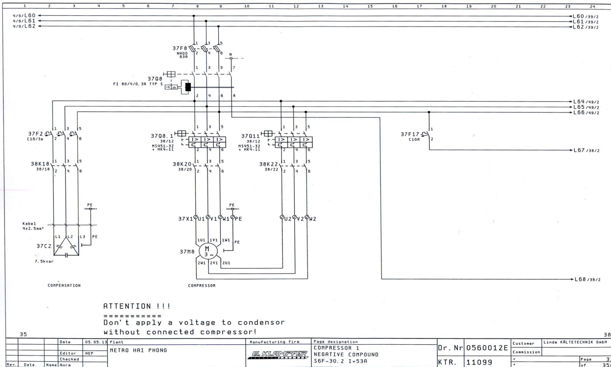
Hình 2.4. Mạch động lực máy nén lạnh của hệ thống lạnh sâu
