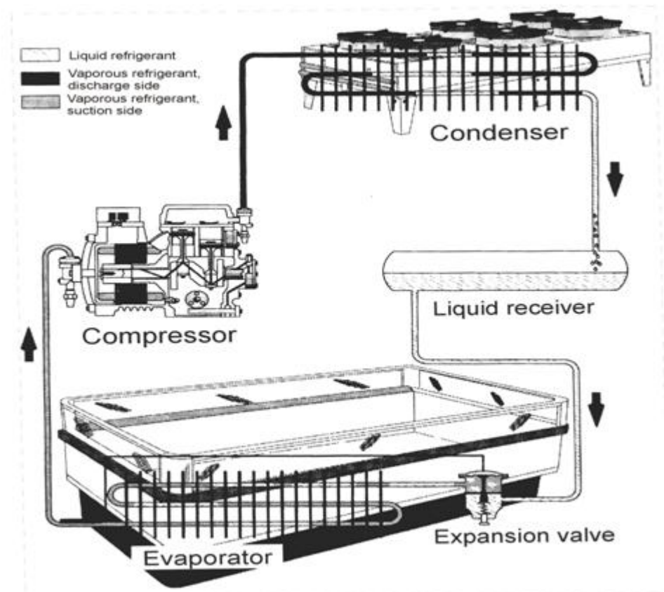
Hình 2.1. Cấu trúc của hệ thống lạnh hệ âm trong siêu thị Metro Hải Phòng
