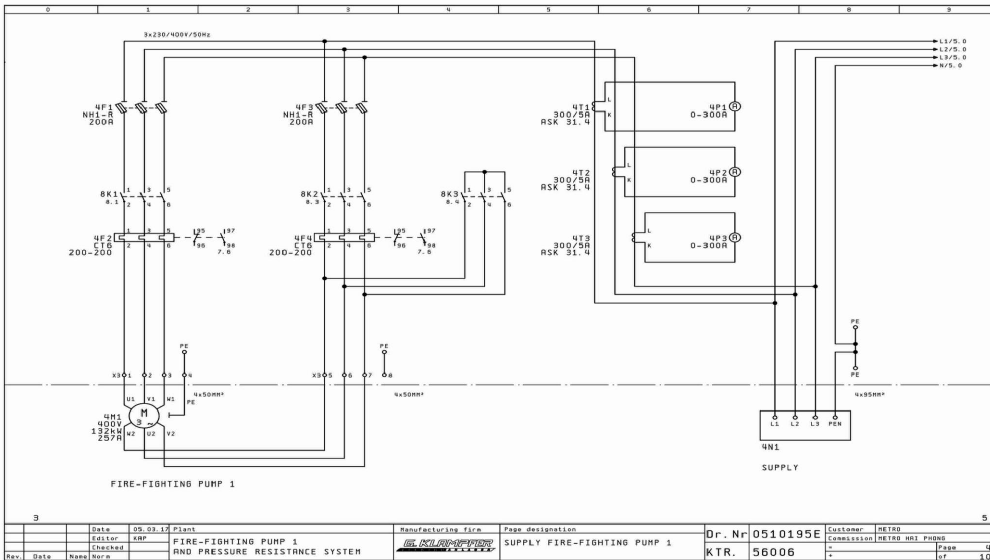
Hình 3.7. Mạch động lực của động cơ lai bơm số 1
