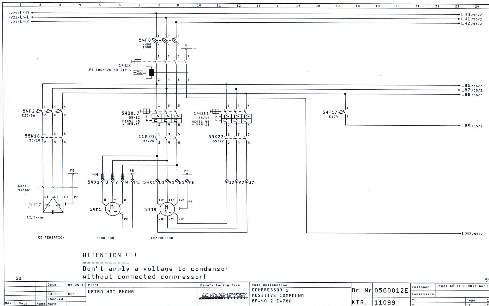
Hình 2.7. Mạch động lực máy nén lạnh của hệ thống lạnh duy trì thực phẩm
