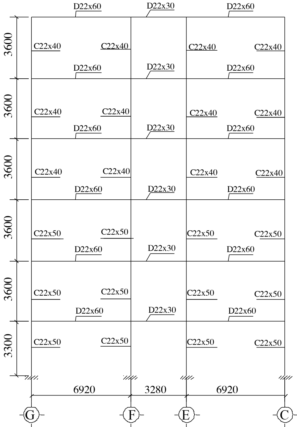
Hình 2.1: Sơ đồ kết cấu khung ngang
