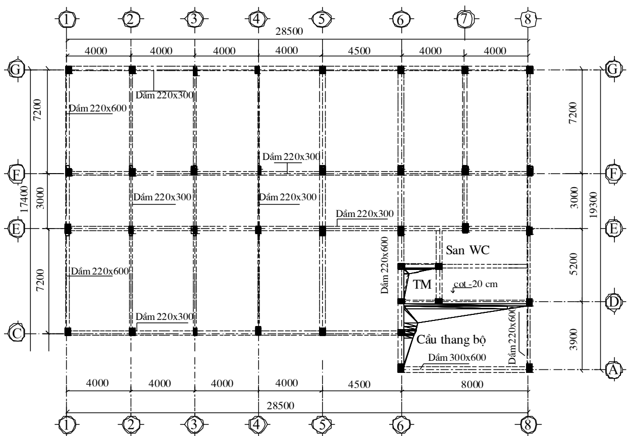
Hình 4.3: Mặt bằng kết cấu tầng điển hình
