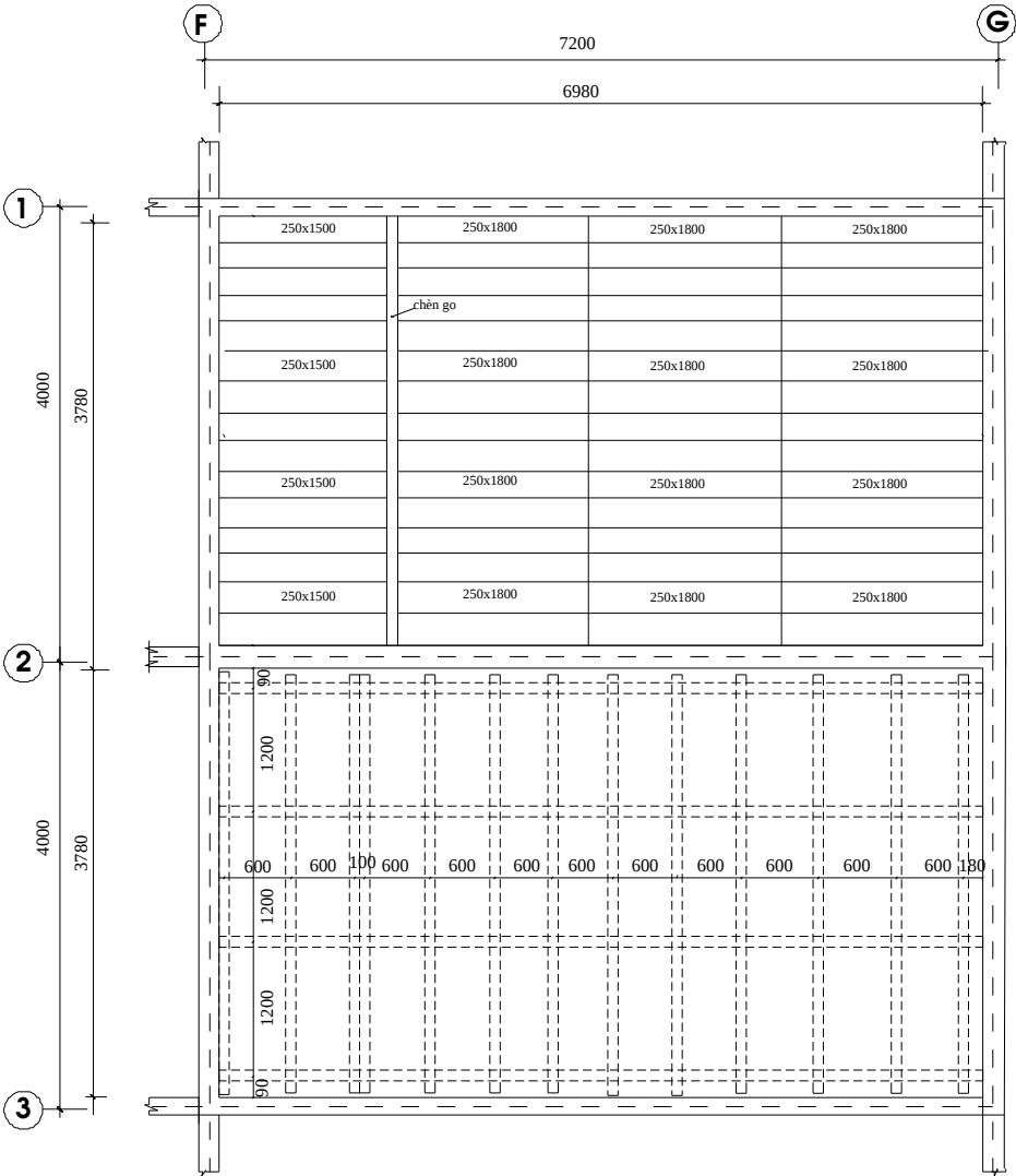
Mặt bằng bố trí xà gồ ô sàn S1
