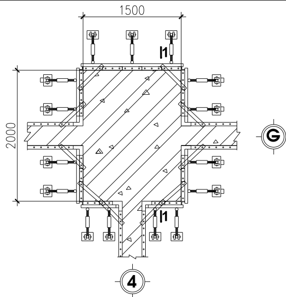
MẶT BẰNG VÁN KHUÔN ĐÀI MÓNG M1
