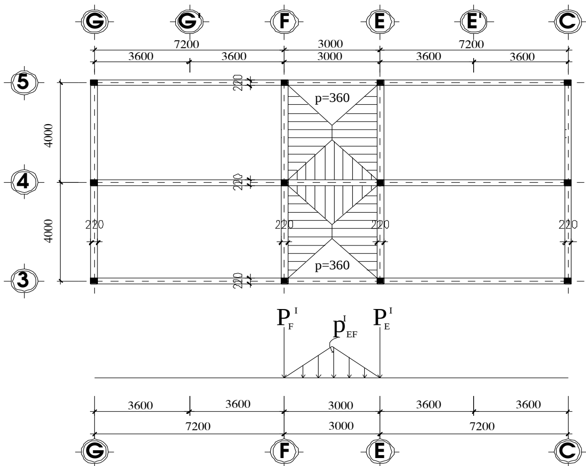
Mặt bằng truyền tải và sơ đồ dòn tải hoạt tải 1- tầng 3
