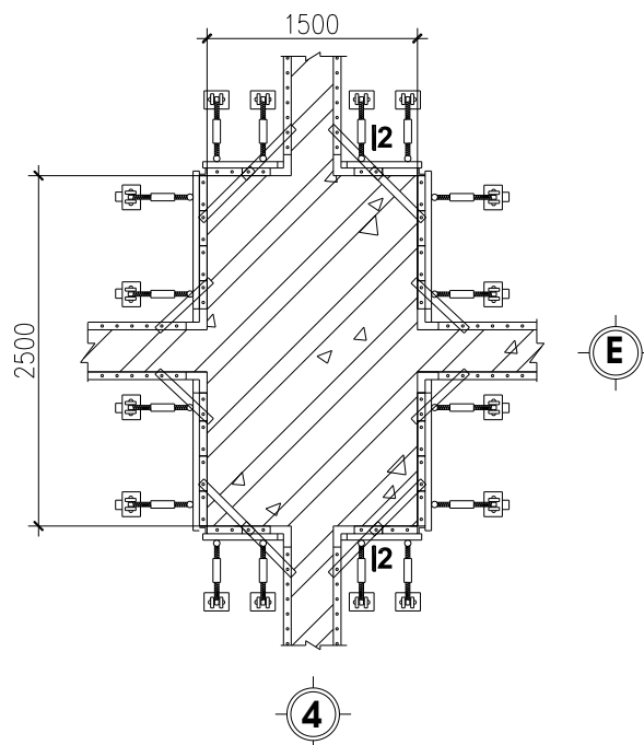
MẶT BẰNG VÁN KHUÔN ĐÀI MÓNG M2
