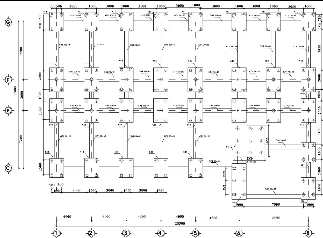
MẶT BẰNG HỒ TRÍ ĐÀI, CỌC
