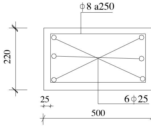
Hình 2.1 :Bố trí thép cột số 07
