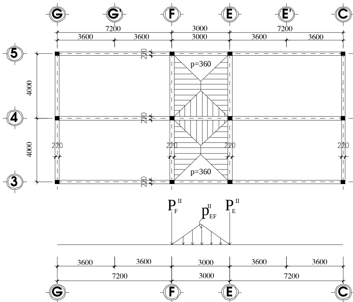
Mặt bằng truyền tải và sơ đồ dồn tải của hoạt tải 2- tầng 2,4,6
