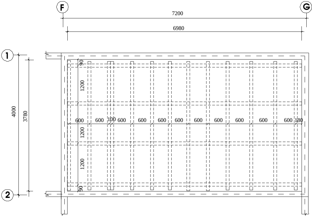
Mặt bằng bố trí xà gồ ô sàn S1
