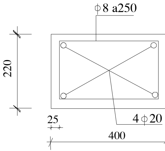
Hình 2.1 :Bố trí thép cột số 07
