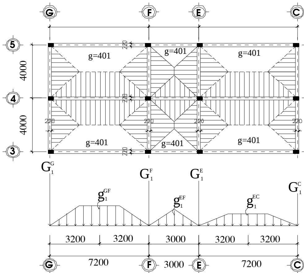
Mặt bằng truyền tải và sơ đồ dồn tải sàn tầng 2,3,4
