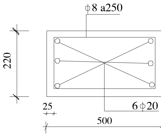
Hình 2.1 :Bố trí thép cột số 01
