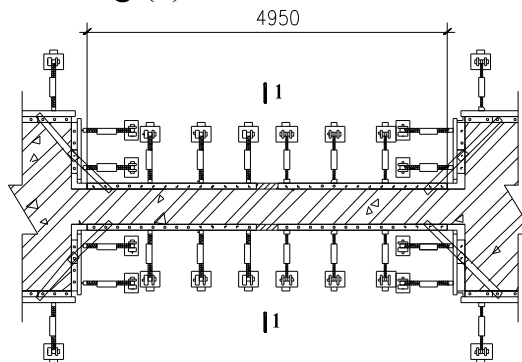
MẶT BẰNG VÁN KHUÔN GIẢNG MÓNG GM1
