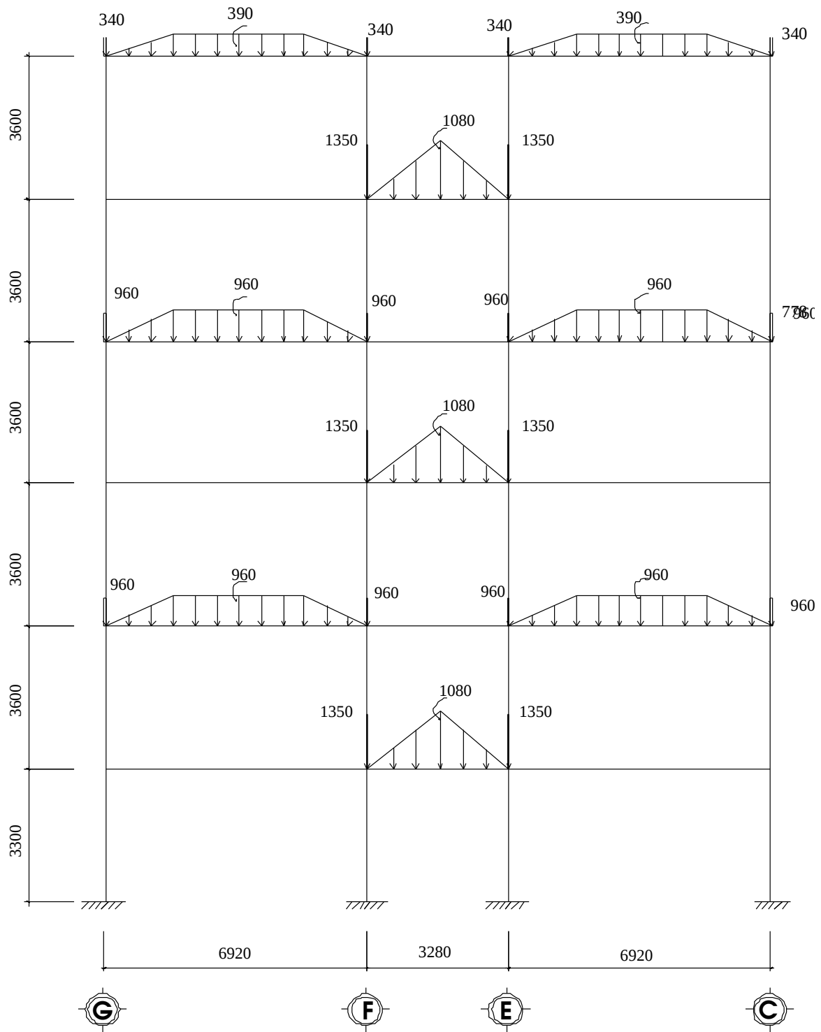
Sơ đồ hoạt tải 2 tác dụng vào khung.
