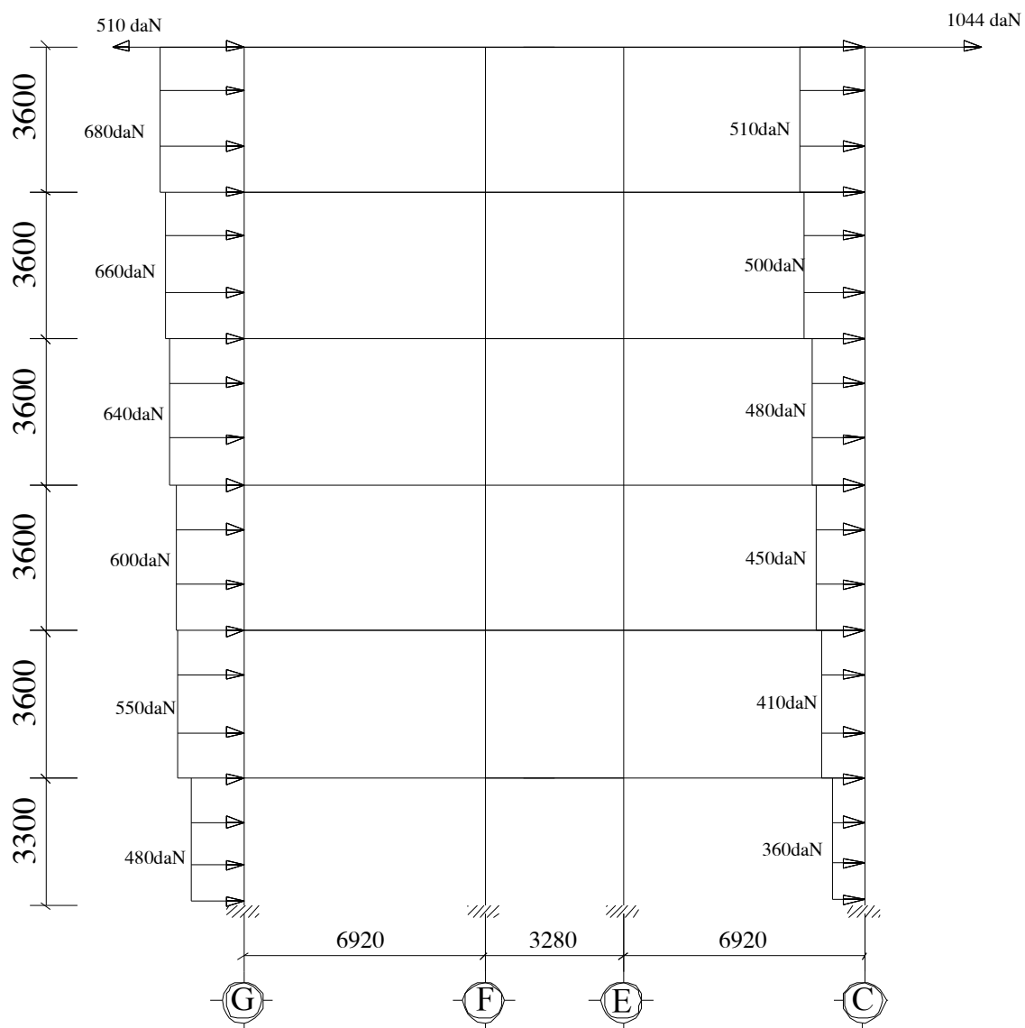
Hình 3.1: Sơ đồ gió trái tác dụng vào khung
