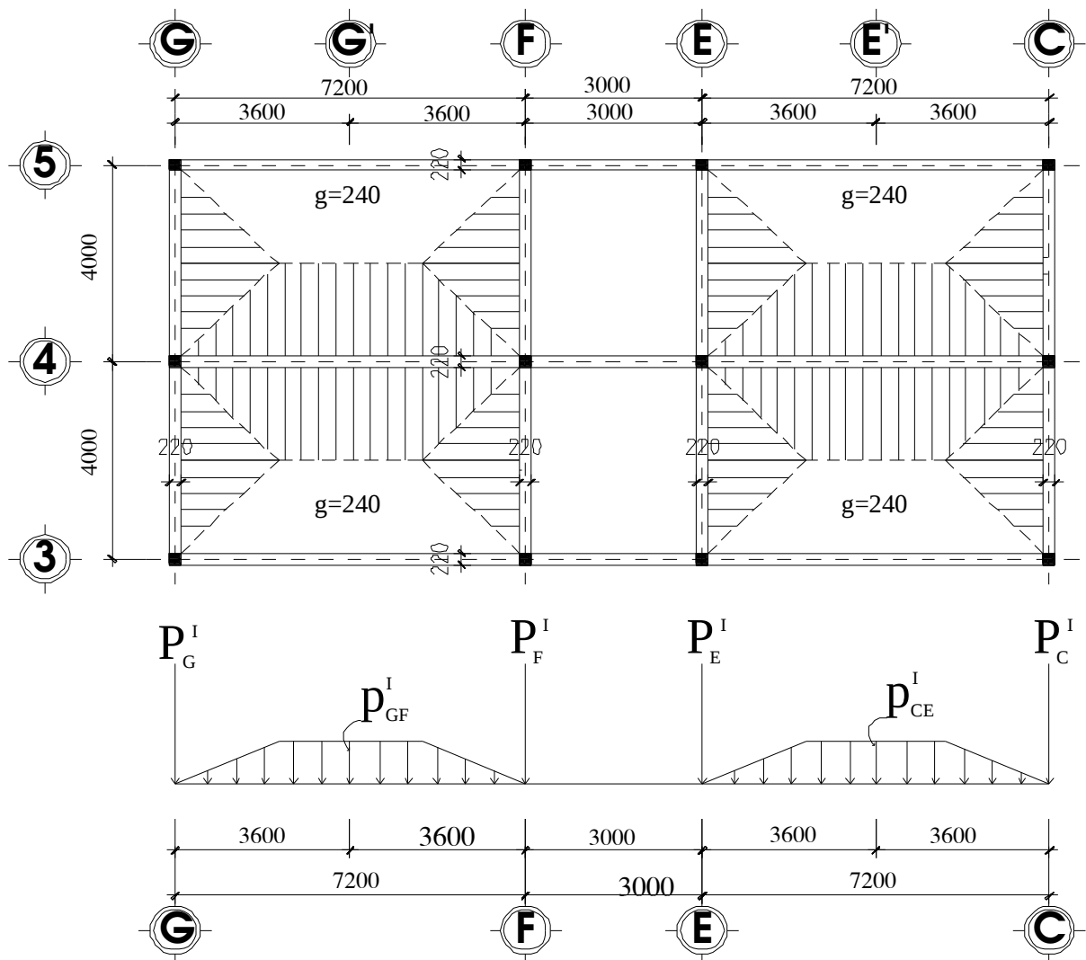
Mặt bằng truyền tải và sơ đồ dồn tải - tầng 2,4,6
