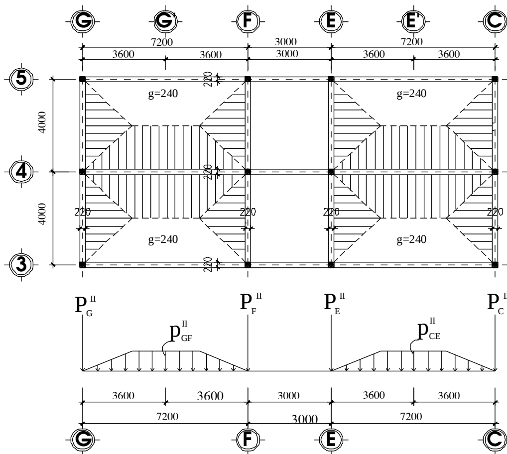
Mặt bằng truyền tải và sơ đồ dồn tải Của hoạt tải 2- tầng 3,5
