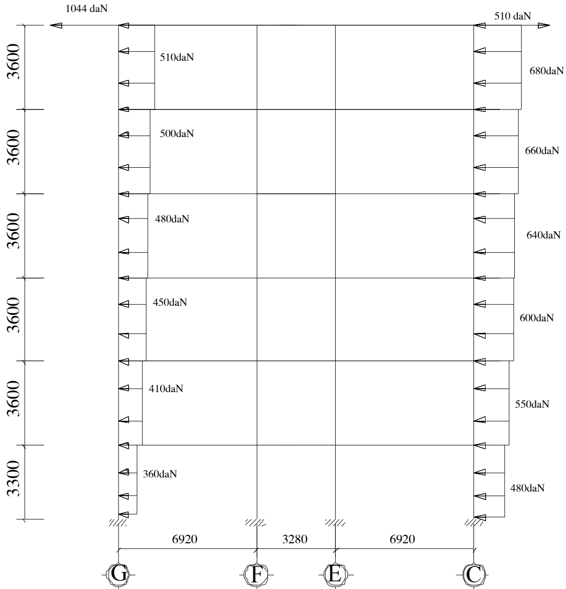
Hình 3.2: Sơ đồ gió phải tác dụng vào khung.
