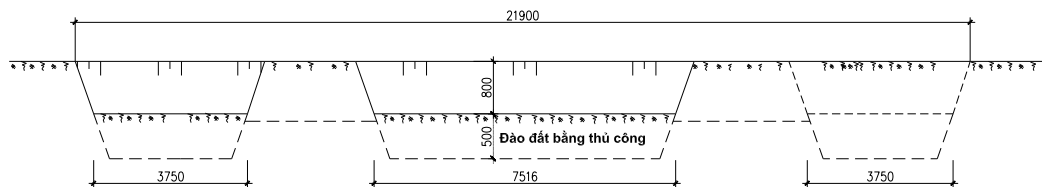
Mặt cắt 2-2
