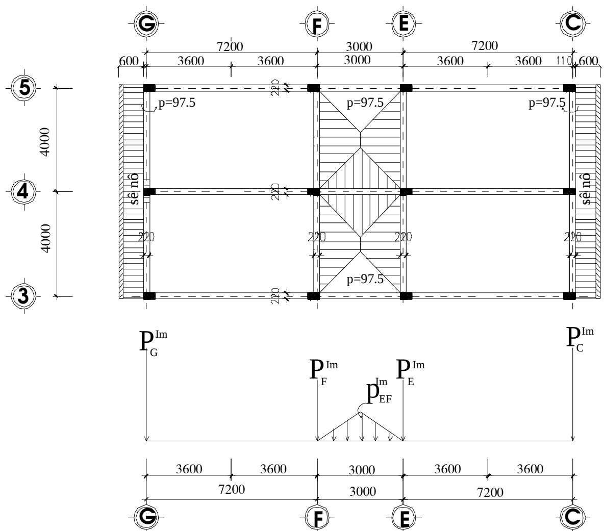
Mặt bằng truyền tải và sơ đồ dồn tải của hoạt tải 1 tầng mái
