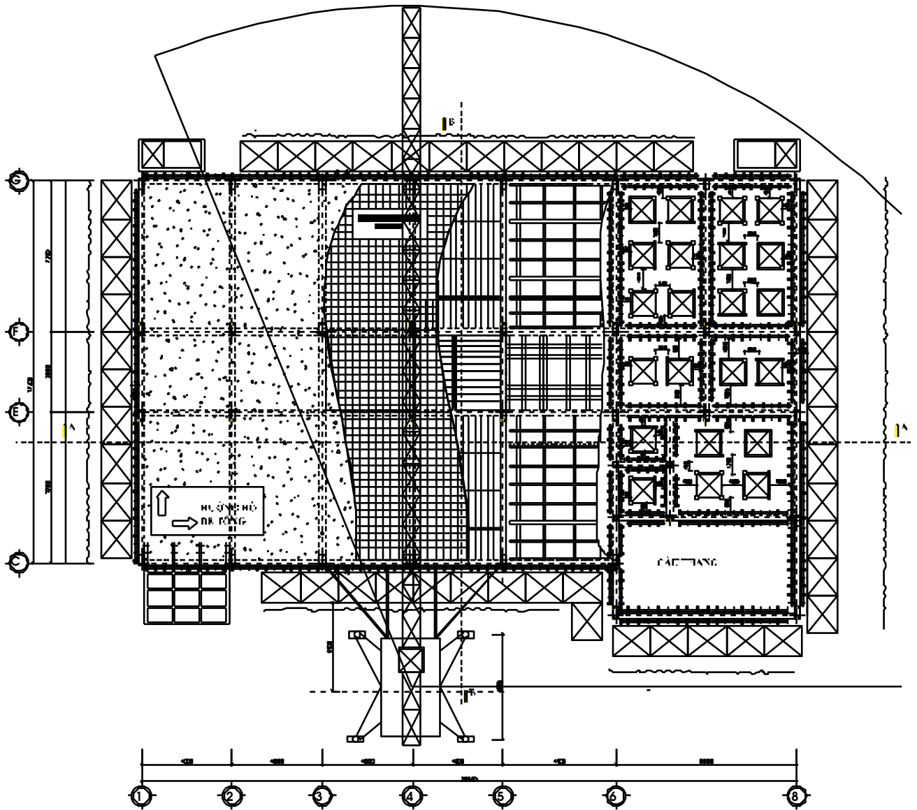
Mặt bằng thi công tầng điển hình.
