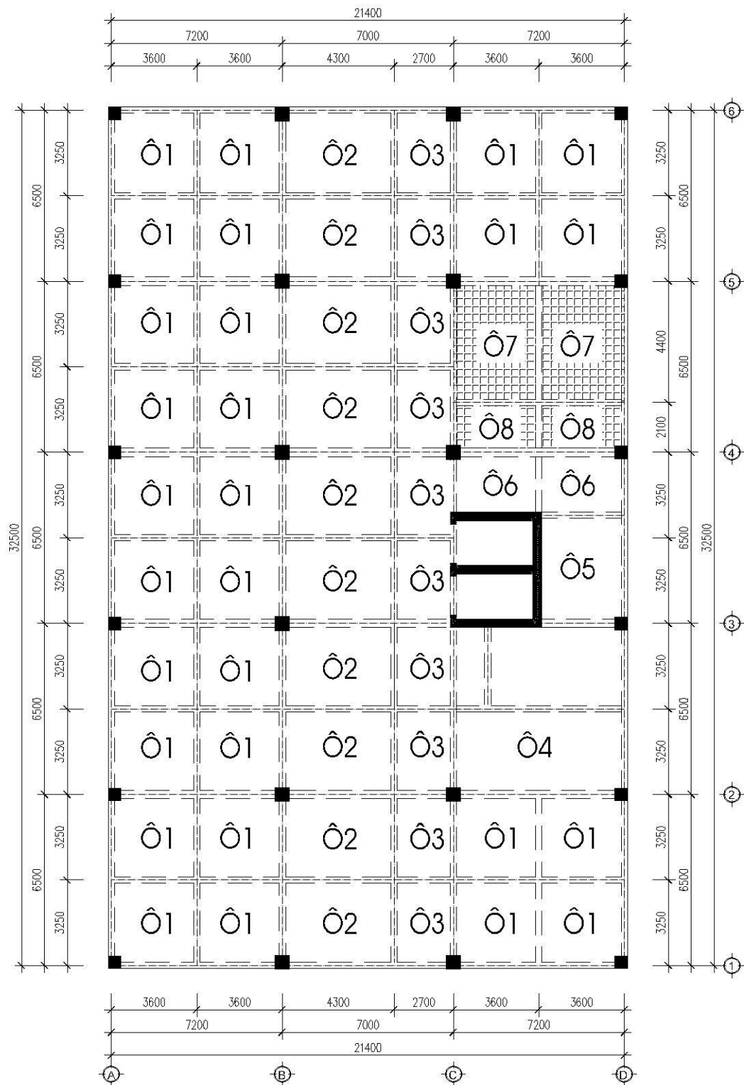
Chia số sàn điển hình
