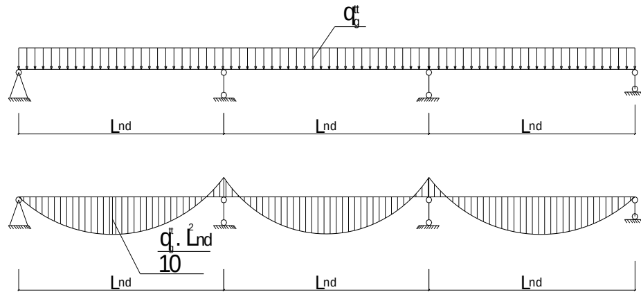
Hình 26: Sơ đồ tính cốp pha giăng móng
