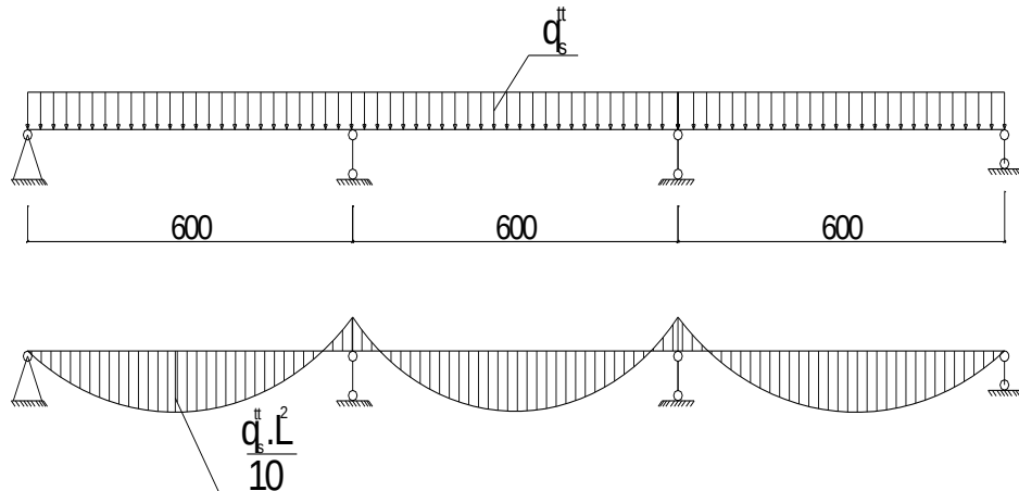
Hình 39: Sơ đồ tính cốp pha sàn
