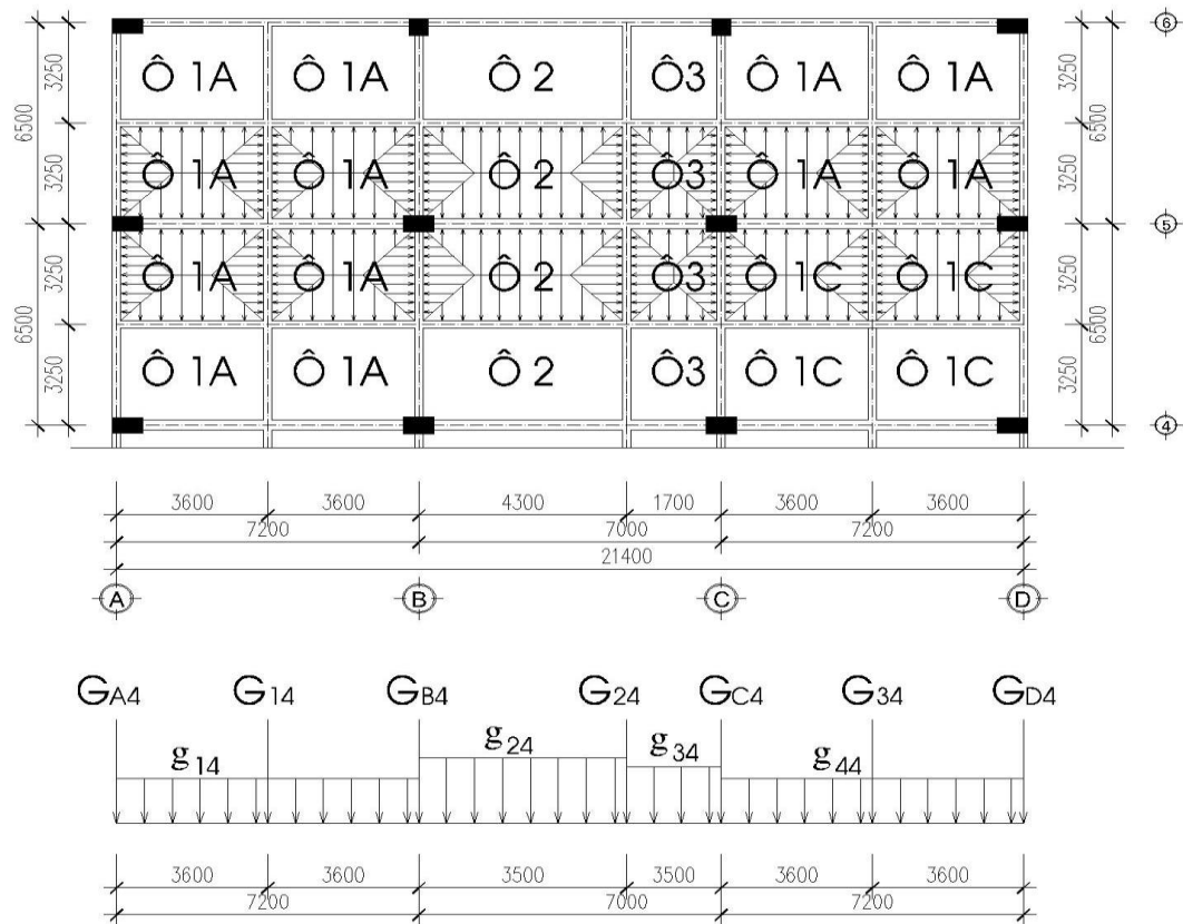
Hình 4: Mặt bằng truyền tải, Sơ đồ chất tải sàn tầng 4,5,6,7
