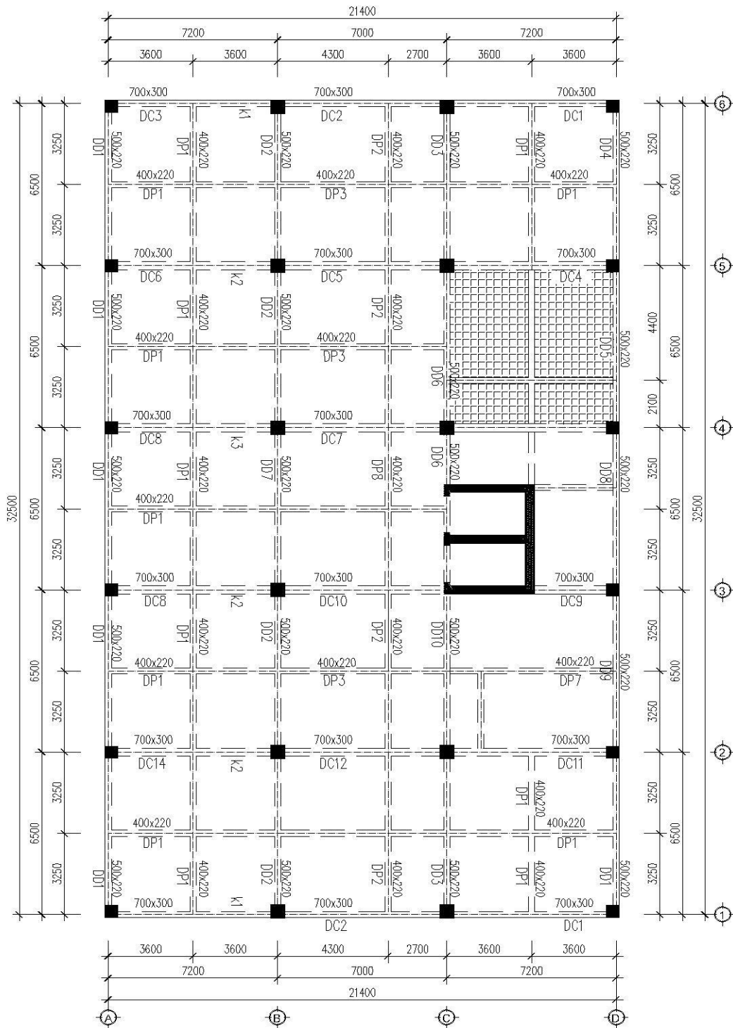
Mặt bằng kết cấu sàn tầng 06
