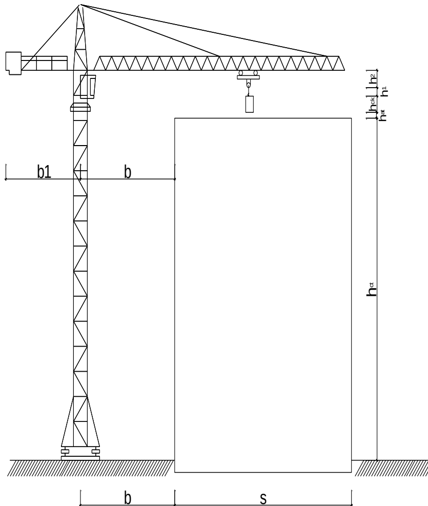
Hình 30: Cần trục tháp KH-504
