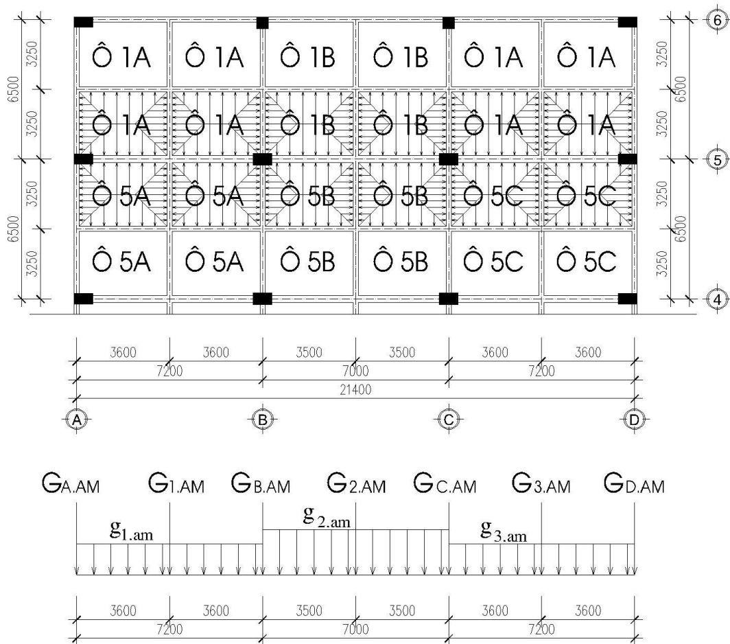
Hình 6: Mặt bằng truyền tải, Sơ đồ chất tải sàn tầng áp mái
