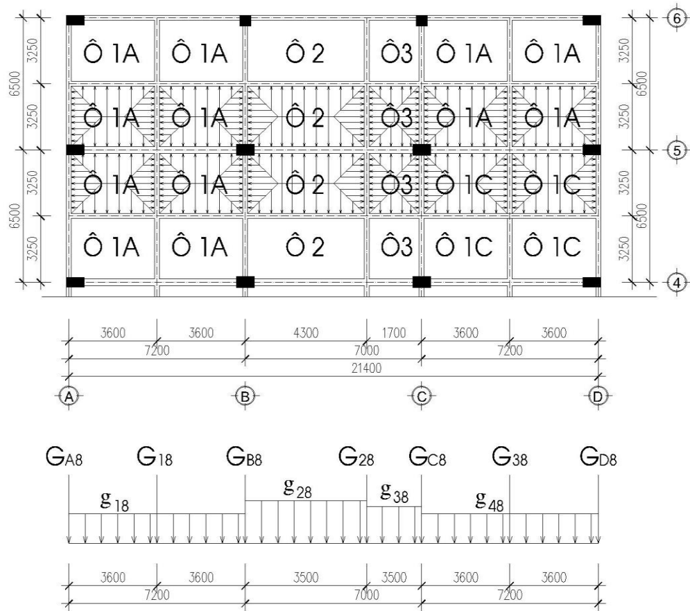
Hình 5: Mặt bằng truyền tải, Sơ đồ chất tải sàn tầng 8,9
