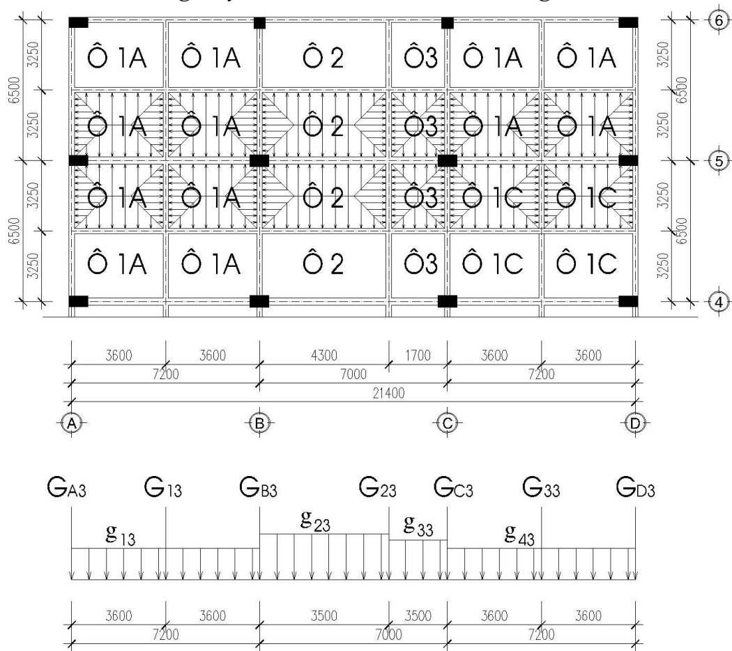
Hình 5: Mặt bằng truyền tải, Sơ đồ chát tải sàn tầng3
