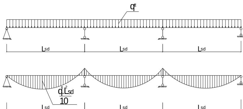
Hình 24: Sơ đồ tính toán sườn ngang đỡ cốp pha móng
