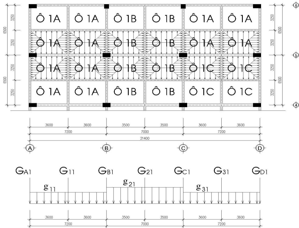
Hình 3: Mặt bằng truyền tải, Sơ đồ chát tải sàn tầng 1
