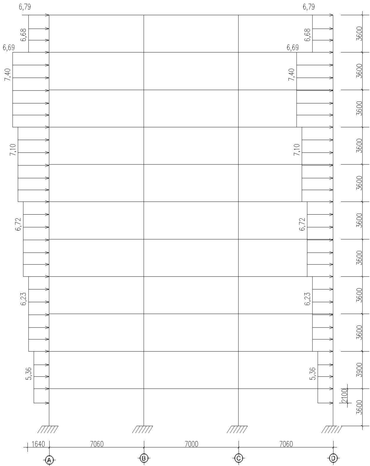
SƠ ĐỒ GIÓ TRÁI TÁC DỤNG VÀO KHUNG TRỤC 2
