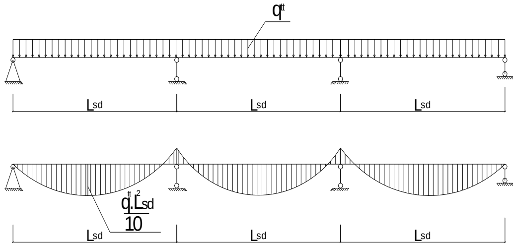
Hình 35: Sơ đồ tính cốp pha thành dầm
