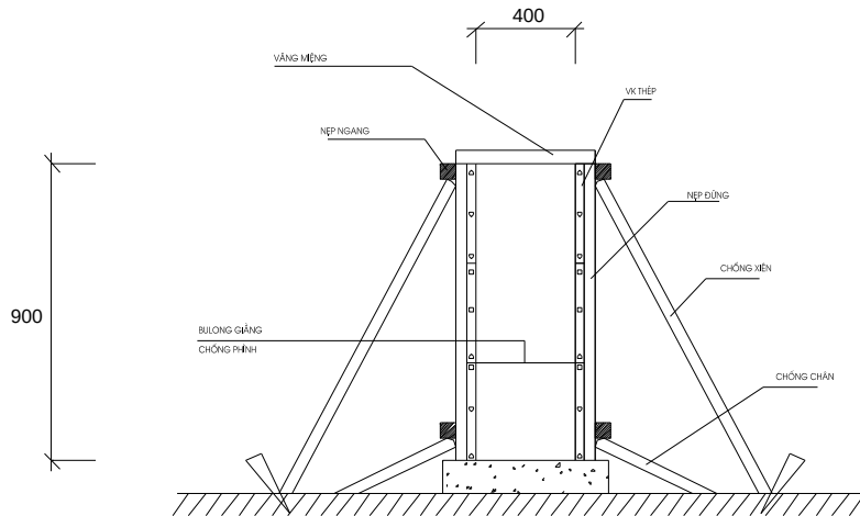
Hình 25: Cấu tạo ván khuôn giăng
