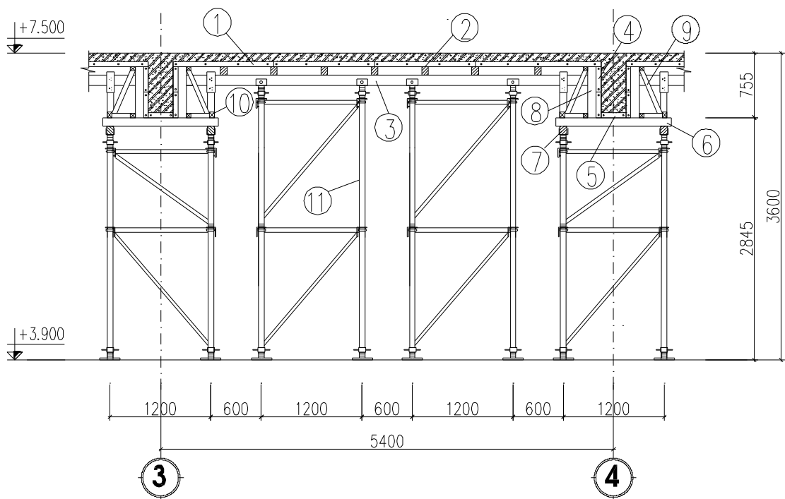
MẶT CẮT 3 - 3
