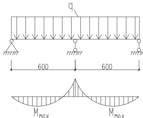
SƠ ĐỒ TÍNH VÁN KHUÔN THÀNH DẦM
