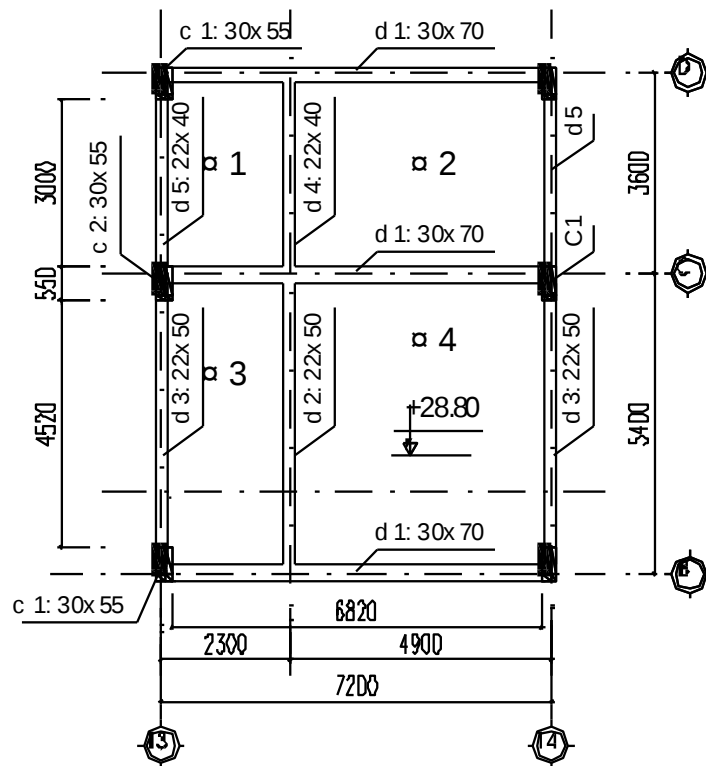
mặt bằng khung cột tầng lầu
