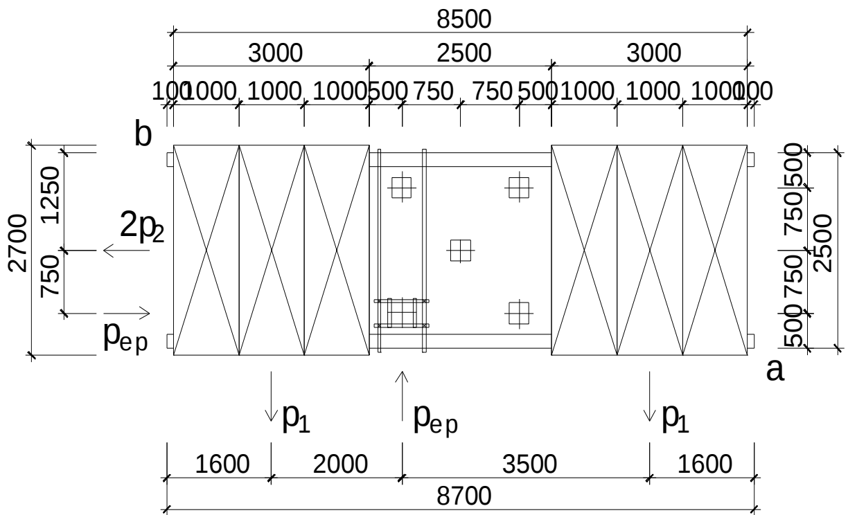
SƠ ĐỒ TÍNH TOÁN ĐỐI TRỌNG
