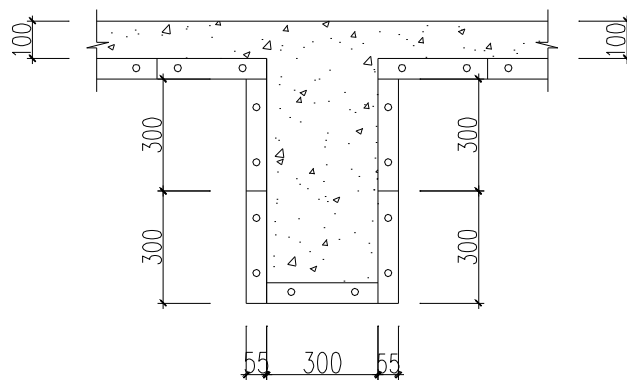
MẶT CẮT VÁN KHUÔM DẦM CHÍNH
