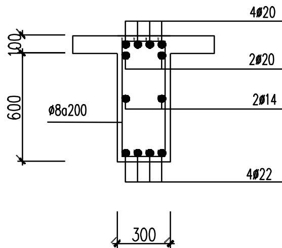
BỐ TRÍ CỐT THÉP CHO DẦM D66
