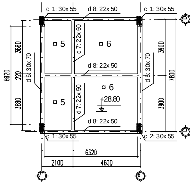
mặt bằng khung cột tầng trệt
