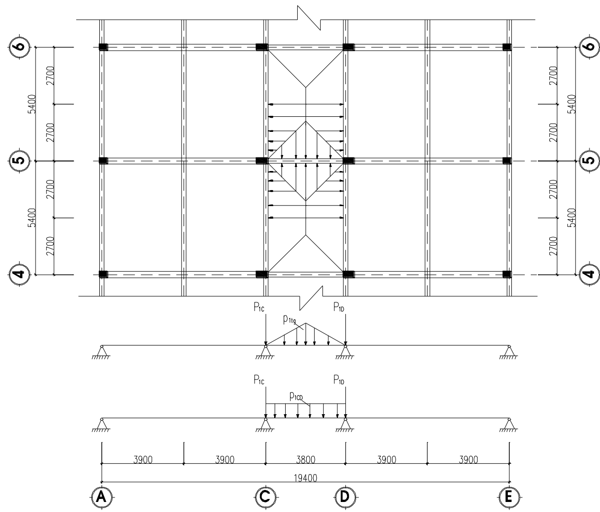
SƠ ĐỒ PHÂN HOẠT TẢI 1- TẦNG 2, 4
