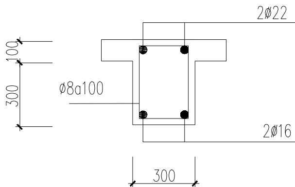
BỐ TRÍ CỐT THÉP CHO DẦM D78
