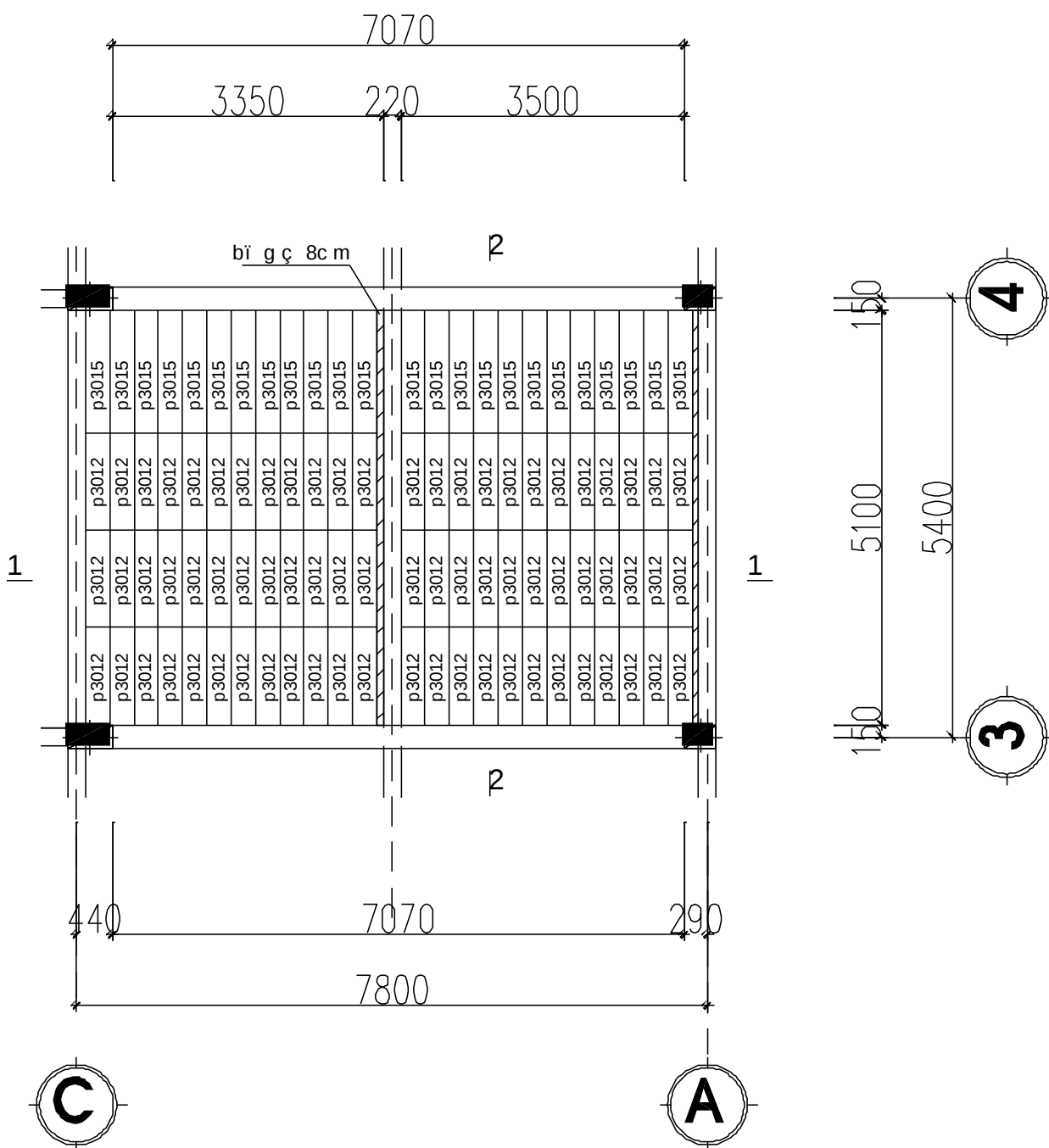
TỔ HỢP VÁN KHUÔN Ô SÀN ĐIỆN HÌNH
