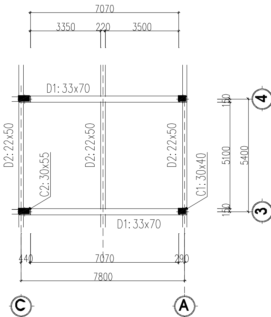
MẶT BẰNG Ô SÀN ĐIỂN HÌNH
