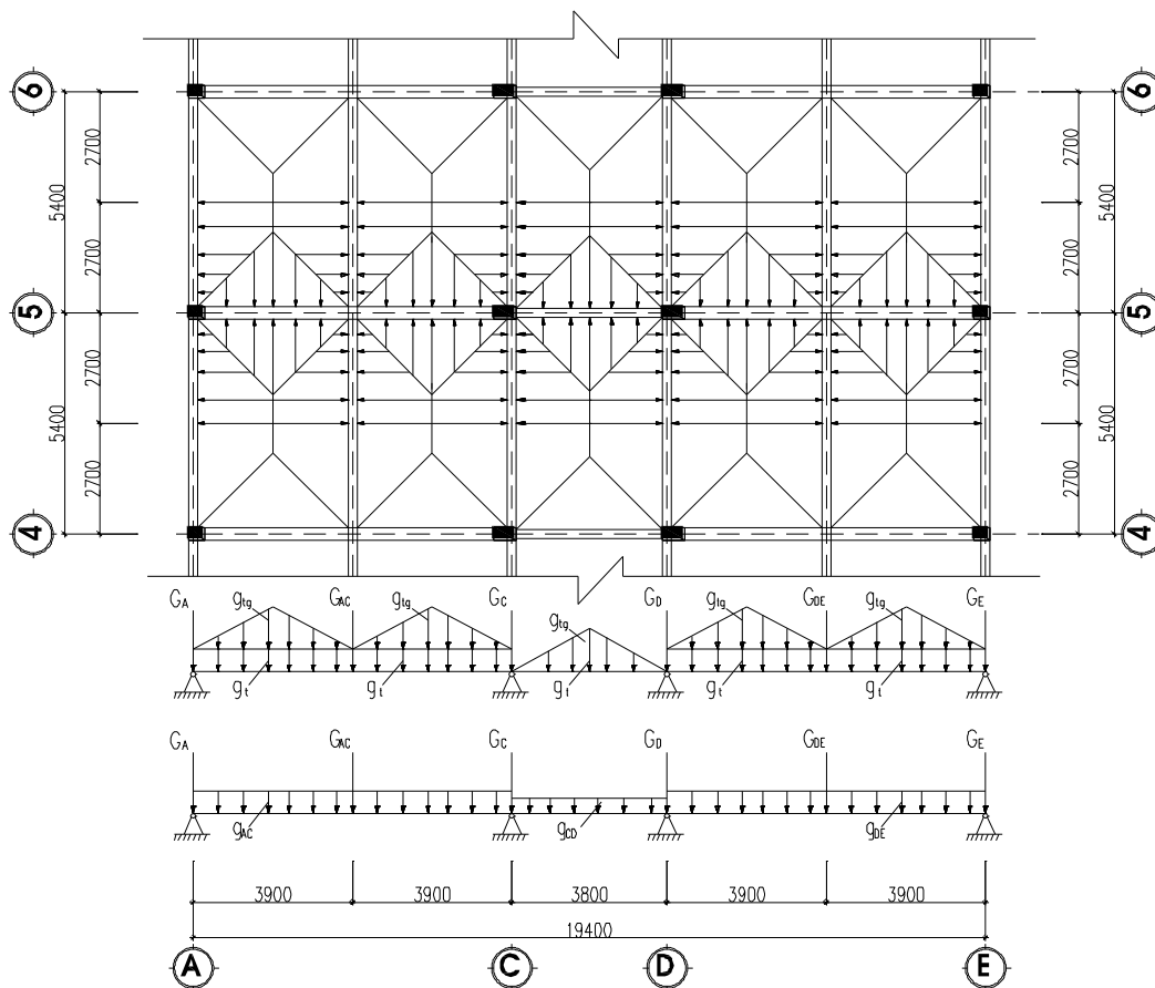
MẶT BẰNG PHÂN TẢI DO TÍNH TẢI TẦNG 2,3,4,5
