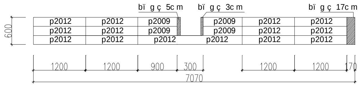
Tổ hợp ván khuôn thành dầm chính D1 (30x70) phía có dầm phụ
