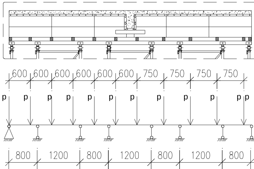
SƠ ĐỒ TÍNH XÀ DỌC ĐỒ XÀ NGANG
