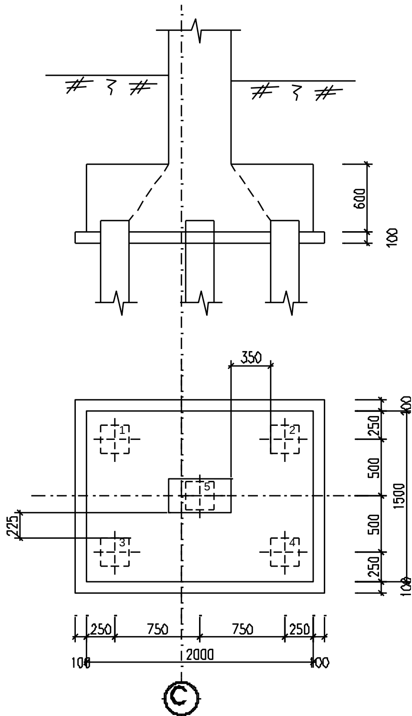
Sơ đồ xác định khối móng khối móng chọc thủng
