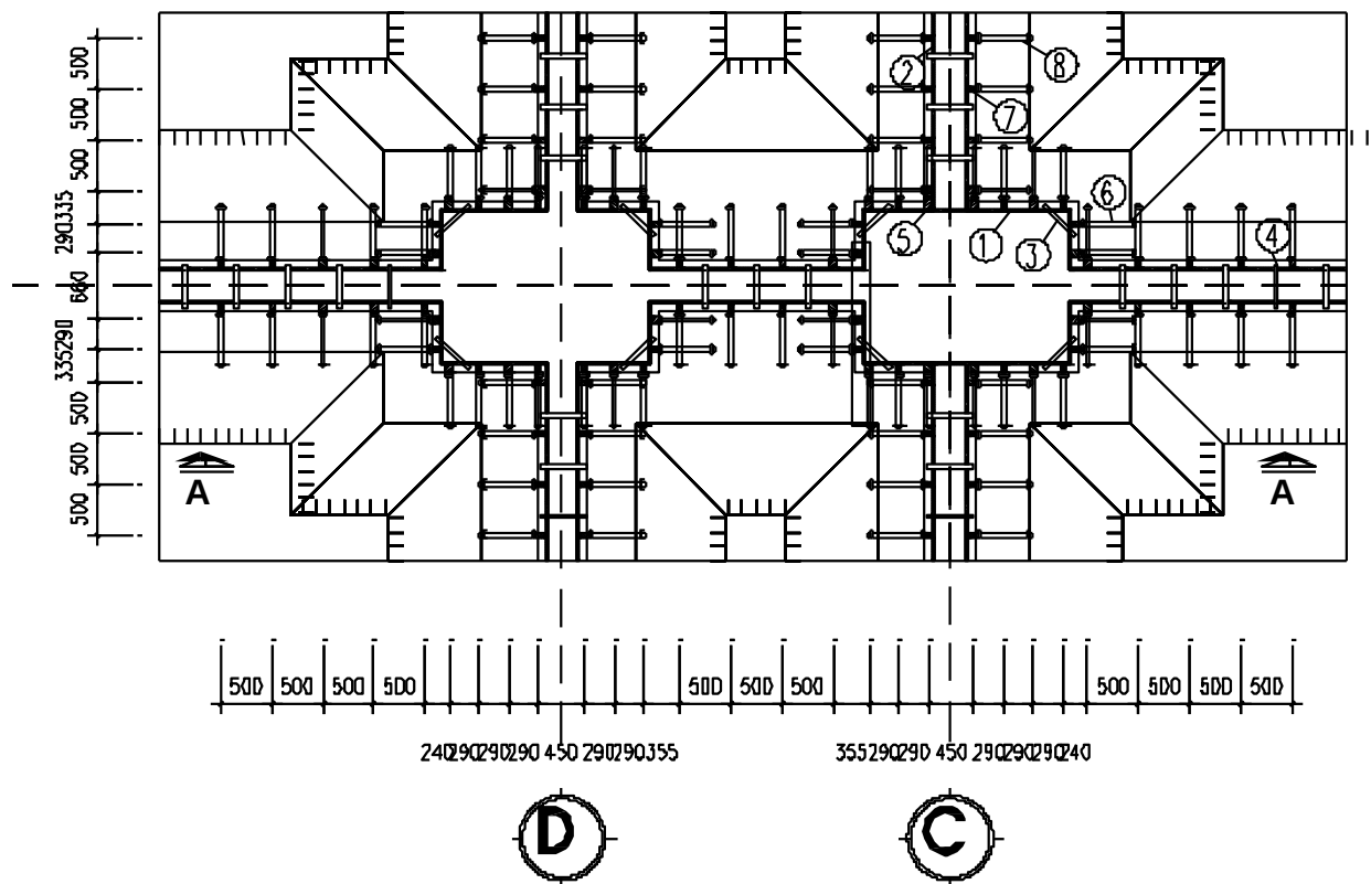
MẶT BẰNG HỒ MÓNG TRỤC C - D
