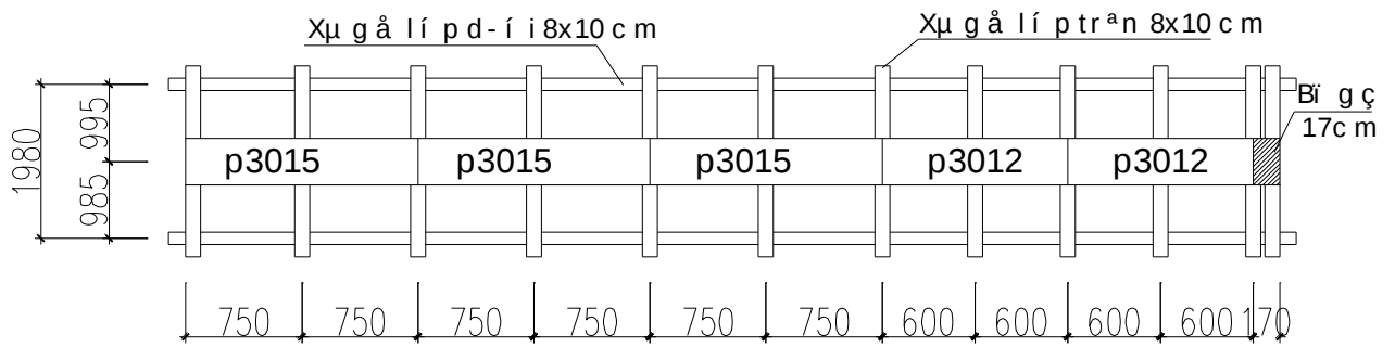
Tổ hợp ván khuôn đáy dầm chính D1 (30x70)
