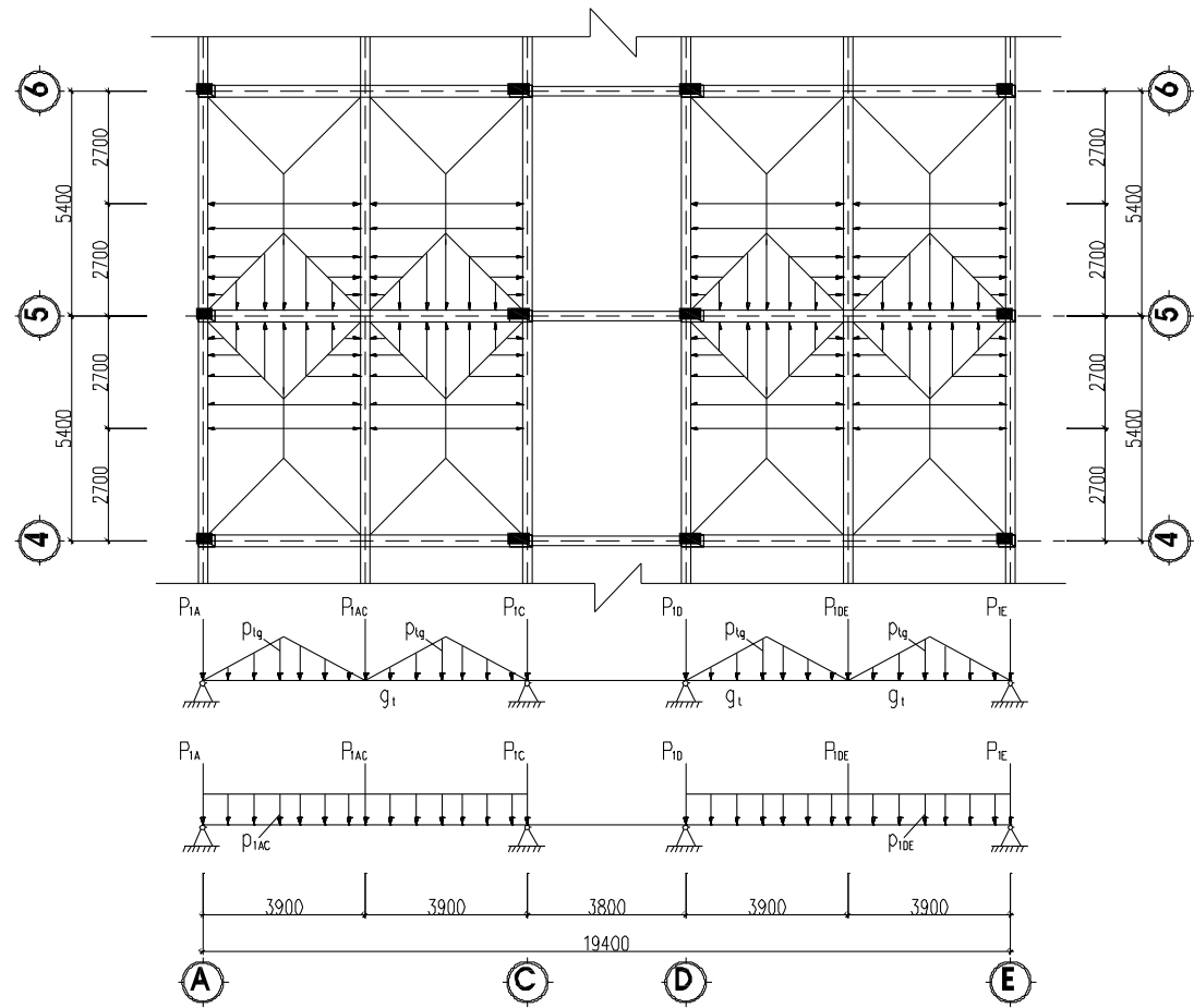
SƠ ĐỒ PHÂN BỐ HOẠT TẢI 1- TẦNG 3, 5
