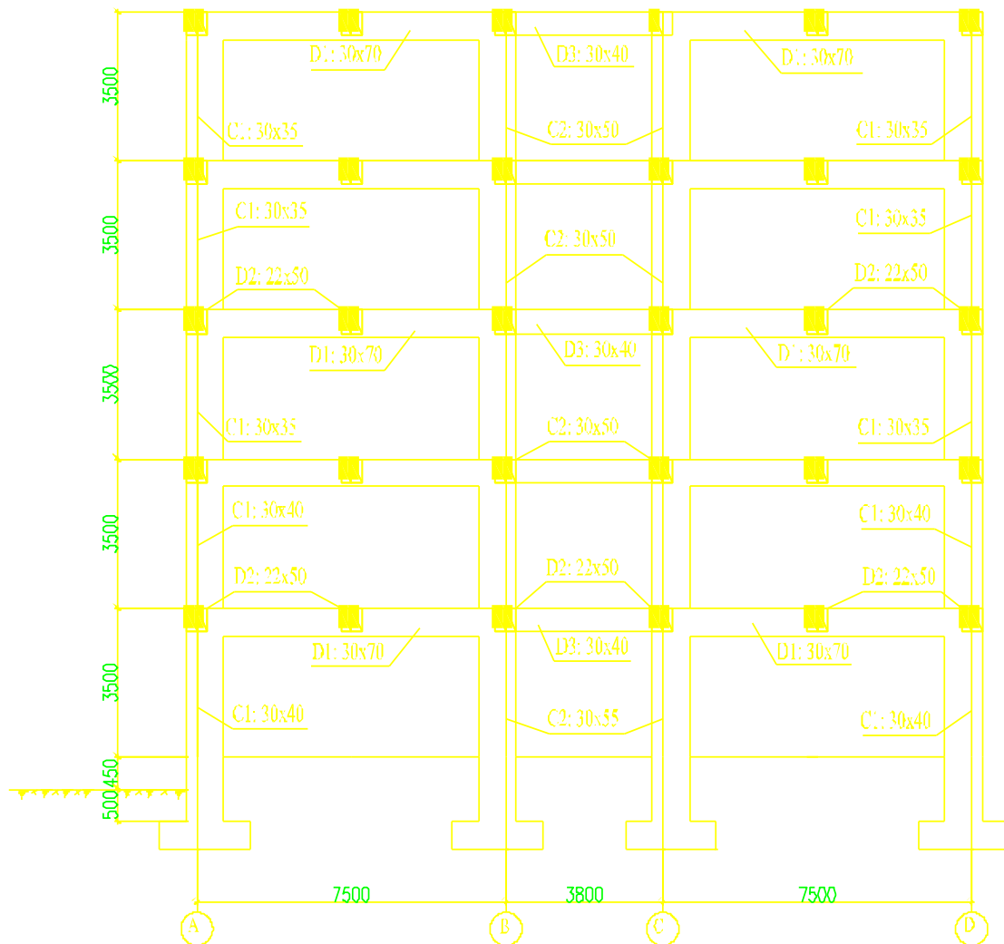
SƠ ĐỒ HÌNH HỌC KHUNG NGANG
