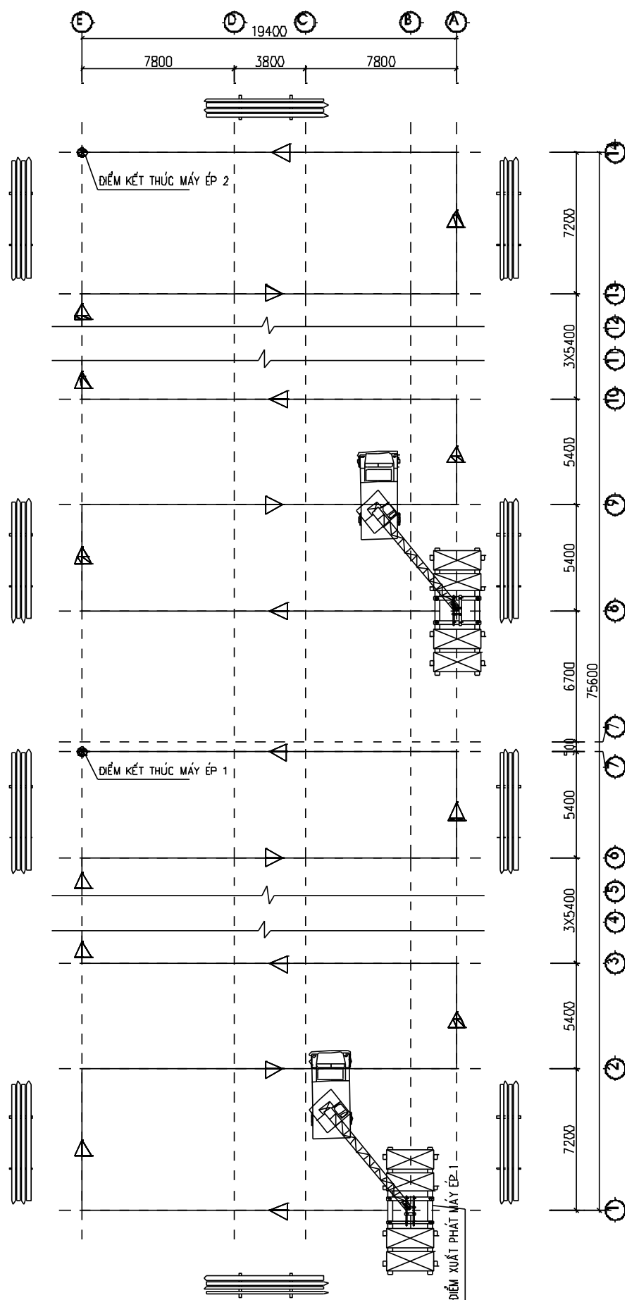
SƠ ĐỒ DI CHUYỂN THI CÔNG ÉP CỌC
