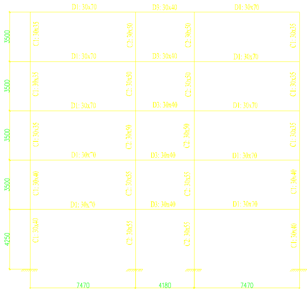
SƠ ĐỒ KẾT CẤU KHUNG NGANG
