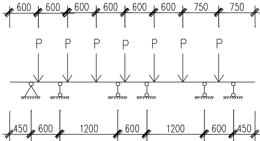
SƠ ĐỒ TÍNH XÀ GỒ LỚP DƯỚI CỦA SÀN
