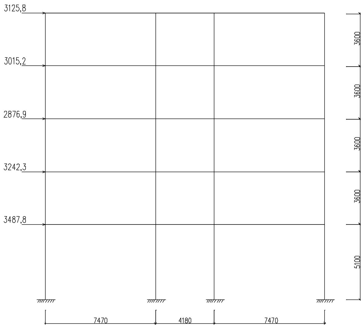
SƠ ĐỒ GIÓ TRÁI TÁC DỤNG VÀO KHUNG TRỤC 5
