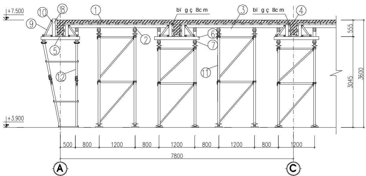
MẶT CẮT 2 - 2
