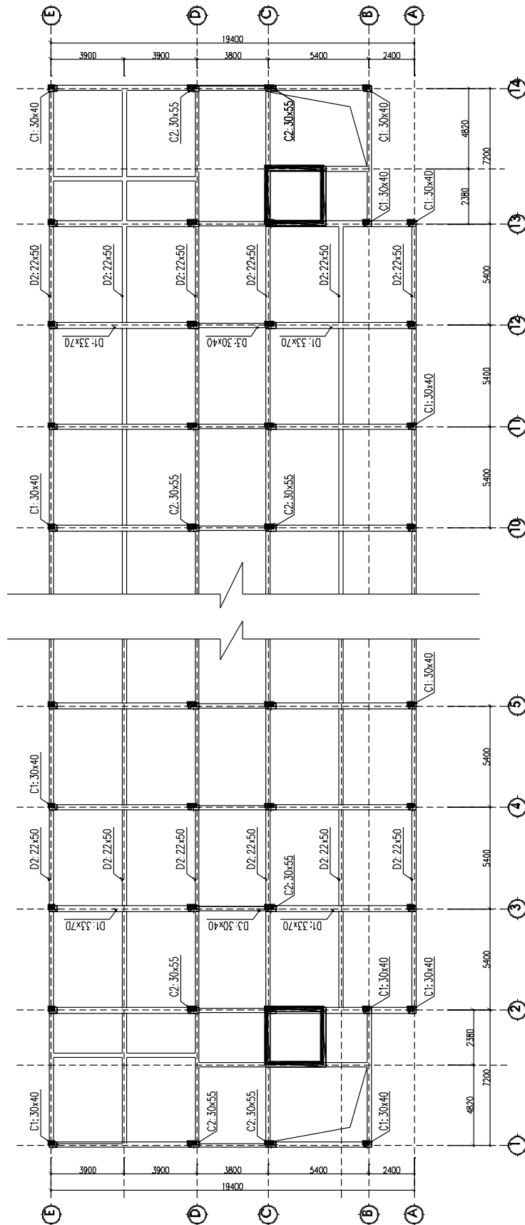
MẶT BẰNG KẾT CẤU ĐIỂN HÌNH
