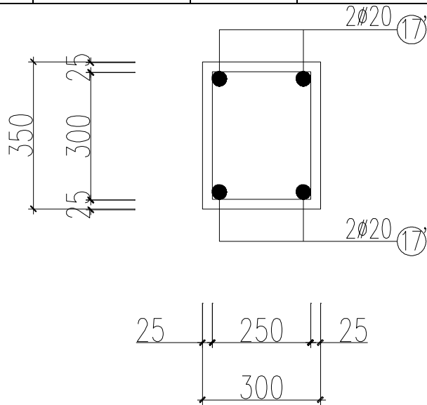
BỐ TRÍ CỐT THÉP TRONG CỘT BIÊN C1: 30X35
