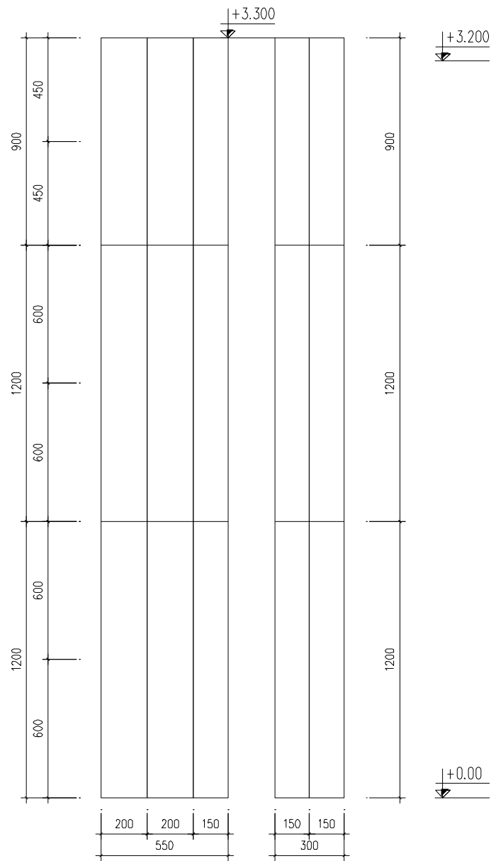
Tổ hợp ván khuôn cột giữa tầng 1: 300x550x3200 (mm)
