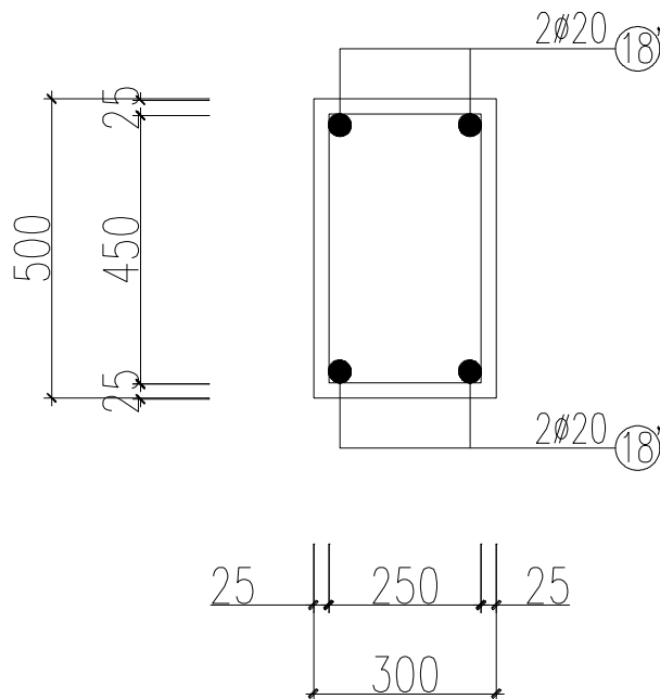
BỐ TRÍ CỐT THÉP TRONG CỘT C2: 30X50
