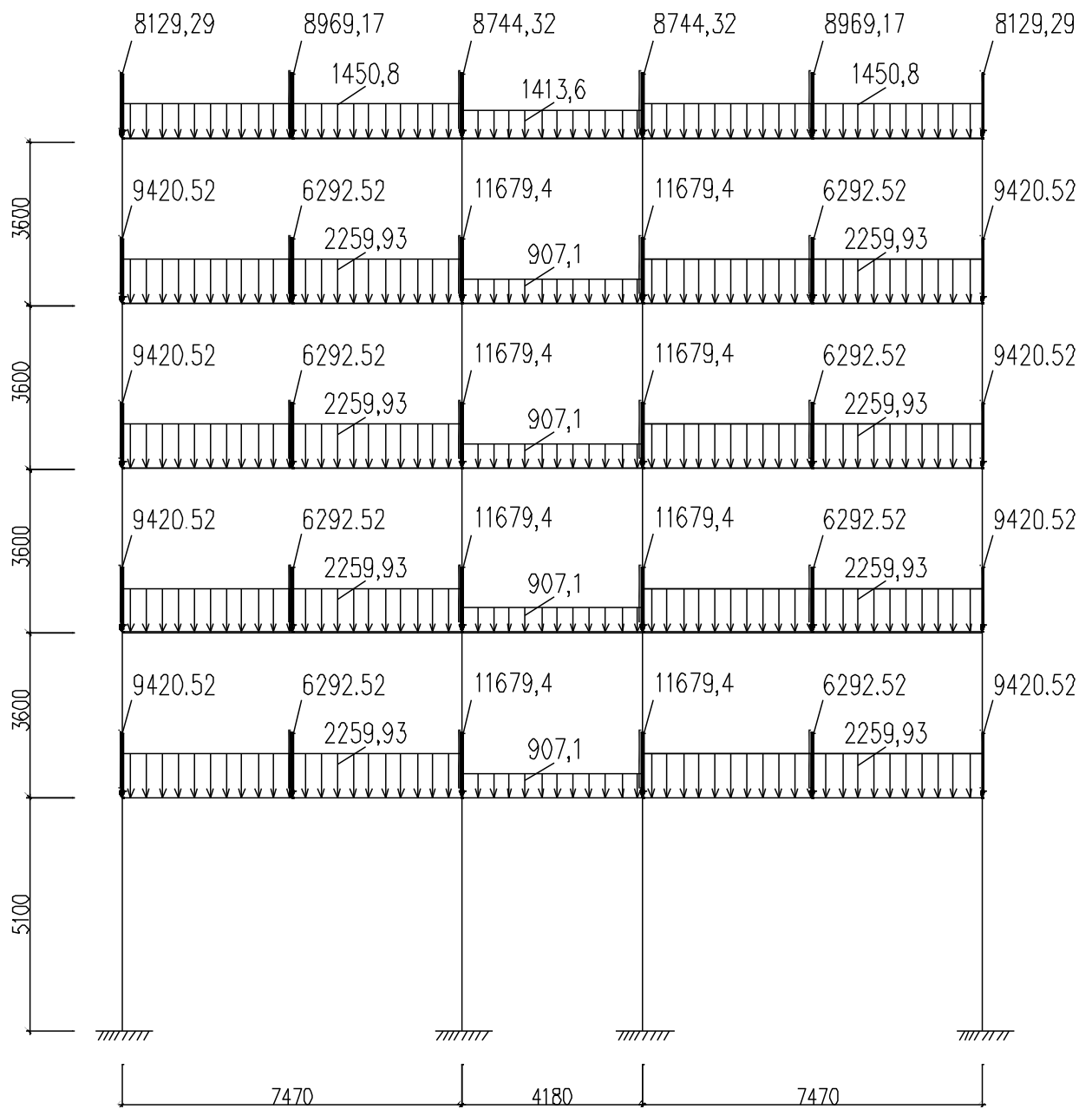
SƠ ĐỒ TÍNH TẢI TÁC DỤNG VÀO KHUNG
