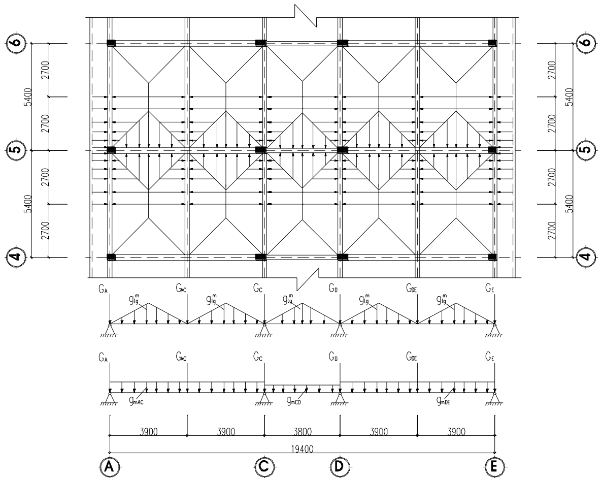
SƠ ĐỒ PHÂN BỐ TỈNH TẢI TẦNG MÁI
