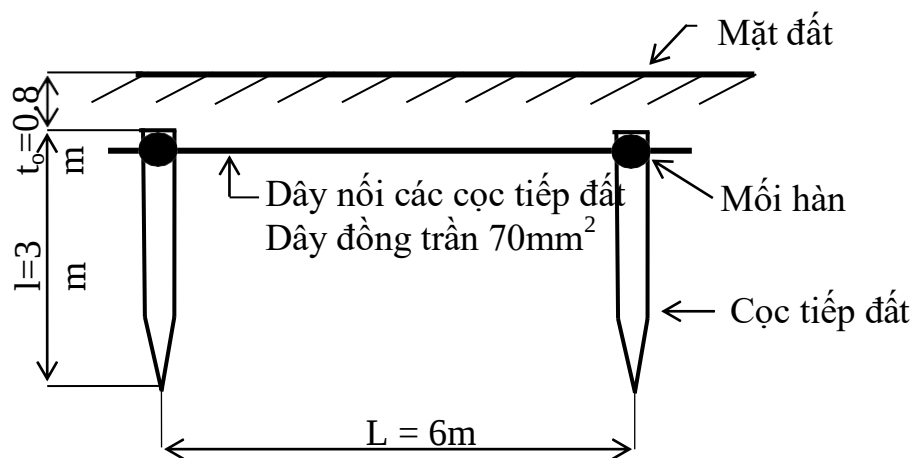
Hình 4.4: Hệ thống nối đất chống sét
