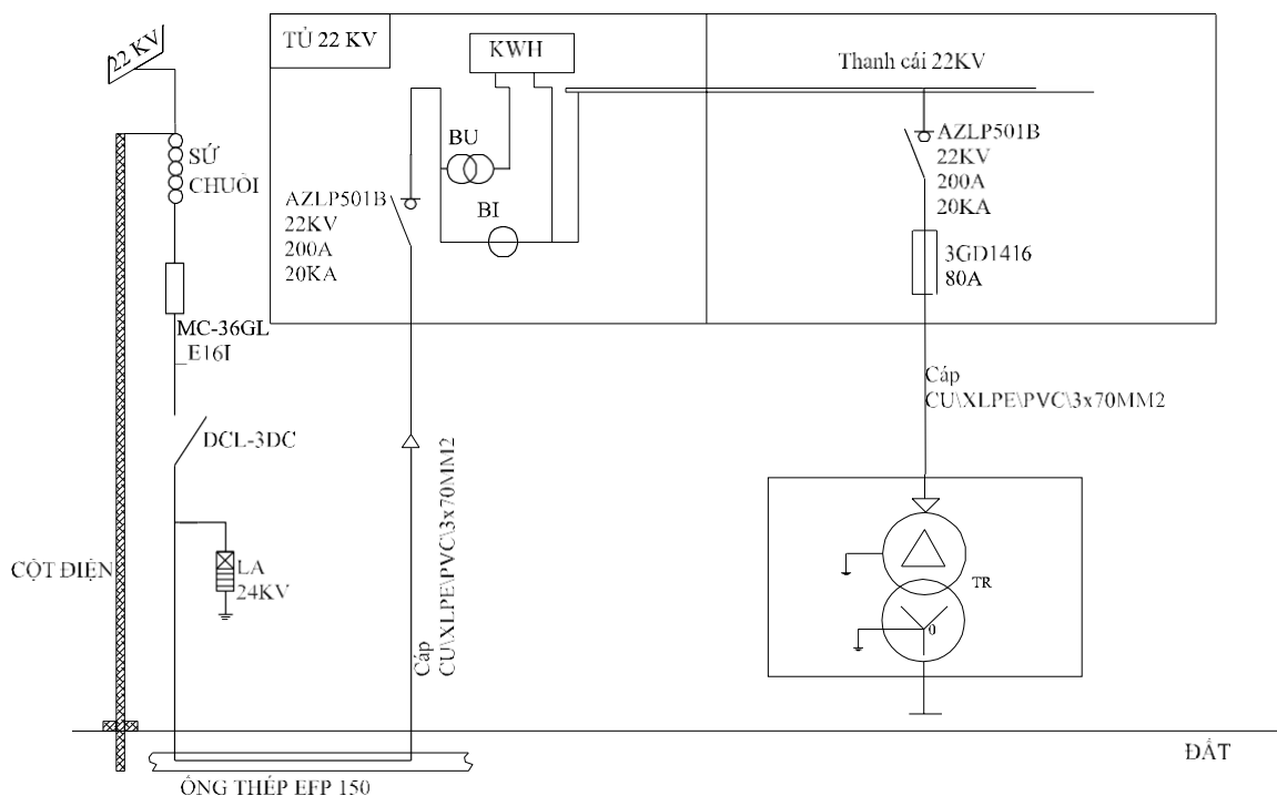
Hình 2.2. Sơ đồ mạng cao áp tòa nhà 7 tầng
