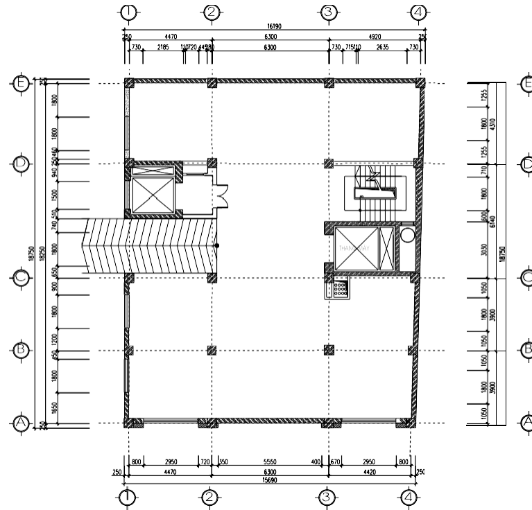
Hình 4.1: Mặt bằng diện tích của tòa nhà 7 tầng
