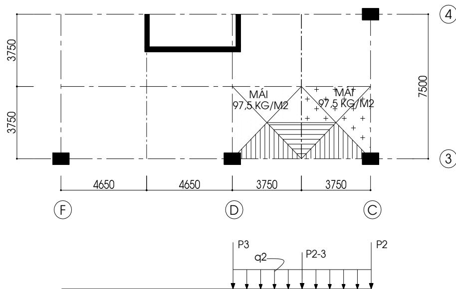
Hình 3.11: Sơ đồ phân hoạt tải 1 – mái
