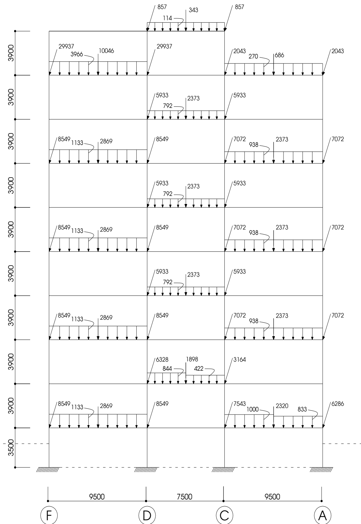
Hình 3.13: Sơ đồ hoạt tải 1 tác dụng vào khung K3
