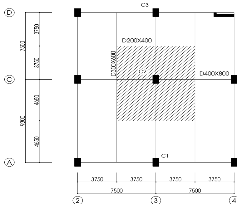
Hình 1.2: Mặt bằng diện truyền tải của cột C2
