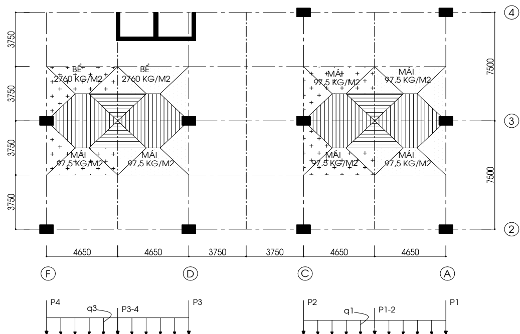
Hình 3.10: Sơ đồ phân hoạt tải 1 – tầng mái
