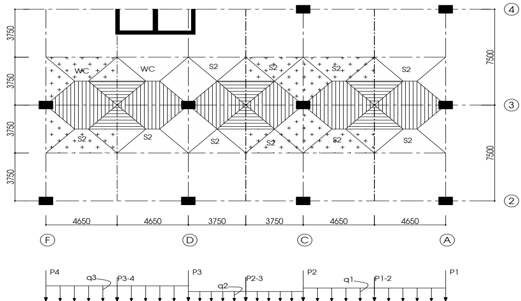
Hình 3.3: Sơ đồ phân tải tầng 3-8
