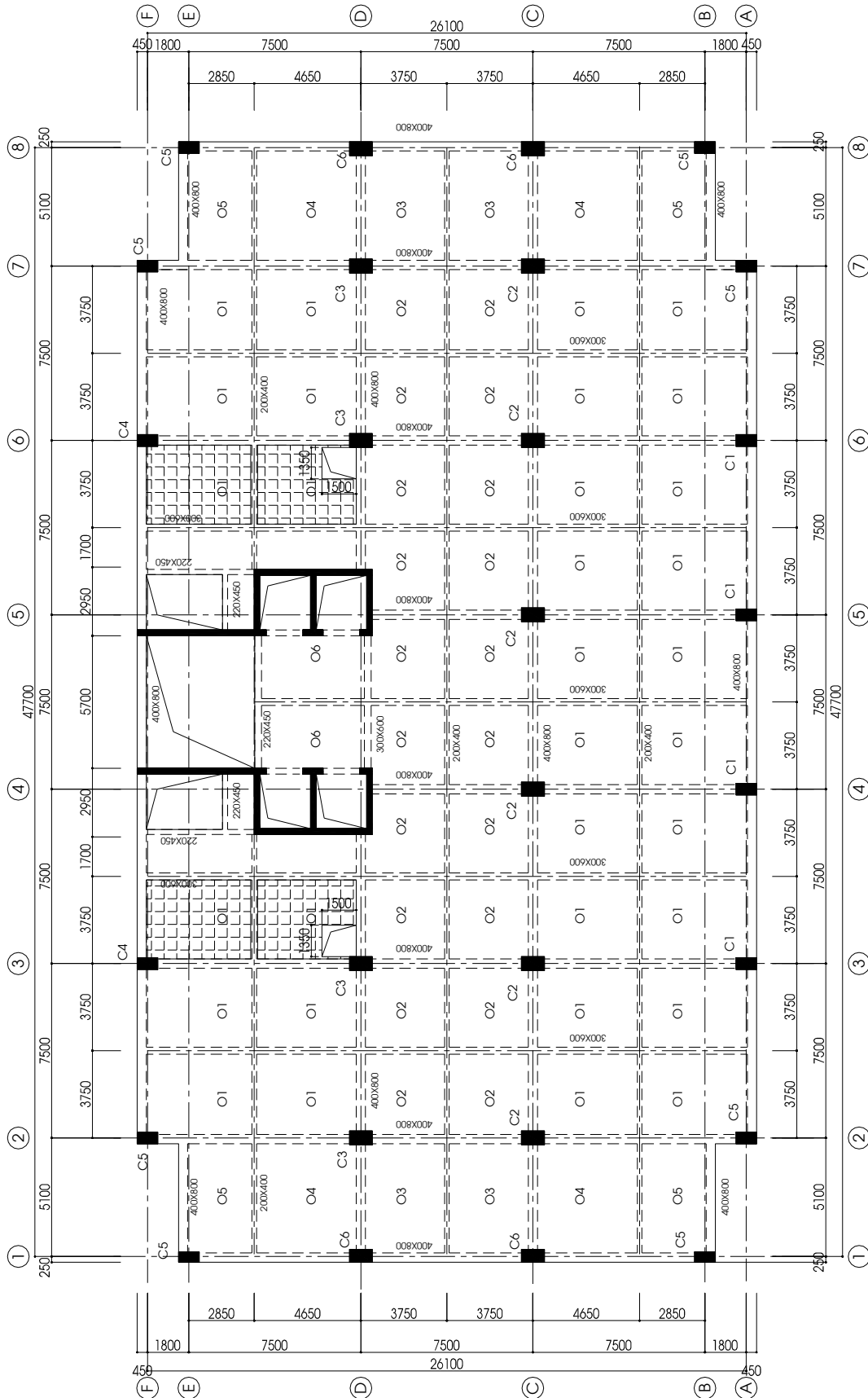
MẶT BẰNG KẾT CẤU SÀN TẦNG ĐIỂN HÌNH
