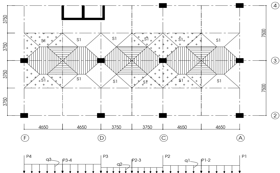
Hình 3.1: Sơ đồ phân tích tải tầng 1
