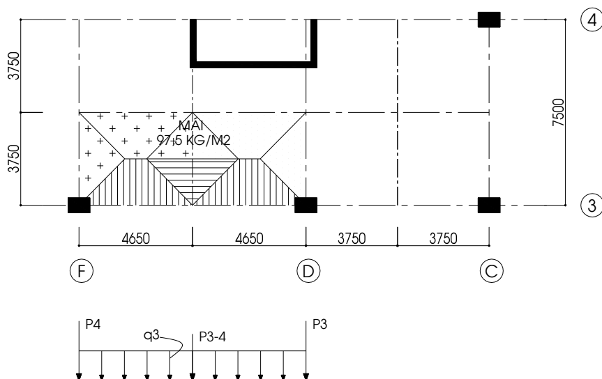
Hình 28: Sơ đồ phân hoạt tải 2 – mái
