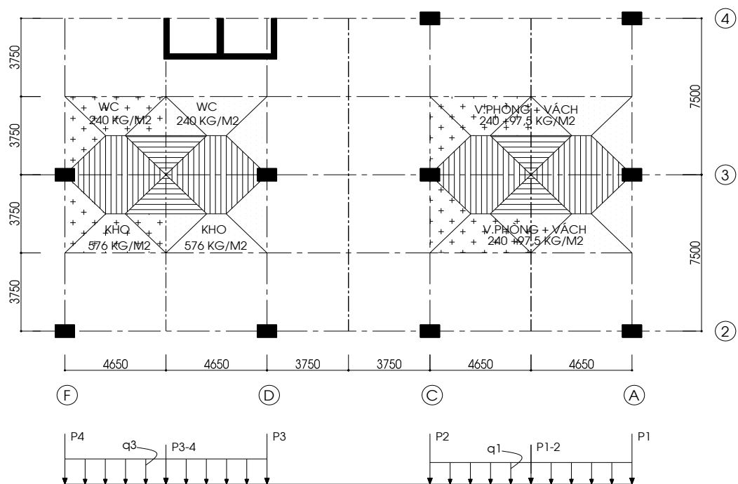
Hình 26: Sơ đồ phân hoạt tải 2 – tầng 4-6-8
