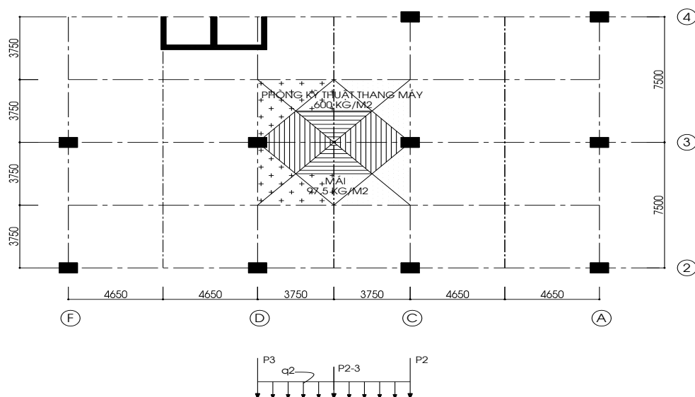
Hình 27: Sơ đồ phân phối tải 2 – tầng mái
