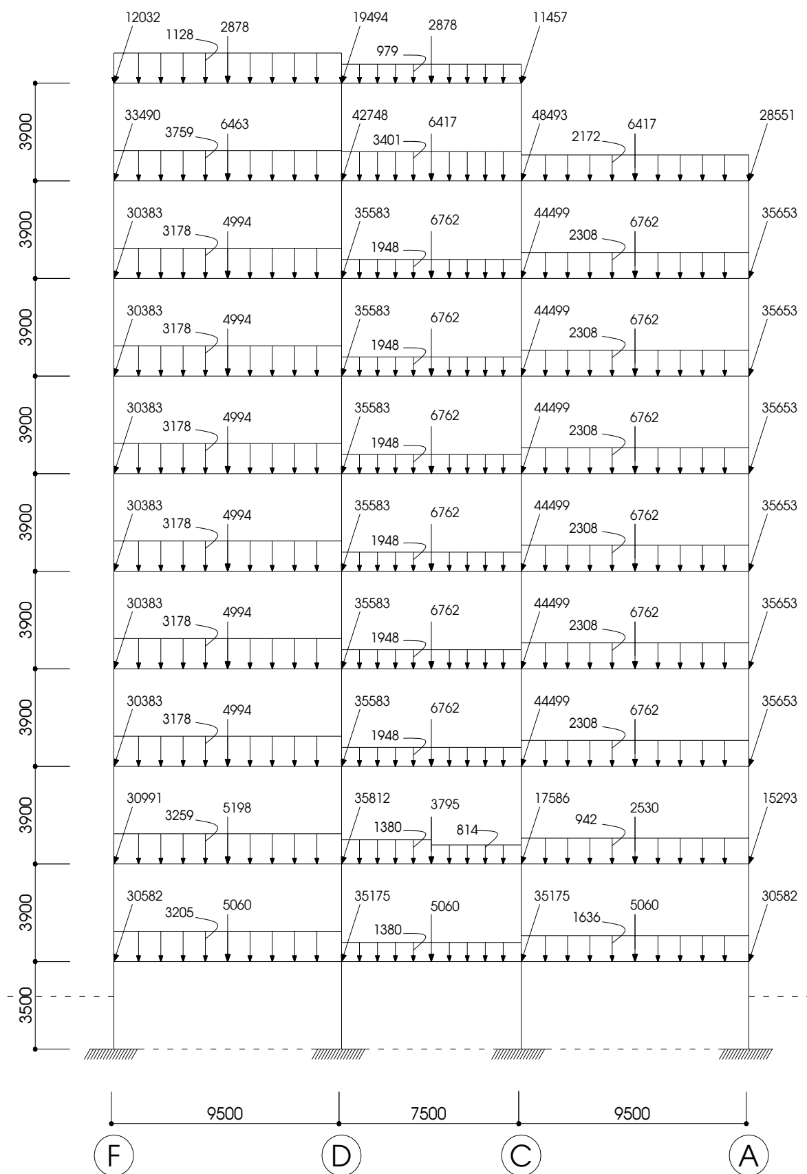
Hình 3.12: Sơ đồ tĩnh tải tác dụng vào khung K3
