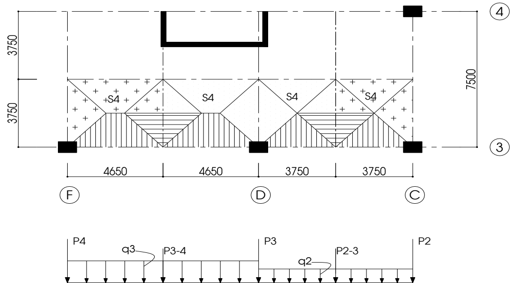
Hình 3.5: Sơ đồ phân tính tải mái.
