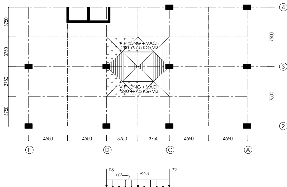
Hình 3.9: Sơ đồ phân hoạt tải 1 – tầng 4-6-8
