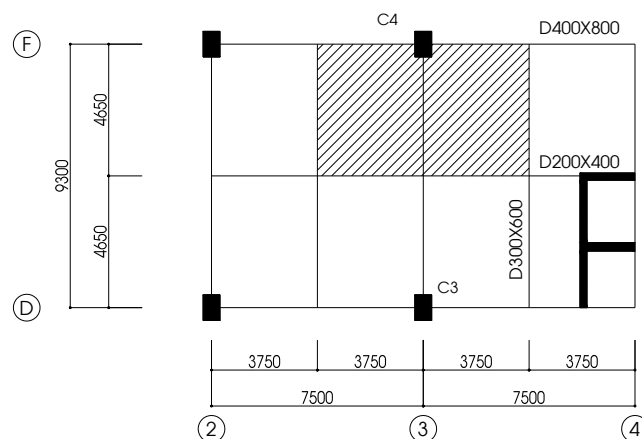
Hình 1.4: Mặt bằng diện truyền tải của cột C4
