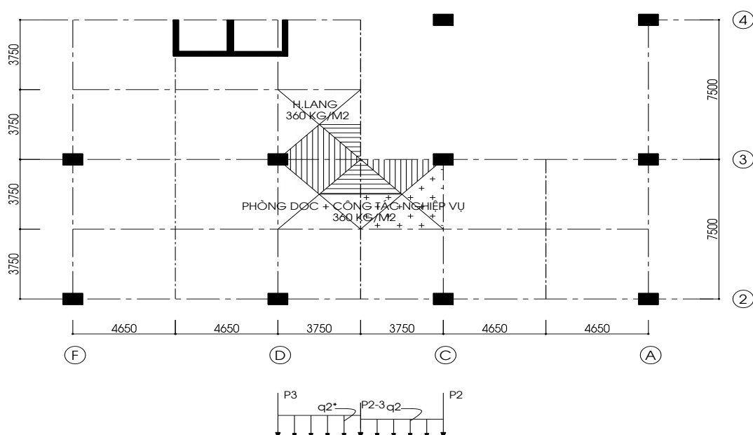
Hình 3.7: Sơ đồ phân hoạt tải 1 – tầng 2
