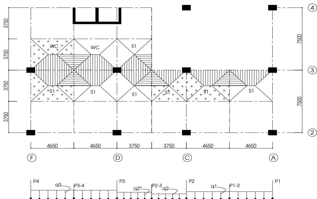
Hình 3.2: Sơ đồ phân bố tải trọng tầng 2
