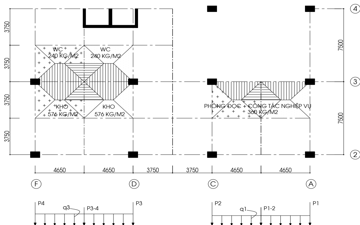
Hình 24: Sơ đồ phân hoạt tải 2 – tầng 2
