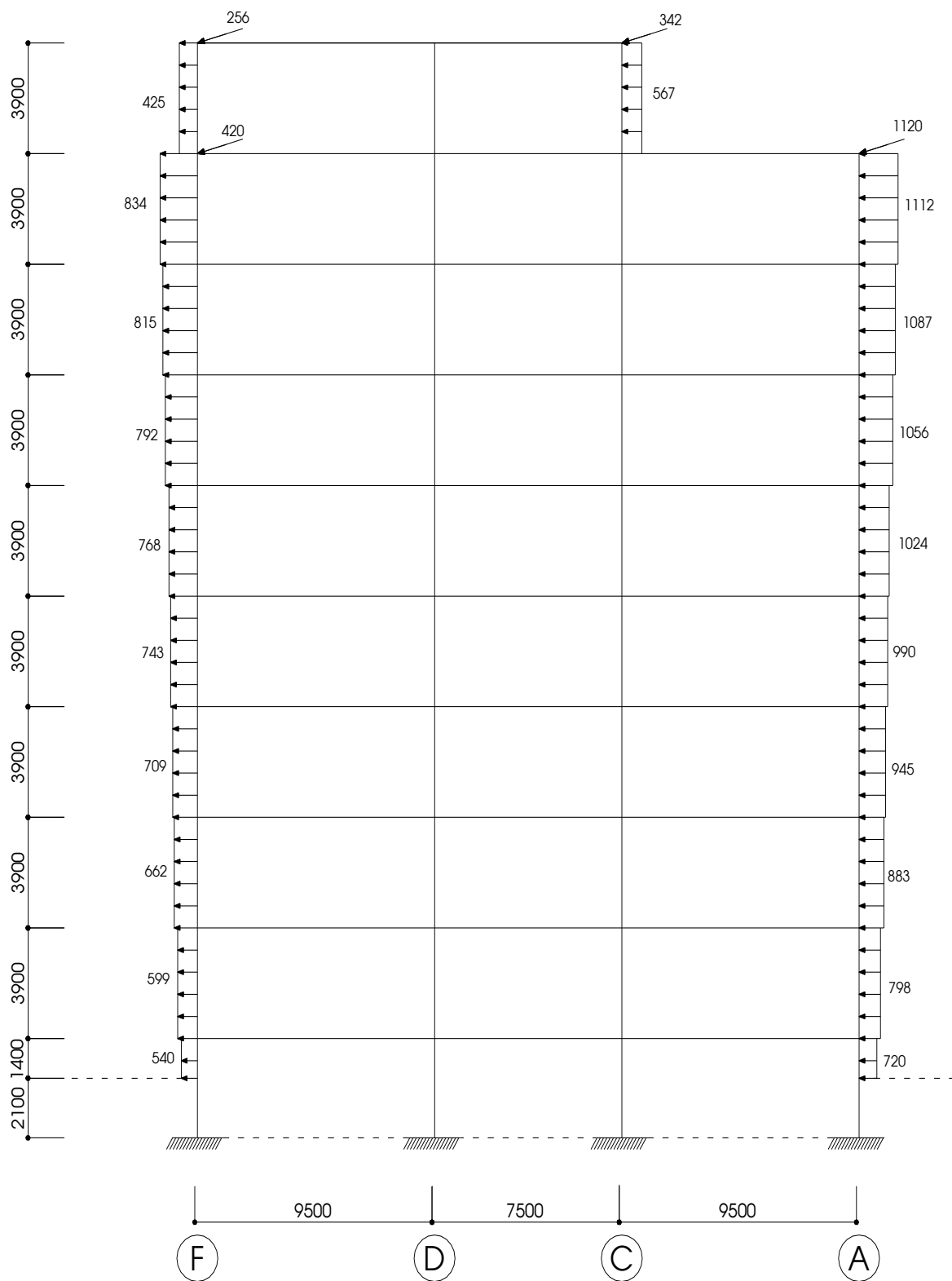
Hình 3.16: Sơ đồ gió phải tác dụng vào khung K3
