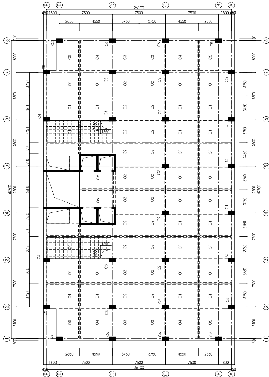
Hình 1.1: Mặt bằng kết cấu sàn tầng điển hình
