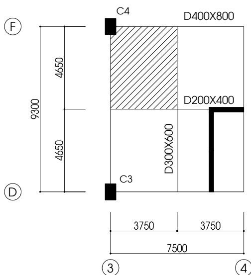
Hình 1.5: Mặt bằng diện truyền tải của cột C4 trên mái
