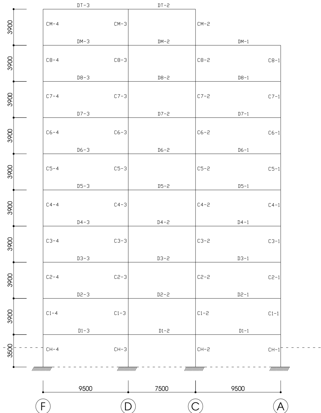
Hình 3.17: Sơ đồ phần tử dầm, cột của khung
