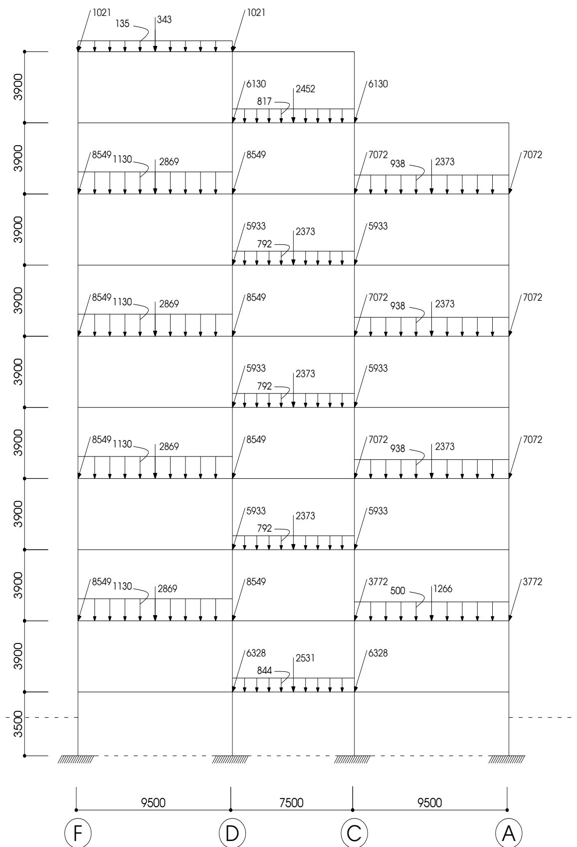
Hình 3.14: Sơ đồ hoạt tải 2 tác dụng vào khung K3
