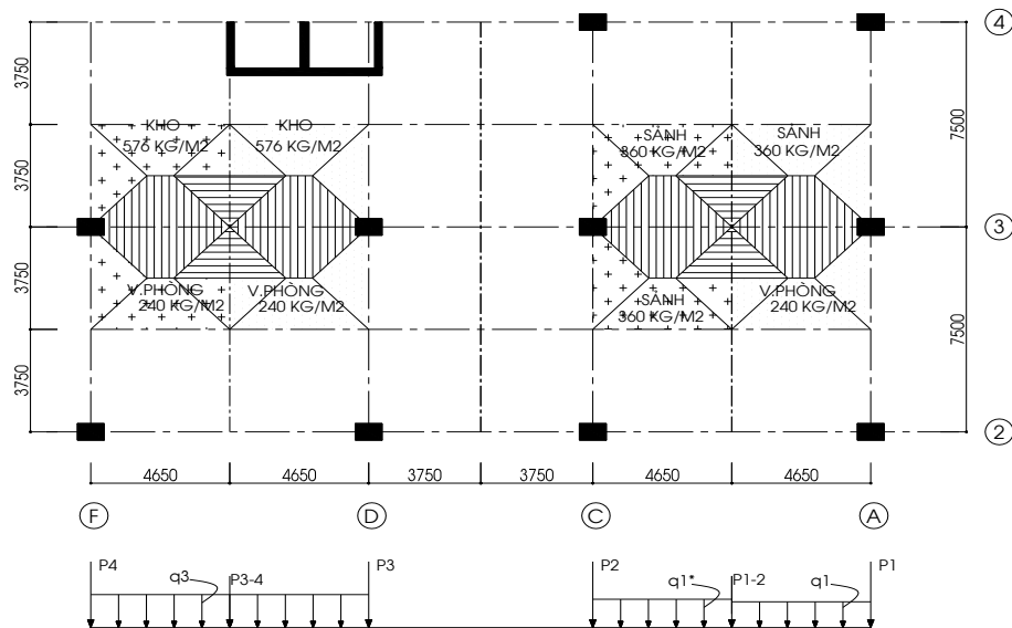
Hình 3.6: Sơ đồ phân hoạt tải 1 – tầng 1
