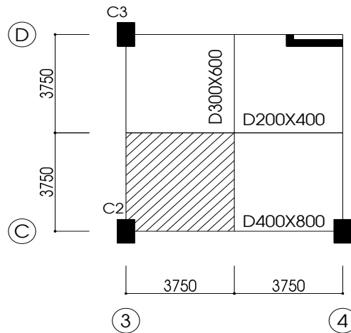
Hình 1.3: Mặt bằng diện truyền tải của cột C2 trên mái
