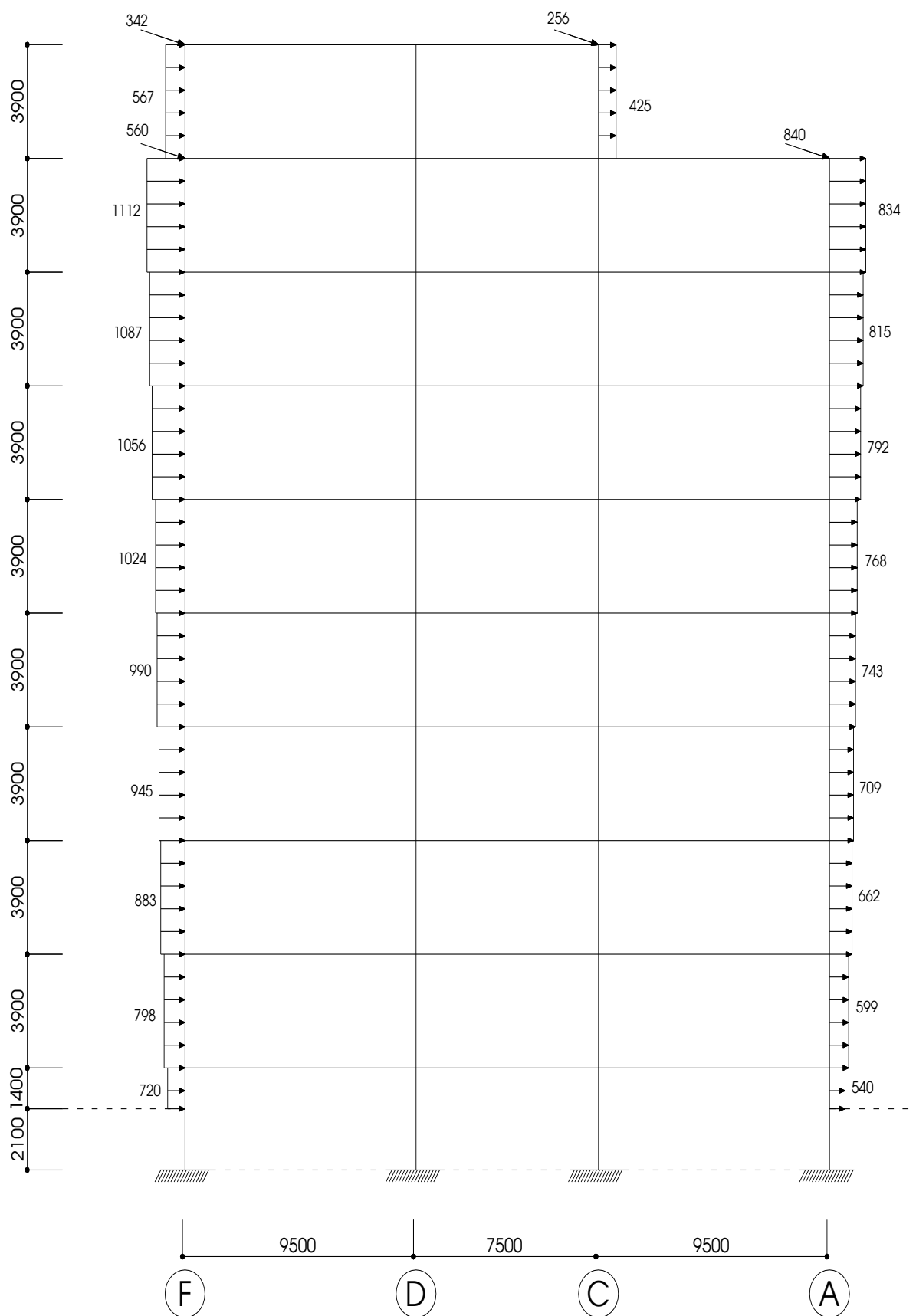
Hình 3.15: Sơ đồ gió trái tác dụng vào khung K3
