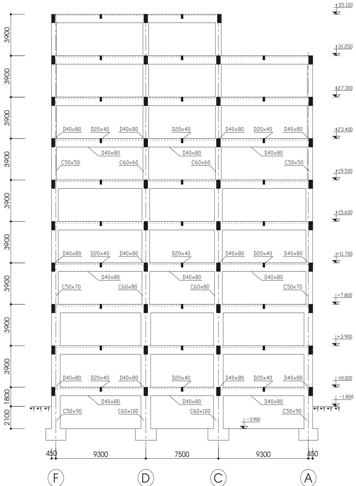
Hình 1.6: Sơ đồ hình học khung ngang trục 3
