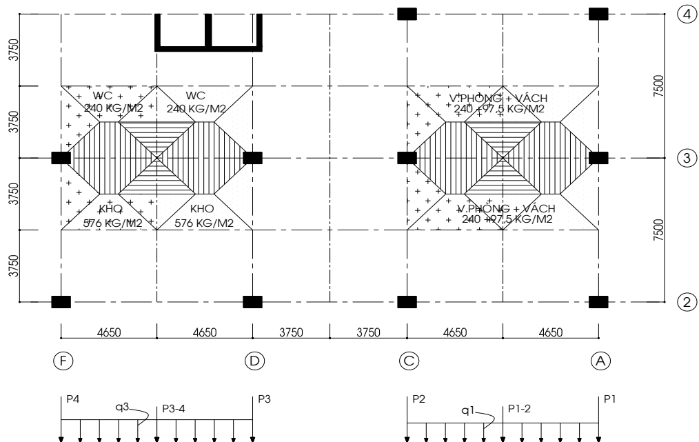
Hình 3.8: Sơ đồ phân hoạt tải 1 – tầng 3-5-7
