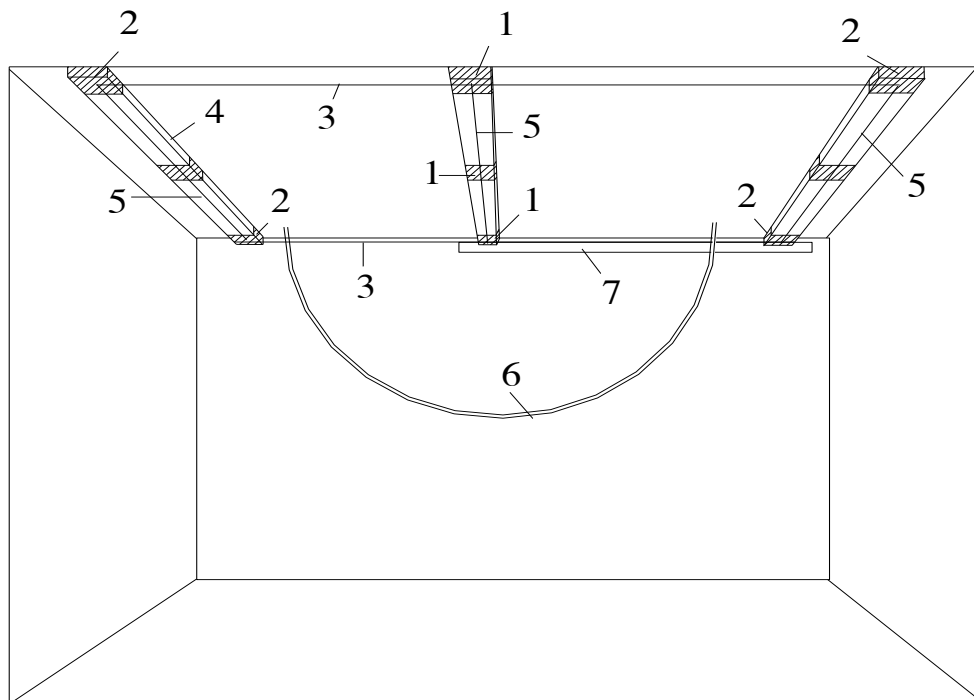
Làm dải móc vữa để trát trần
