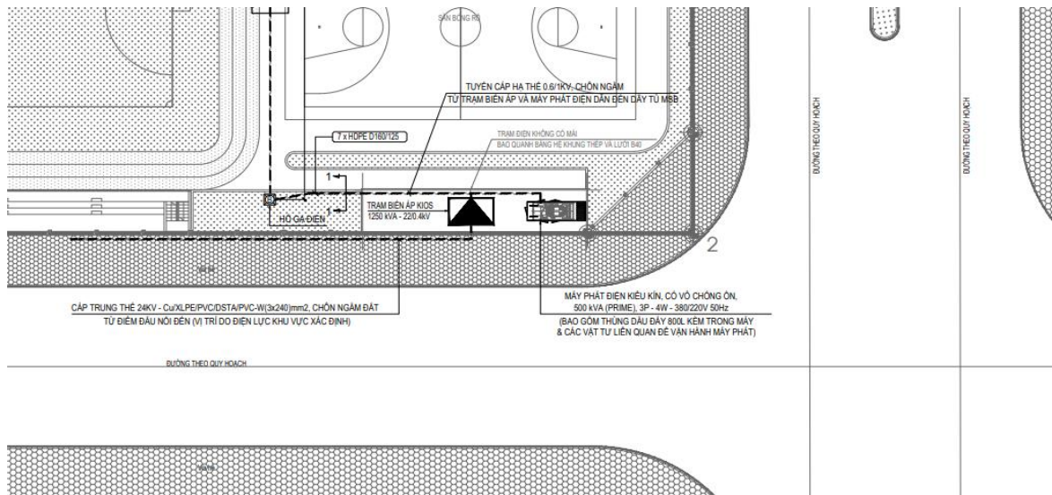
Hình 3.1 Sơ đồ vị trí đặt trạm biến áp
