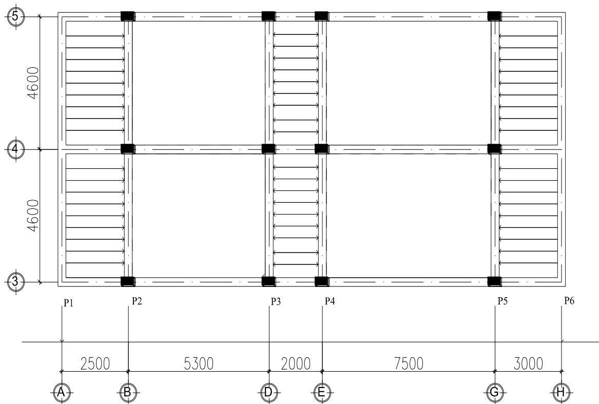
MẶT BẰNG DÒN HOẠT TẢI TẦNG MÁI SD 1
