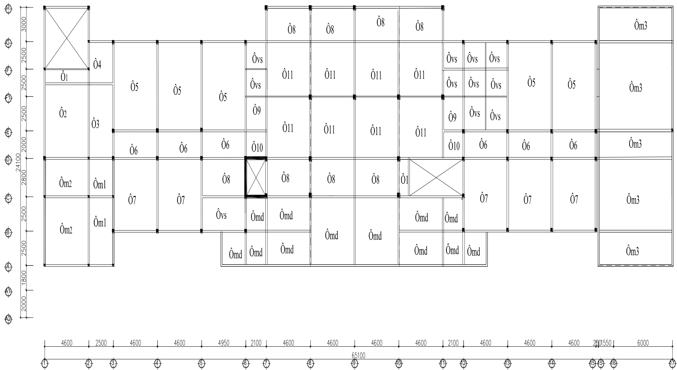
MẶT BẰNG KẾT CẤU Ô SÀN TẦNG 5
