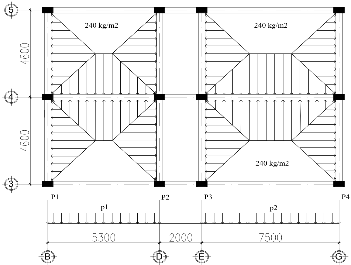
Bảng 3.15: Hoạt tải phân bố truyền tầng 2-10 sơ đồ 1
