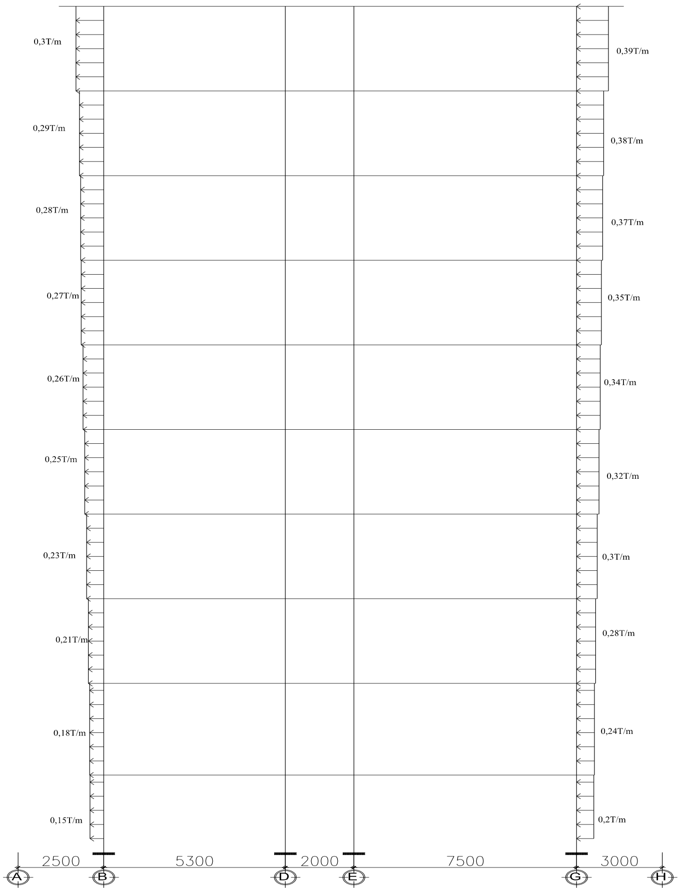
SƠ ĐỒ GIÓ PHẢI TRUYỀN VÀO KHUNG TRỤC 4
