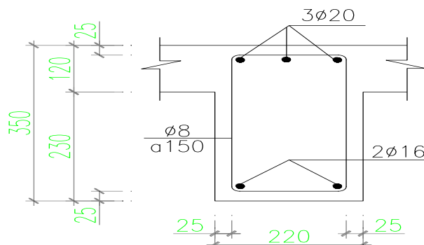
MC DẦM D72
