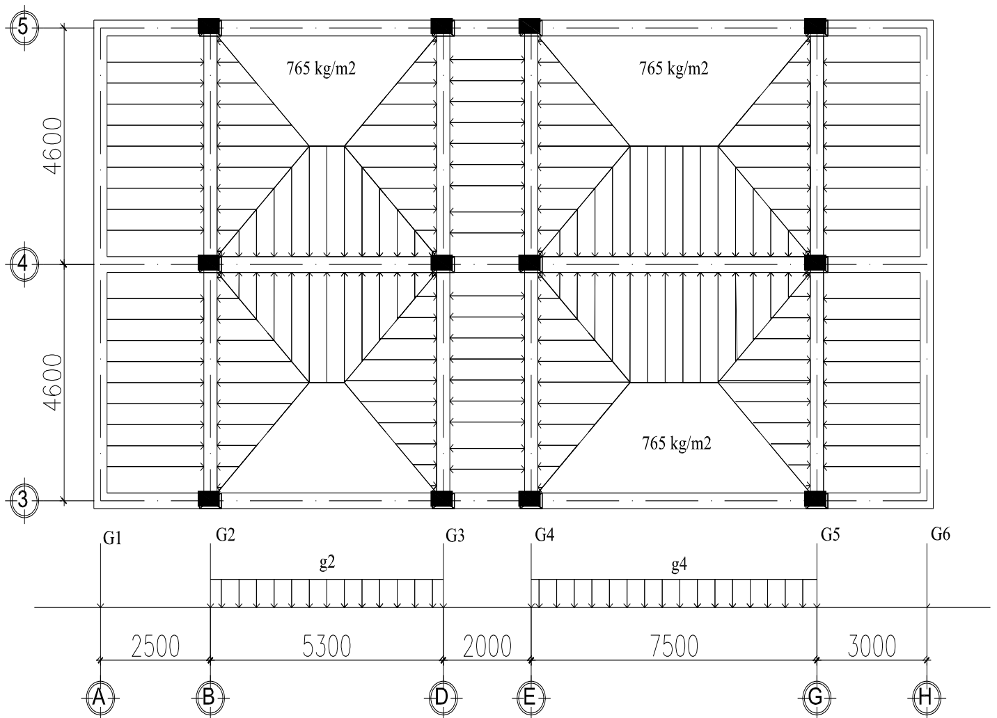
MẶT BẰNG DÒN TẢI TẦNG MÁI
