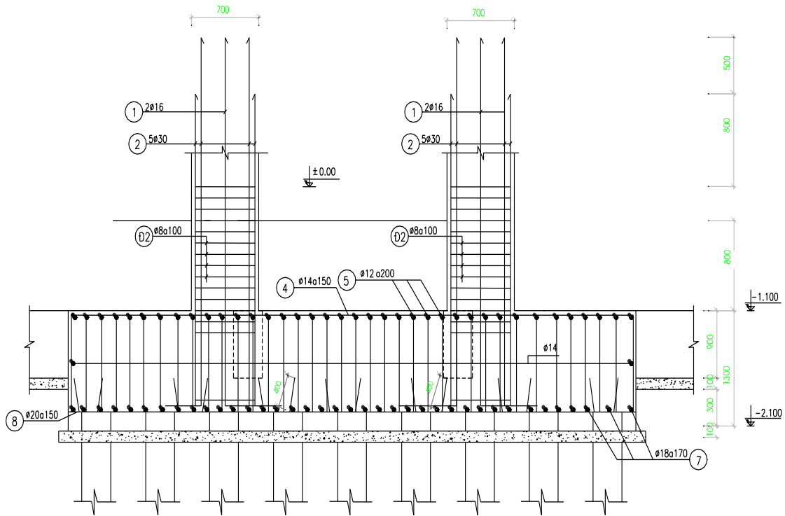
MẶT CẮT 2-2
