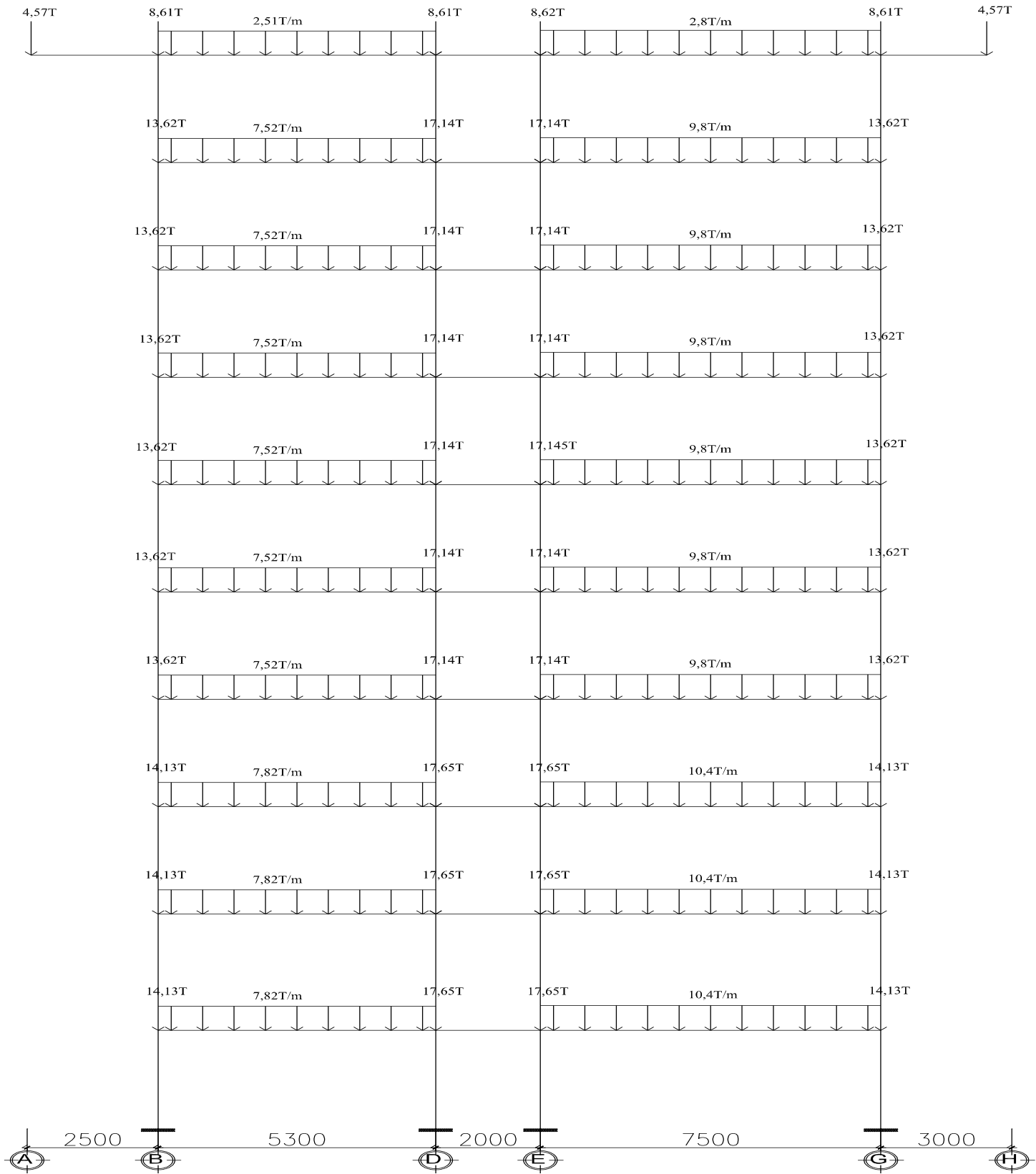
SƠ ĐỒ TÍNH TẢI TRUYỀN VÀO KHUNG TRỤC 4
