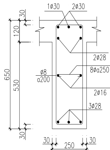
MC DÀM D64
