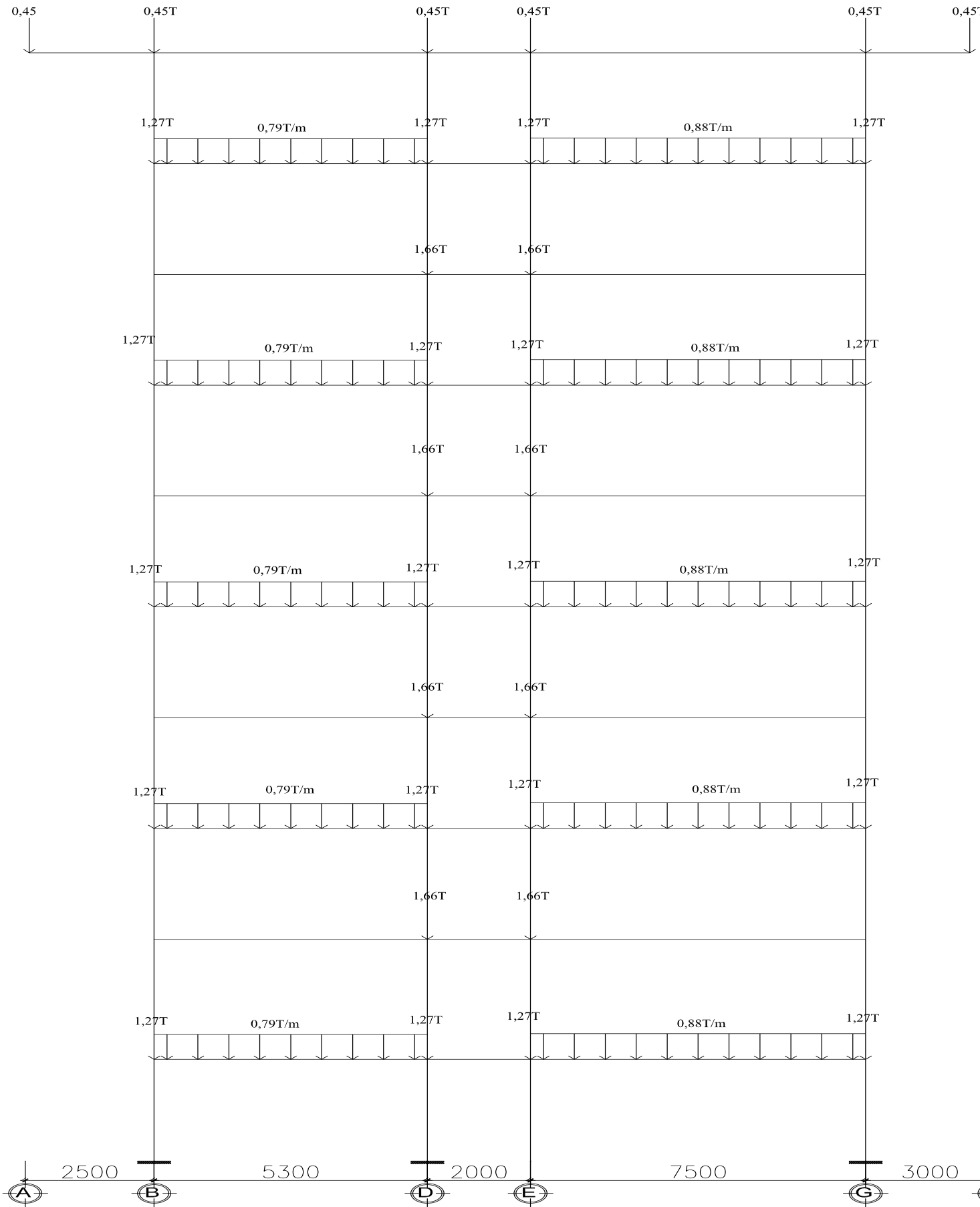
SƠ ĐỒ HOẠT TẢI 2 TRUYỀN VÀO KHUNG TRỤC 4
