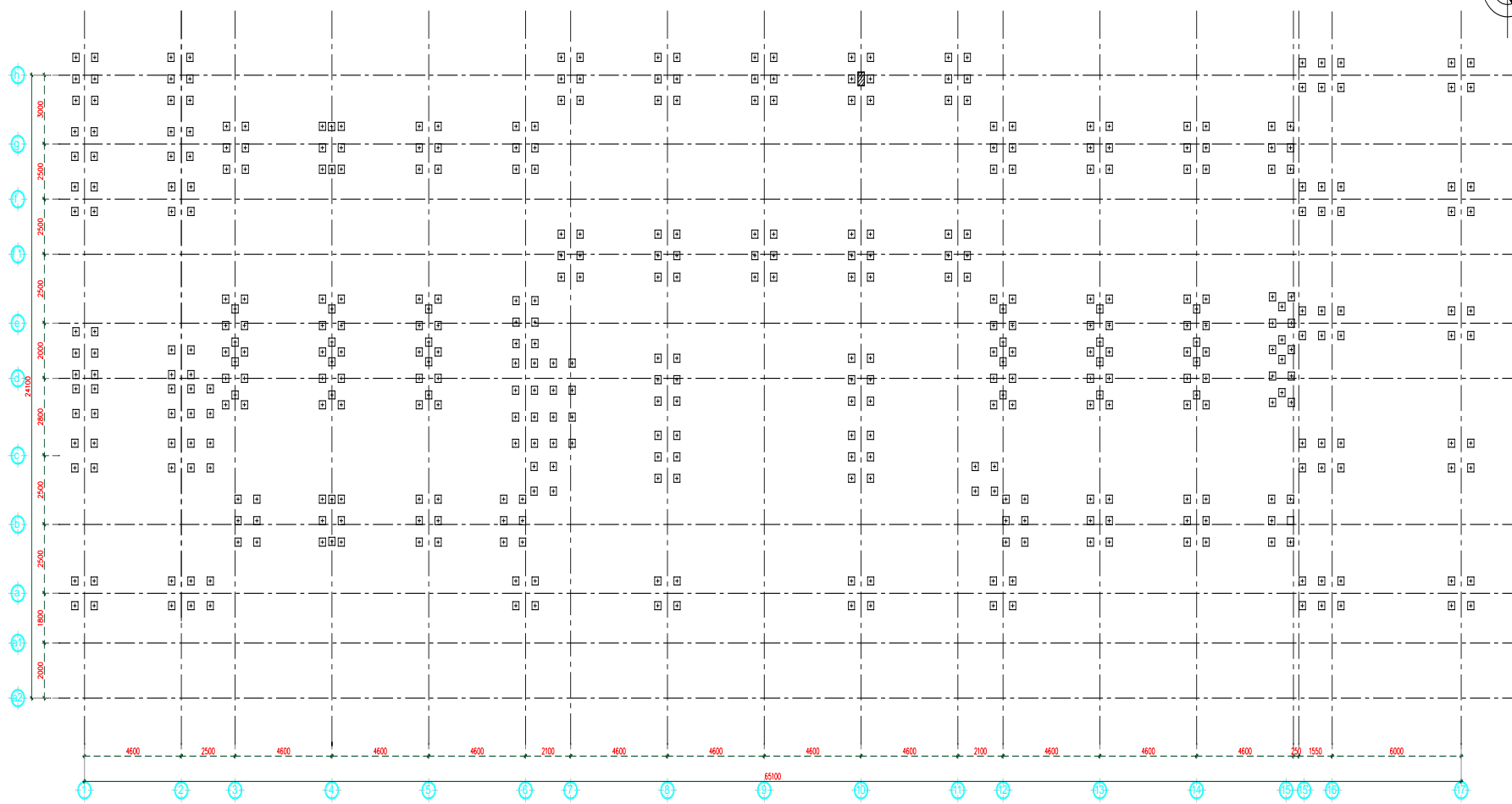
MẶT BẰNG ĐỊNH VỊ CỘC
