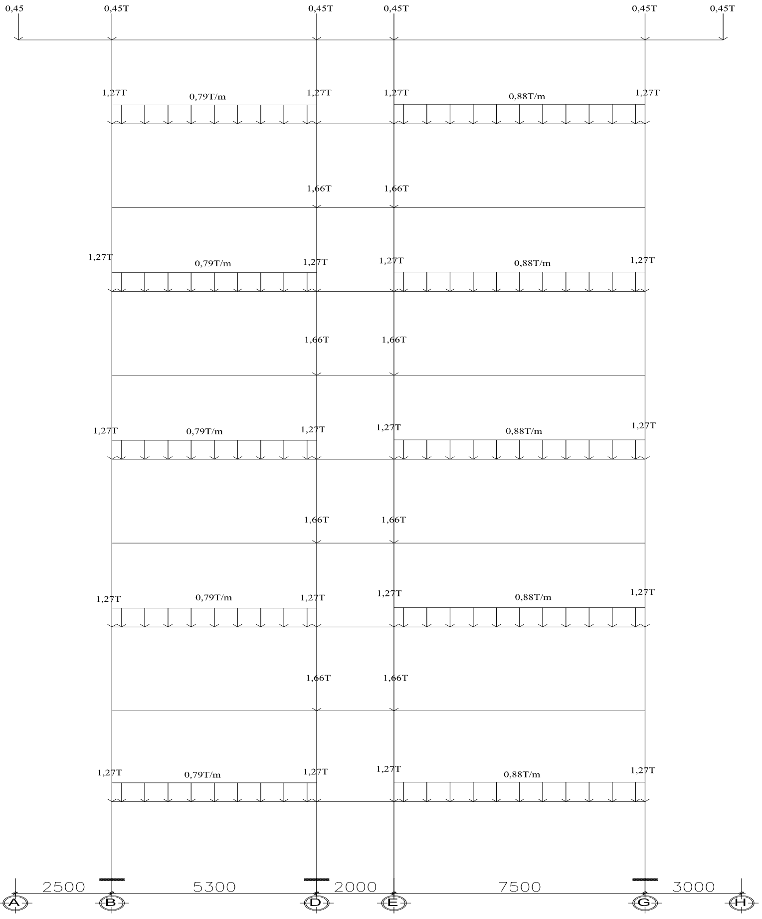
SƠ ĐỒ HOẠT TẢI 1 TRUYỀN VÀO KHUNG TRỤC 4
