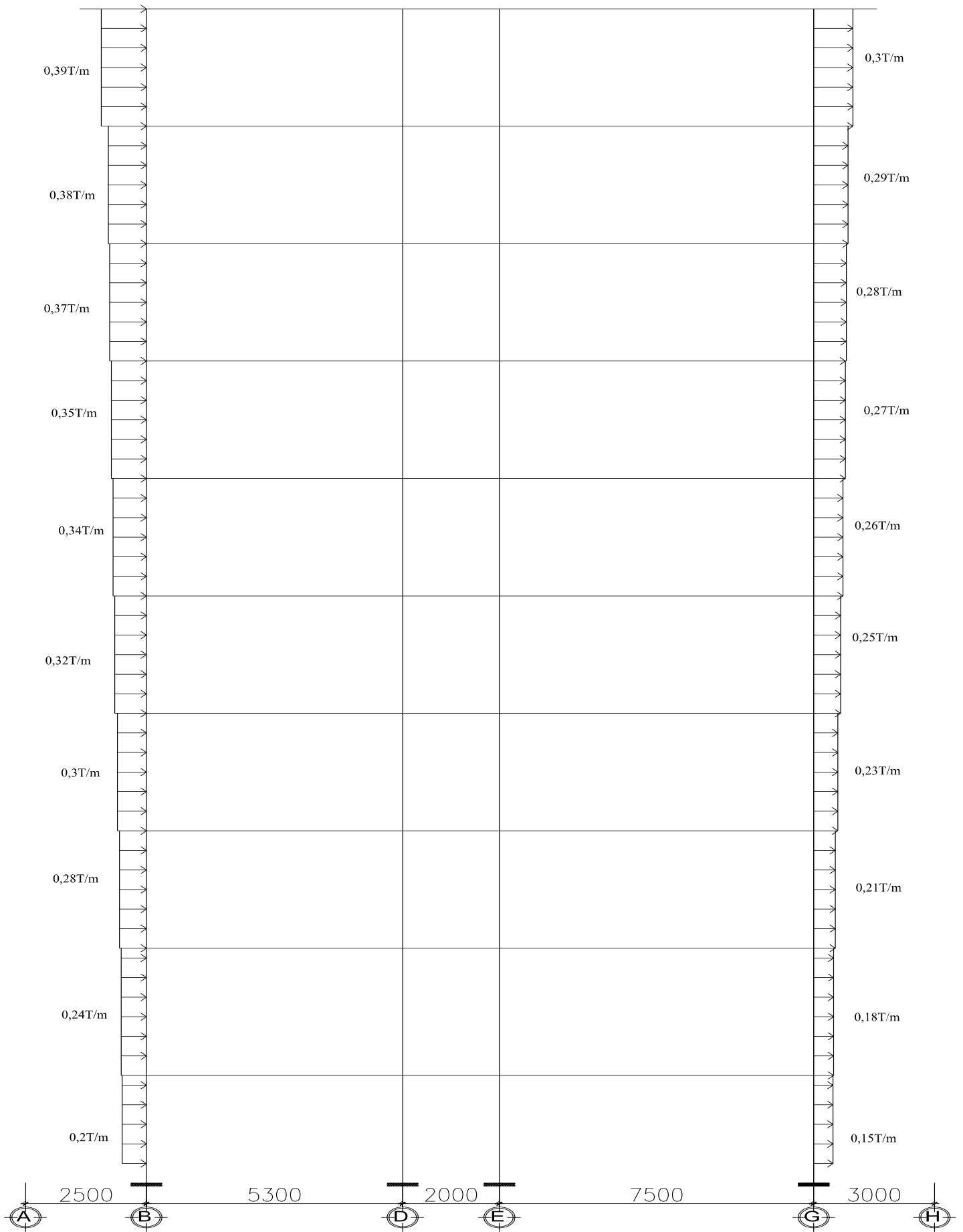
SƠ ĐỒ GIÓ TRÁI TRUYỀN VÀO KHUNG TRỤC 4
