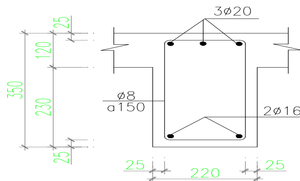
MC DẦM D42
