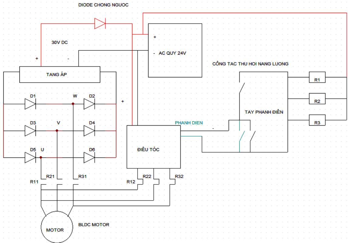
Hình 3.8: Sơ đồ nguyên lý mạch hãm và thu hồi năng lượng
