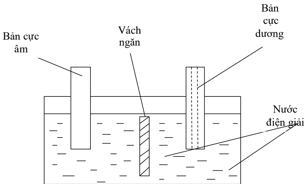
Hình 2.36: Cấu trúc chung của một tế bào ắc quy.
