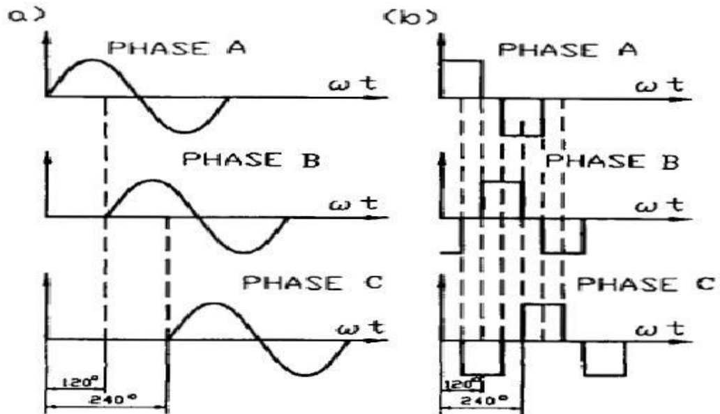
Hình 2.14: Giảm đồ so sánh dạng sóng sin ba pha và DC ba pha
