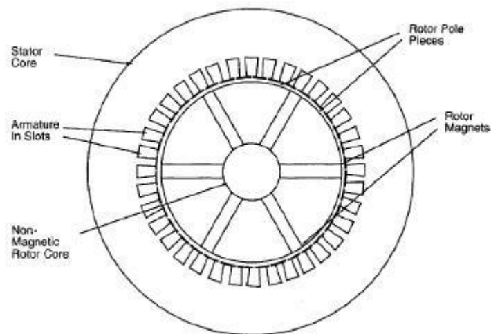
Hình 2.12: Kiểu rotor nam châm nằm bên trong.
