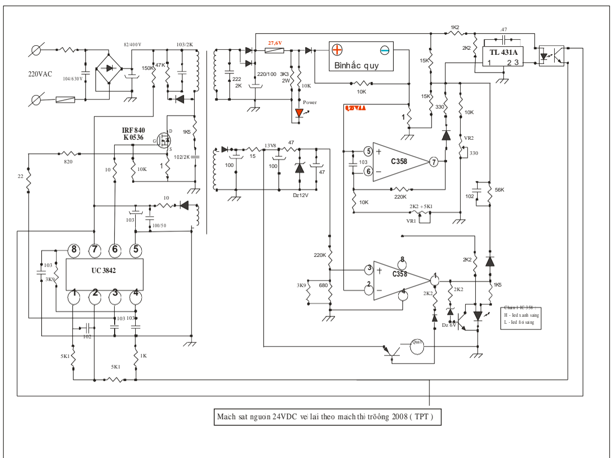
Hình 2.38: Mạch sạc ắc quy xe điện sử dụng IC UC3842.
