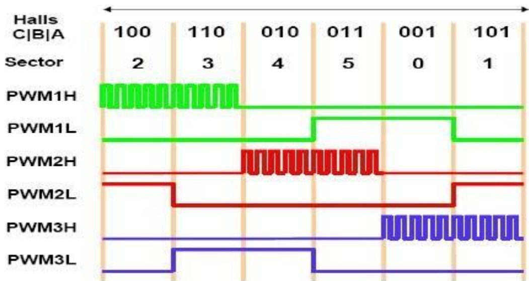
Hình 2.23: Giản đồ xung điều khiển PWM kênh trên.
