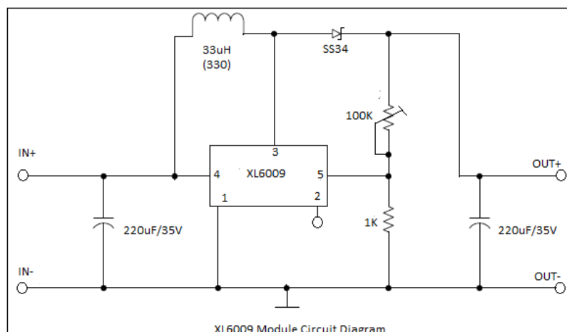
Hình 3.10: Sơ đồ nguyên lý của mạch ổn áp
