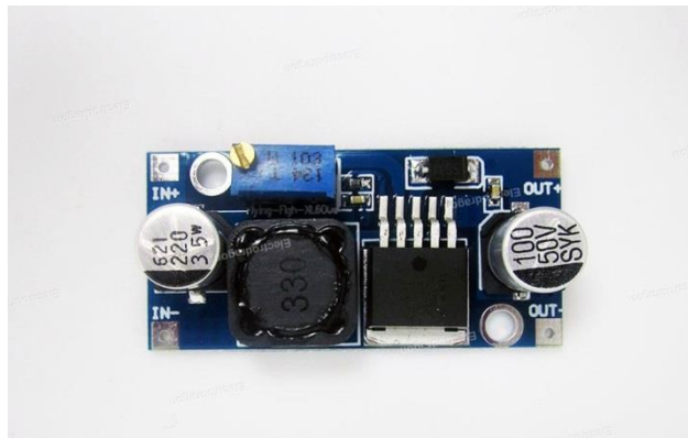
Hình 3.11: Mạch ổn áp
