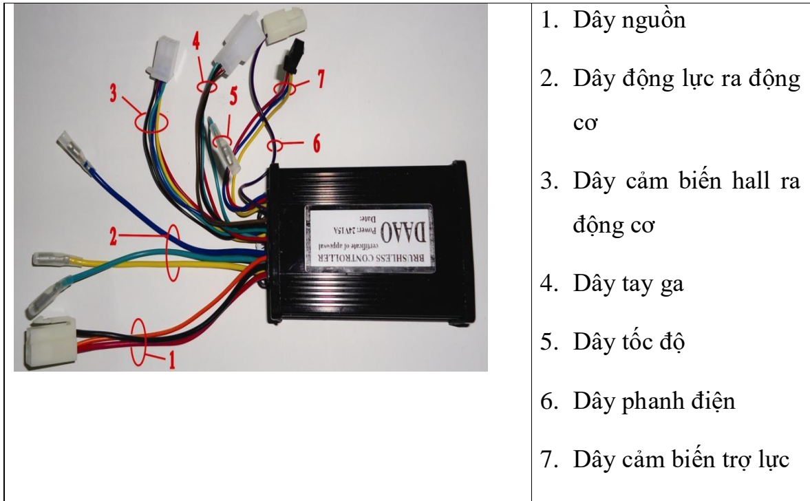
Hình 3.4: Điều tốc xe đạp điện
