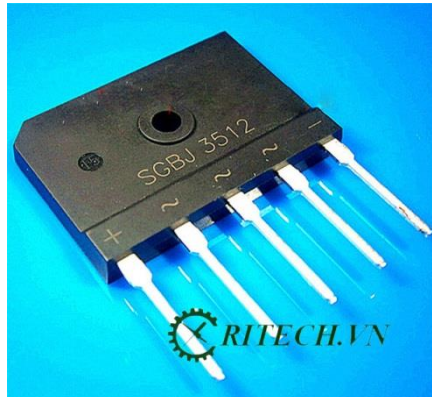
Hình 3.9: Cầu chỉnh lưu 3 pha
