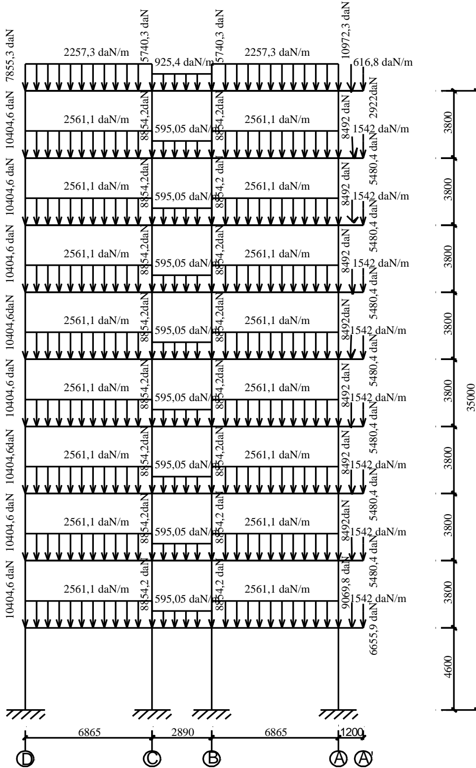
tĩnh tải tác dụng vào khung trục 5
