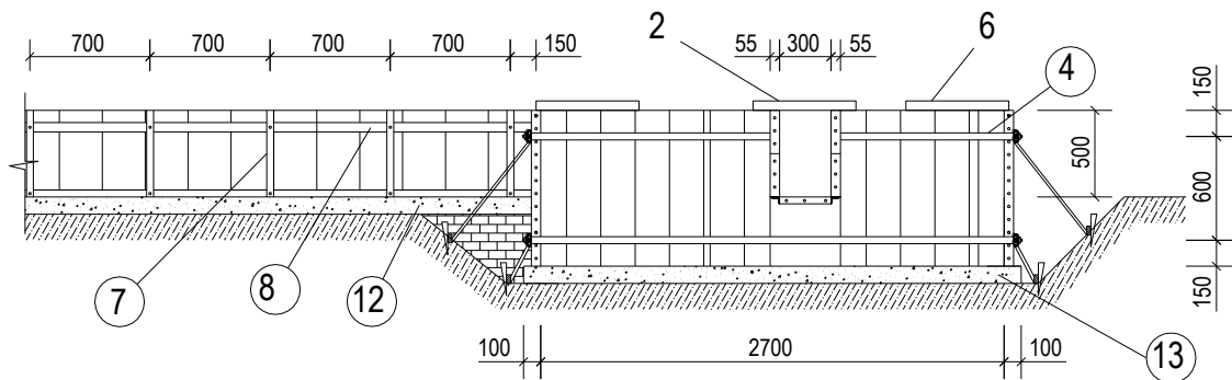
Mặt bên đài móng A5
