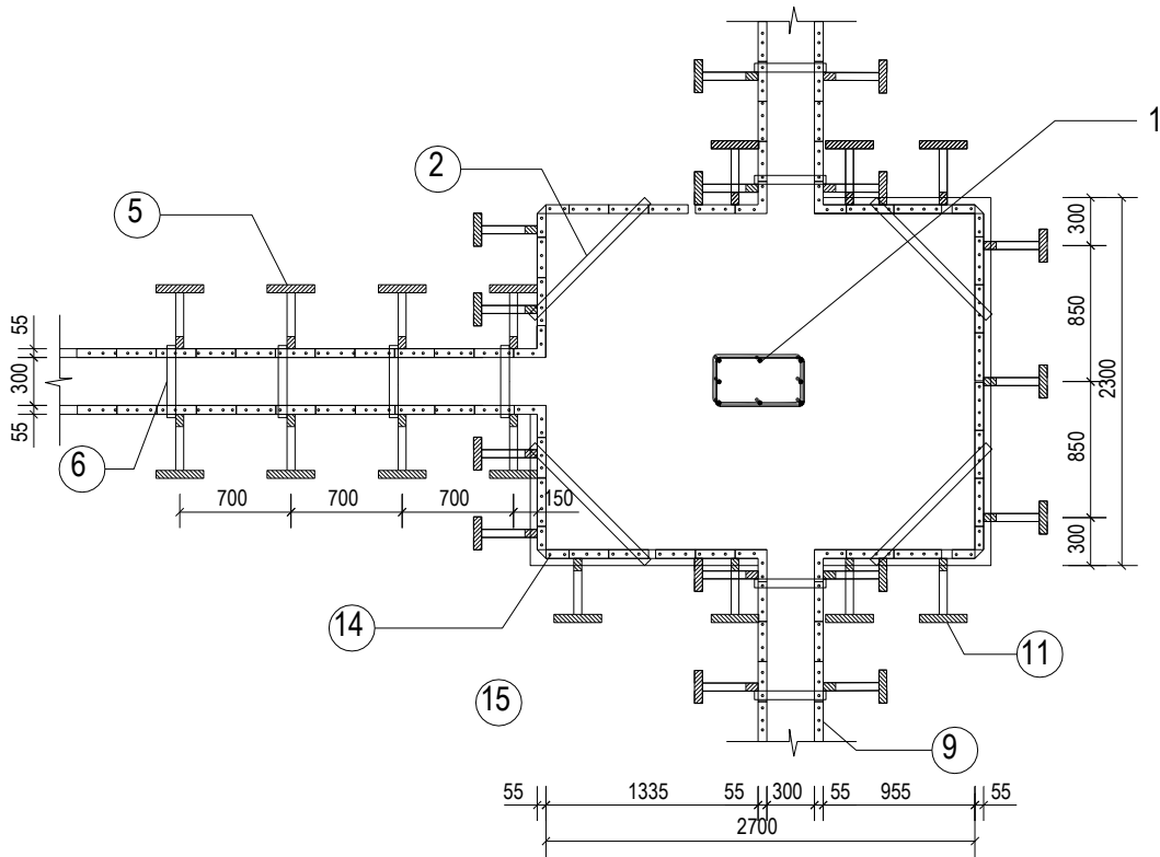
Mặt bằng đài móng A5
