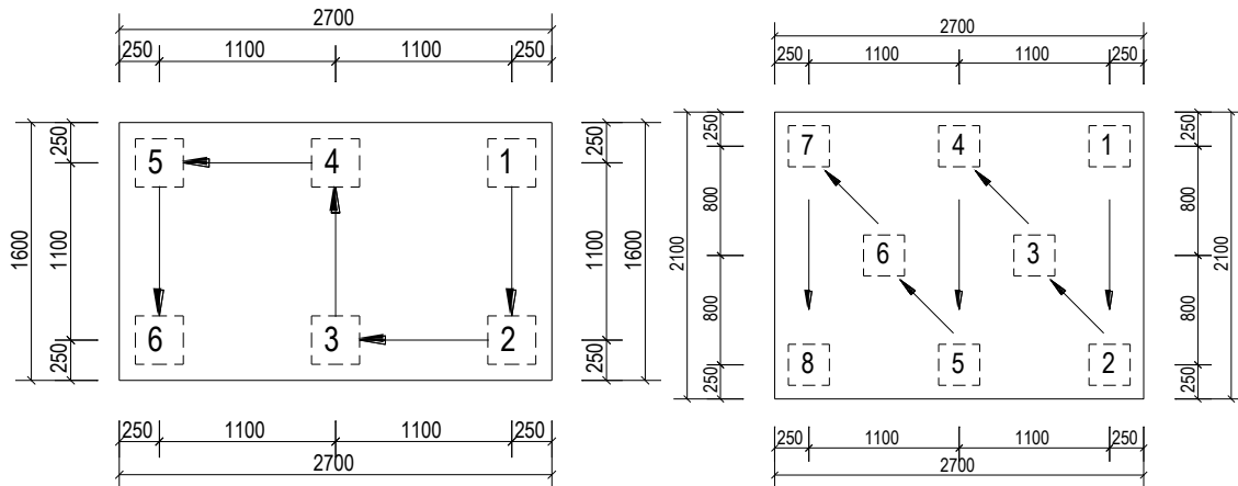
Sơ đồ ép cọc đài móng D5 và A5
