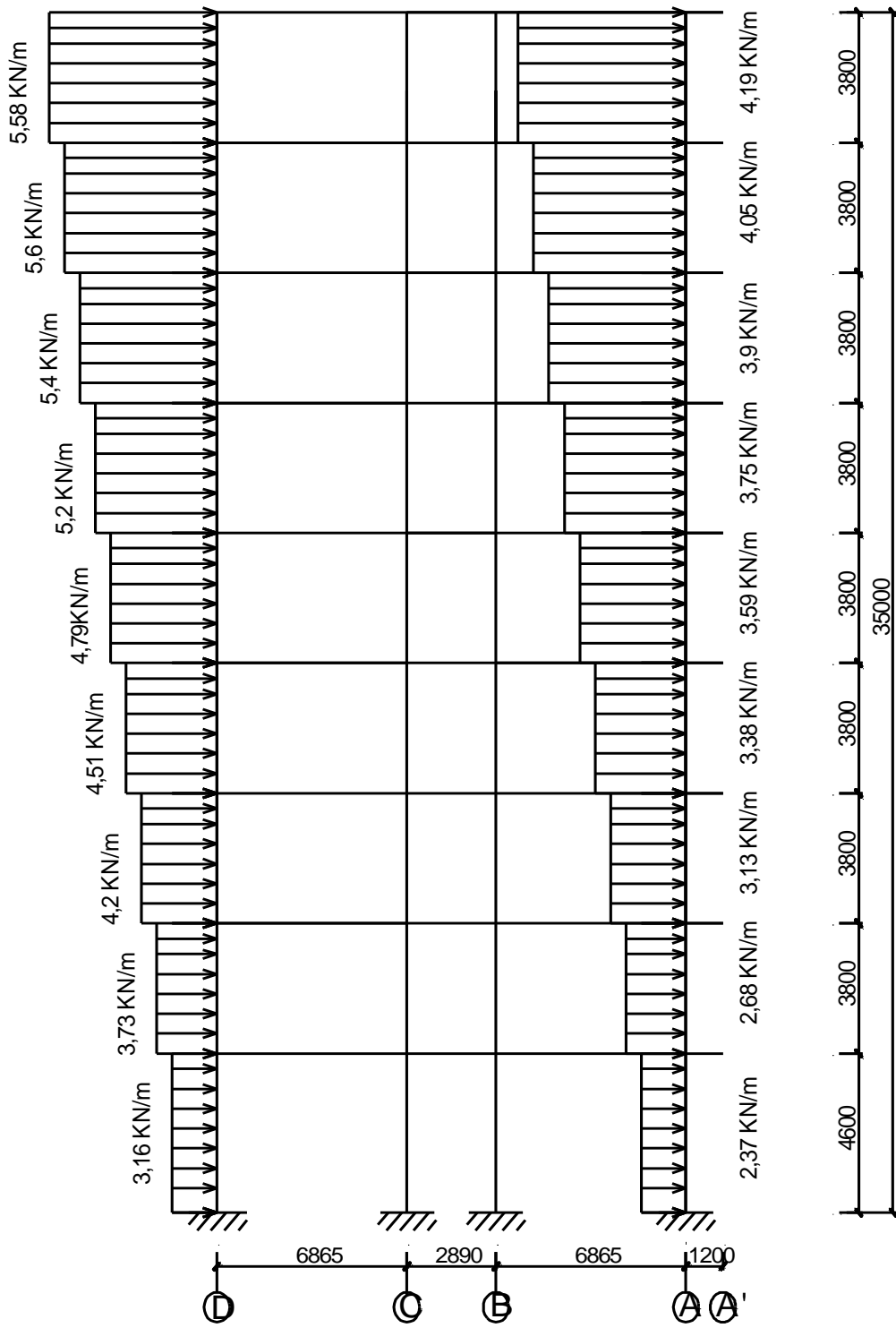
Sơ đồ gió trái tác dụng vào khung trục 5
