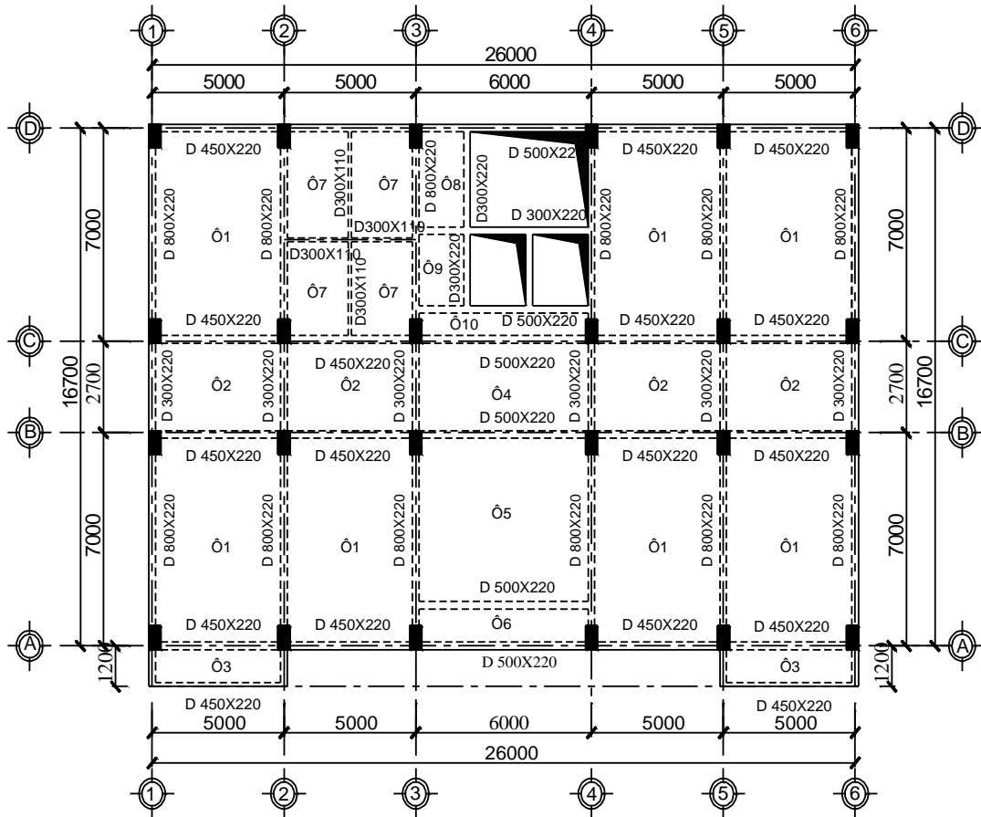
Mặt bằng kết cấu sàn tầng 5
