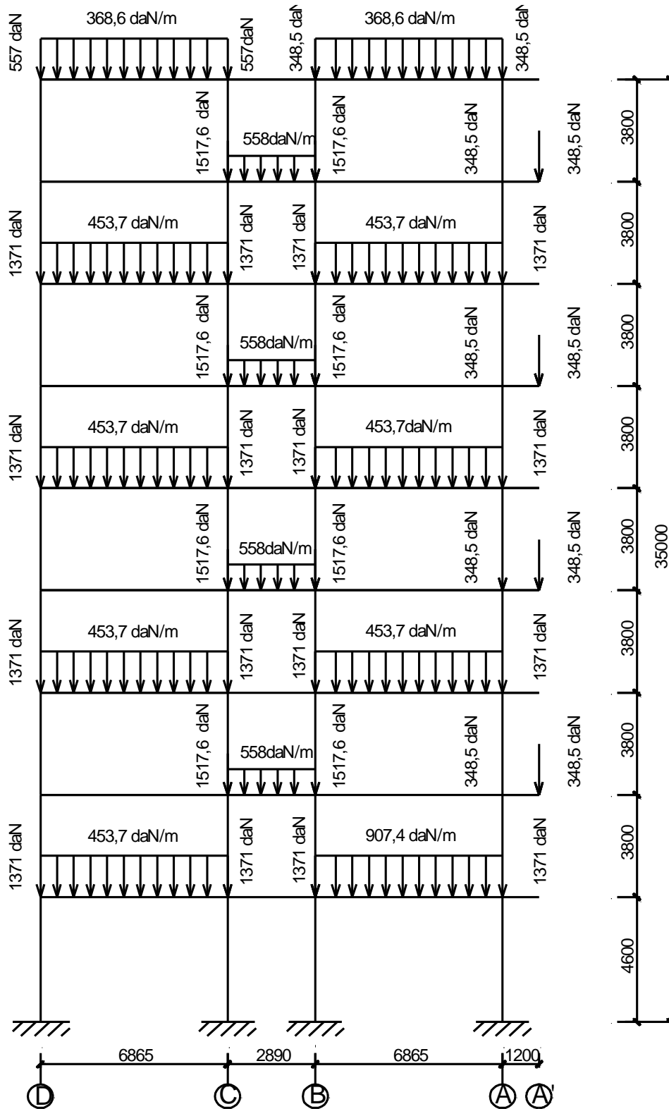
hoạt tải 1 tác dụng vào khung trục 5
