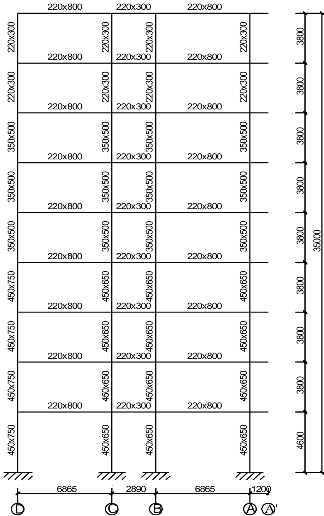
Sơ đồ kết cấu khung trục 5
