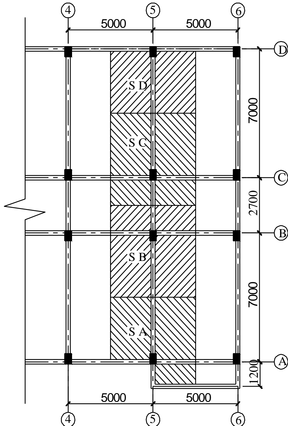
Diện truyền tải của các cột trục 5
