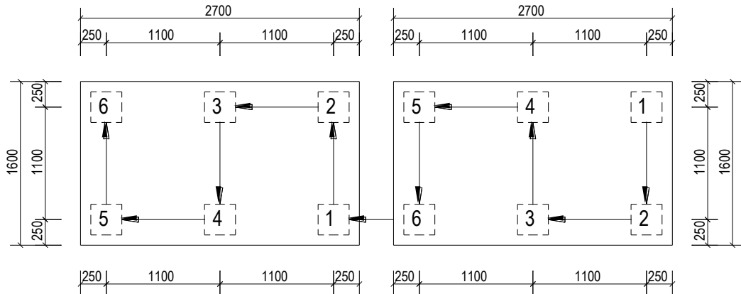
Sơ đồ ép cọc đài móng C5 và B5
