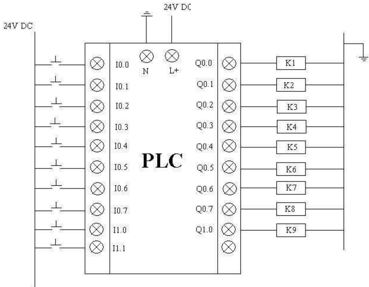
Hình 3.3: Sơ đồ đầu nối đầu vào ra.
