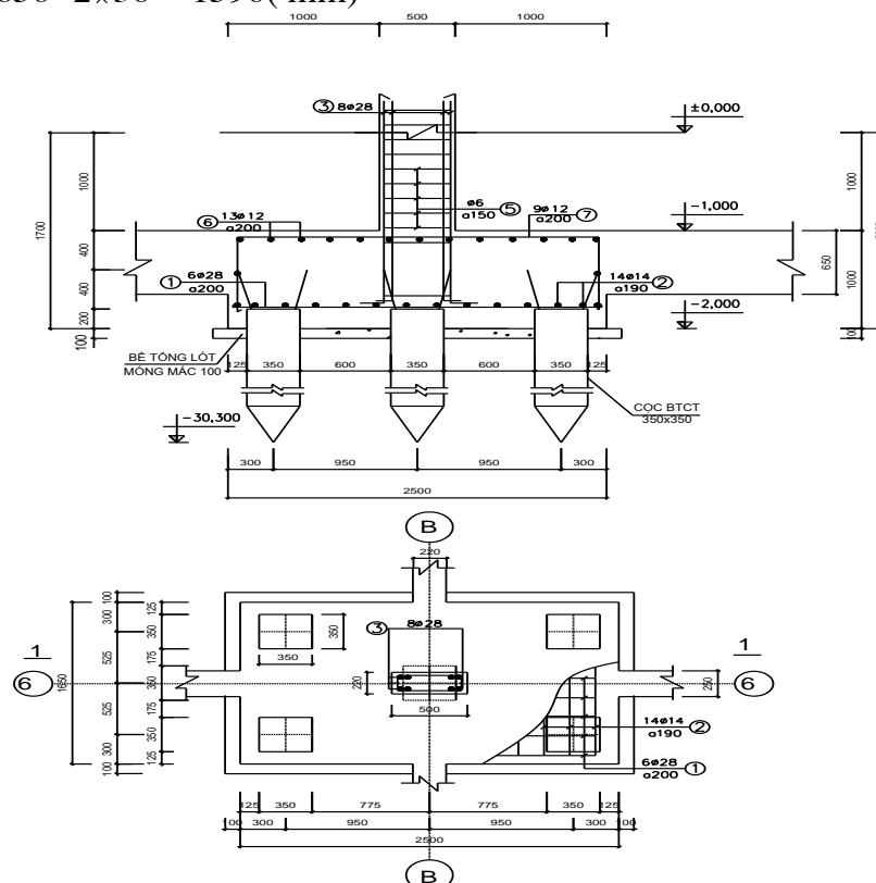
Bố trí thép móng M1
