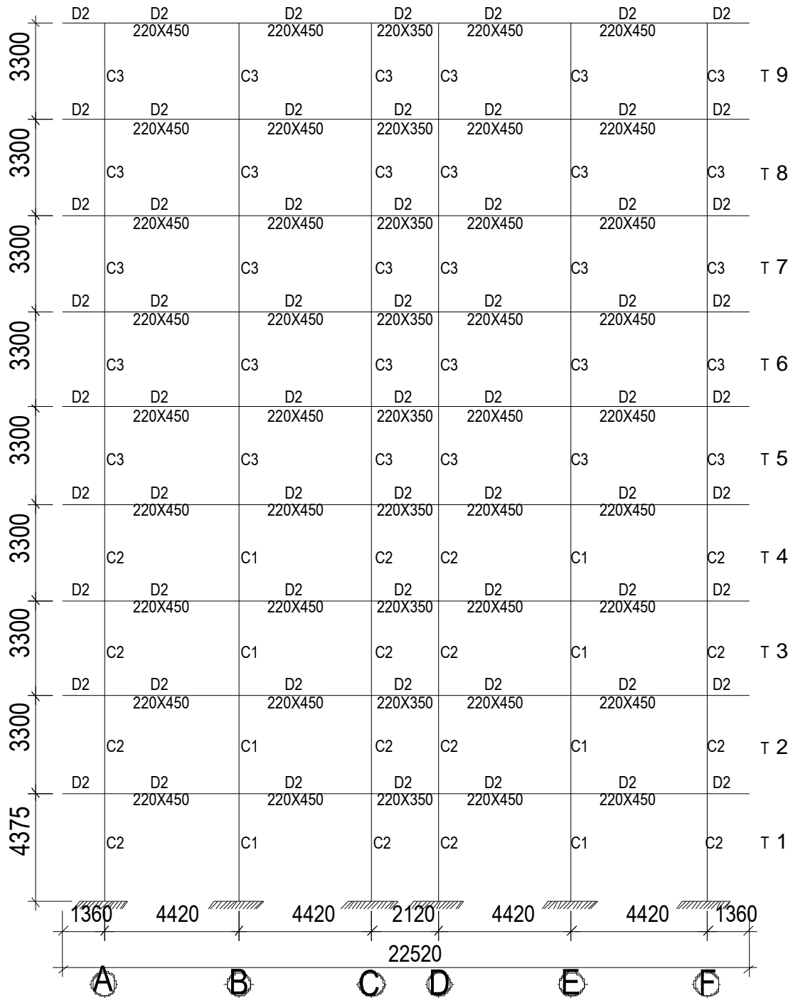
SƠ ĐỒ TÍNH TOÁN KHUNG TRỤC 6
