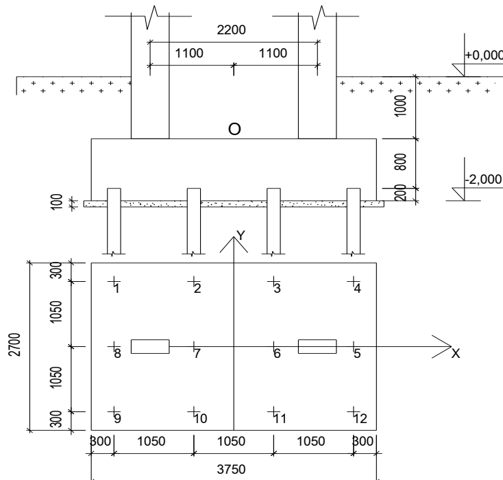
Bố trí cọc
