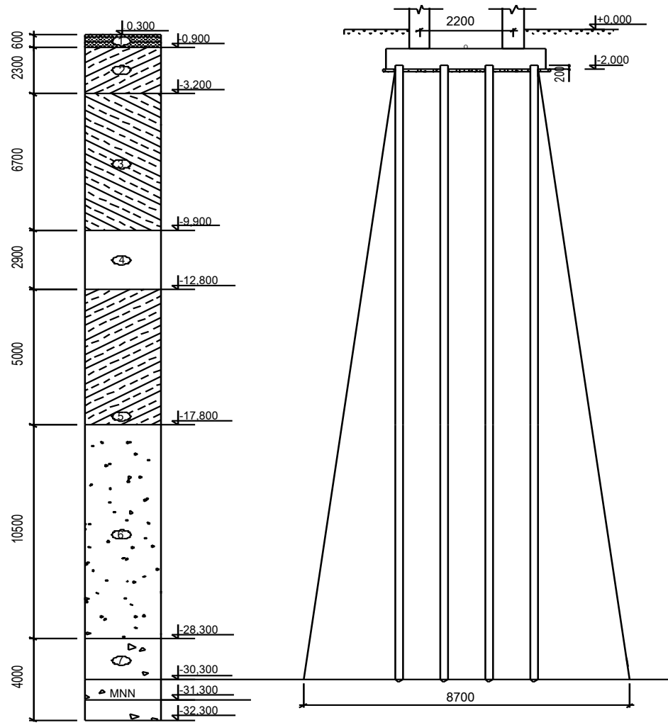
Đáy móng quy - ớc
