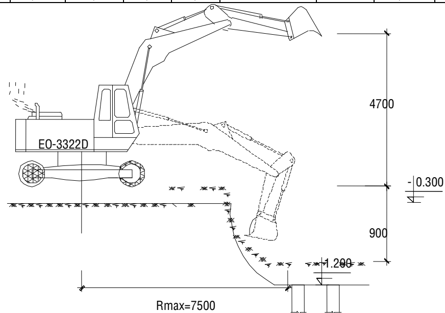
CÁC TƯ THỂ ĐÀO ĐẤT
