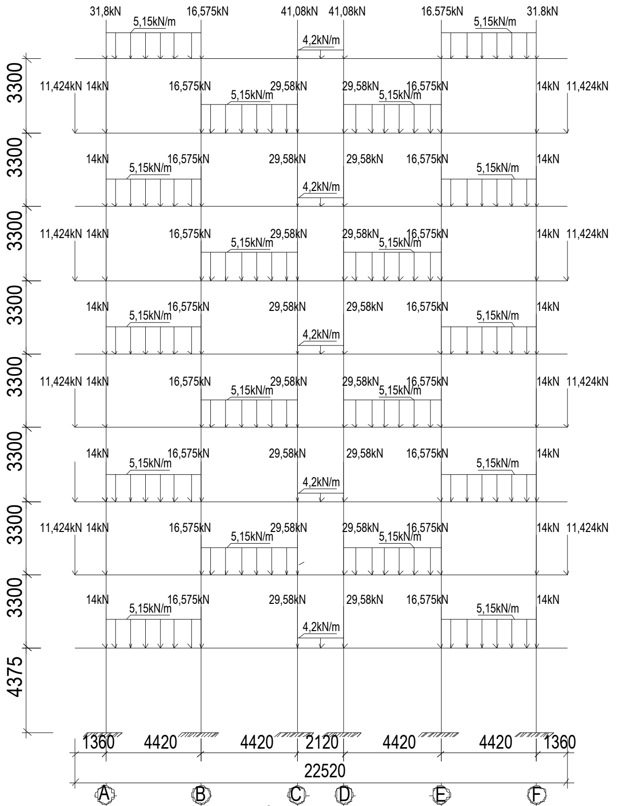
SƠ ĐỒ HOẠT TẢI 2 TÁC DỤNG LÊN KHUNG K6
