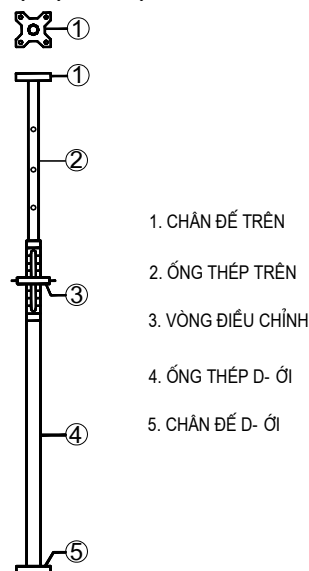
CẤU TẠO CÂY CHỐNG ĐƠN
