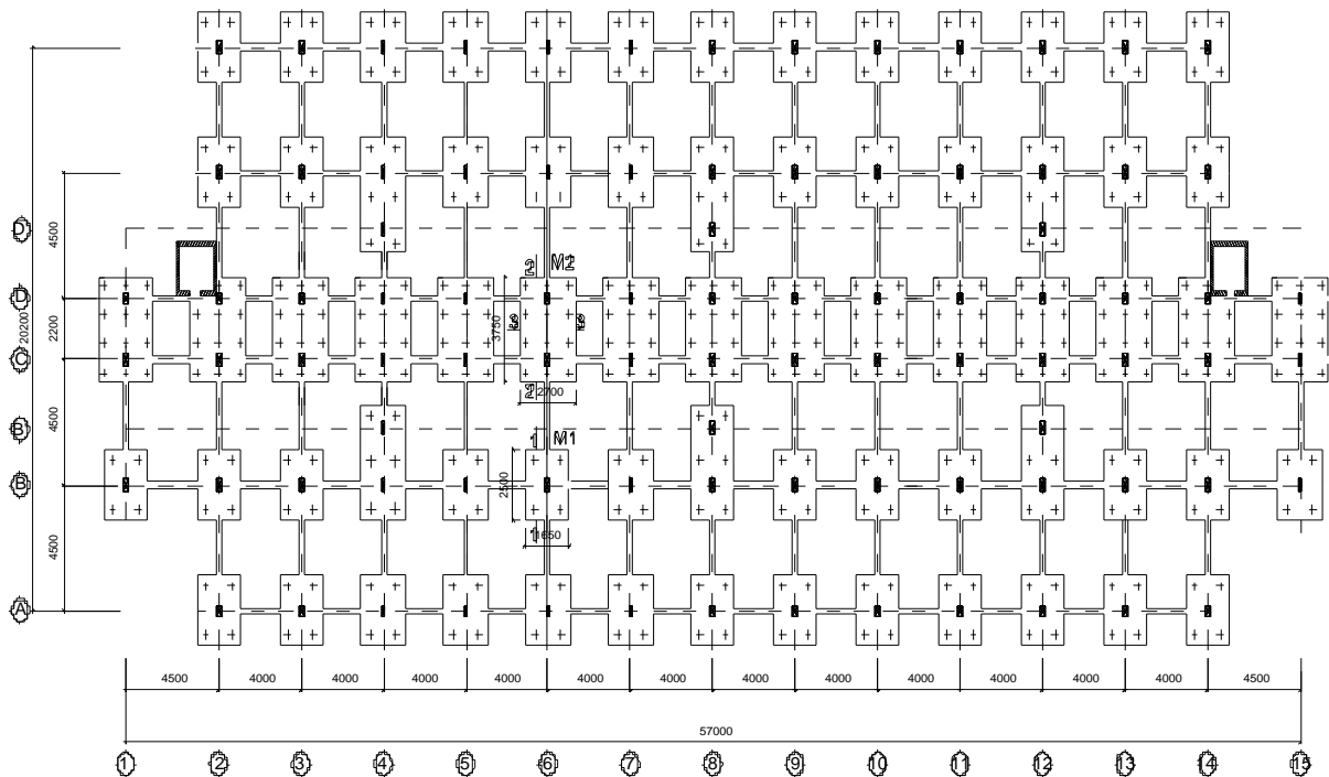
Mặt bằng móng cọc ép.
