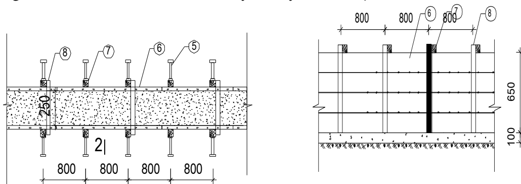
MẶT BẰNG VÁN KHUÔN GIẰNG M? NG TL: 1/30 MẶT ĐỨNG VÁN KHUÔN GIẰNG M? NG TL: 1/30
