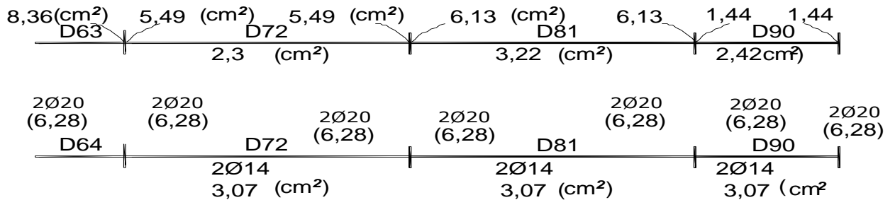
Dầm mái
