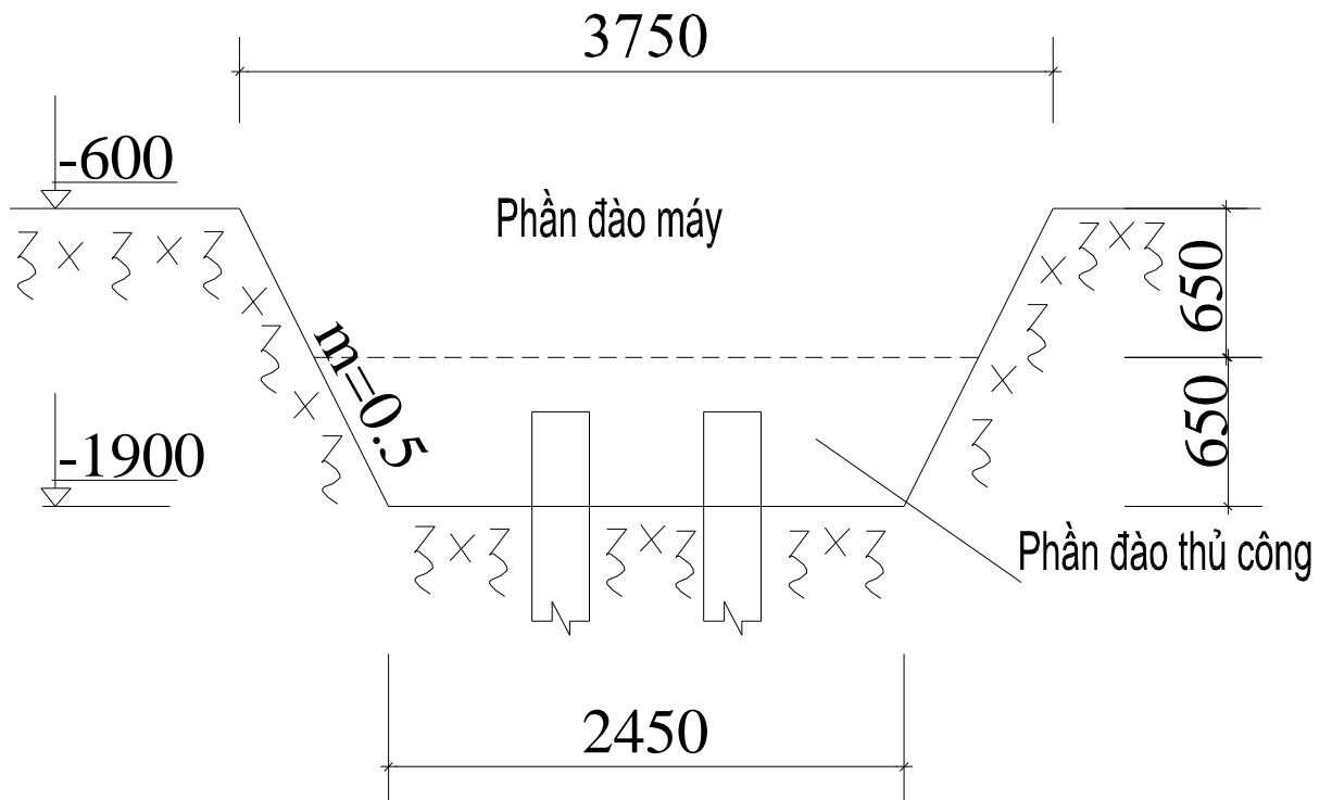
Mặt cắt ngang hố đào móng M1
