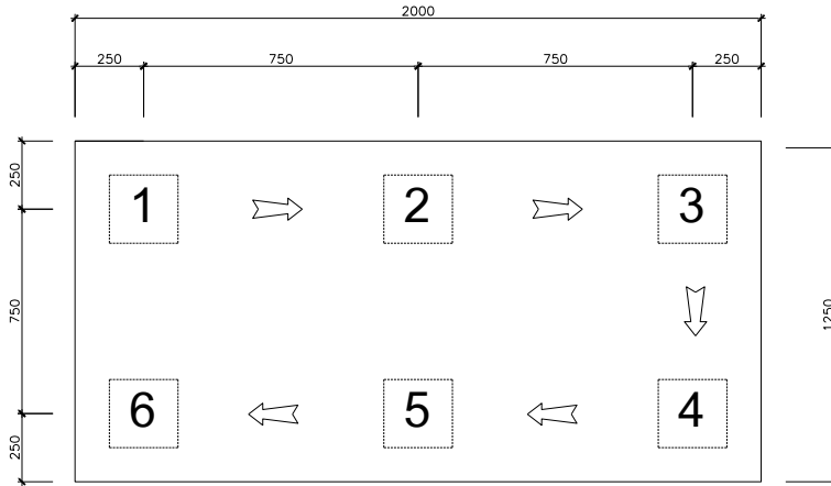
ĐÀI MÓNG M1
