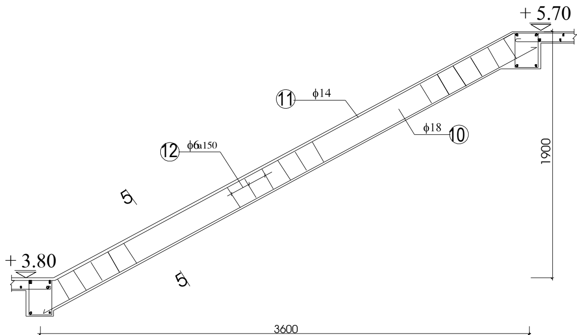
Bố trí thép cột thang
