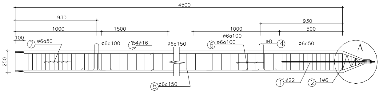
CẤU TẠO ĐOẠN CỌC C1
