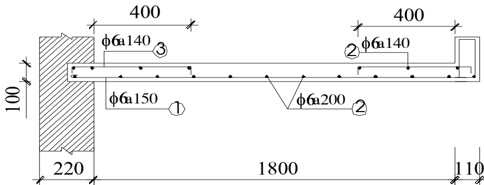
BẢN ĐÀN THANG
