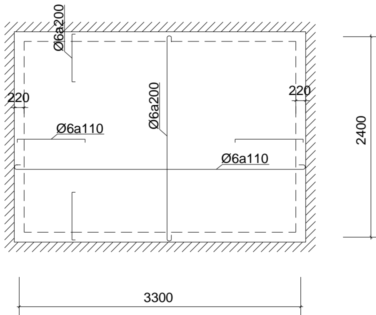
Mặt bằng bố trí thép sàn hành lang
