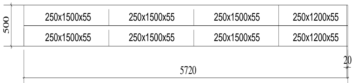
Tổ hợp ván khuôn thành dầm
