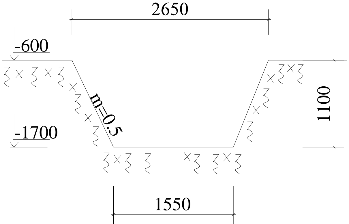
Mặt cắt ngang hố đào giằng móng
