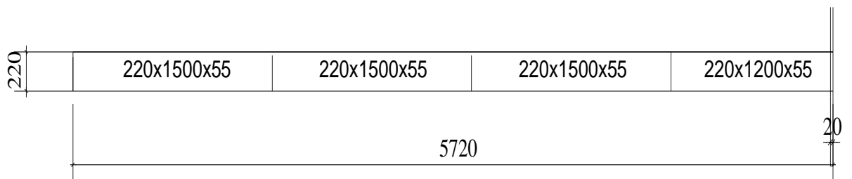
Tổ hợp ván khuôn đáy dầm
