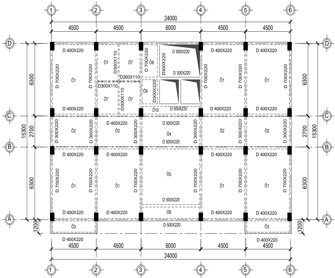
MẶT BẰNG KẾT CẤU SÀN TẦNG ĐIỂN HÌNH
