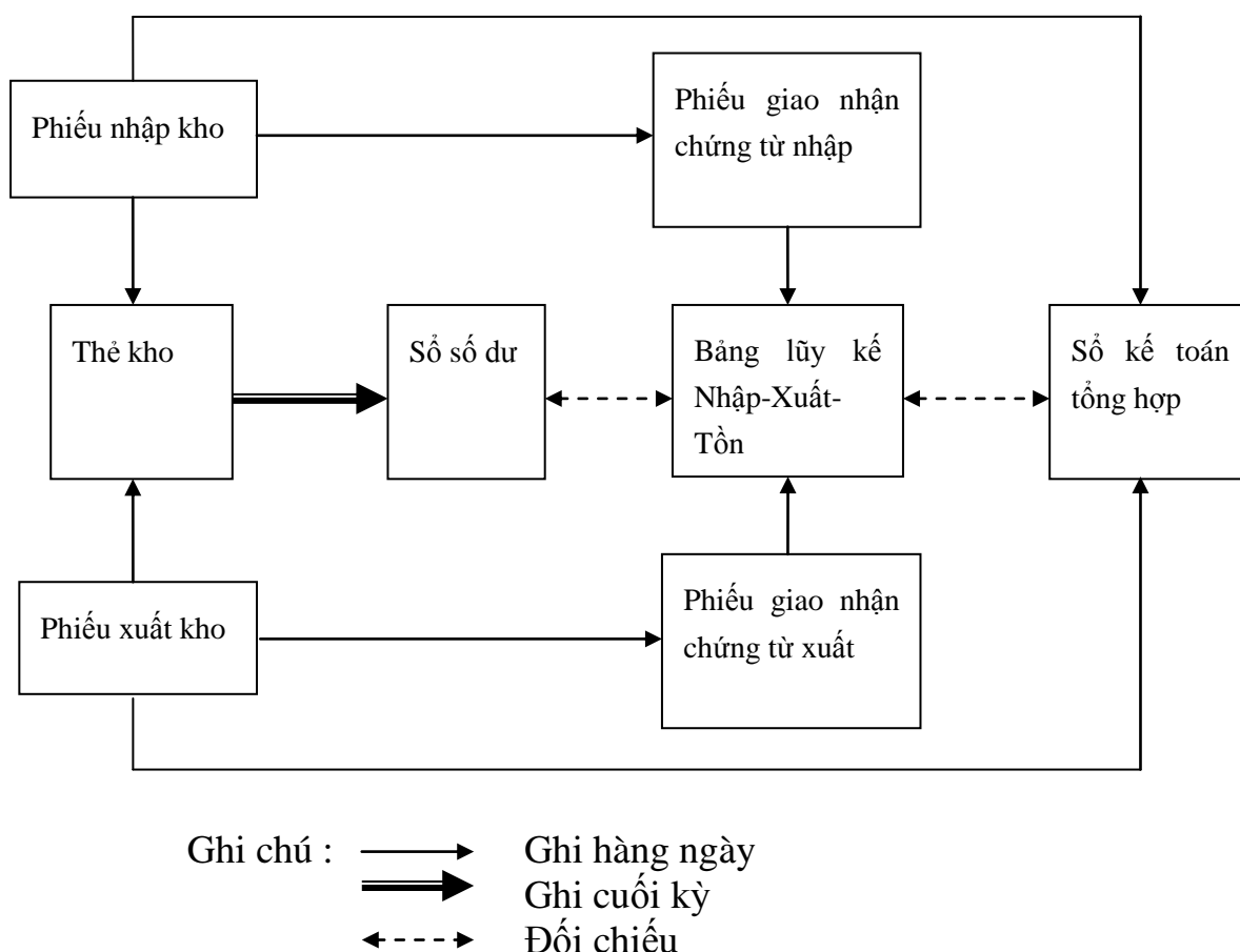
Sơ đồ 1.3: Quy trình hạch toán chi tiết NVL theo phương pháp sổ số dư
