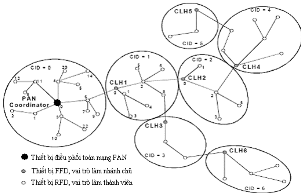
Hình 2.4 Cấu trúc mạng hình cây
