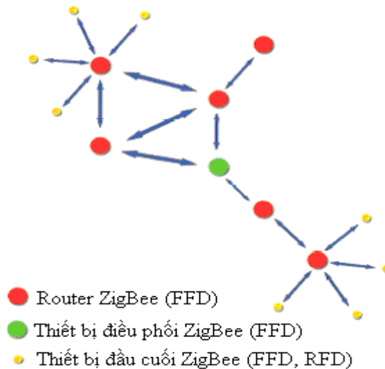
Hình 2.3 Cấu trúc mạng mesh
