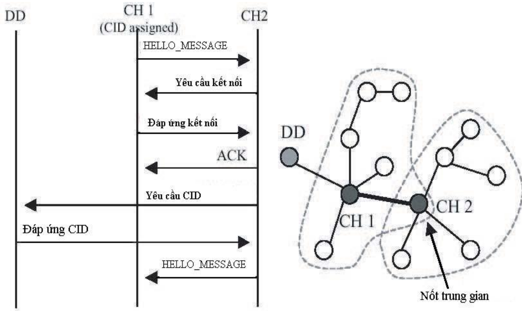
Hình 4.7 Gán địa chỉ nhóm qua nốt gốc
