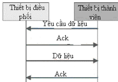
Hình 3.12 kết nối trong mạng không hỗ trợ phát beacon
