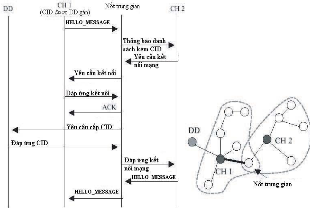
Hình 4.8 Gán địa chỉ nhóm qua nốt gốc và nốt trung gian
