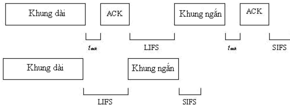
Hình 3.7 Khoảng cách giữa hai khung IFS
