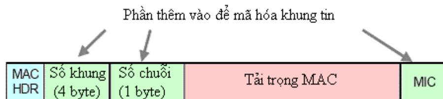
Hình 3.13 Khung tin mã hóa tầng MAC
