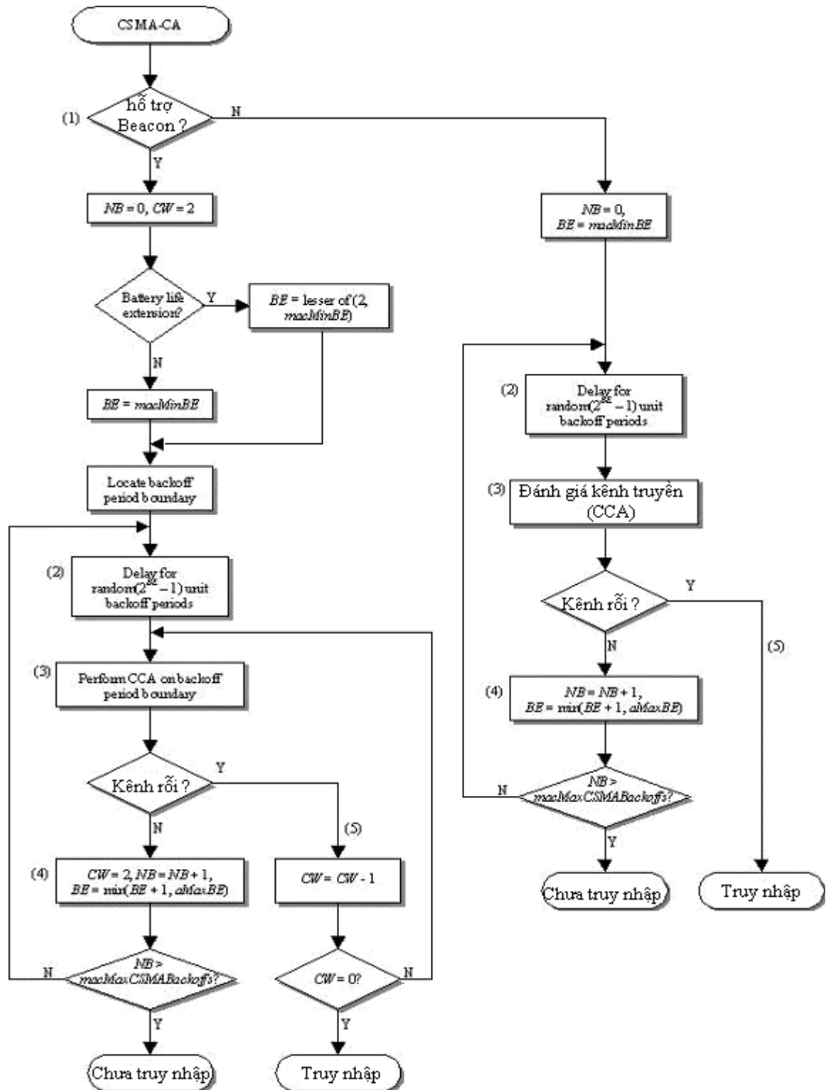
Hình 3.8 Lưu đồ thuật toán
