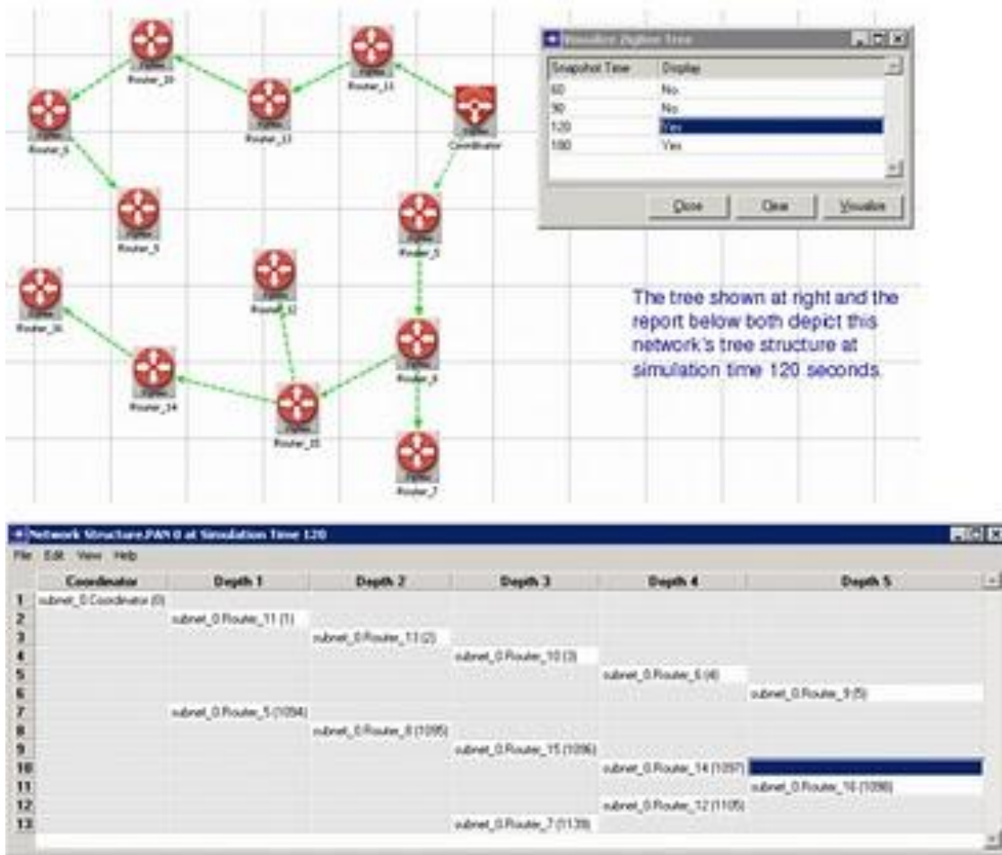
Hình 4.10 Mô phỏng Zigbee với thư viện từ OPNET.
