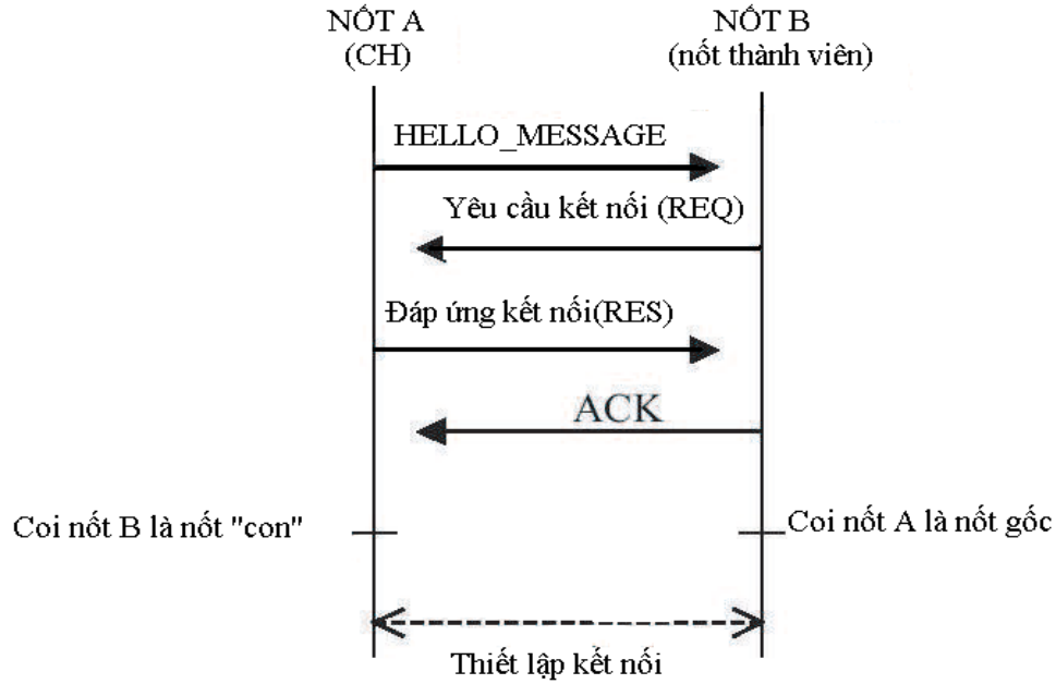
Hình 4.3 Thiết lập kết nối giữa CH và nút thành viên
