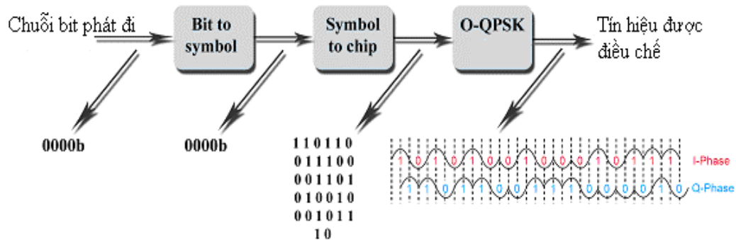
Hình 3.3 Sơ đồ điều chế
