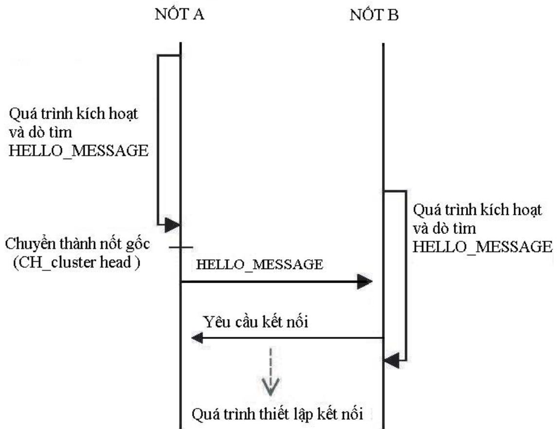
Hình 4.2 Quá trình chọn nốt gốc (CH)
