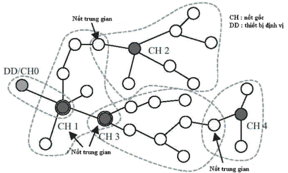
Hình 4.9 Mạng cây đa nhánh và các nốt trung gian
