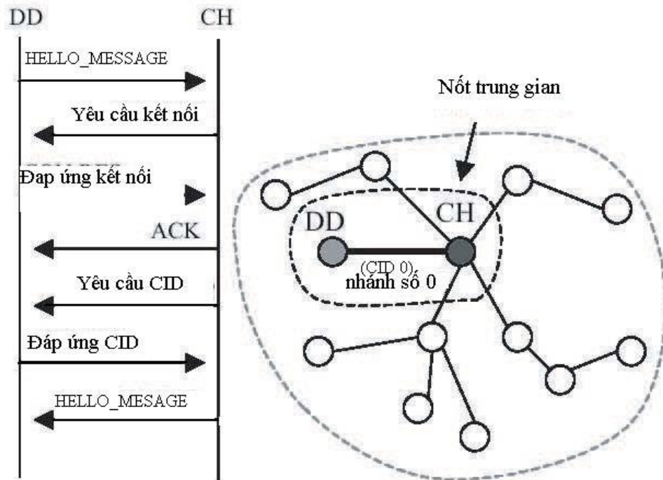
Hình 4.5 Gán địa chỉ nhóm trực tiếp
