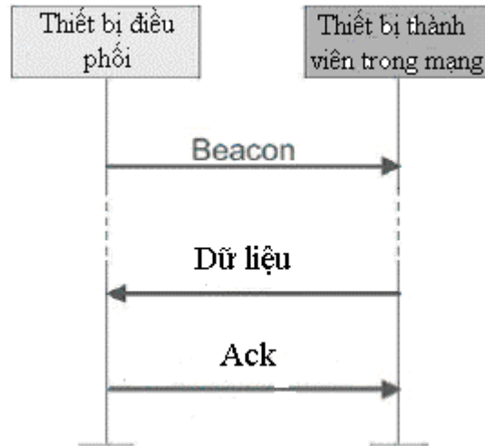
Hình 3.10 liên lạc trong mạng có hỗ trợ beacon.
