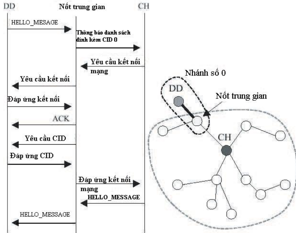
Hình 4.6 Gán địa chỉ nhóm qua nút trung gian
