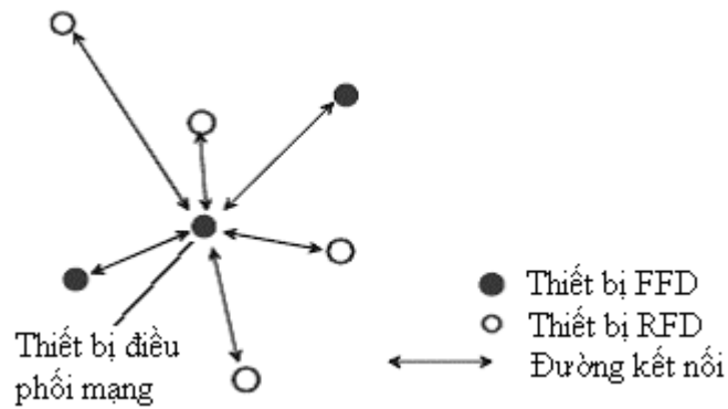
Hình 2.2 Cấu trúc mạng hình sao
