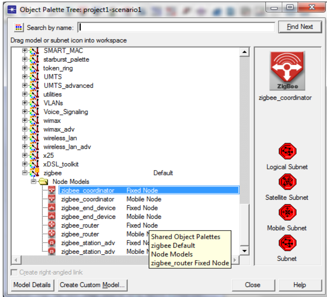
Hình 4.13 Mô tả nút mạng định tuyến của ZigBee trong OPNET.
