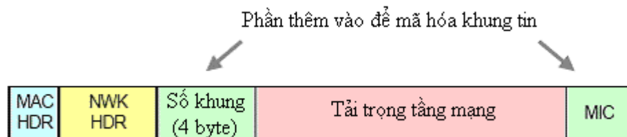
Hình 3.14 Khung tin mã hóa tầng mạng
