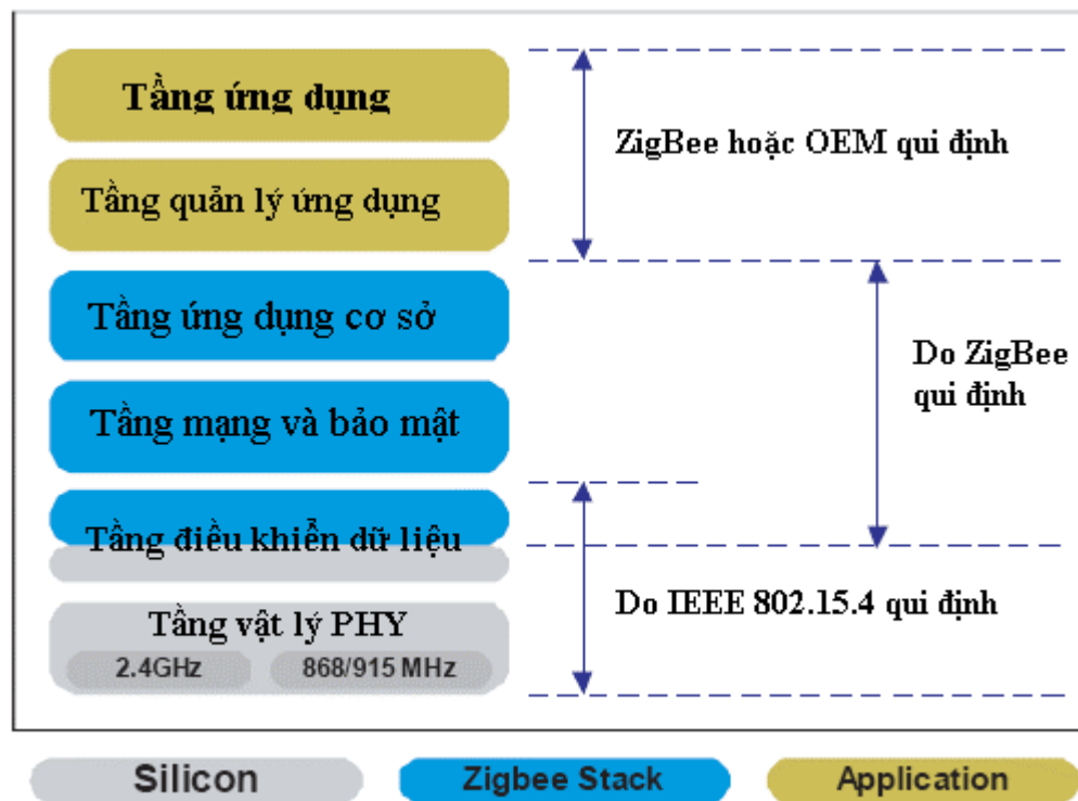
Hình 3.1 Mô hình giao thức của ZigBee
