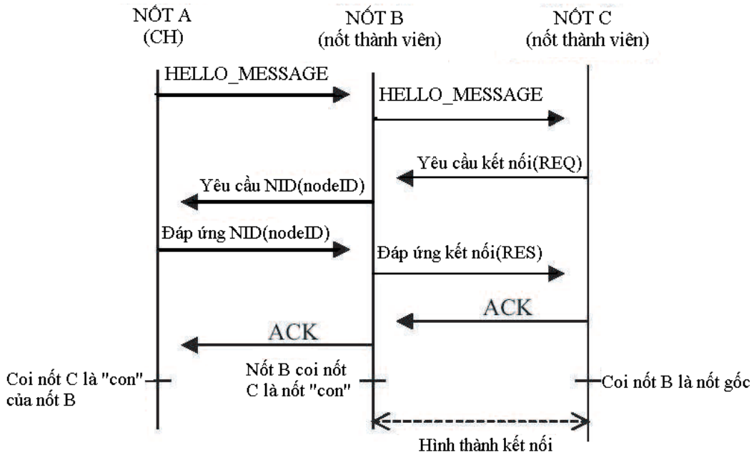
Hình 4.4 Quá trình hình thành nhánh nhiều bậc
