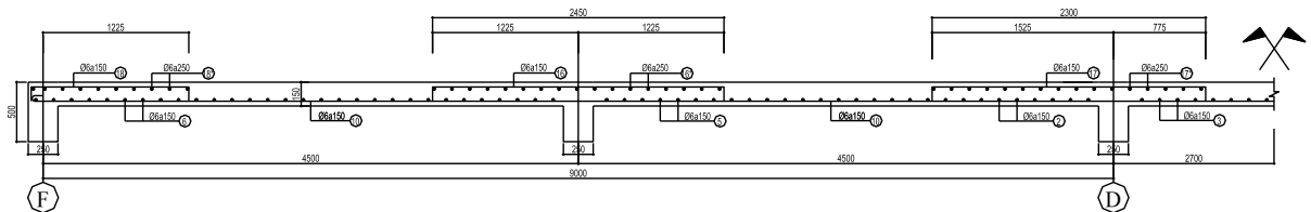
Hình 3.5 Mặt cắt 2-2
