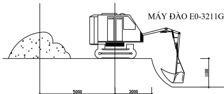
Hình 8.2: Máy đào gầu nghịch
