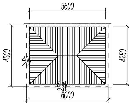
Hình 2.16:Sơ đồ ô truyền tải 1
