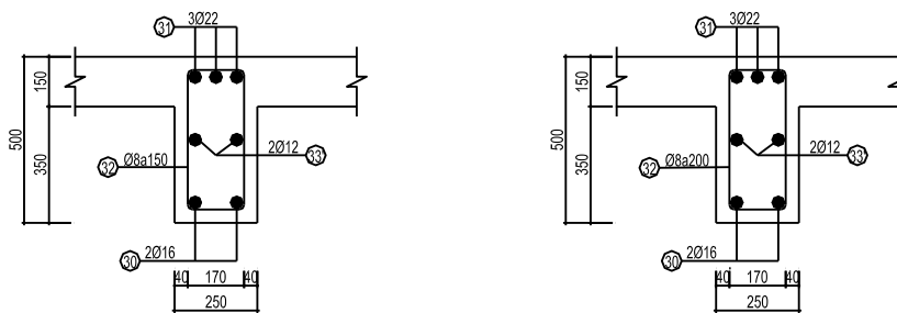
Hình 4.6: Mặt cắt dầm
