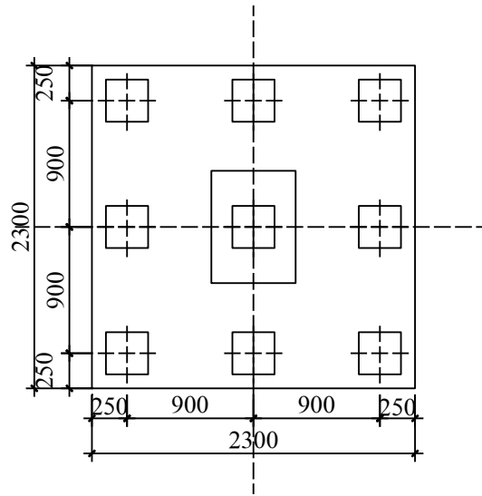
Hình 7.2: Sơ đồ bố trí cọc trong mặt bằng
