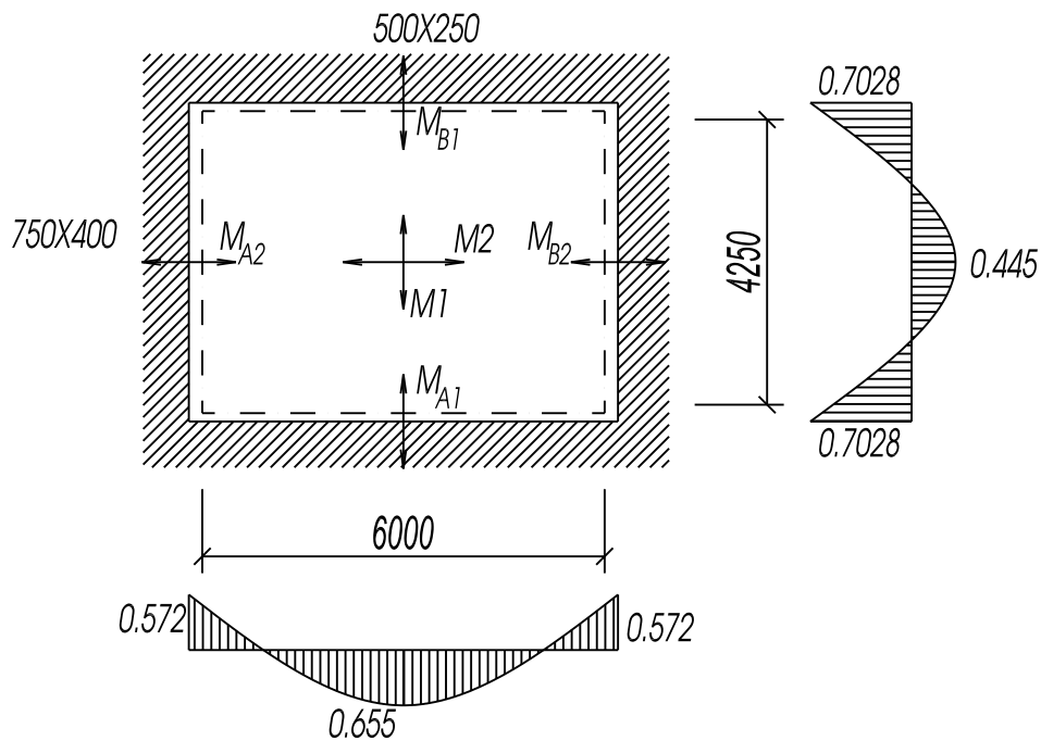
Hình 3.1 Sơ đồ tính toán ô sàn S1
