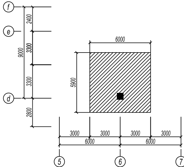
Hình 2.1: Diện tích dồn tải lên cột
