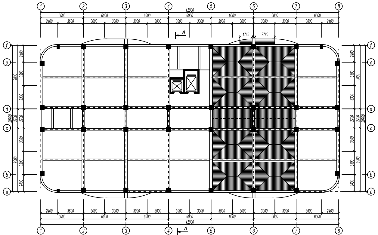
Hình 2.4: Sơ đồ truyền tải lên khung 2-2 sàn tầng mái
