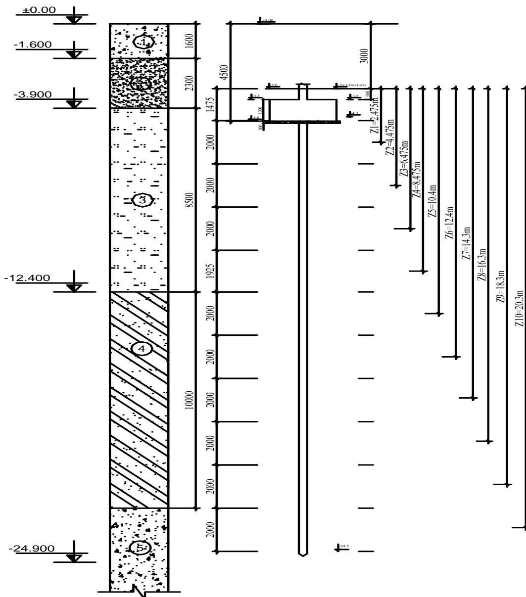
Hình 7.1: Sơ đồ tính sức chịu tải của cọc
