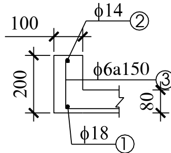
Hình 6.5: Mặt cắt cốt thang
