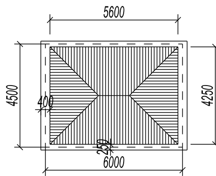
Hình 2.5: Sơ đồ 1 ô truyền tải
