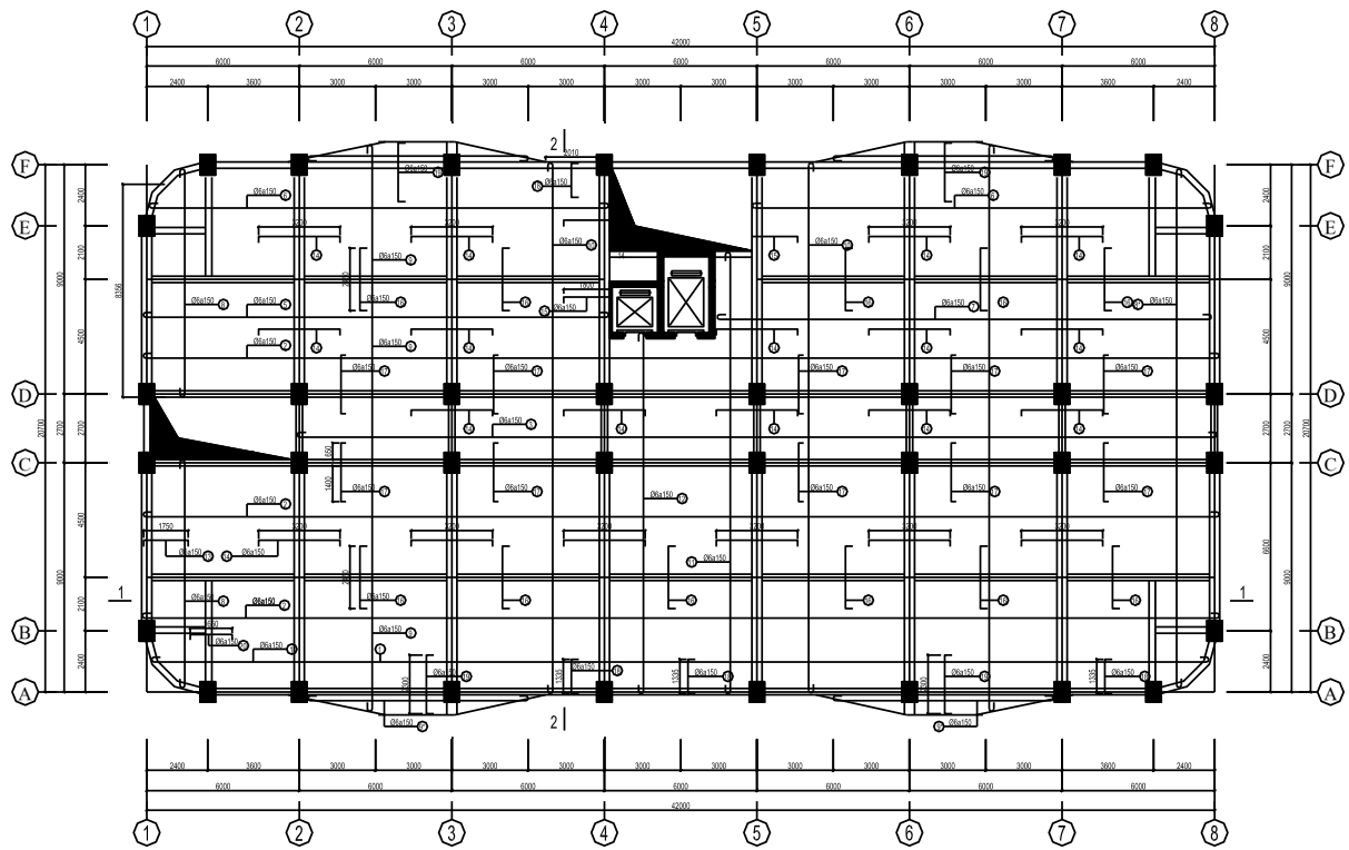
Hình 3.3 Bố trí thép sàn tầng điển hình
