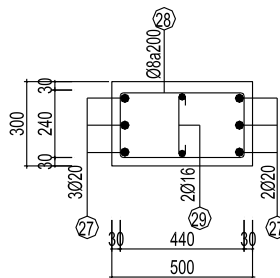
Hình 5.1: Mặt cắt 9-9
