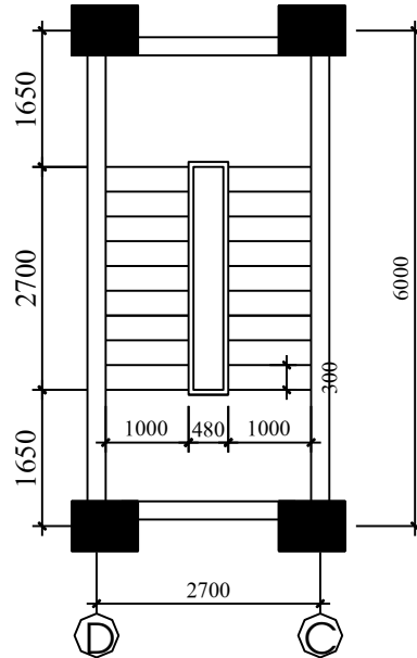
Hình 6.1: Mặt bằng kết cấu thang
