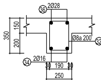
Hình 4.2 Mặt cắt dầm
