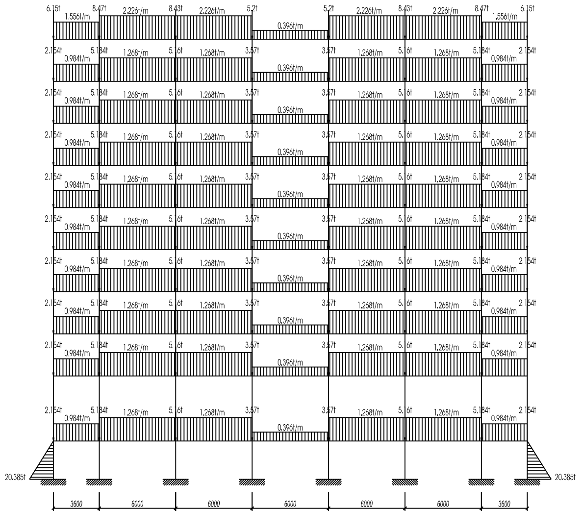
Hình 2.37: Tĩnh tải khung F-F
