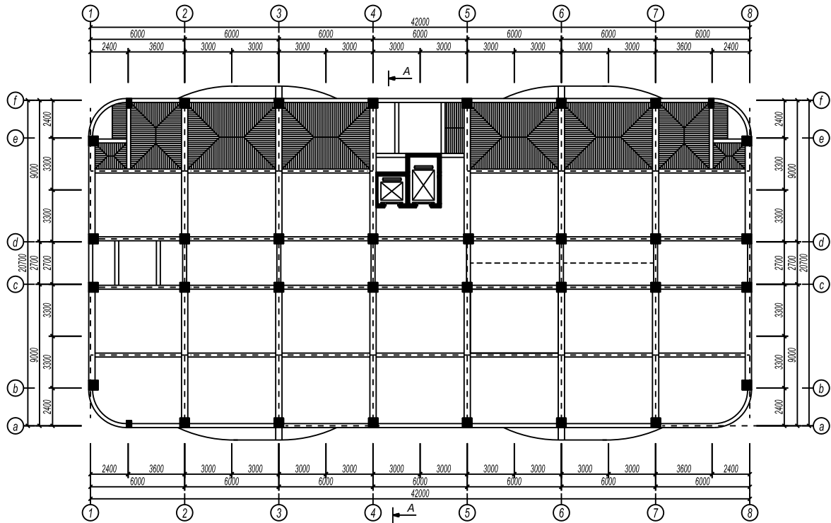
Hình 2.31:Sơ đồ truyền tải lên khung F-F sàn tầng mái
