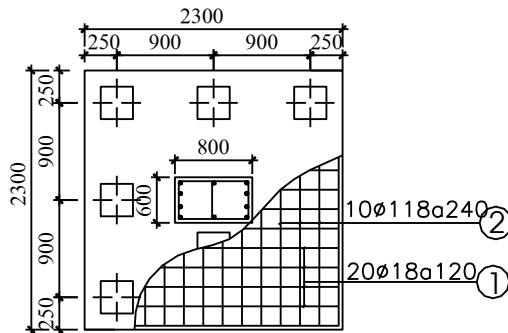
Hình 7.6: Bố trí cốt thép trong đài
