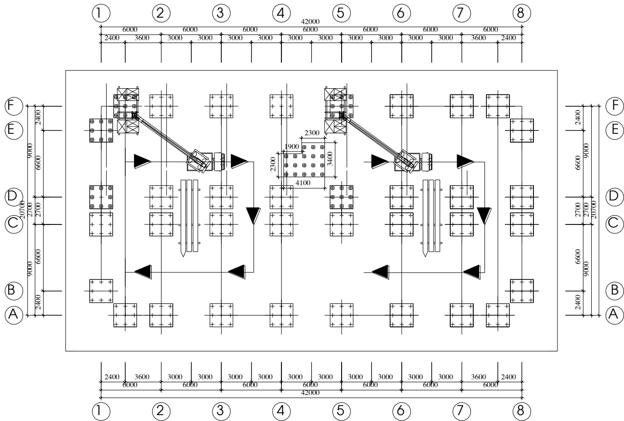
Hình 8.8: Sơ đồ ép cọc toàn móng
