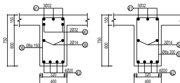
Hình 4.5 Mặt cắt dầm
