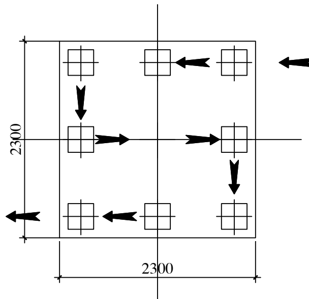
Hình 8.6:Sơ đồ ép cọc móng M1
