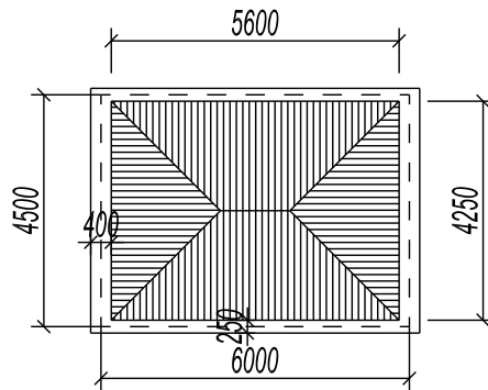
Hình 2.32:Sơ đồ ô truyền tải 1
