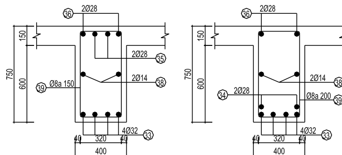
Hình 4.1 Mặt cắt dầm
