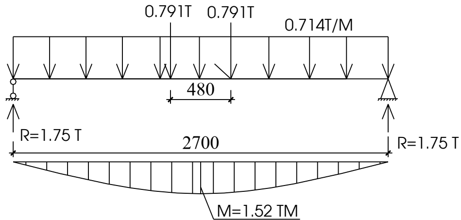
Hình 6.8: Sơ đồ tính dầm thang
