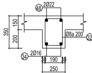
Hình 4.4 Mặt cắt dầm
