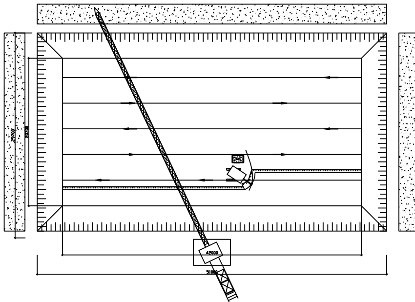
Hình 8.4: Mặt bằng thi công đào đất lớp 2
