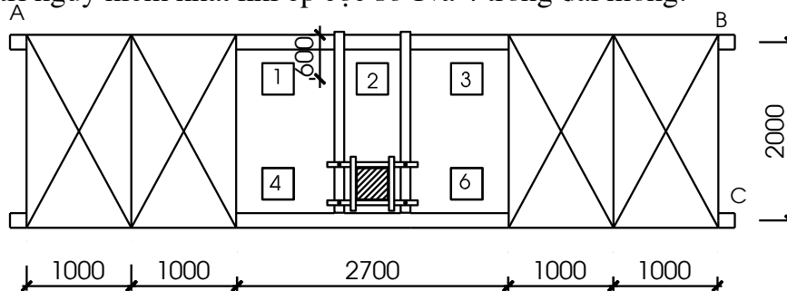
Hình 8.5: Sơ đồ bố trí đối trọng
