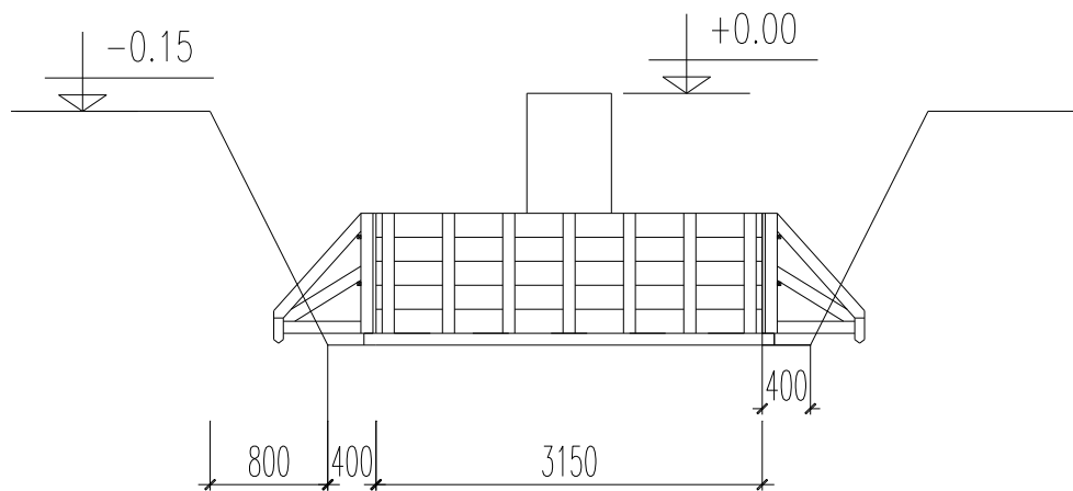
MẶT CẮT VÁN KHUÔN MÓNG
