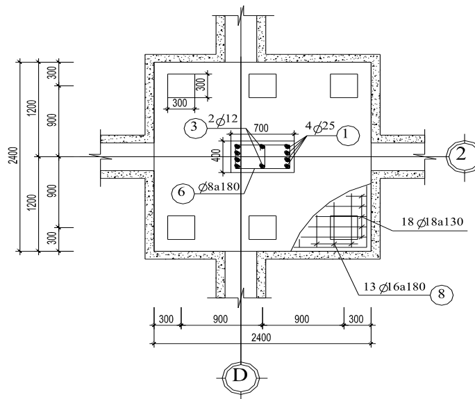
CỘT THÉP ĐÀI CỌC MÓNG M2
