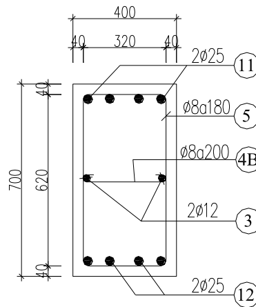
MẶT CẮT CỘT 2 TRỤC D
