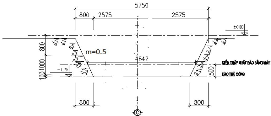
MẶT CẮT DỌC HỐ MÓNG M1( TRỤC C, F)
