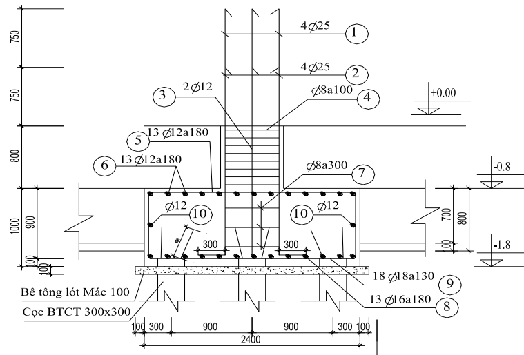
CỘT THÉP ĐÀI CỌC MÓNG M2
