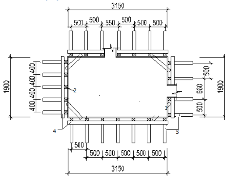
MẶT BẰNG MÓNG MI
