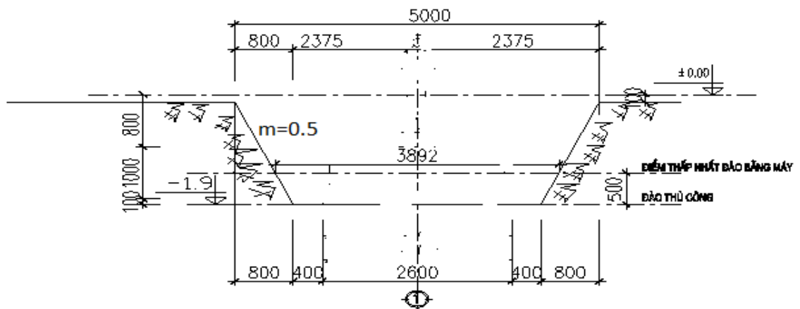
MẶT CẮT NGANG HỒ MÓNG M2( TRỤC D, E)
