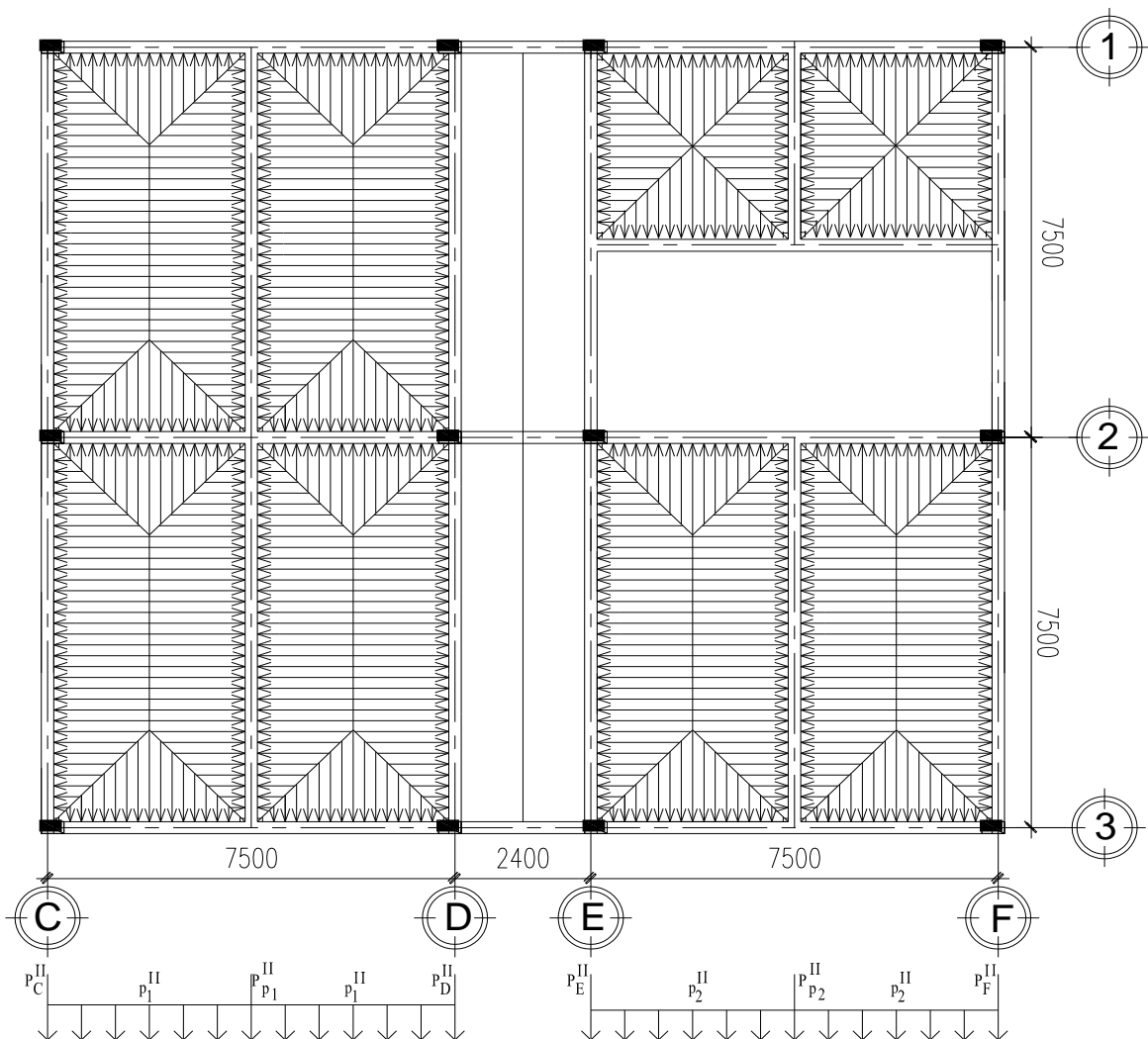
MẶT BẰNG PHÂN BỐ HOẠT TẢI 2 TẦNG 2,4,6
