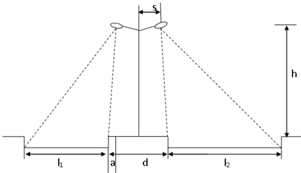
Hình 4.1: Biểu diễn cột đèn chiếu sáng trên toàn bộ tuyến đường Các thông số kỹ thuật:
