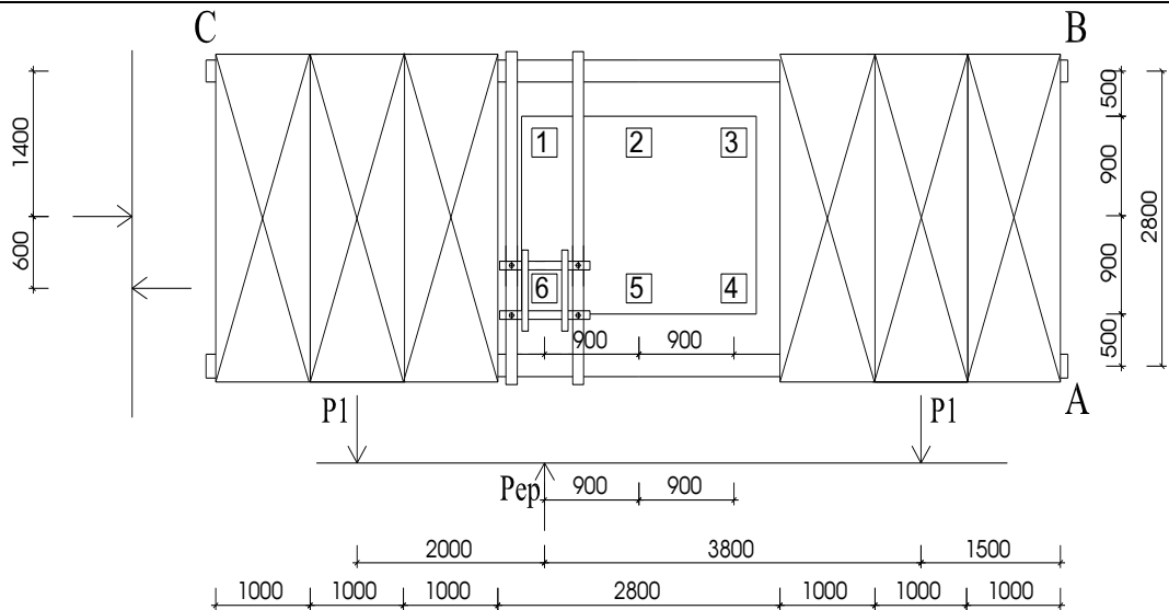
Hình 3: Mặt bằng bố trí đôi trọng ép cọc
