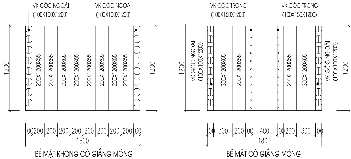
Hình 9: Tổ hợp ván khuôn các cạnh của móng M2
