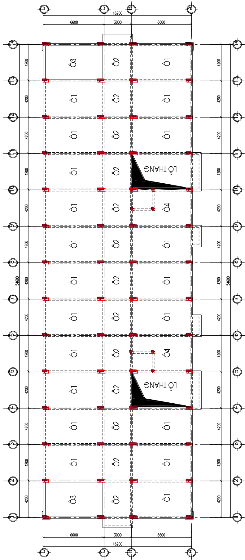
Mặt bằng kết cấu ô sàn tầng điển hình
