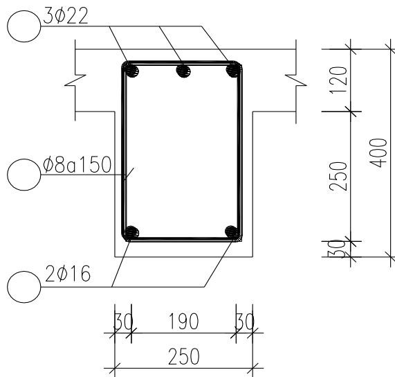
CẮT DẪM 54
