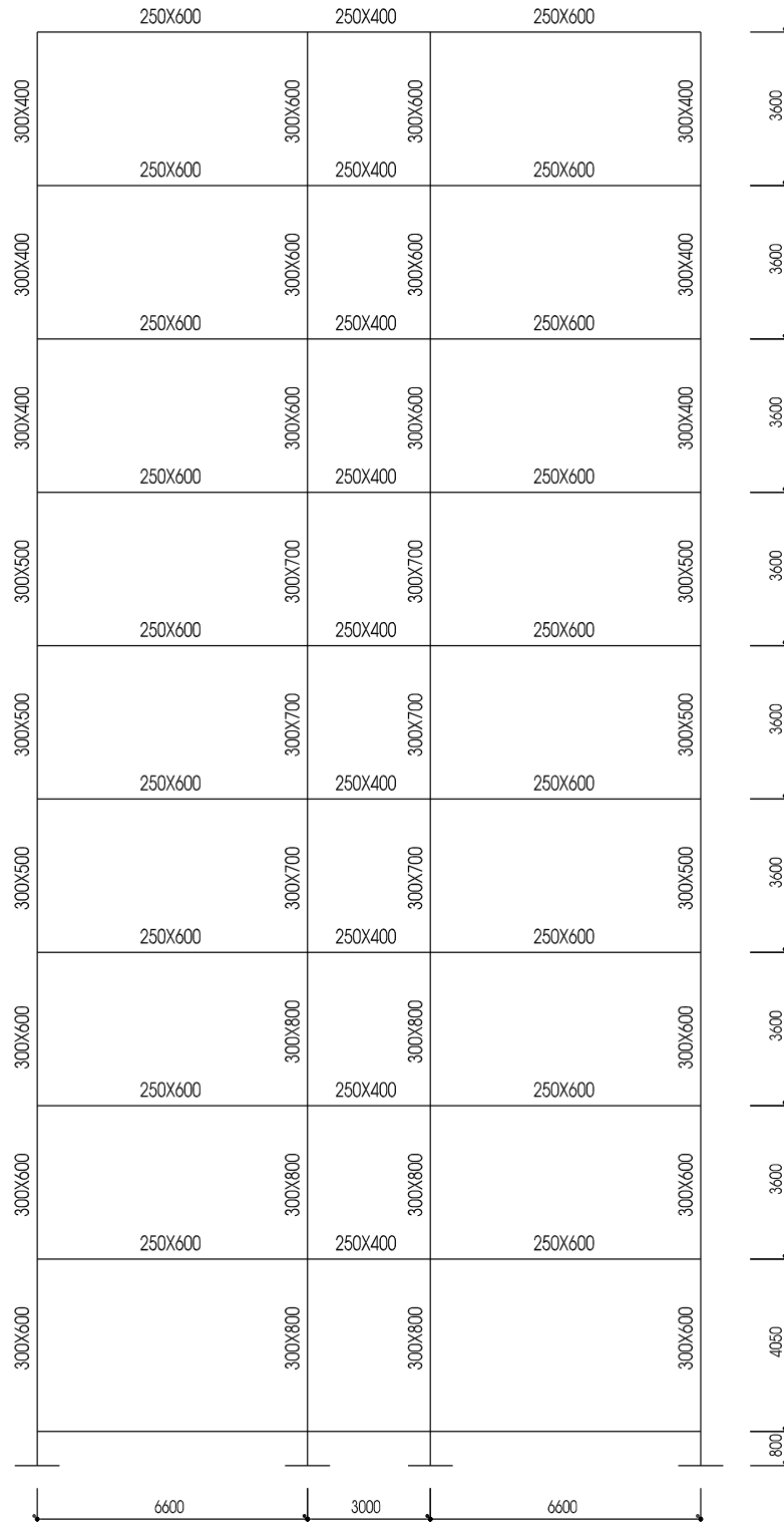
SƠ ĐỒ HÌNH HỌC KHUNG K3 - TRUC3
