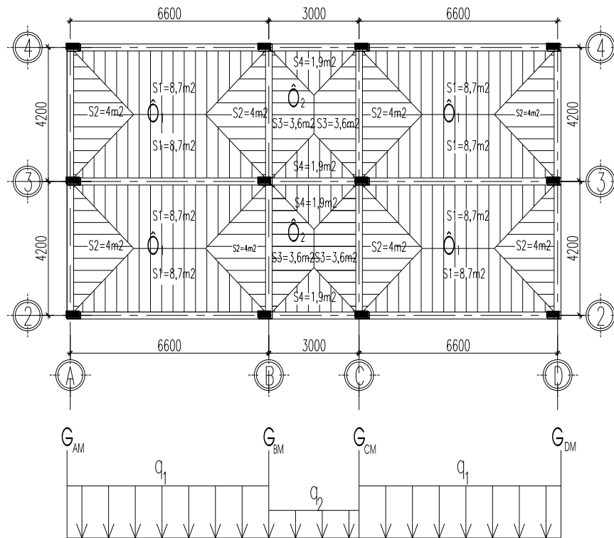
MẶT BẰNG PHÂN TẢI TẦNG MÁI
