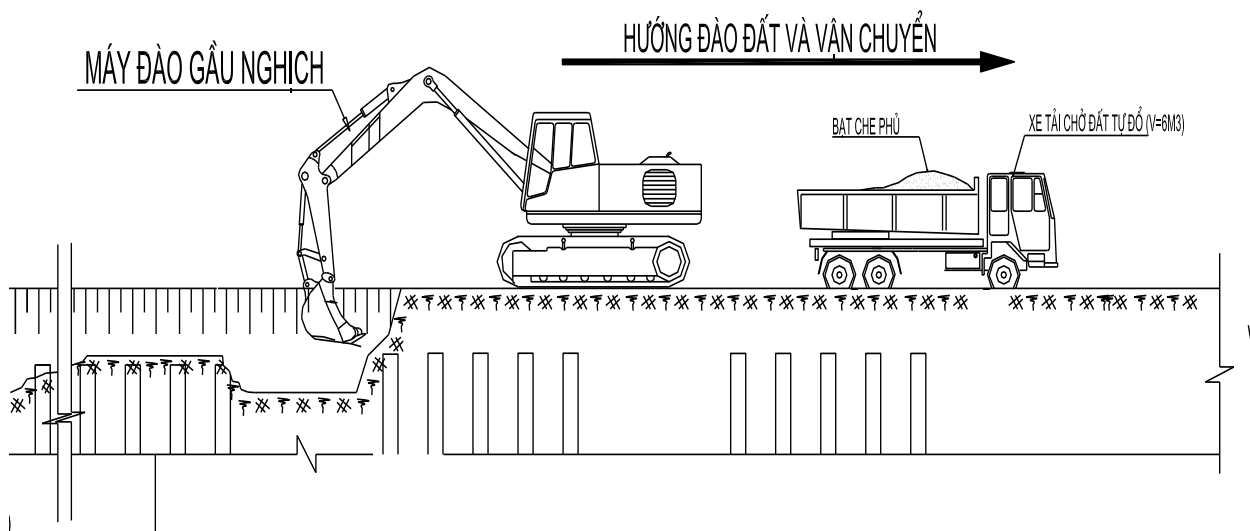
Hình 6: Thi công đào đất bằng máy
